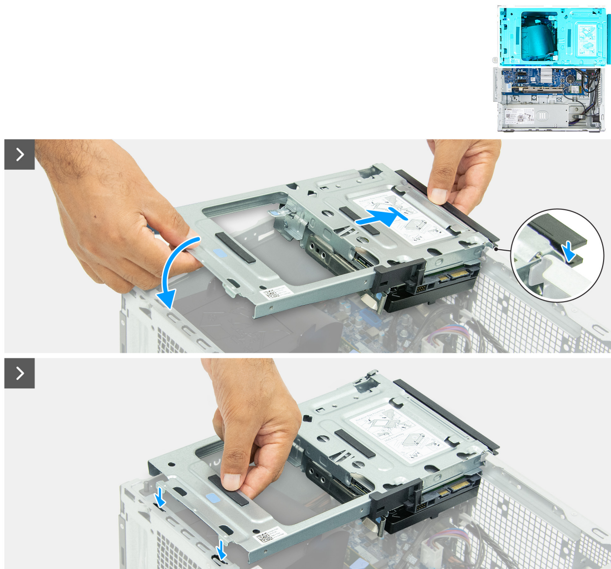
Obrázek 40. Montáž pozice pro disk
