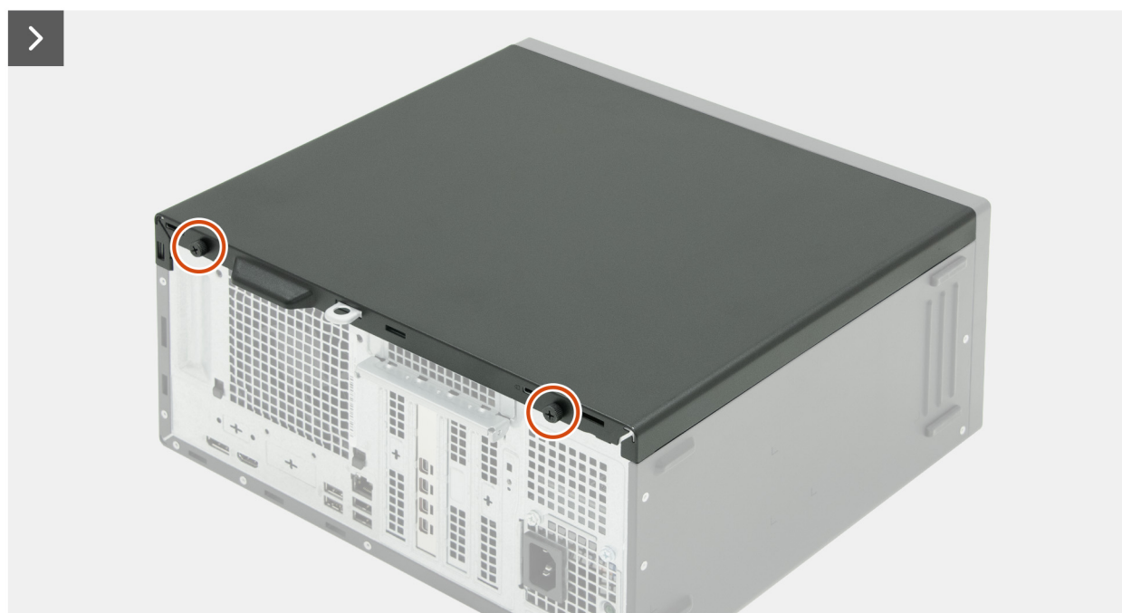
Obrázek 9. Demontáž levého bočního krytu
