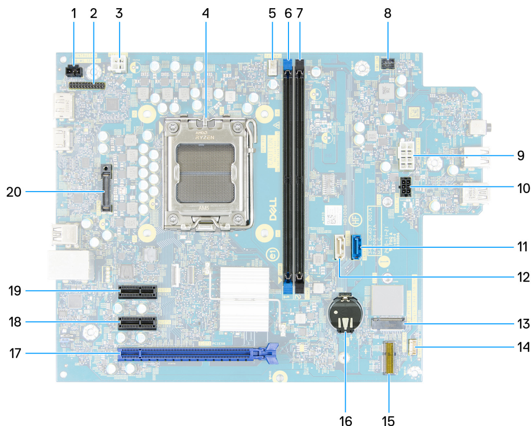
Obrázek 66. Popisky základní desky
