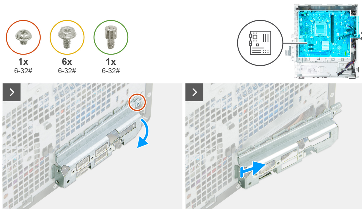
Obrázek 67. Demontáž základní desky
