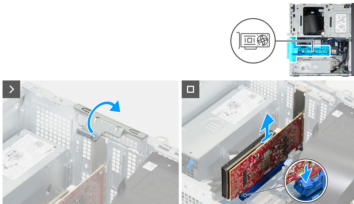
Obrázek 30. Demontáž grafické karty
