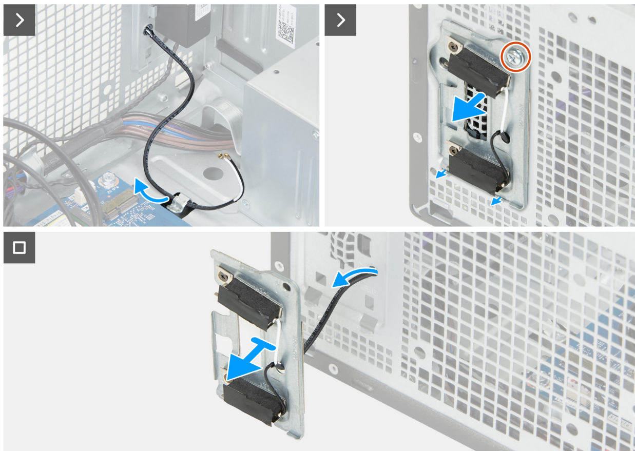
Obrázek 56. Demontáž anténních modulů
