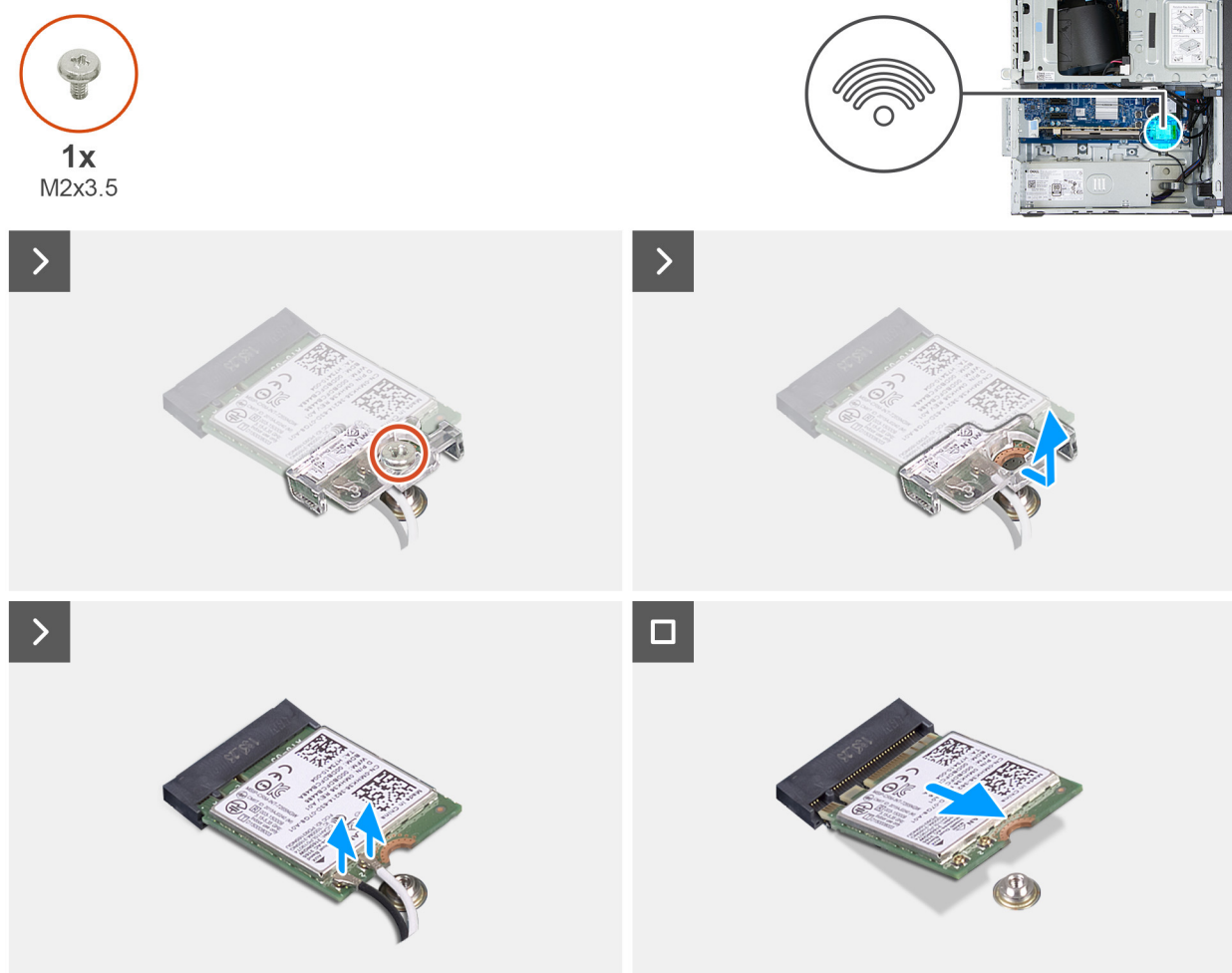
Obrázek 32. Demontáž bezdrátové karty
