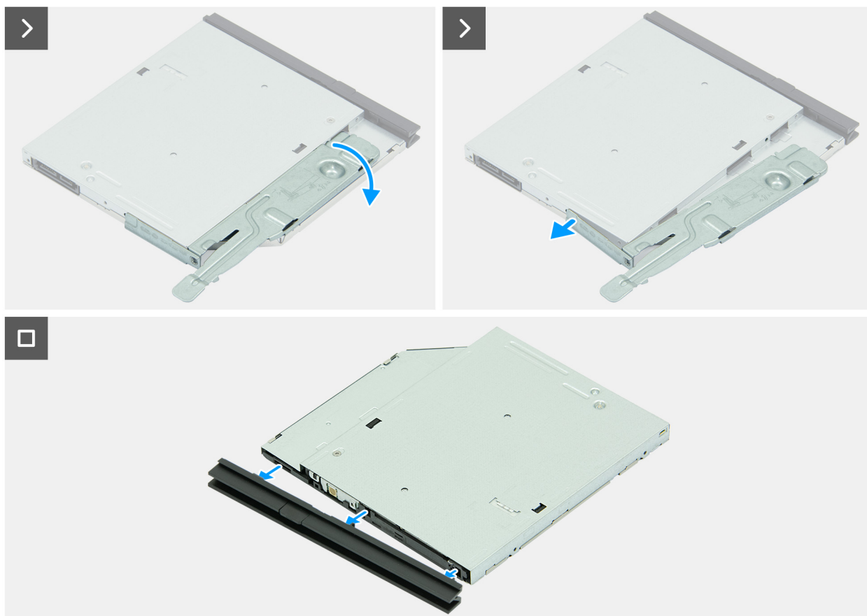
Obrázek 35. Vyjmutí optické jednotky
