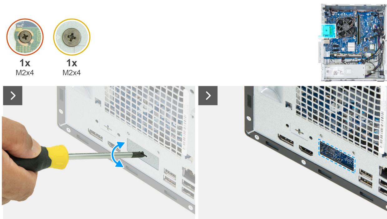
Obrázek 49. Montáž modulu volitelného portu
