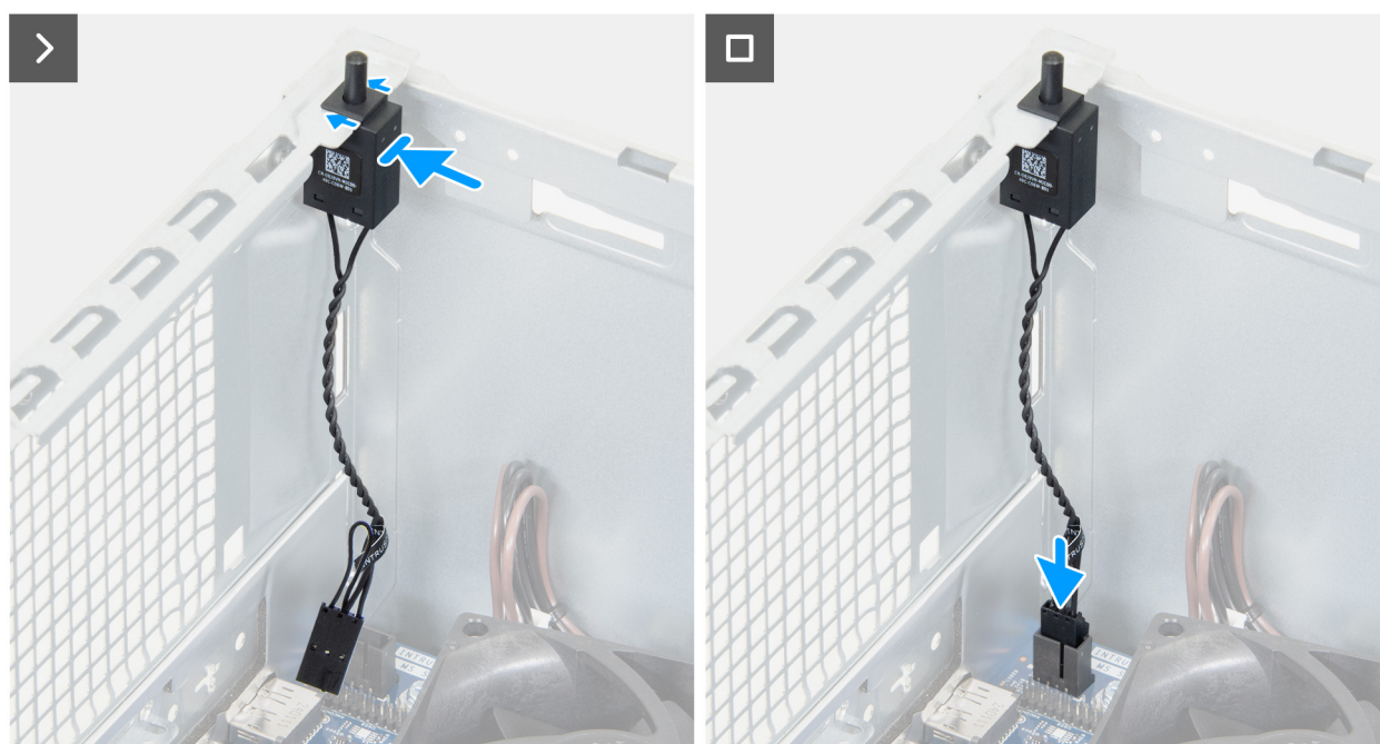
Obrázek 45. Montáž spínače detekce vniknutí do šasi
