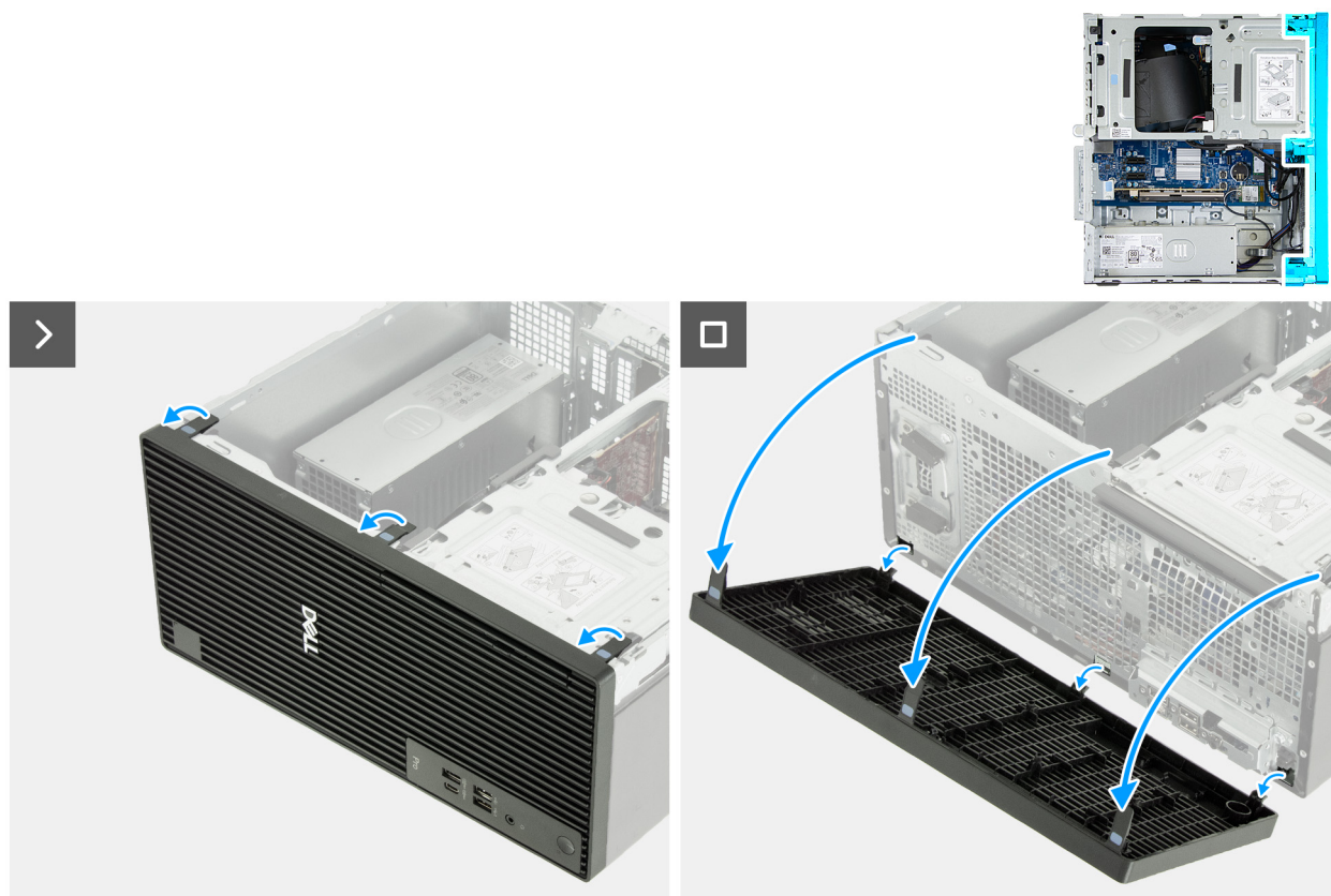
Obrázek 19. Demontáž čelního krytu
