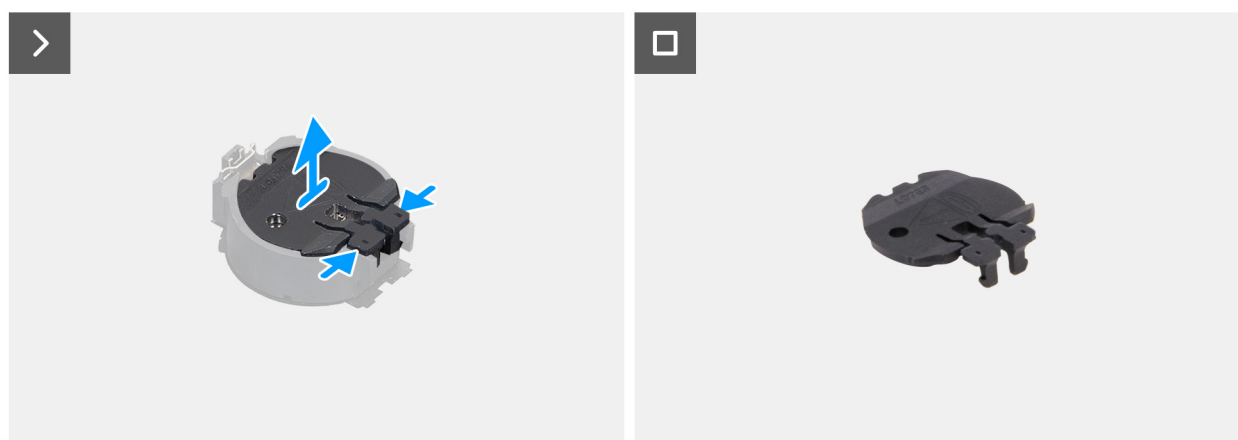
Obrázek 13. Demontáž krytu knoflíkové baterie
