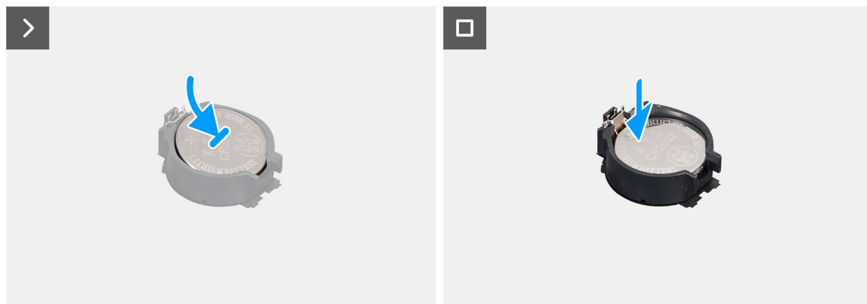
Obrázek 16. Montáž knoflíkové baterie
