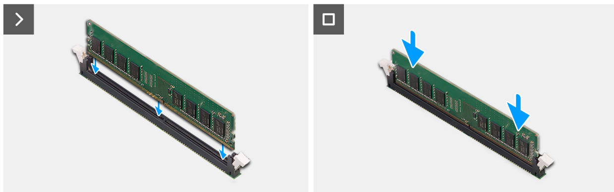
Obrázek 24. Instalace paměti
