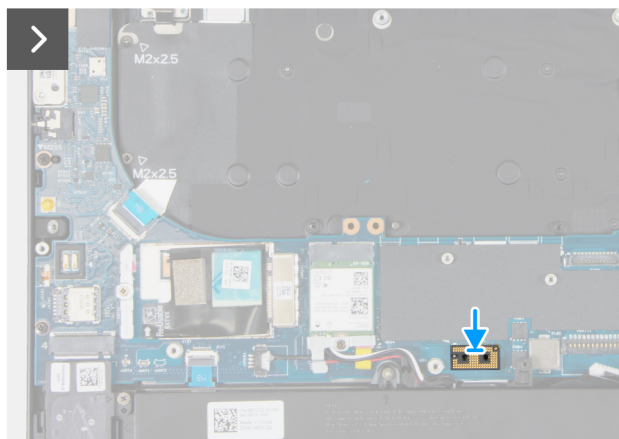
Rysunek 72. Instalowanie płyty zasilania
