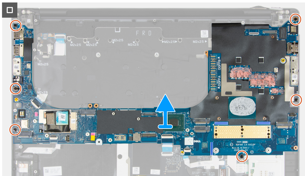
Rysunek 110. Wymontowywanie płyty głównej
