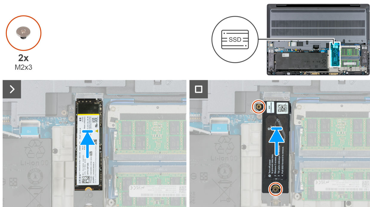
Rysunek 37. Instalowanie dysku SSD M.2 2280 w gnieździe 3 (SSD3)
