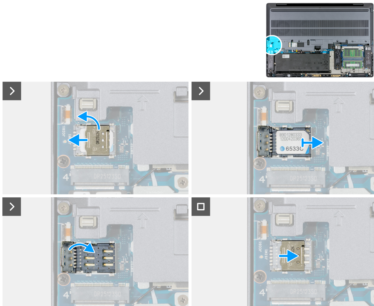
Rysunek 50. Wymontowywanie karty sieci SIM
