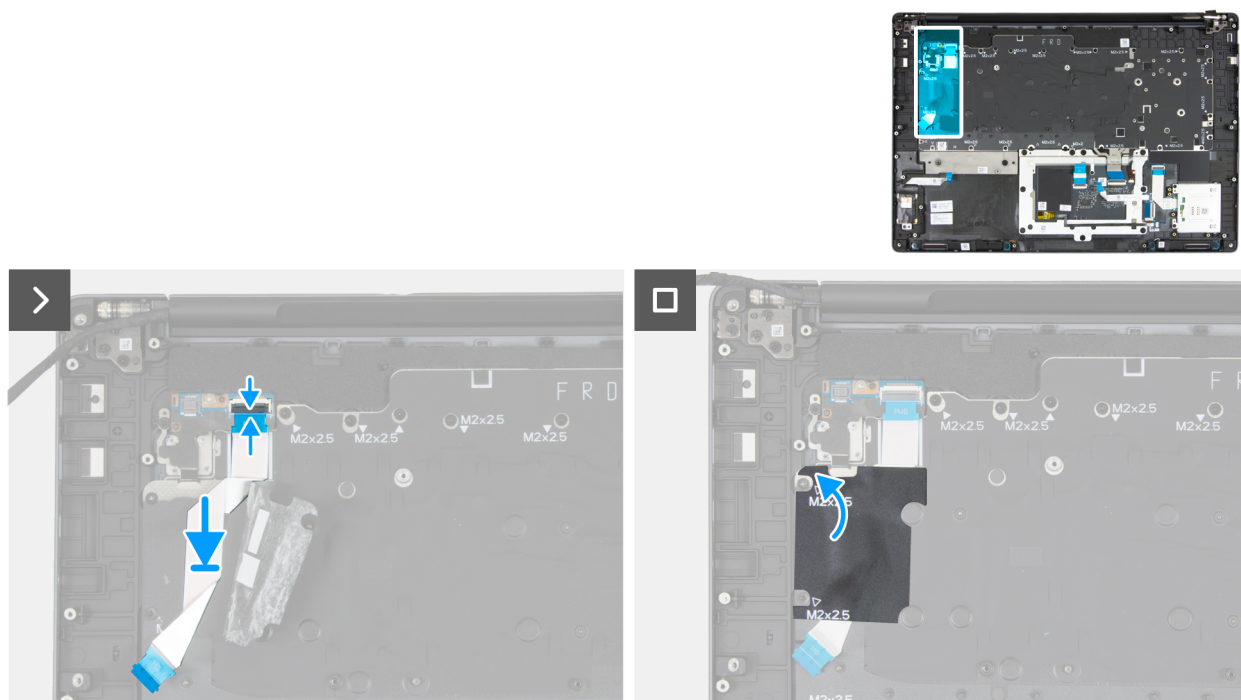
Rysunek 126. Instalowanie płyty przycisku zasilania
