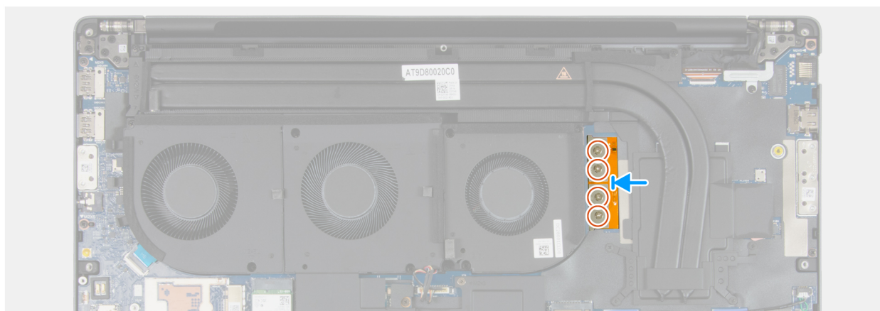
Rysunek 58. Instalowanie zintegrowanego złącza płaskiego FPC
