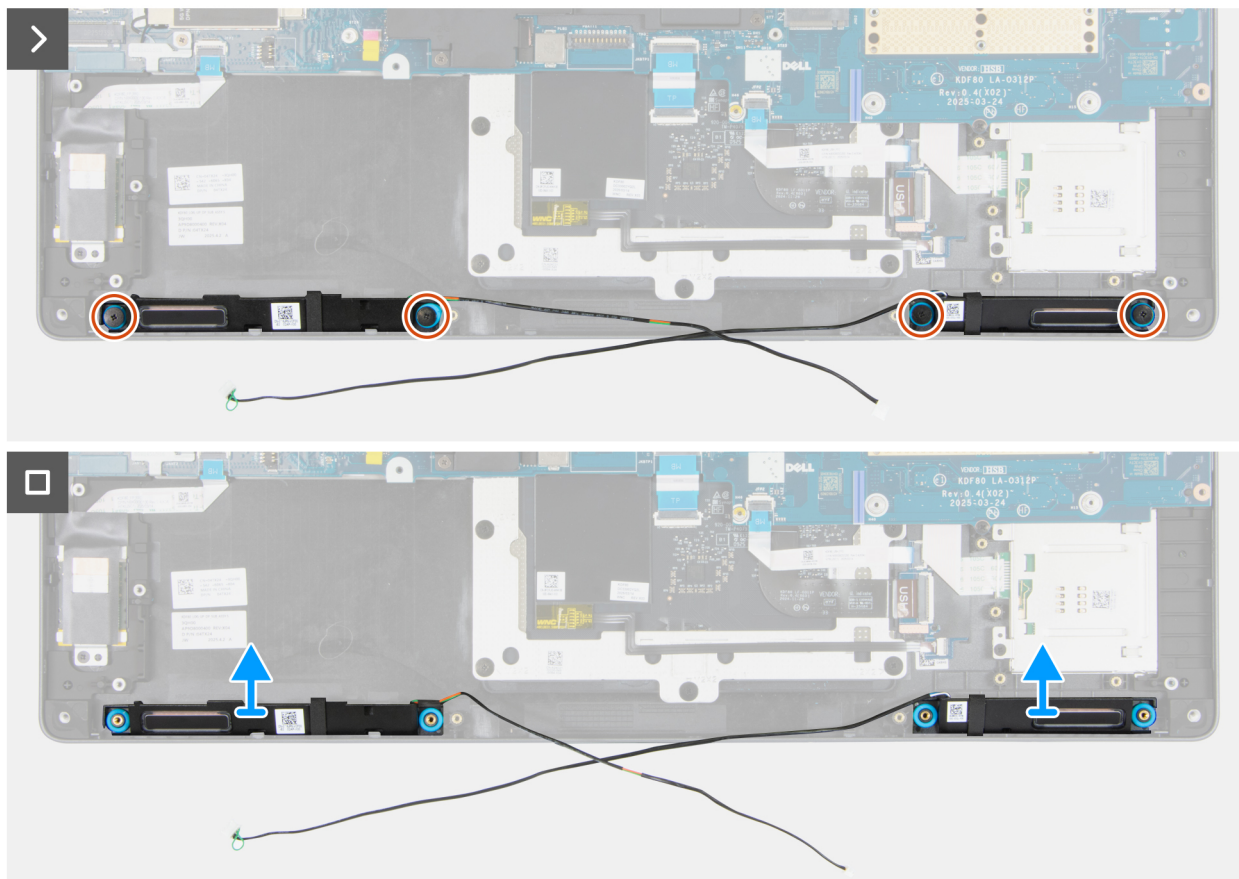
Rysunek 81. Wymontowywanie głośników
