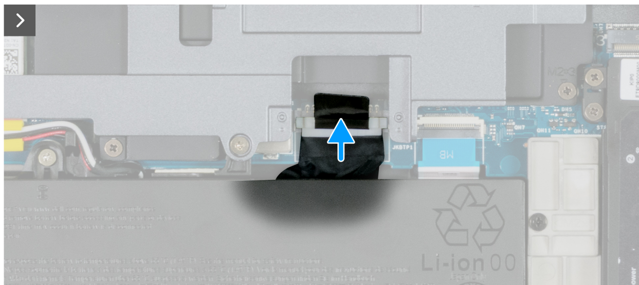
Rysunek 21. Podłączanie kabla baterii
