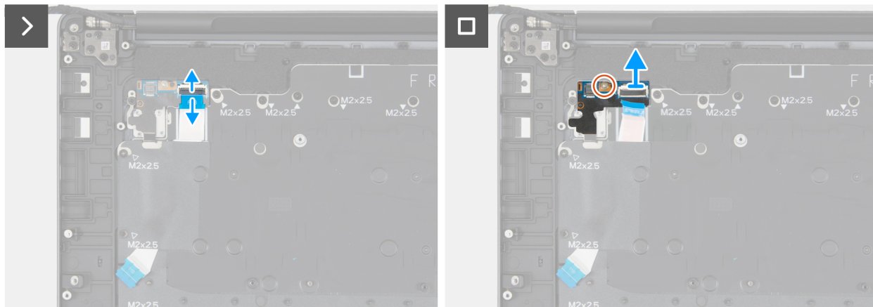
Rysunek 127. Wymontowywanie płyty przycisku zasilania
