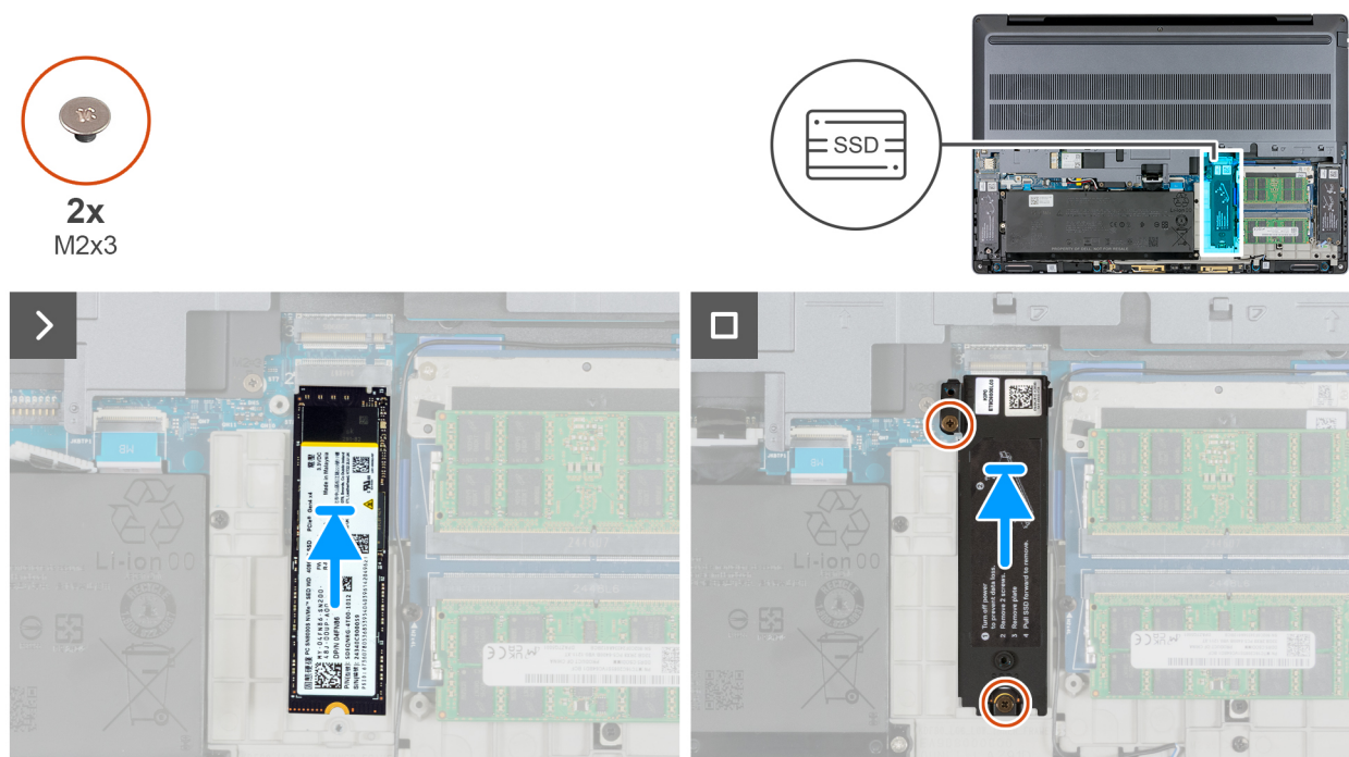
Rysunek 39. Instalowanie dysku SSD M.2 2280 w gnieździe 2 (SSD2)
