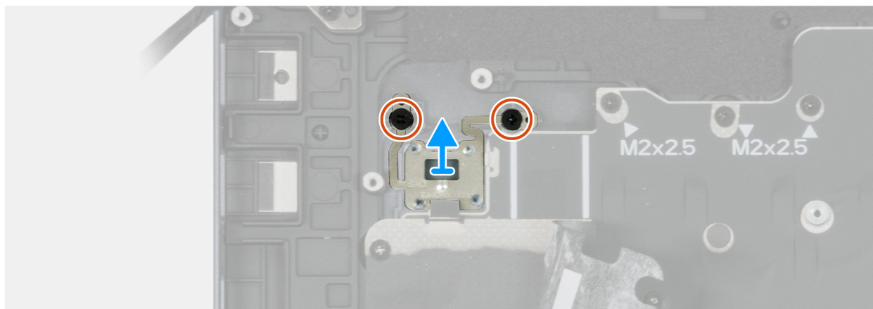
Rysunek 129. Wymontowywanie przycisku zasilania
