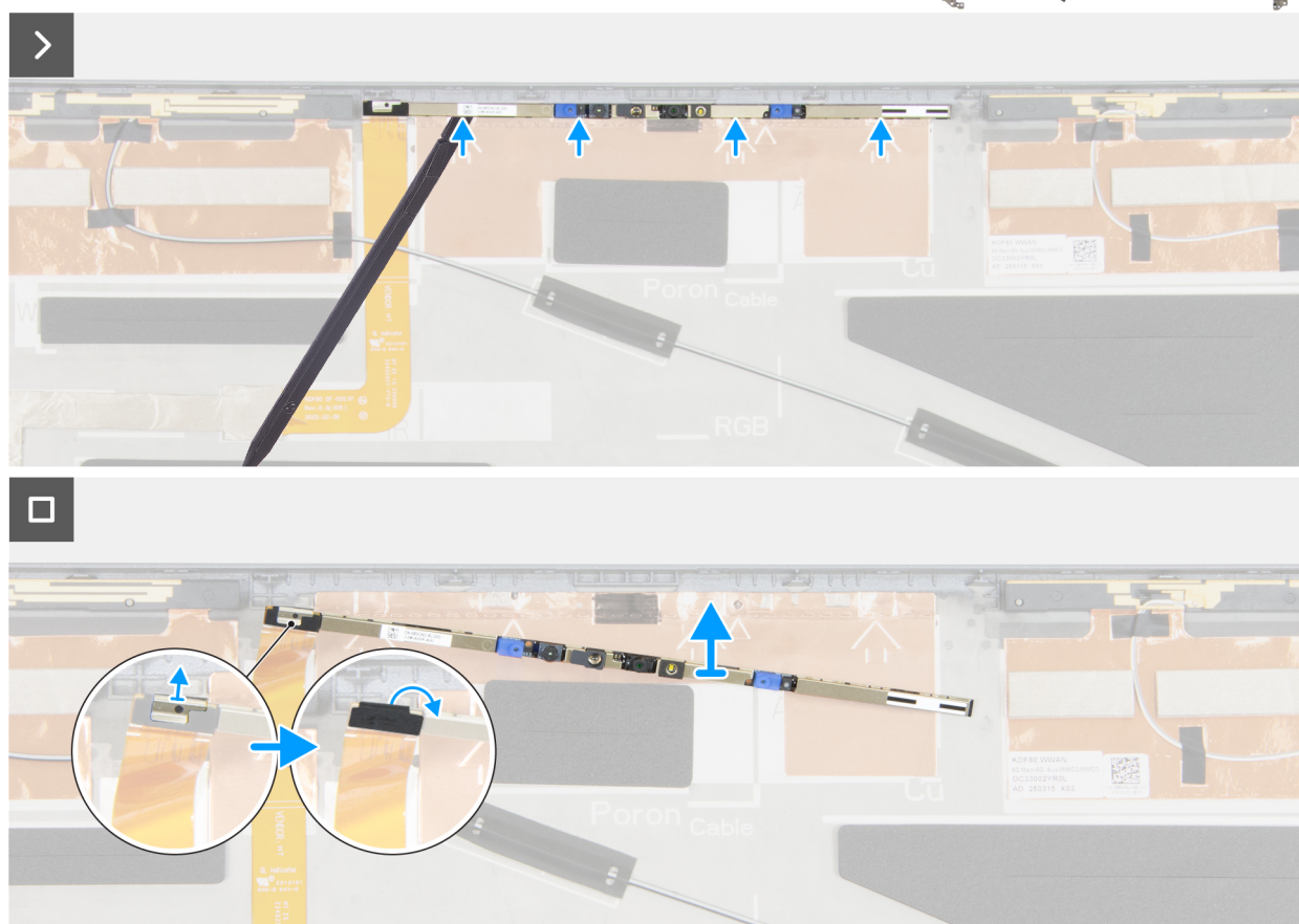
Rysunek 103. Wymontowywanie modułu kamery
