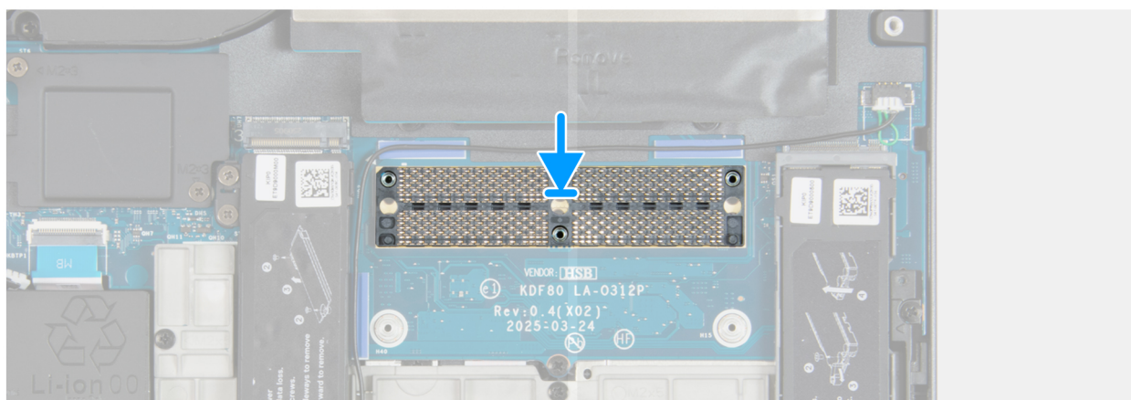
Rysunek 70. Instalowanie złącza pamięci
