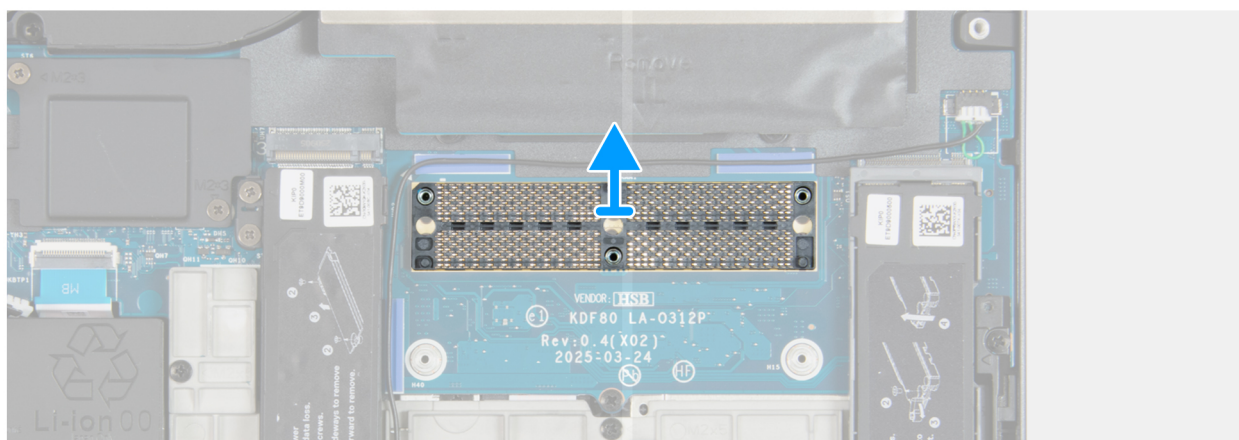
Rysunek 69. Wymontowywanie złącza pamięci
