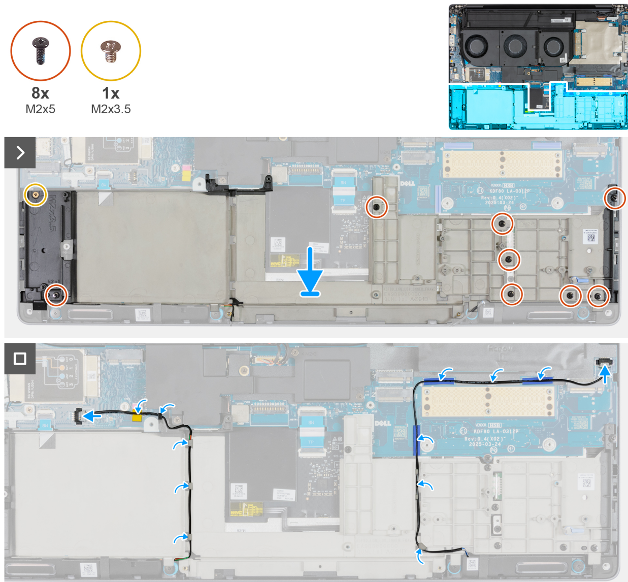
Rysunek 80. Instalowanie ramy wewnętrznej
