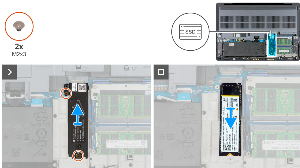
Rysunek 36. Wymontowywanie dysku SSD M.2 2280 z gniazda 3 (SSD3)
