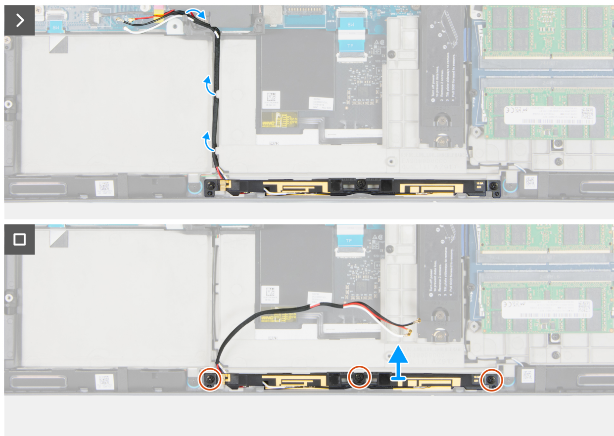
Rysunek 77. Wymontowywanie modułu anteny sieci WLAN
