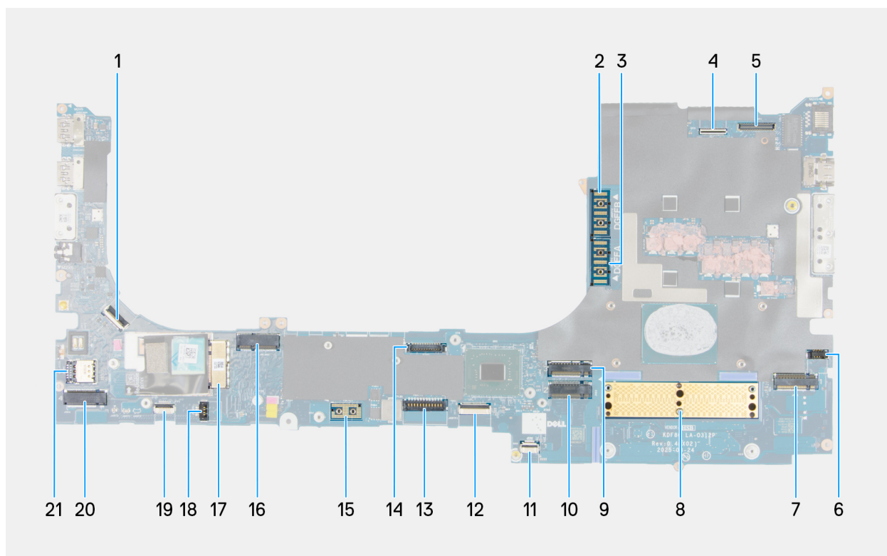
Rysunek 108. Elementy płyty głównej
