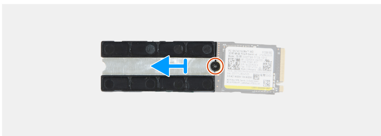
Rysunek 42. Wymontowywanie dysku SSD M.2 2230
