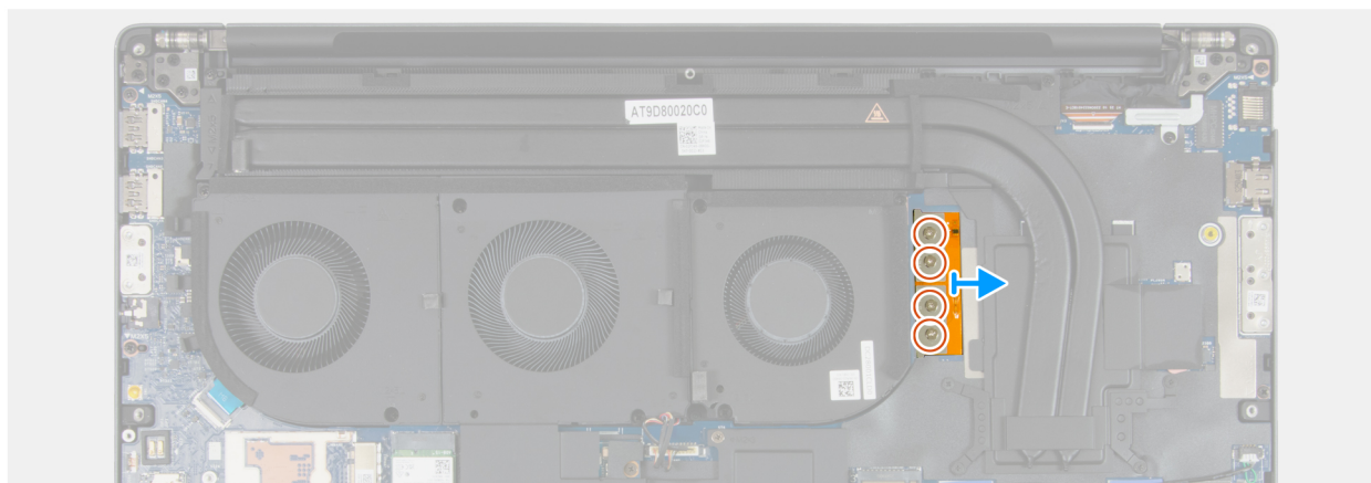
Rysunek 57. Wymywanie zintegrowanego złącza płaskiego FPC
