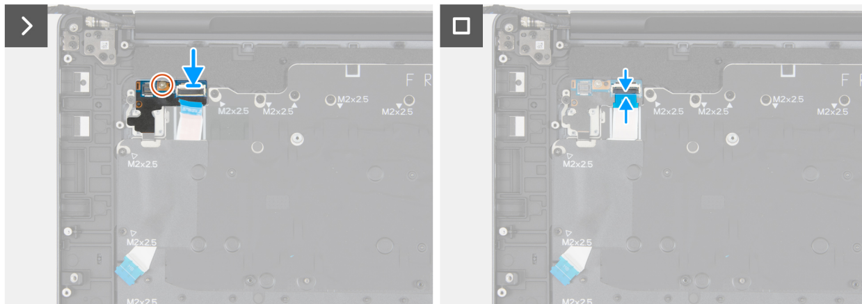
Rysunek 128. Instalowanie płyty przycisku zasilania
