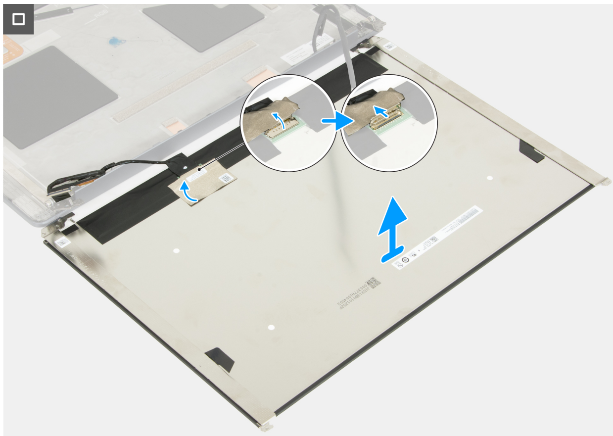
Rysunek 96. Wymontowywanie wyświetlacza
