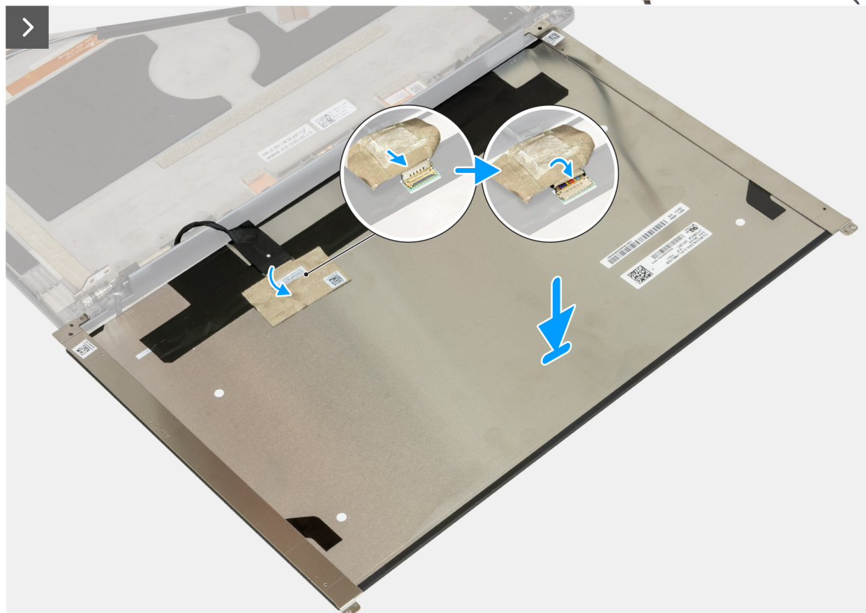
Rysunek 93. Instalowanie panelu wyświetlacza dla ekranów dotykowych
