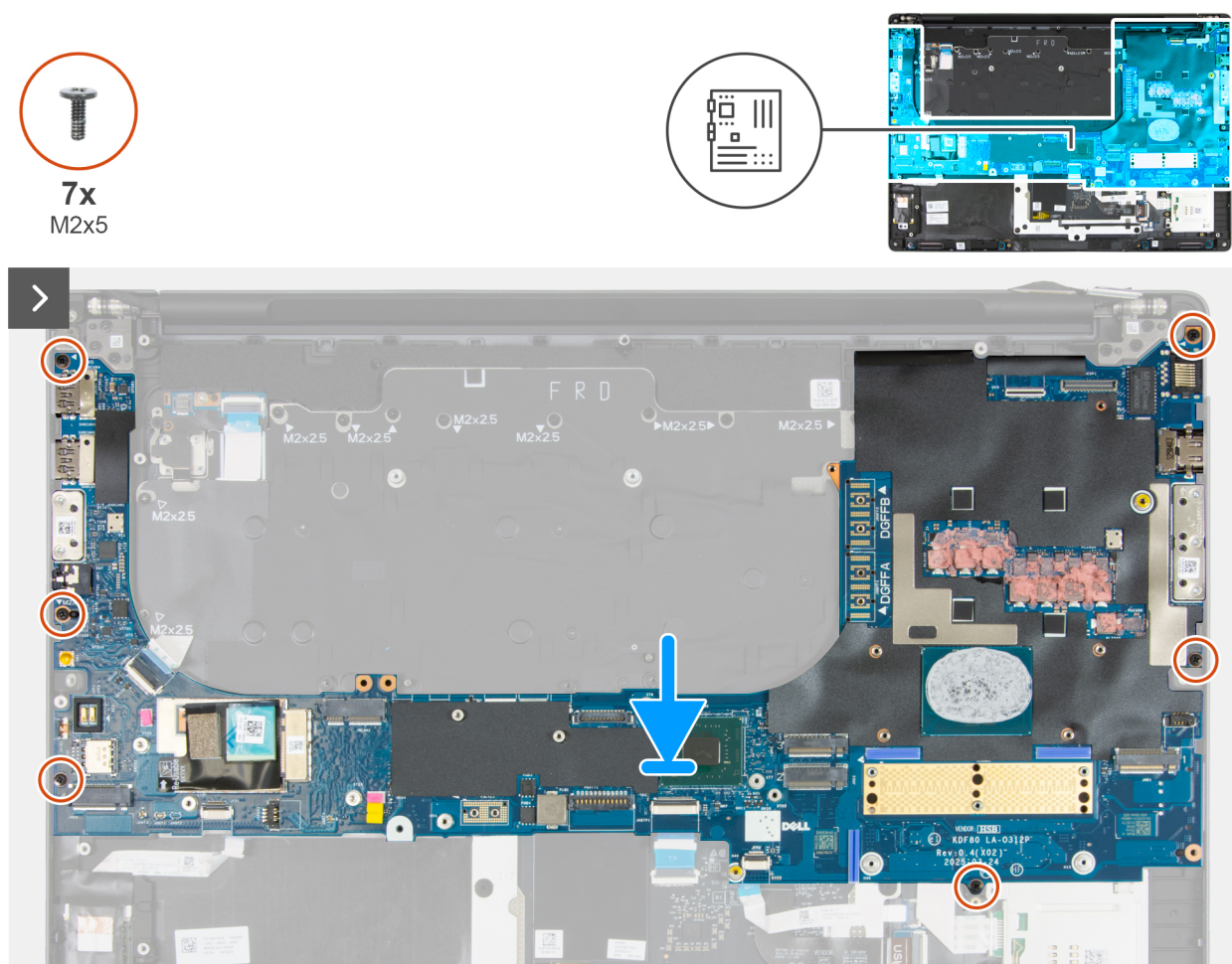
Rysunek 113. Instalowanie płyty głównej
