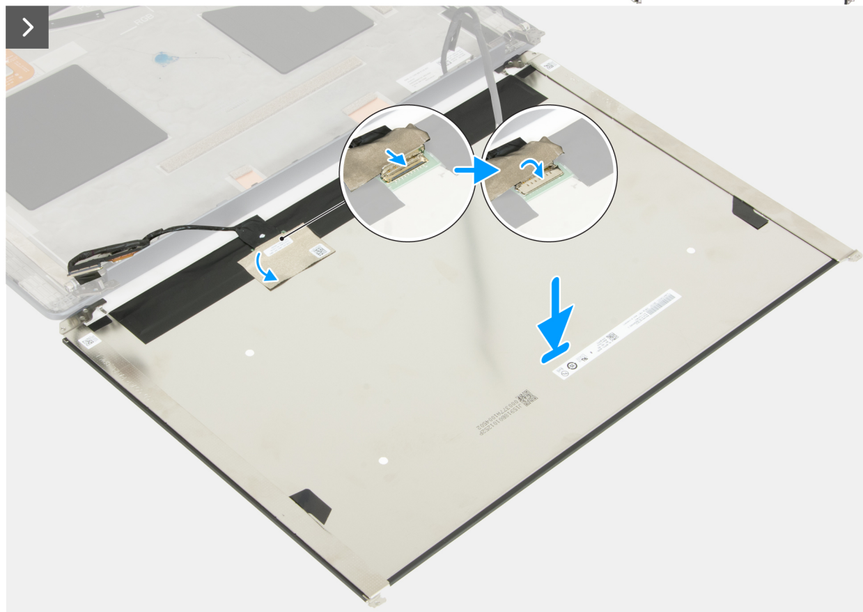
Rysunek 97. Instalowanie wyświetlacza
