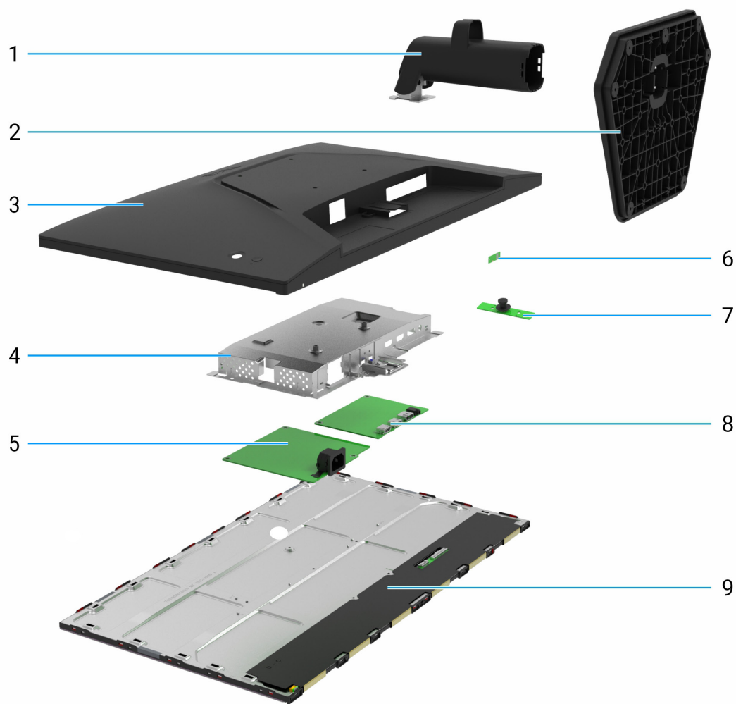
Figure 4. Principaux composants du moniteur SE2425HG/SE2725HG
