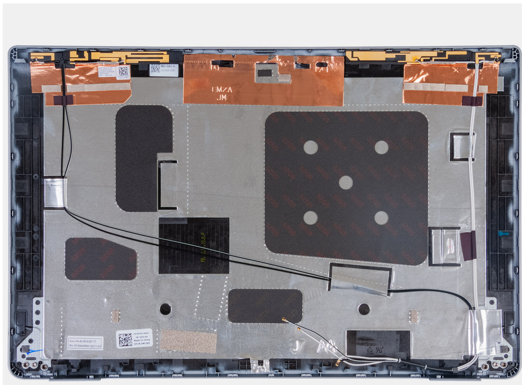
Afbeelding 107. Achterpaneel beeldscherm
