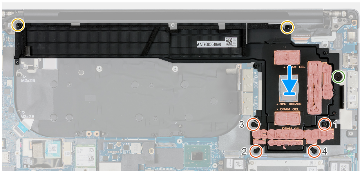
Afbeelding 76. De koelplaat installeren voor computers die met discrete graphics worden geleverd
