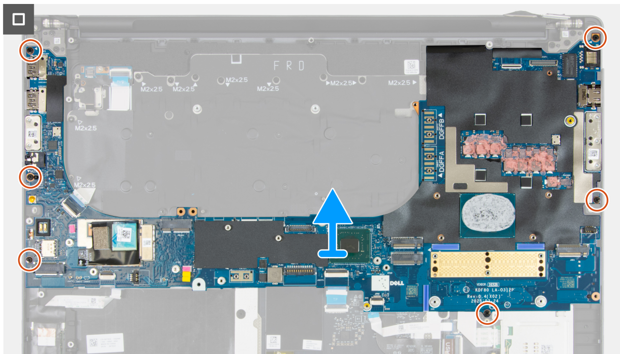
Afbeelding 110. De systeemkaart verwijderen
