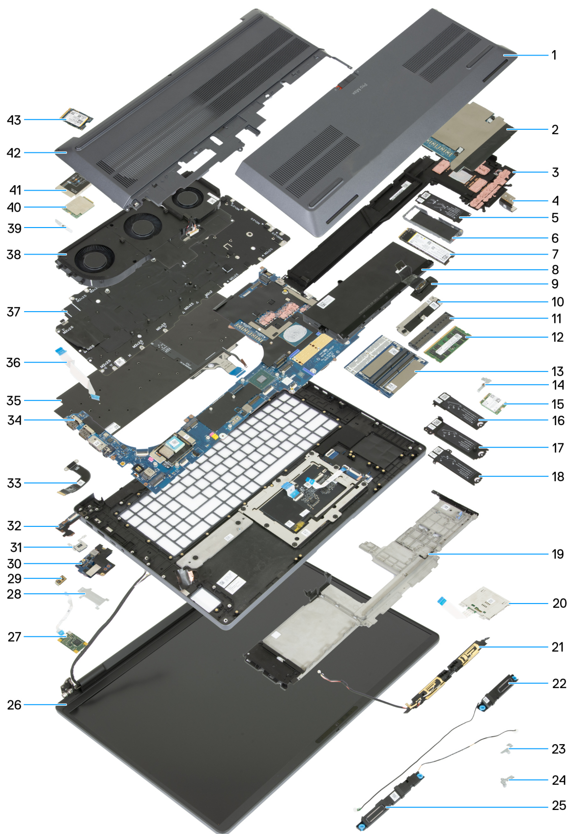
Abbeelding 9. Belangrijkste onderdelen van de Dell Pro Max 18 Plus MB18250
