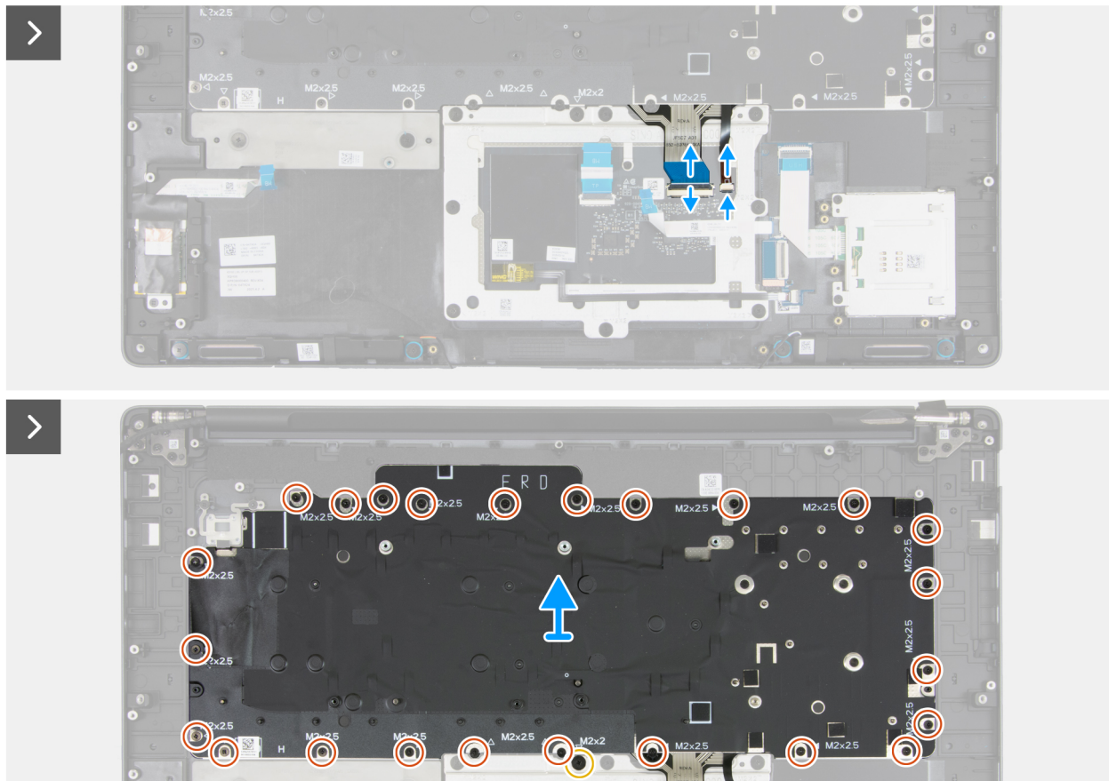
Afbeelding 119. Het toetsenbord verwijderen
