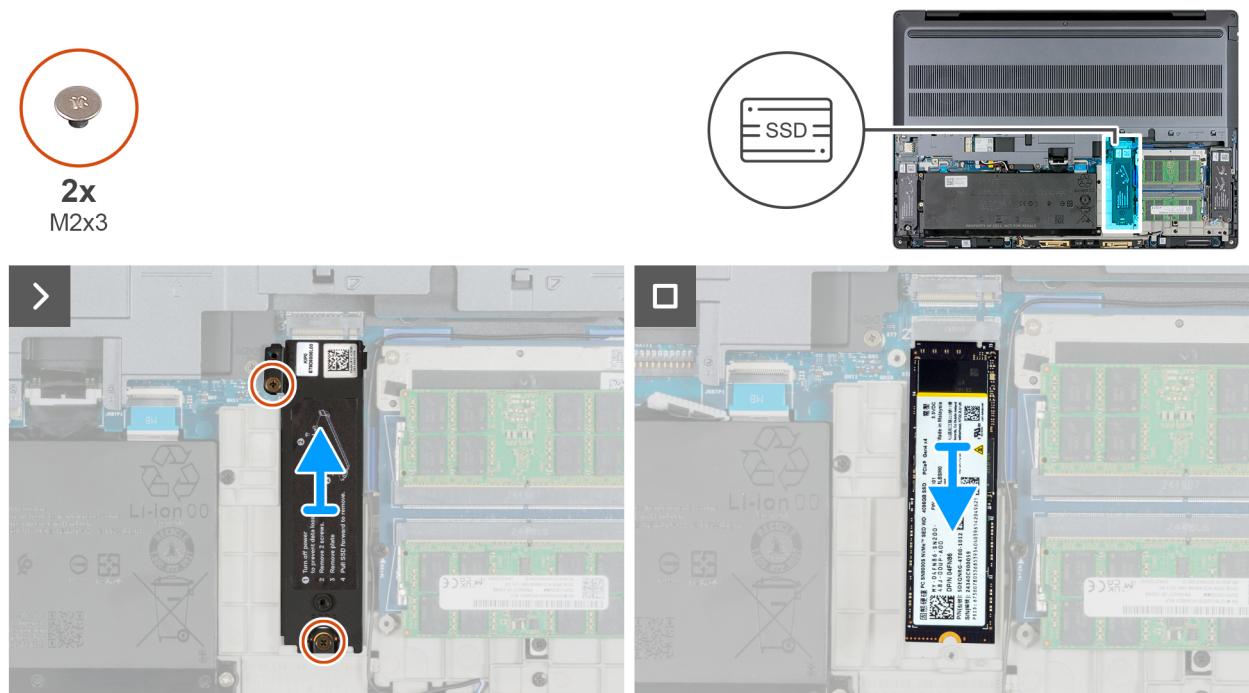
Afbeelding 38. De M.2 2280 SSD verwijderen uit slot 2 (SSD2)
