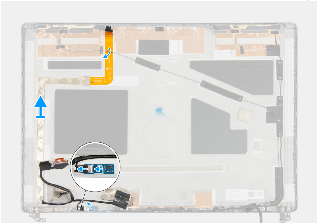
Afbeelding 104. De beeldschermkabel verwijderen
