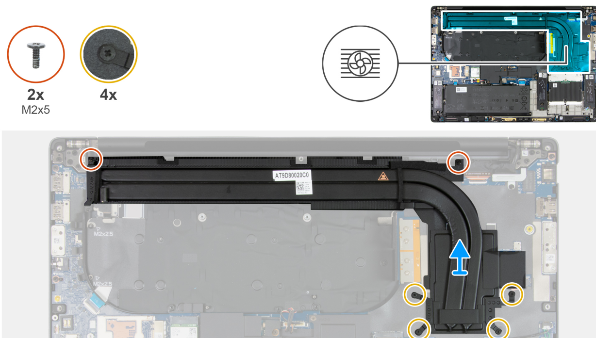
Afbeelding 73. De koelplaat verwijderen voor computers die worden geleverd met een geïntegreerde grafische kaart
