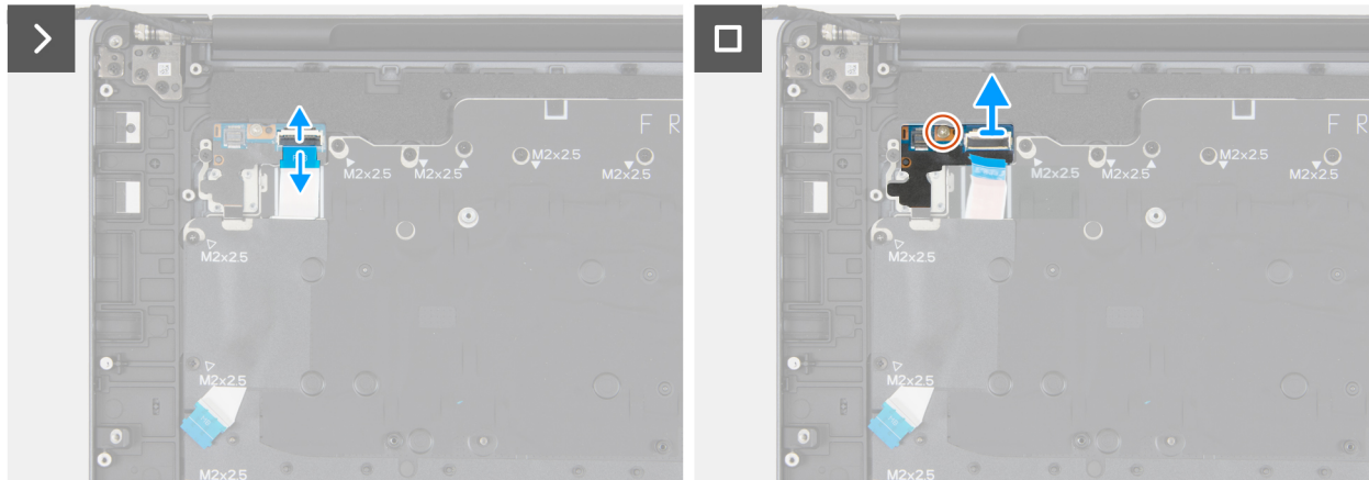
Afbeelding 127. De aan/uit-knopkaart verwijderen
