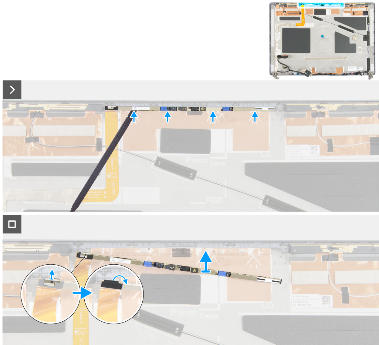
Afbeelding 103. De cameramodule verwijderen
