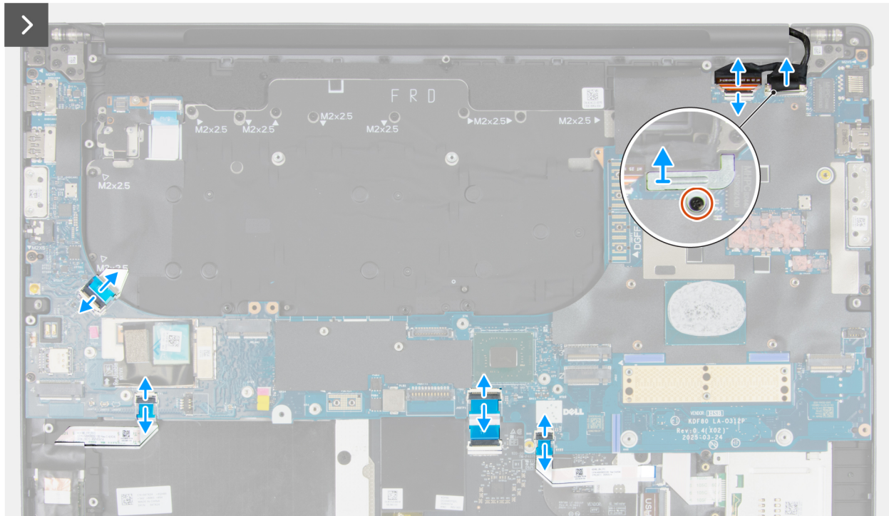
Afbeelding 109. De systeemkaart verwijderen
