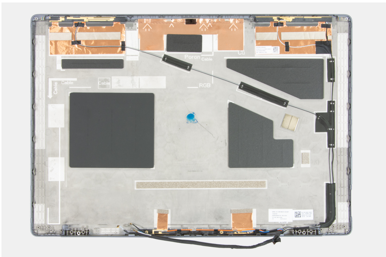
Afbeelding 106. Achterpaneel beeldscherm
