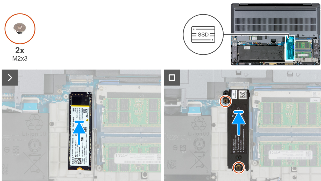
Afbeelding 39. De M.2 2280 SSD in slot 2 (SSD2) installeren
