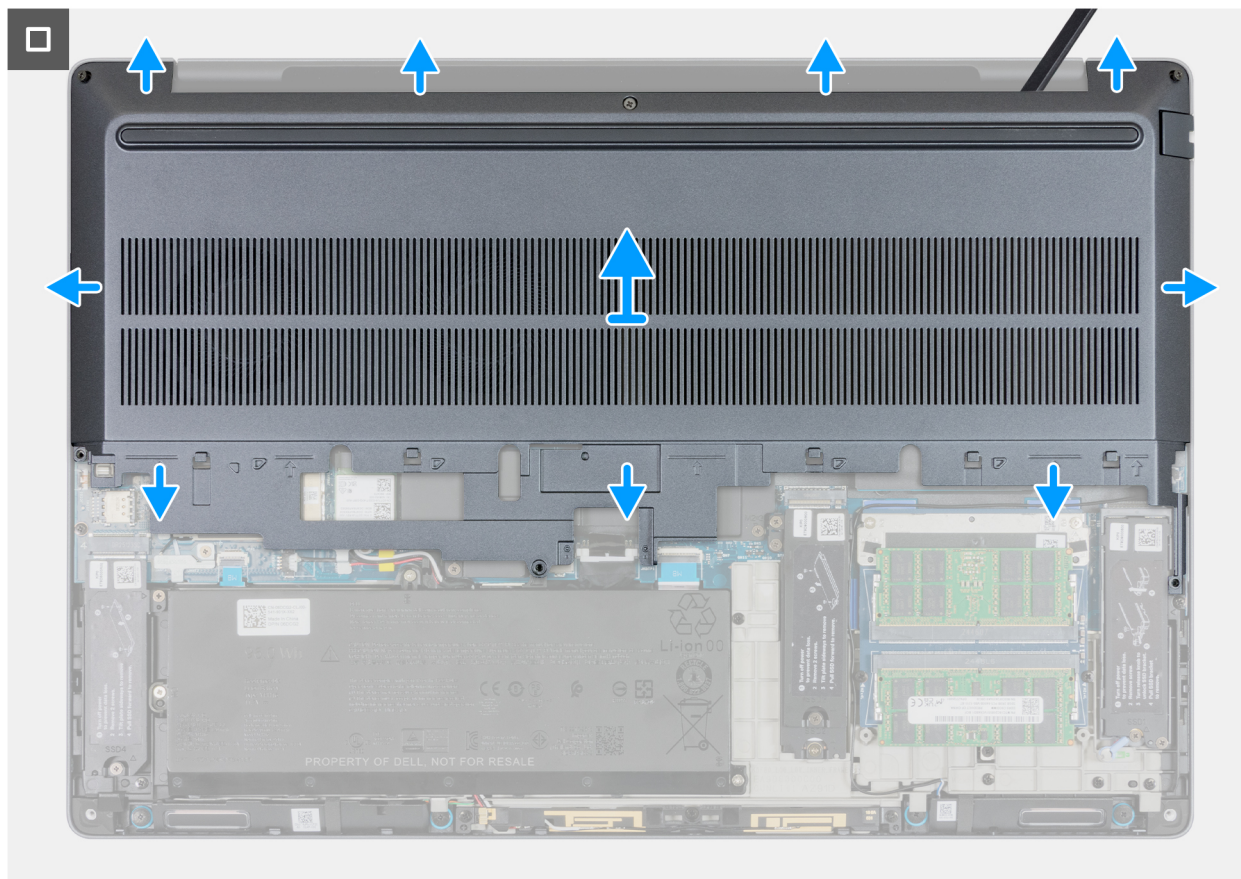
Afbeelding 19. De onderplaat van de palmsteun- en toetsenbordeenheden tillen
