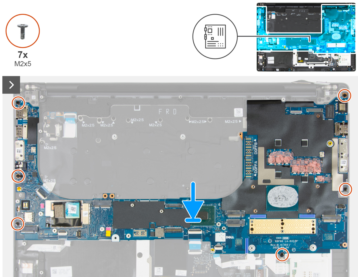
Afbeelding 113. De systeemkaart installeren
