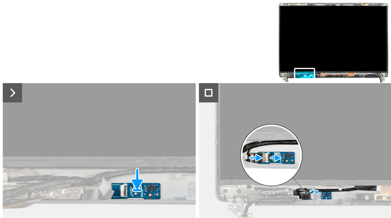
Afbeelding 102. De sensorkaart plaatsen
