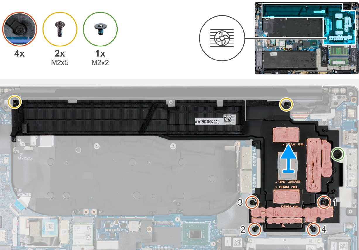
Afbeelding 75. De koelplaat verwijderen voor computers die worden geleverd met discrete graphics
