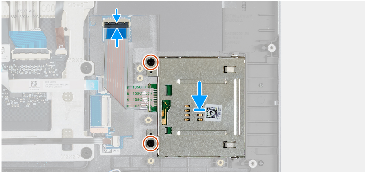
Afbeelding 124. De smartcardlezer installeren
