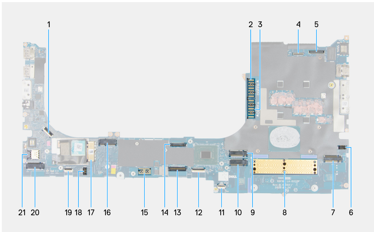
Afbeelding 112. Onderdelen van de systeemkaart
