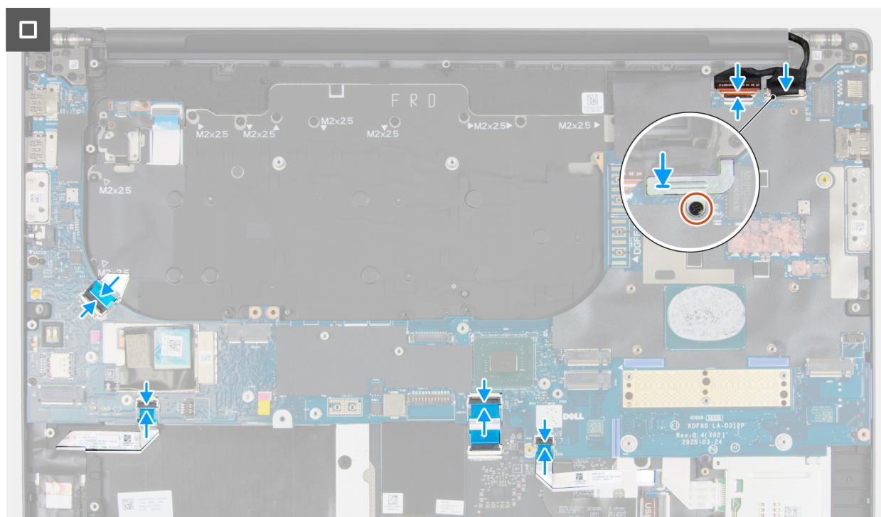
Afbeelding 114. De systeemkaart installeren
