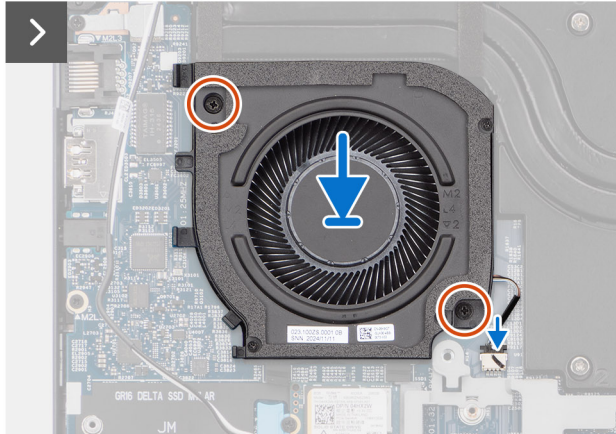
Abbildung 31. Installieren des rechten/Prozessorlüfters
