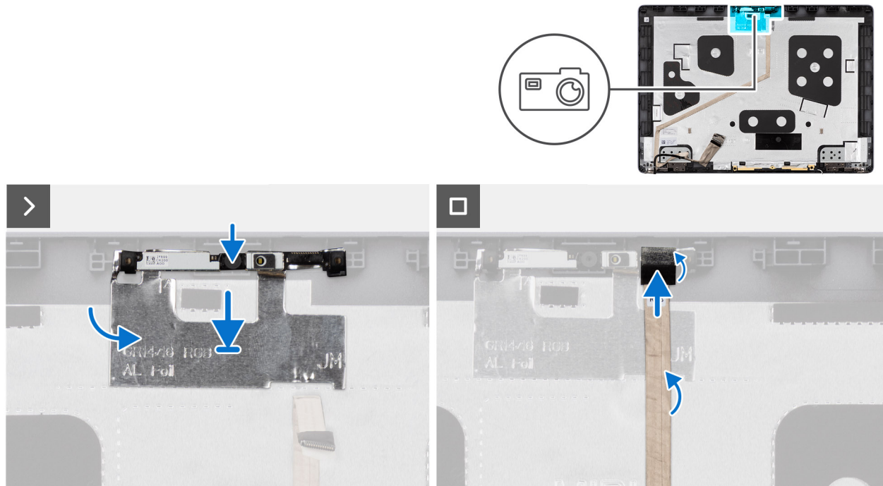
Abbildung 70. Installieren der Kamera
