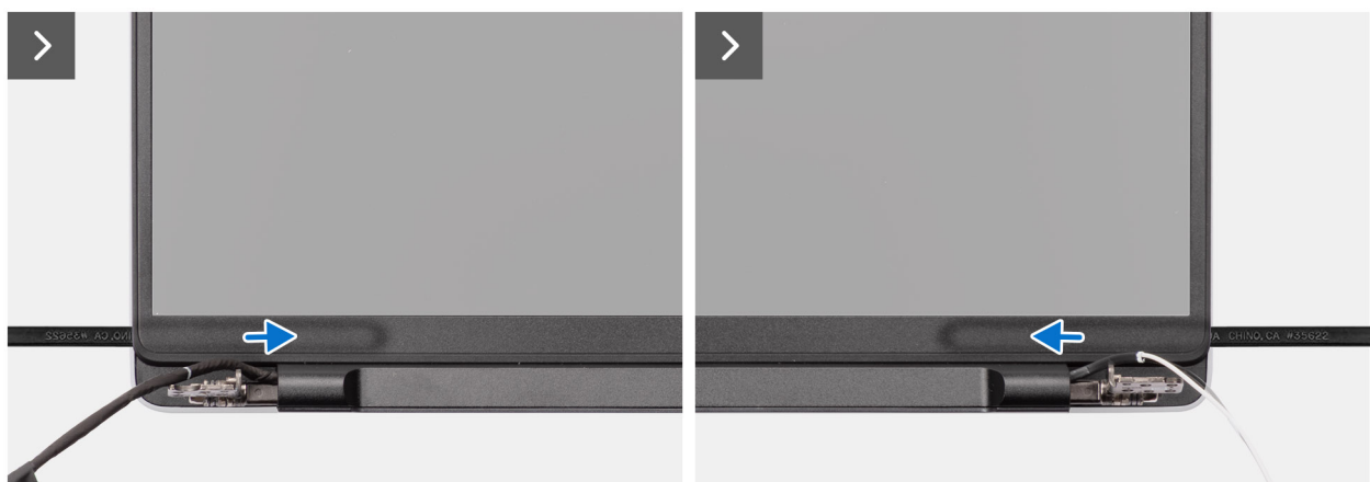
Abbildung 54. Entfernen der Bildschirmblende
