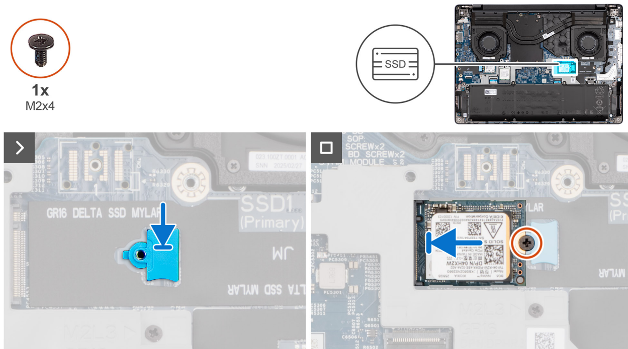
Abbildung 22. Installieren des M.2 2230-Solid-State-Laufwerks
