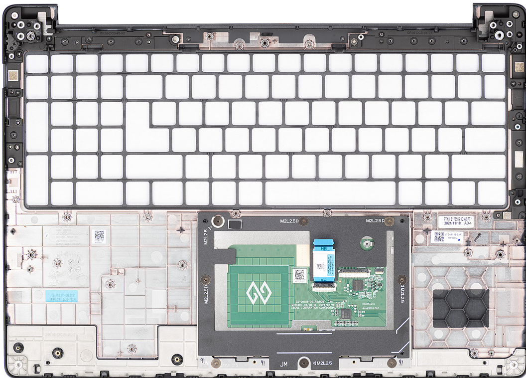
Abbildung 88. Handauflagenbaugruppe
