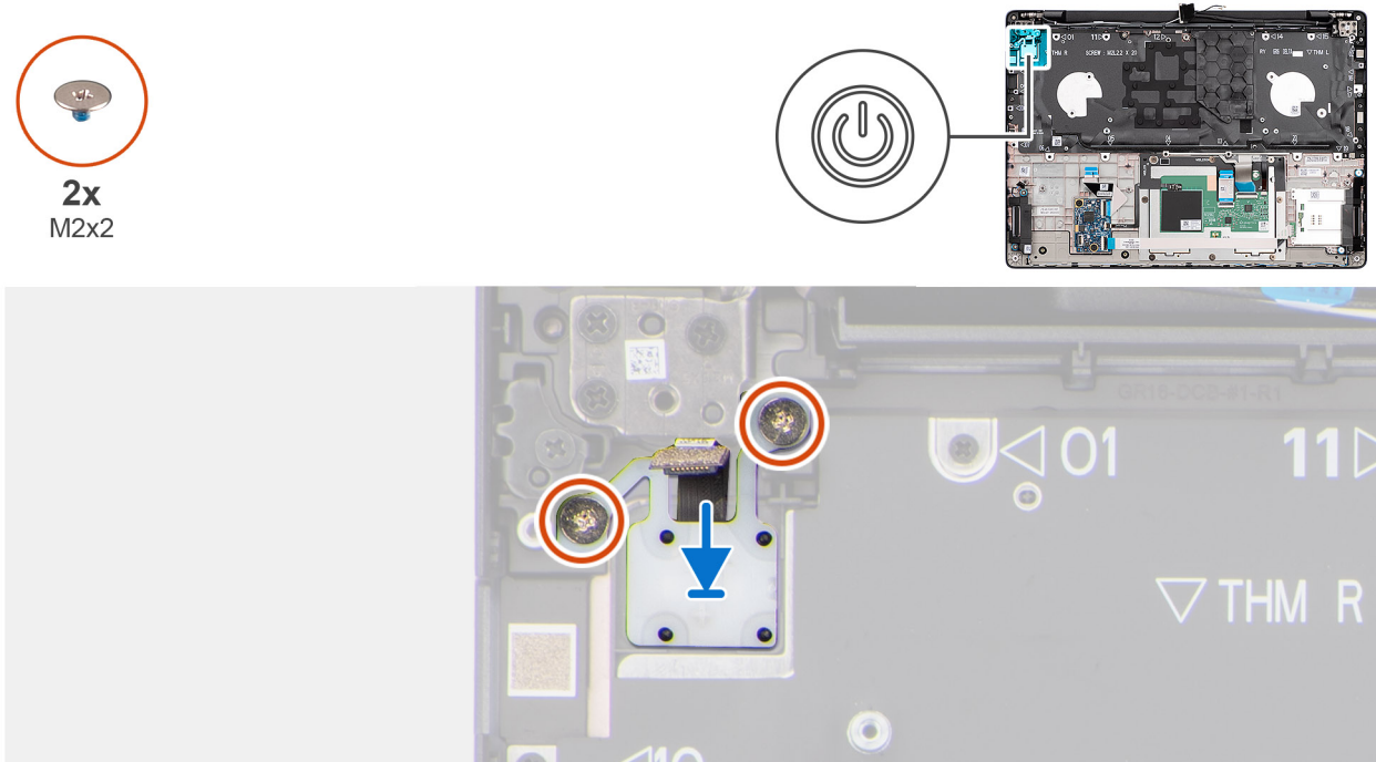
Abbildung 82. Installieren des Netzschalters
