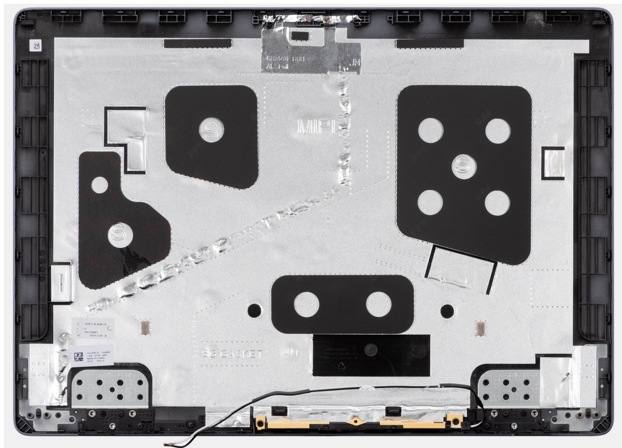
Abbildung 72. Bildschirmrückwand-Antennen-Baugruppe
