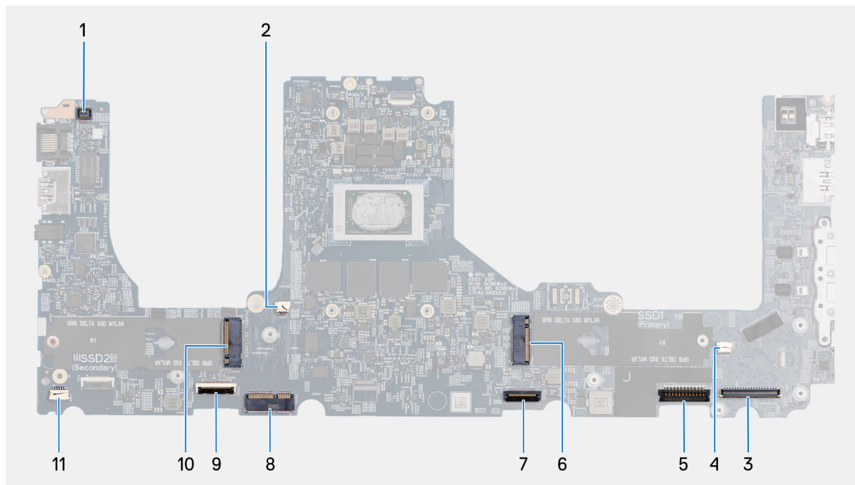
Abbildung 76. Anschlüsse auf der Hauptplatine
