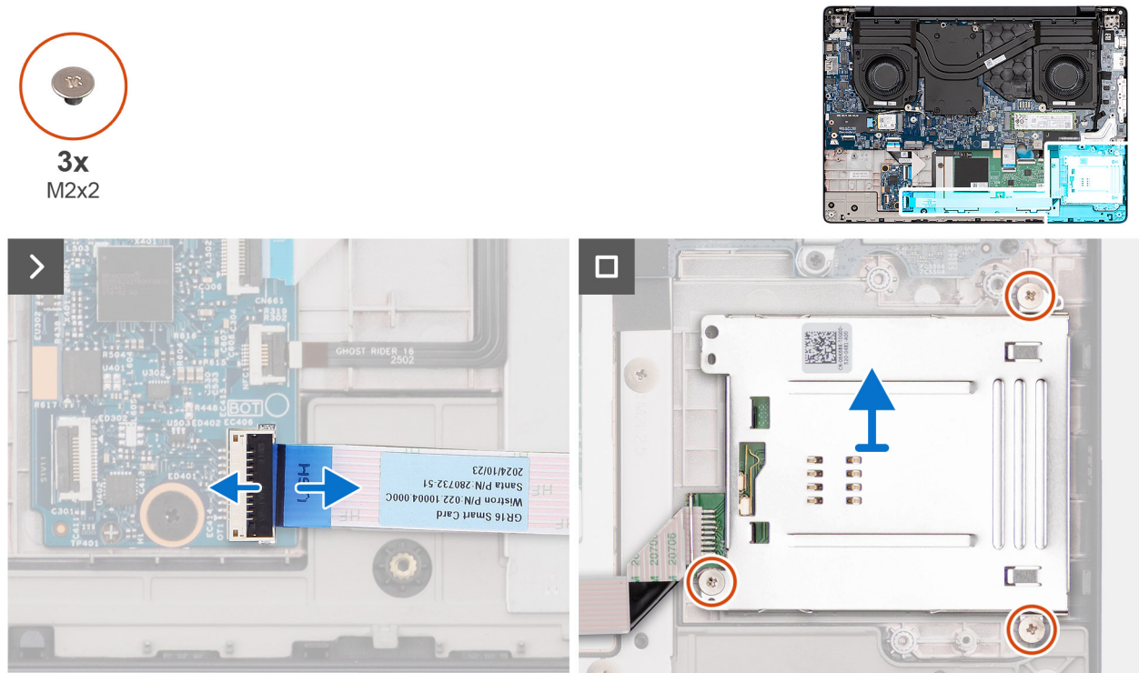
Abbildung 42. Entfernen des Smartcardlesegeräts
