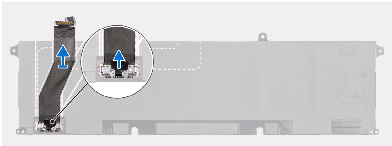
Abbildung 19. Trennen des Akkukabels
