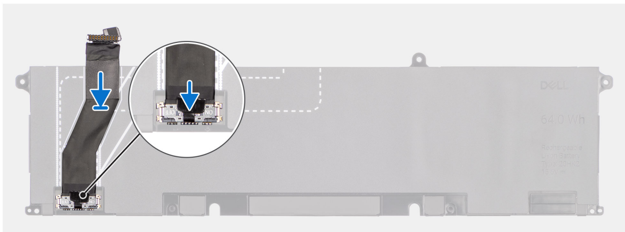
Abbildung 20. Verbinden des Akkukabels
