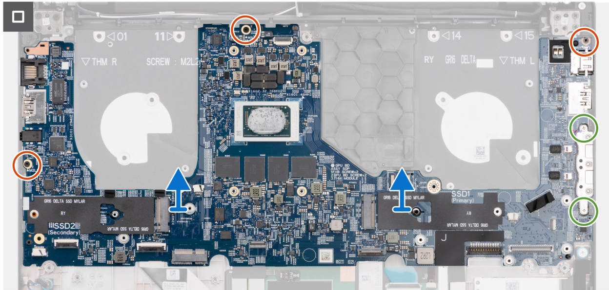
Abbildung 75. Entfernen der Systemplatine
