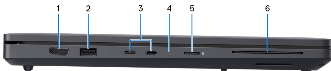
Abbildung 1. Linke Seitenansicht
