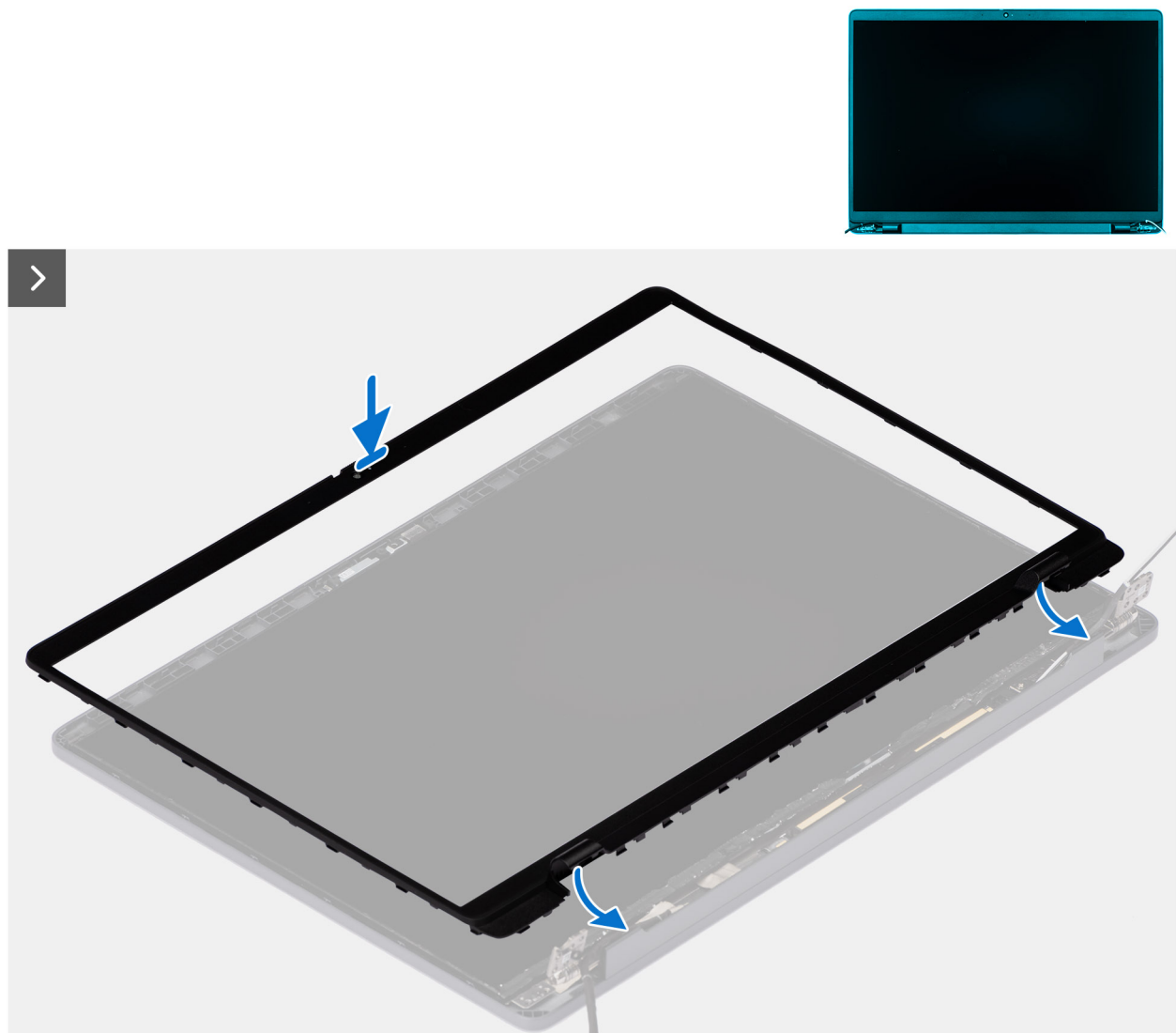
Abbildung 56. Einbauen der Bildschirmblende
