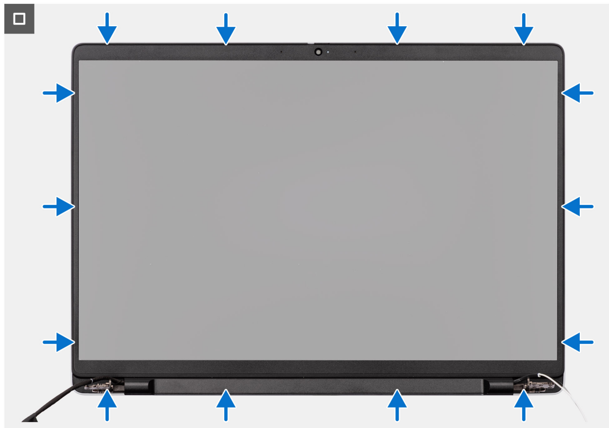
Abbildung 57. Einbauen der Bildschirmblende
