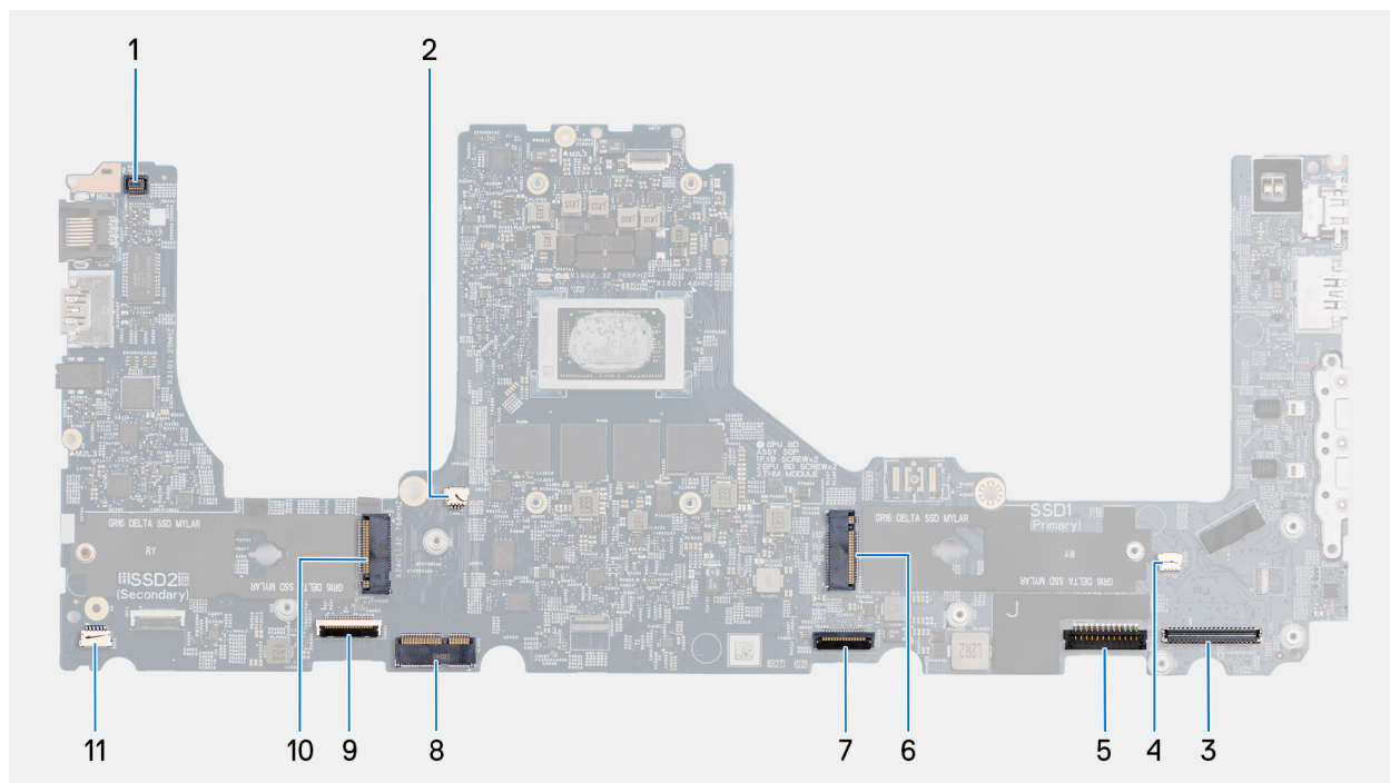
Abbildung 73. Anschlüsse auf der Hauptplatine
