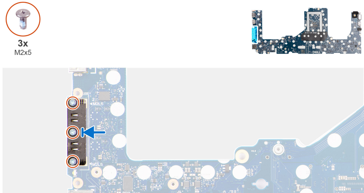
Abbildung 80. Installieren des USB-Typ-C-Moduls
