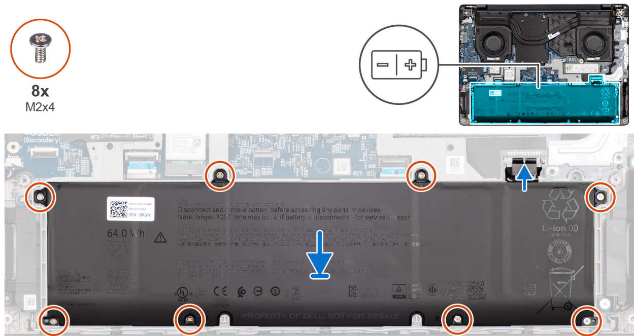
Abbildung 18. Einsetzen des Akkus
