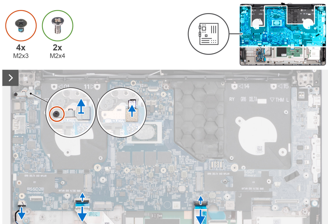
Abbildung 74. Entfernen der Systemplatine
