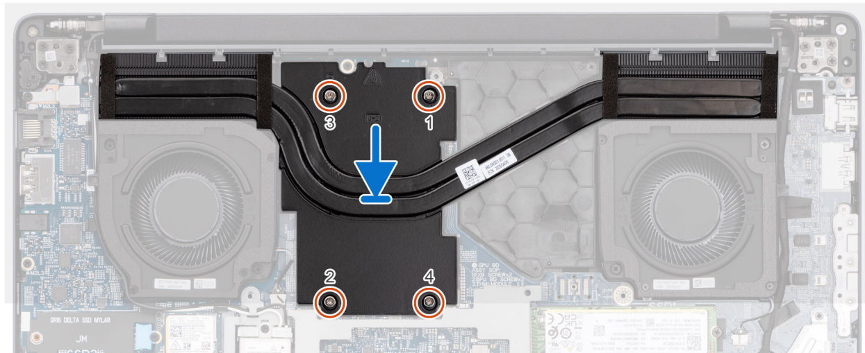
Abbildung 35. Einsetzen des Kühlkörpers
