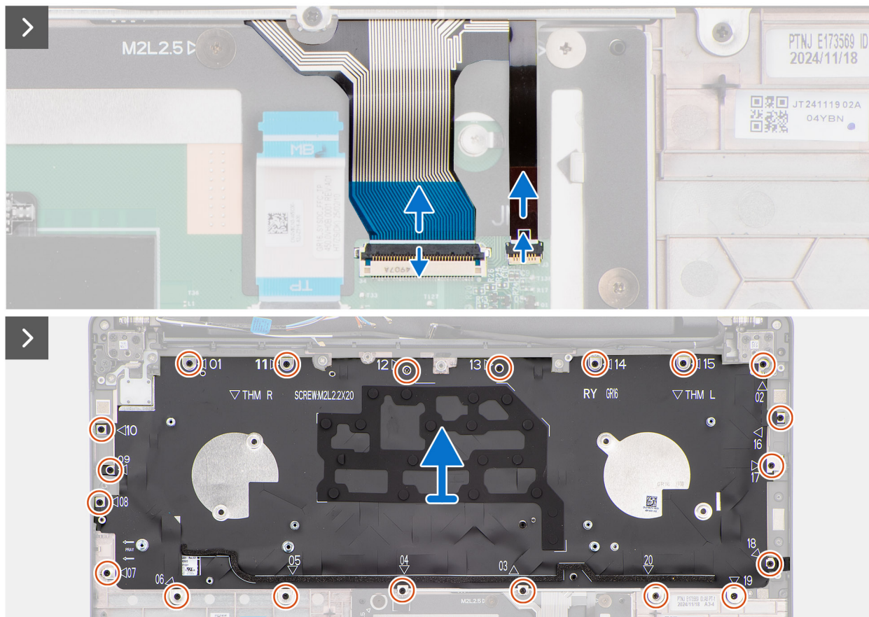
Abbildung 83. Entfernen der Tastatur
