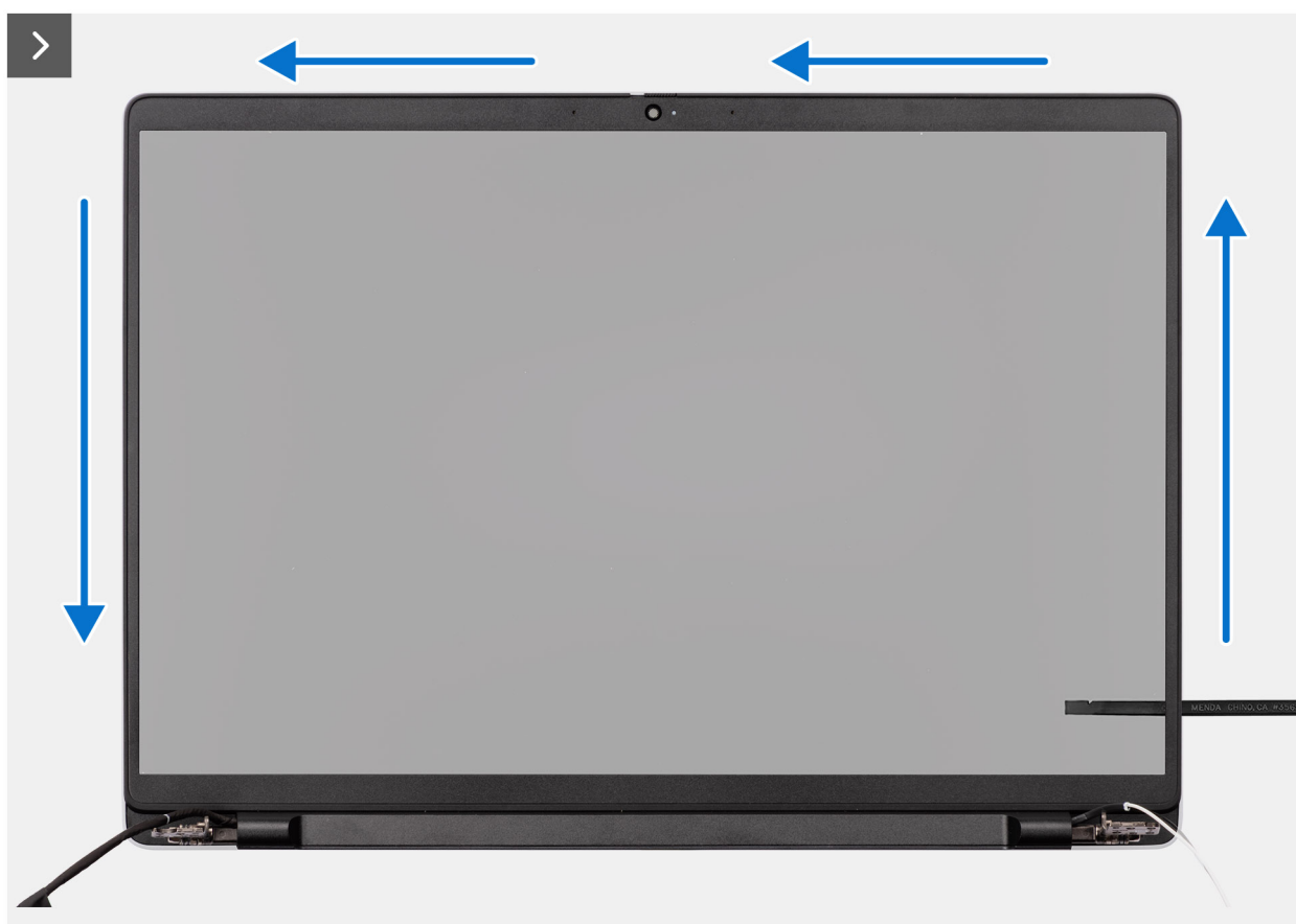
Abbildung 52. Entfernen der Bildschirmblende
