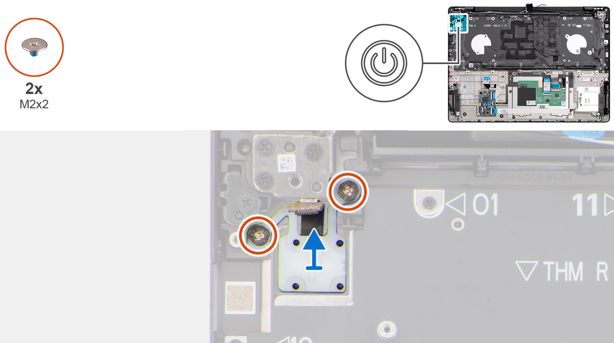
Abbildung 81. Entfernen des Netzschalters
