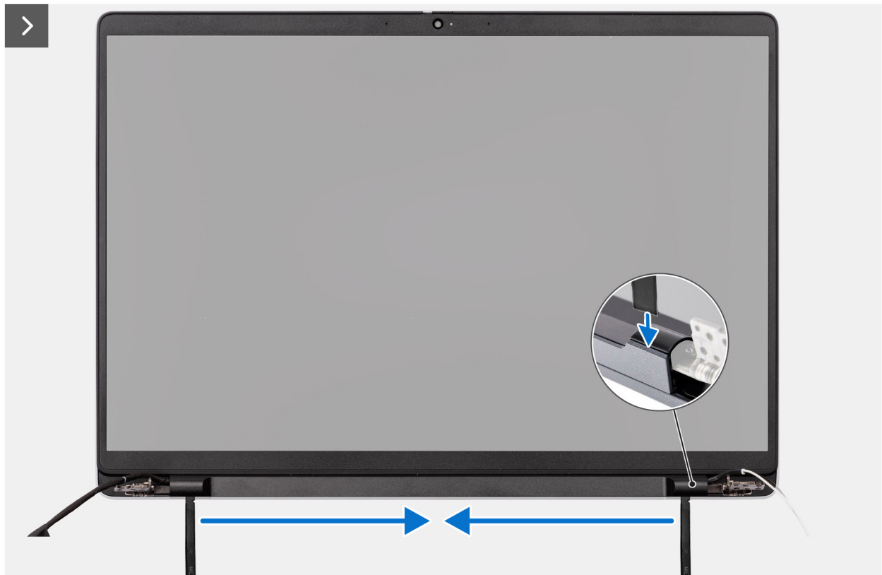
Abbildung 53. Entfernen der Bildschirmblende
