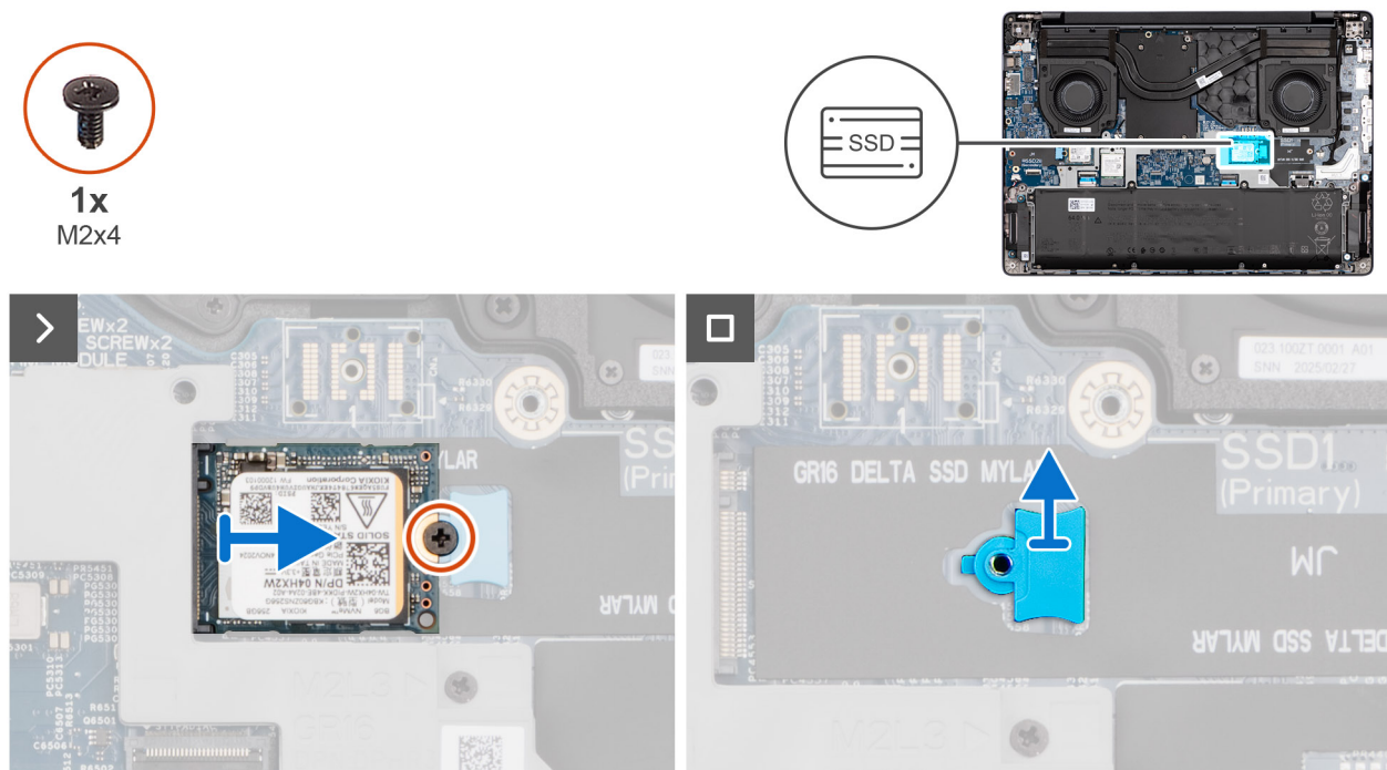
Abbildung 21. Entfernen des M.2-2230-Solid-State-Laufwerks
