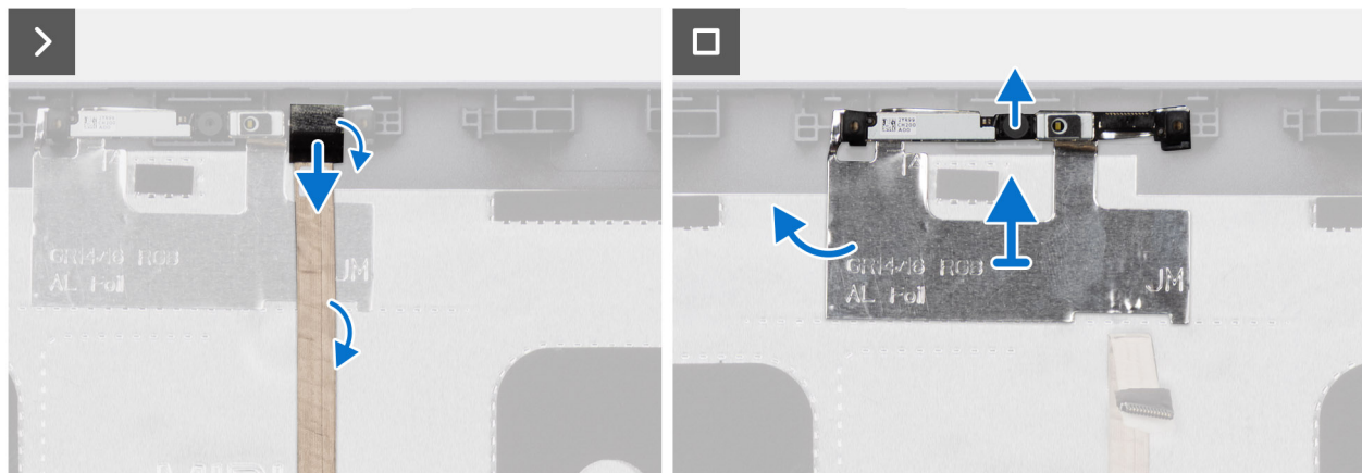
Abbildung 69. Entfernen der Kamera
