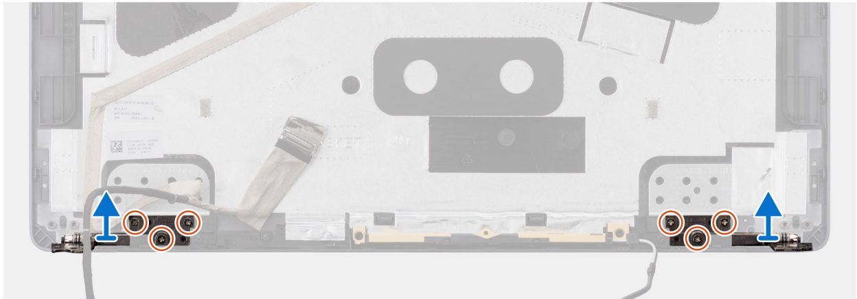
Abbildung 65. Entfernen der Bildschirmscharniere
