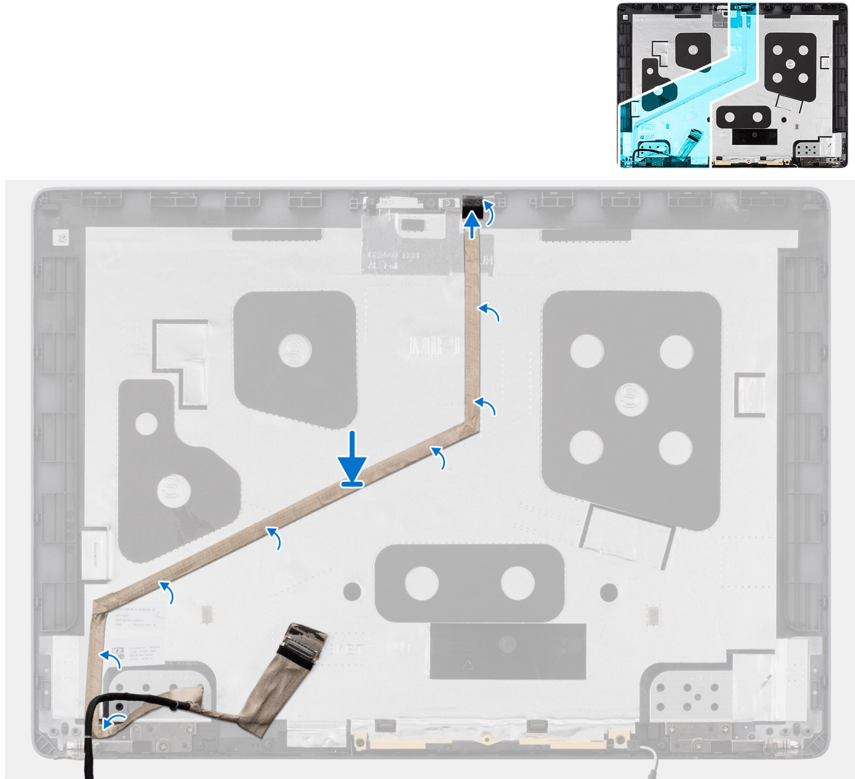
Abbildung 68. Einbauen des Bildschirmkabels
