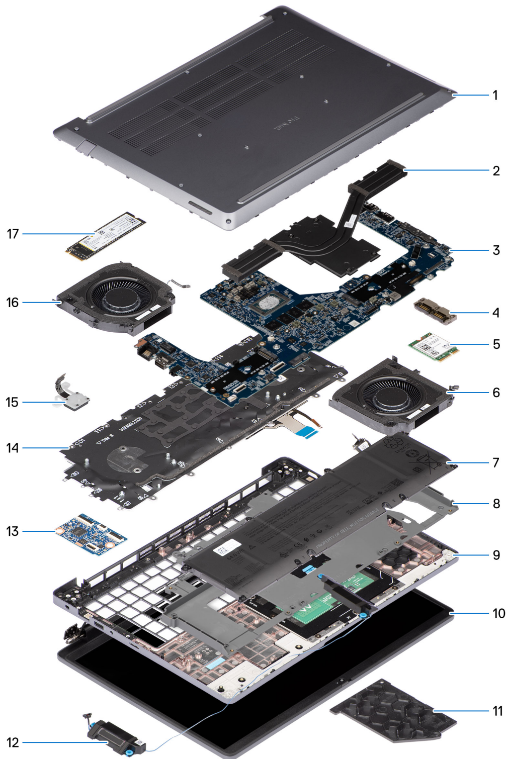
Abbildung 11. Hauptkomponenten Ihres Dell Pro Max 16 MC16255
