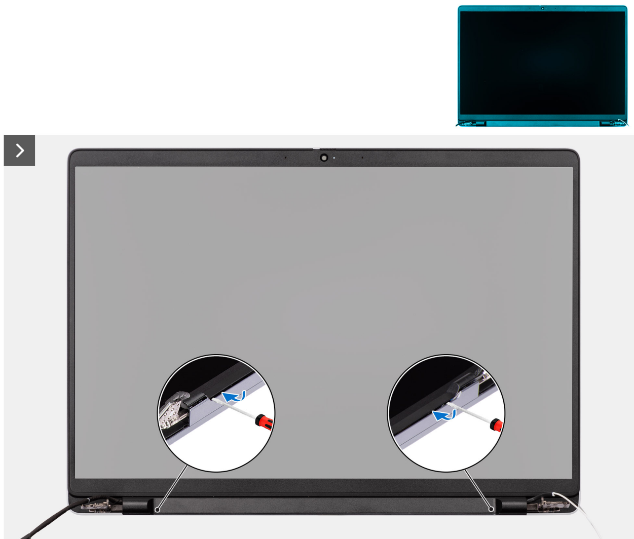
Abbildung 50. Entfernen der Bildschirmblende
