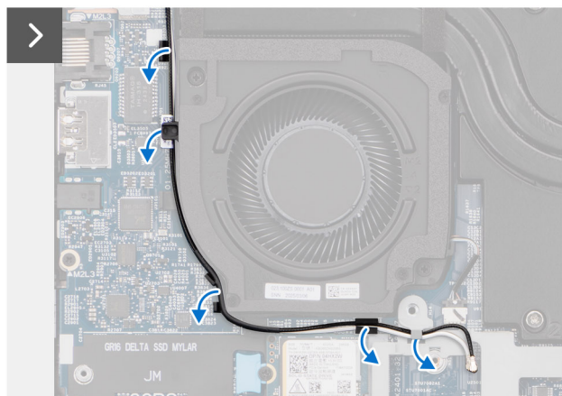
Abbildung 30. Entfernen des rechten/Prozessorlüfters
