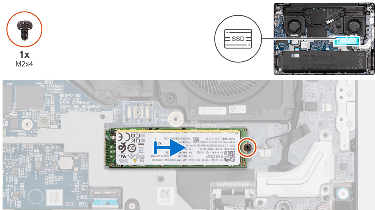
Abbildung 23. Entfernen des M.2-2280-Solid-State-Laufwerks
