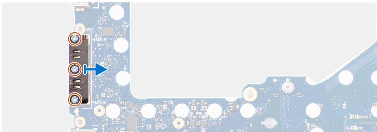
Abbildung 79. Entfernen des USB-Typ-C-Moduls
