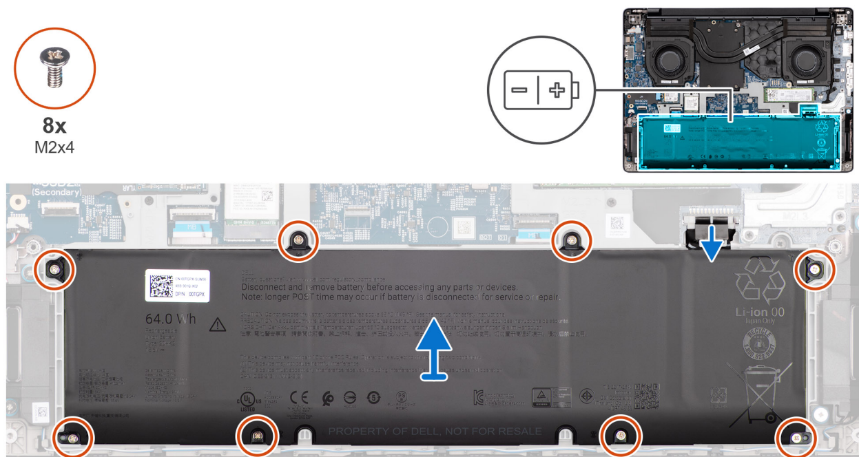
Abbildung 17. Entfernen des Akkus
