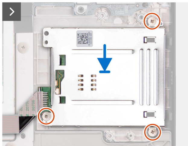
Abbildung 43. Installieren des Smartcardlesegeräts
