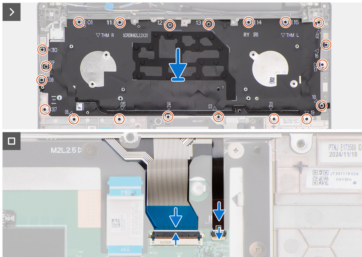
Abbildung 86. Einbauen der Tastatur
