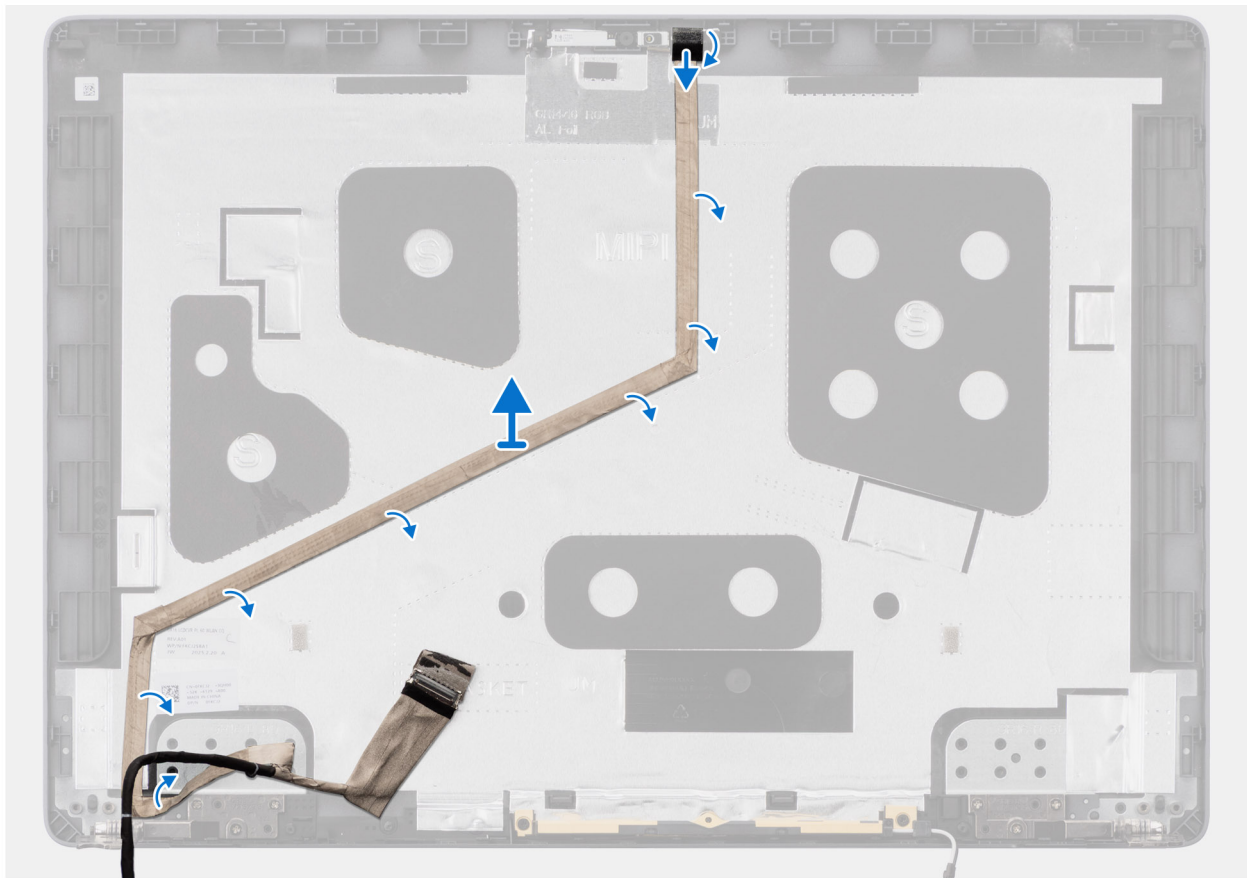
Abbildung 67. Entfernen des Bildschirmkabels
