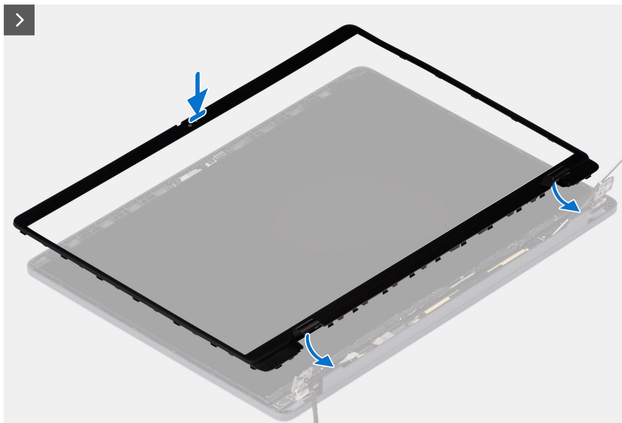
Afbeelding 56. De beeldschermbezel installeren
