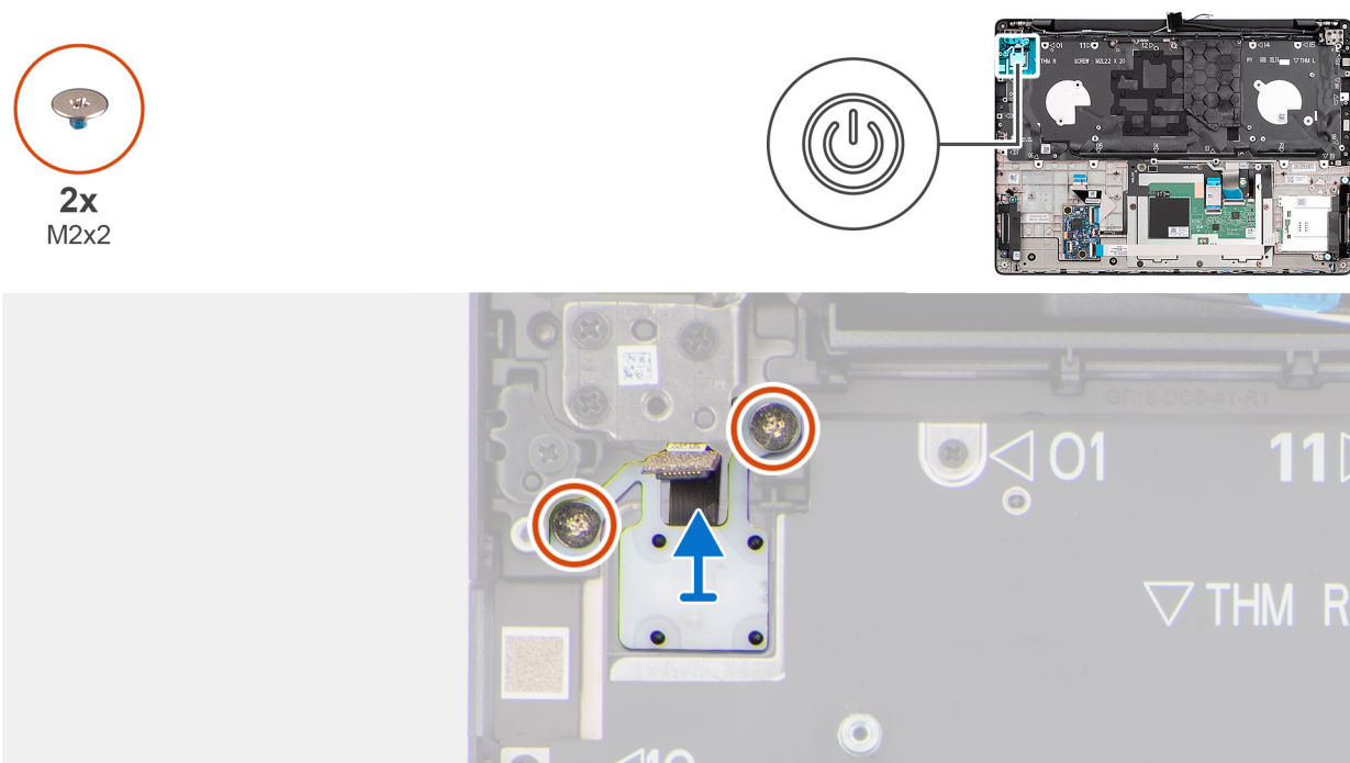
Afbeelding 81. De aan-uitknop verwijderen
