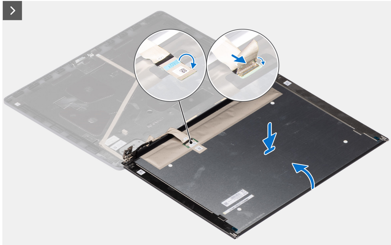
Afbeelding 62. Het beeldschermpaneel installeren
