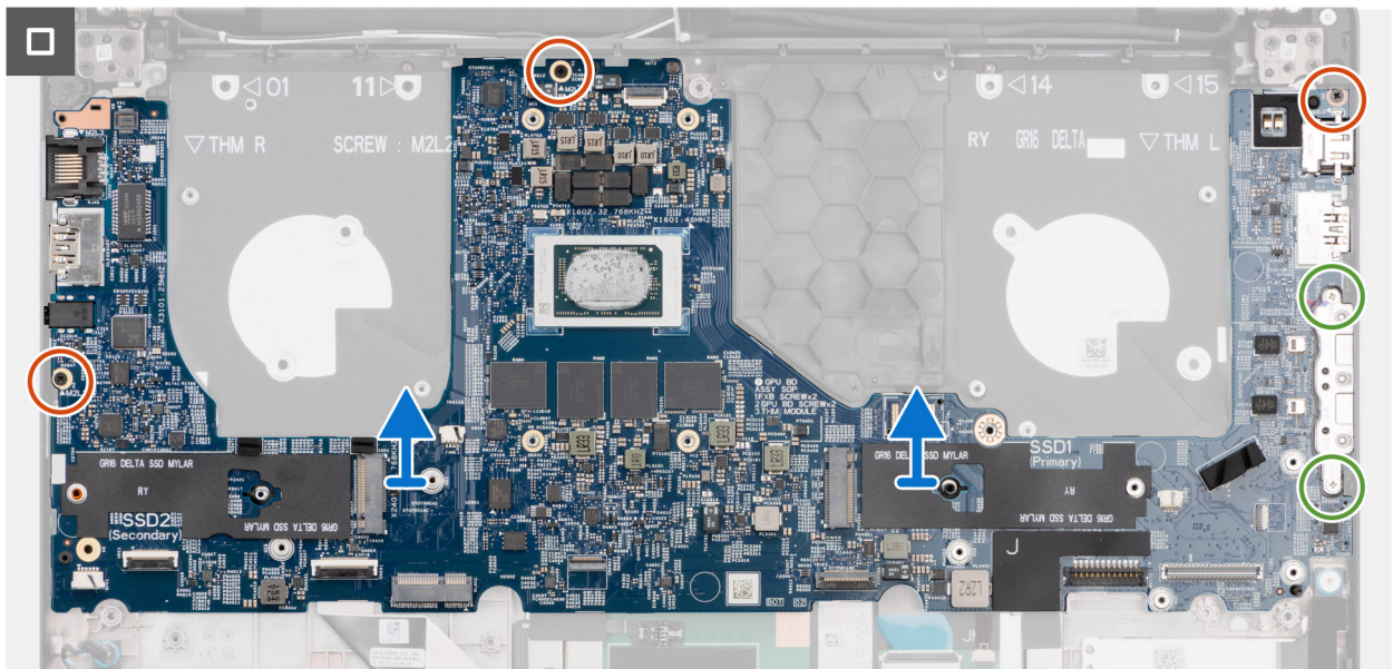
Afbeelding 75. De systeemkaart verwijderen
