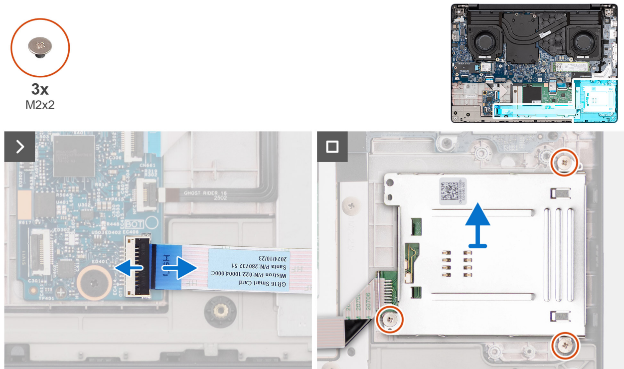
Afbeelding 42. De smartcardlezer verwijderen
