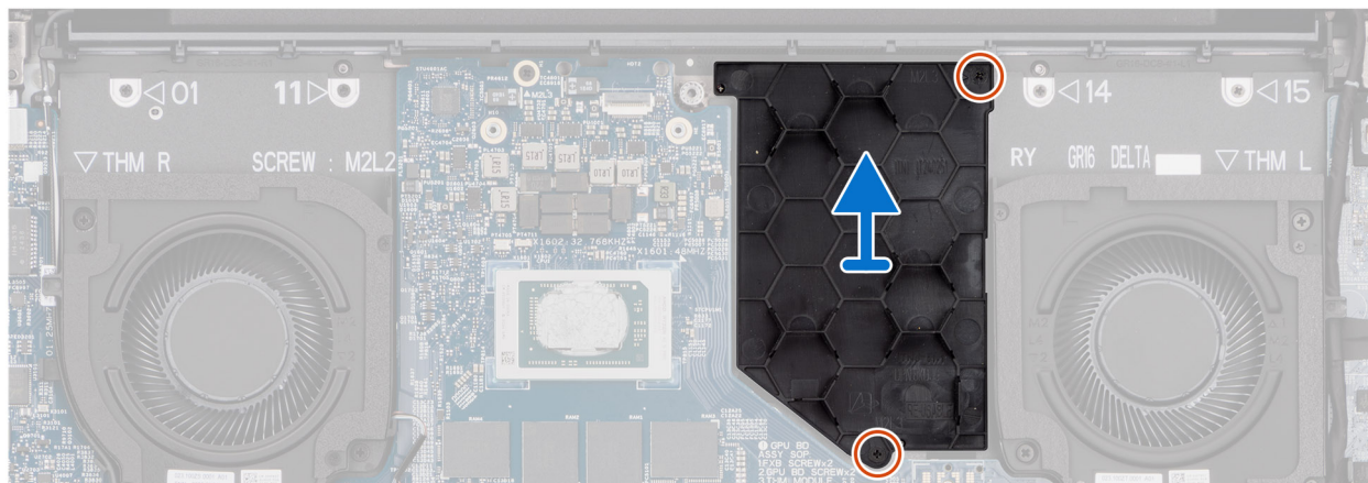
Afbeelding 36. De GPU-vulling verwijderen
