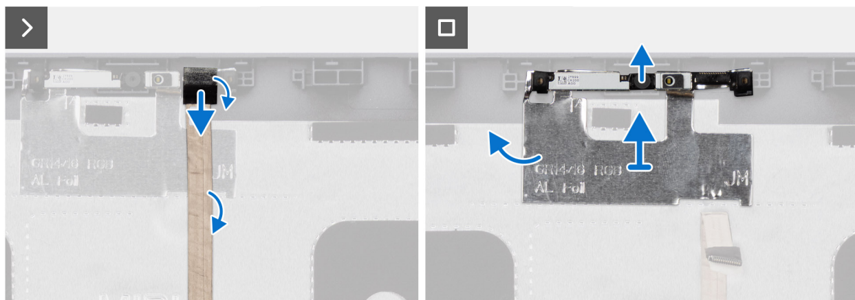
Afbeelding 69. De camera verwijderen
