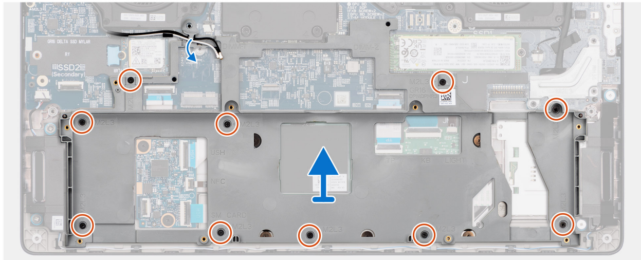
Afbeelding 38. Het batterijframe verwijderen
