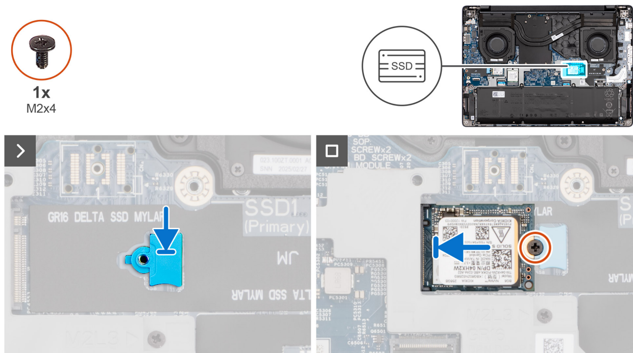
Afbeelding 22. De M.2 2230 SSD plaatsen
