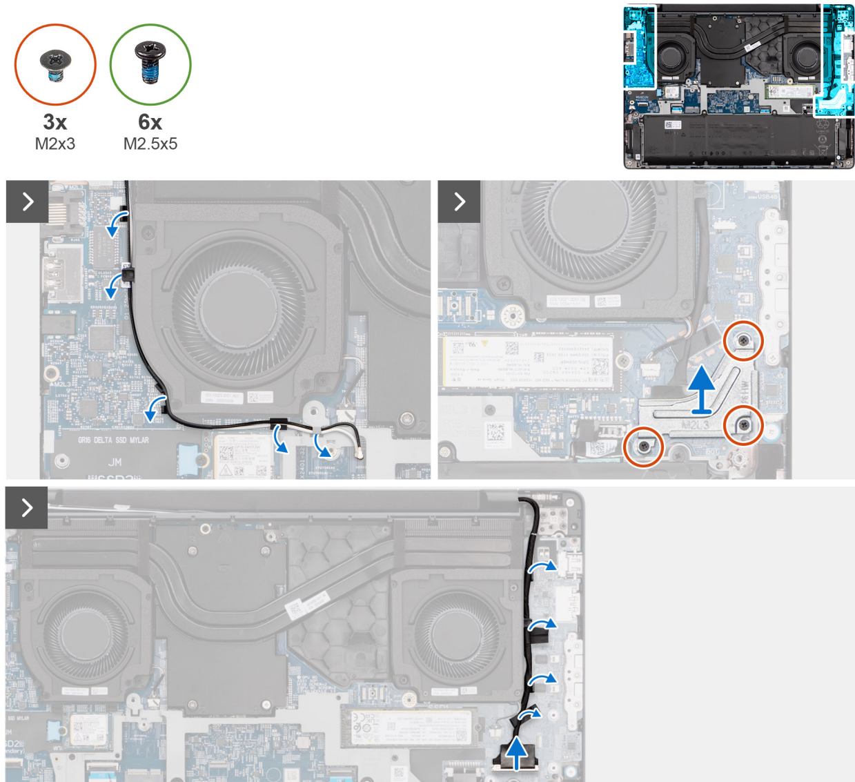
Afbeelding 44. De beeldschermeenheid verwijderen
