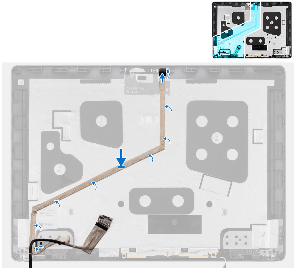
Afbeelding 68. De beeldschermkabel installeren
