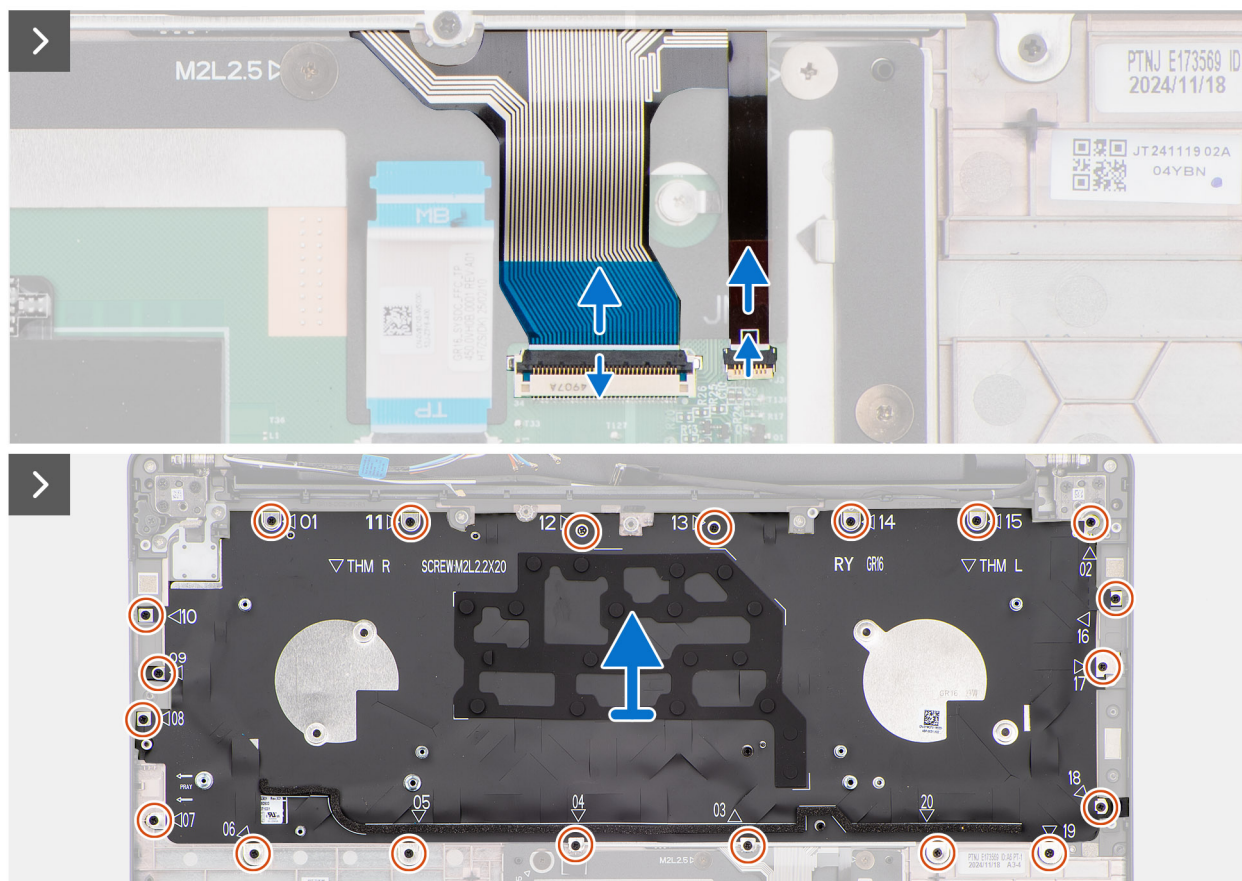
Afbeelding 83. Het toetsenbord verwijderen
