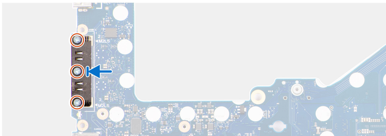
Afbeelding 80. De USB Type-C-module installeren
