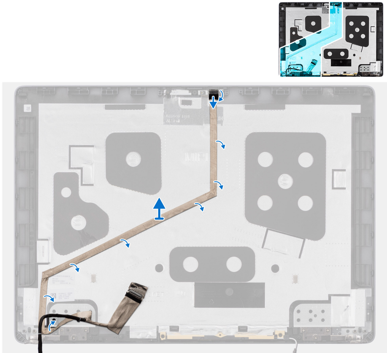
Afbeelding 67. De beeldschermkabel verwijderen
