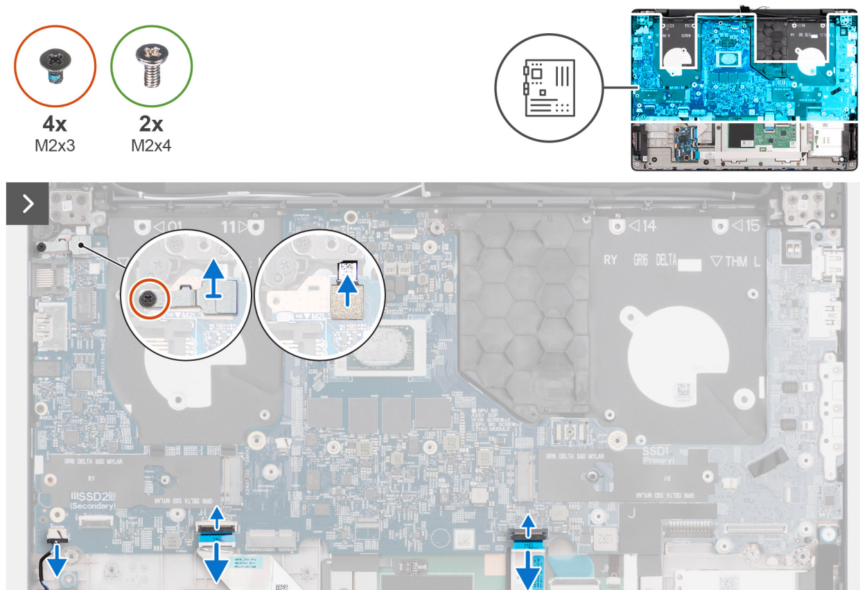
Afbeelding 74. De systeemkaart verwijderen
