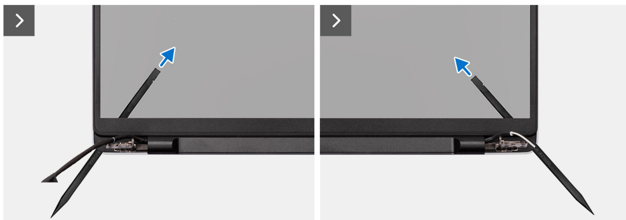
Afbeelding 51. De beeldschermbezel verwijderen
