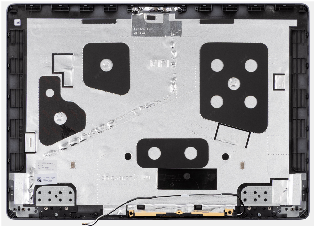
Afbeelding 71. Achterplaat van het beeldscherm en de antenne-eenheid
