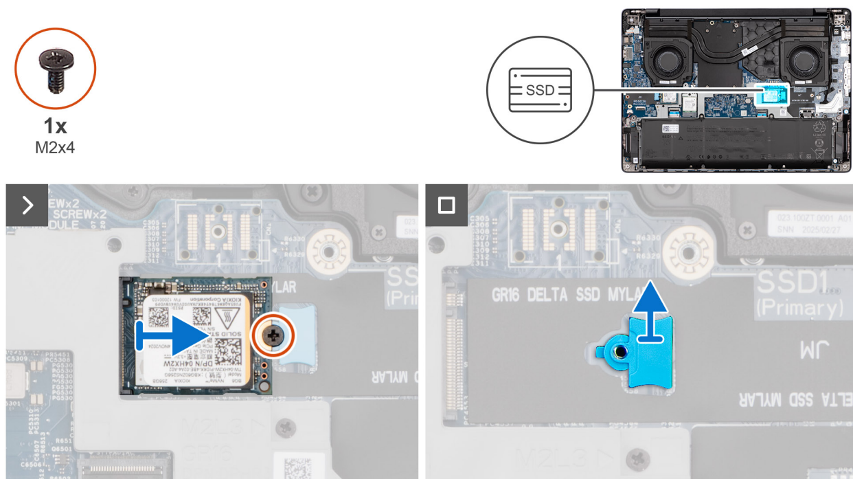
Afbeelding 21. De M.2 2230 SSD verwijderen
