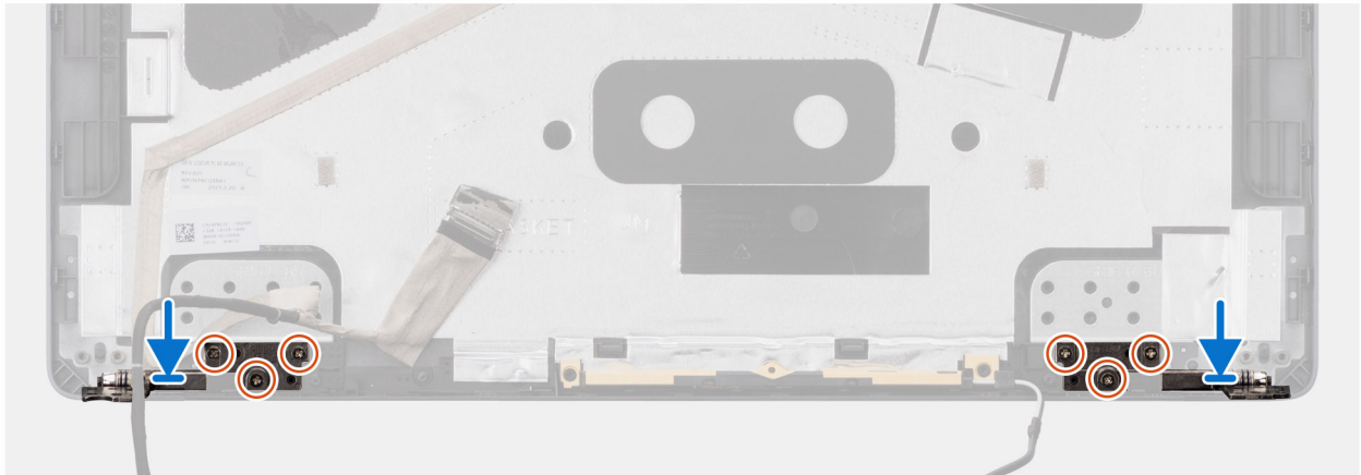
Afbeelding 66. De beeldschermsharnieren installeren
