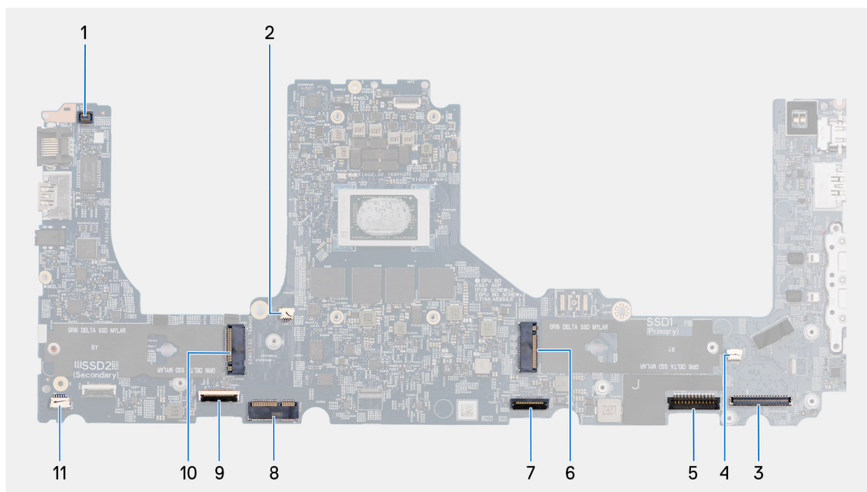
Afbeelding 73. Systeemkaartconnectoren
