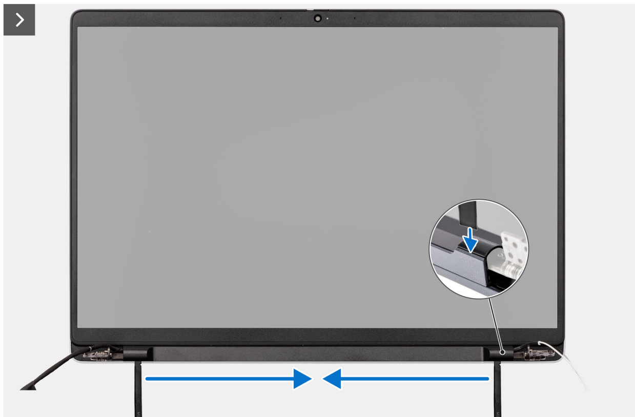
Afbeelding 53. De beeldschermbezel verwijderen
