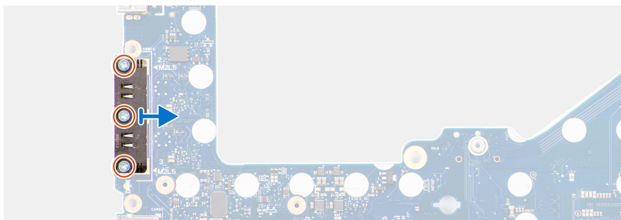
Afbeelding 79. De USB Type-C-module verwijderen
