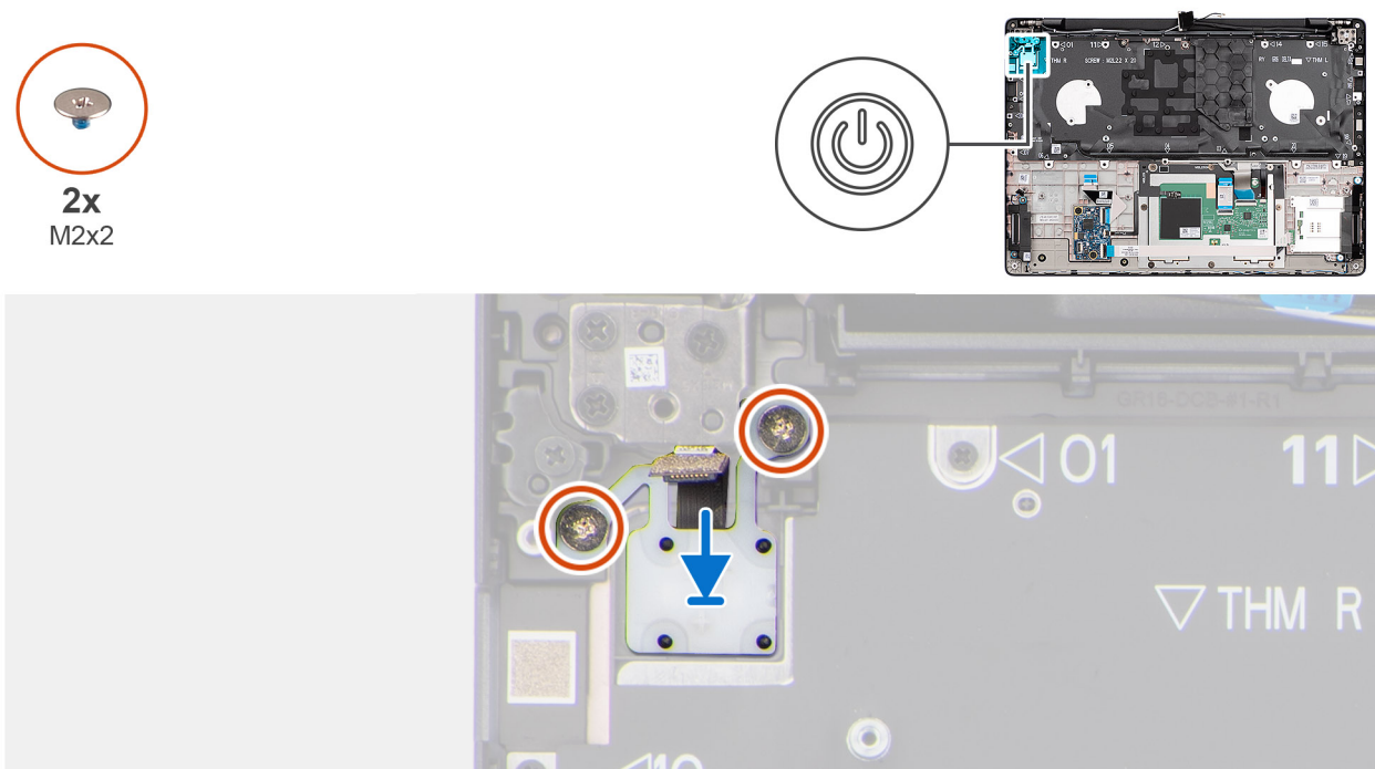
Abbeelding 82. De aan-uitknop plaatsen
