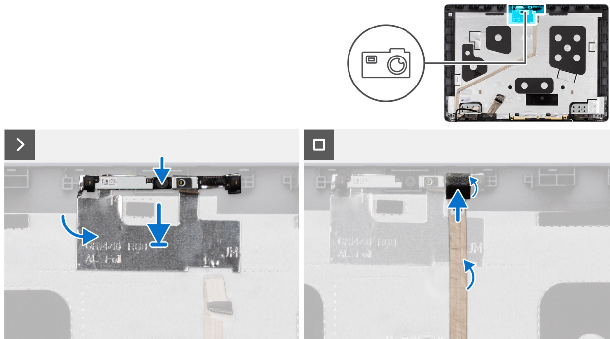
Afbeelding 70. De camera installeren
