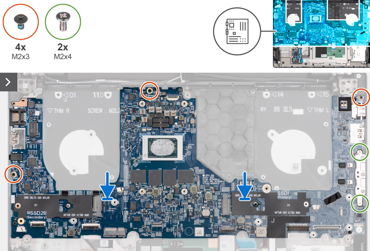
Afbeelding 77. De systeemkaart installeren
