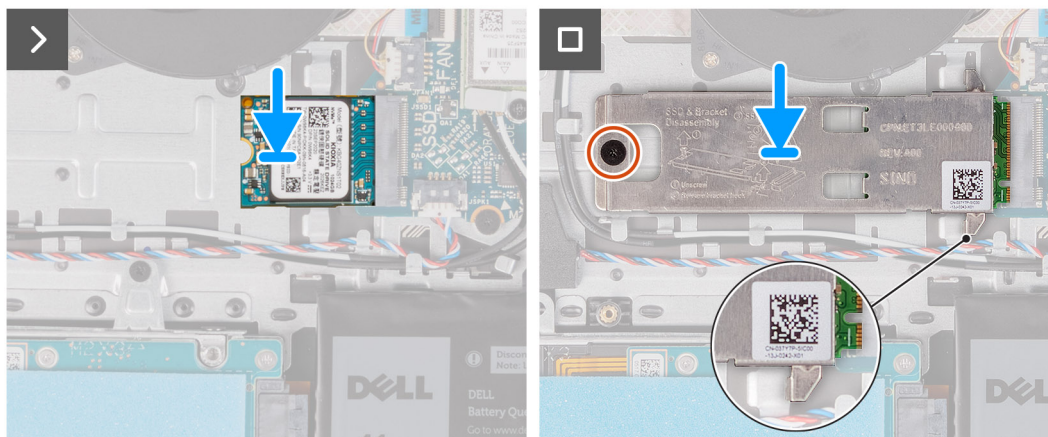
Abbildung 3. Installieren des Solid-State-Laufwerks
