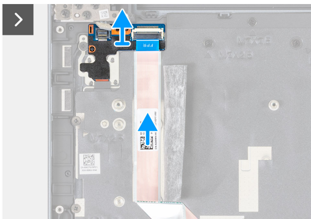
Afbeelding 127. De aan/uit-knopkaart verwijderen
