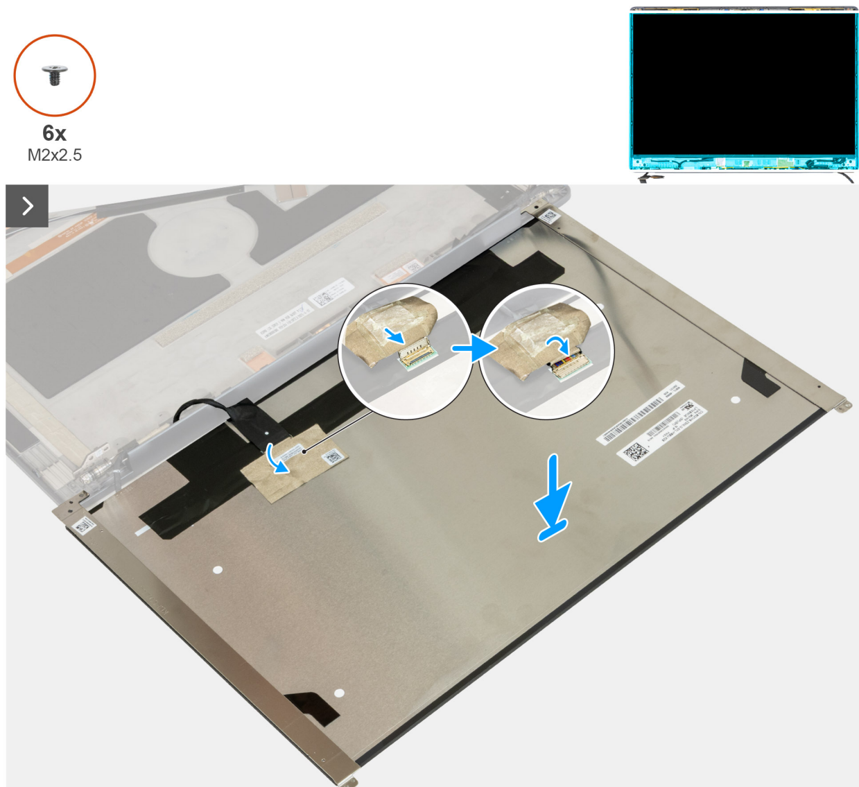
Afbeelding 93. Het beeldschermpaneel voor beeldschermen met touchscreen plaatsen
