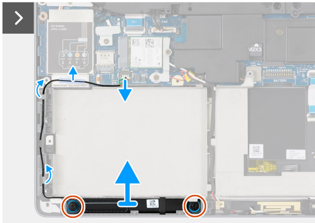
Afbeelding 81. De luidsprekers verwijderen
