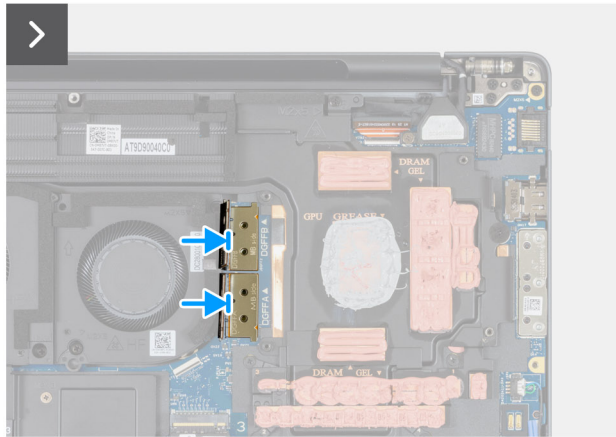
Afbeelding 58. De discrete FPC-balkconnector installeren
