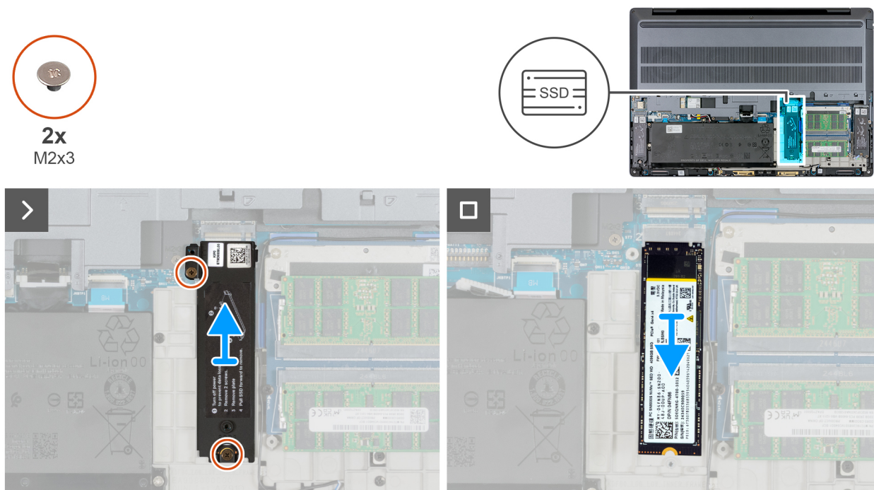
Afbeelding 36. De M.2 2280 SSD verwijderen uit slot 3 (SSD3)
