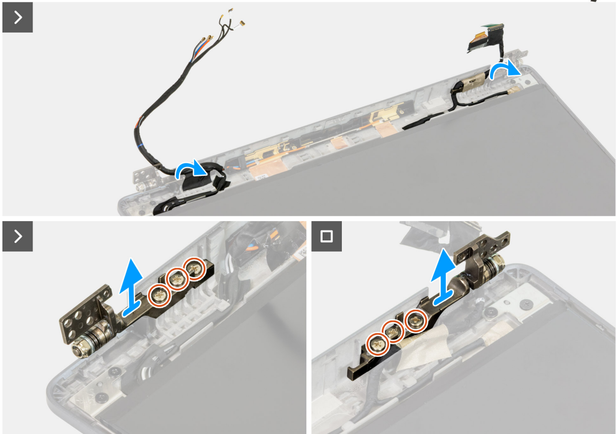
Afbeelding 99. De beeldschermcharnieren verwijderen
