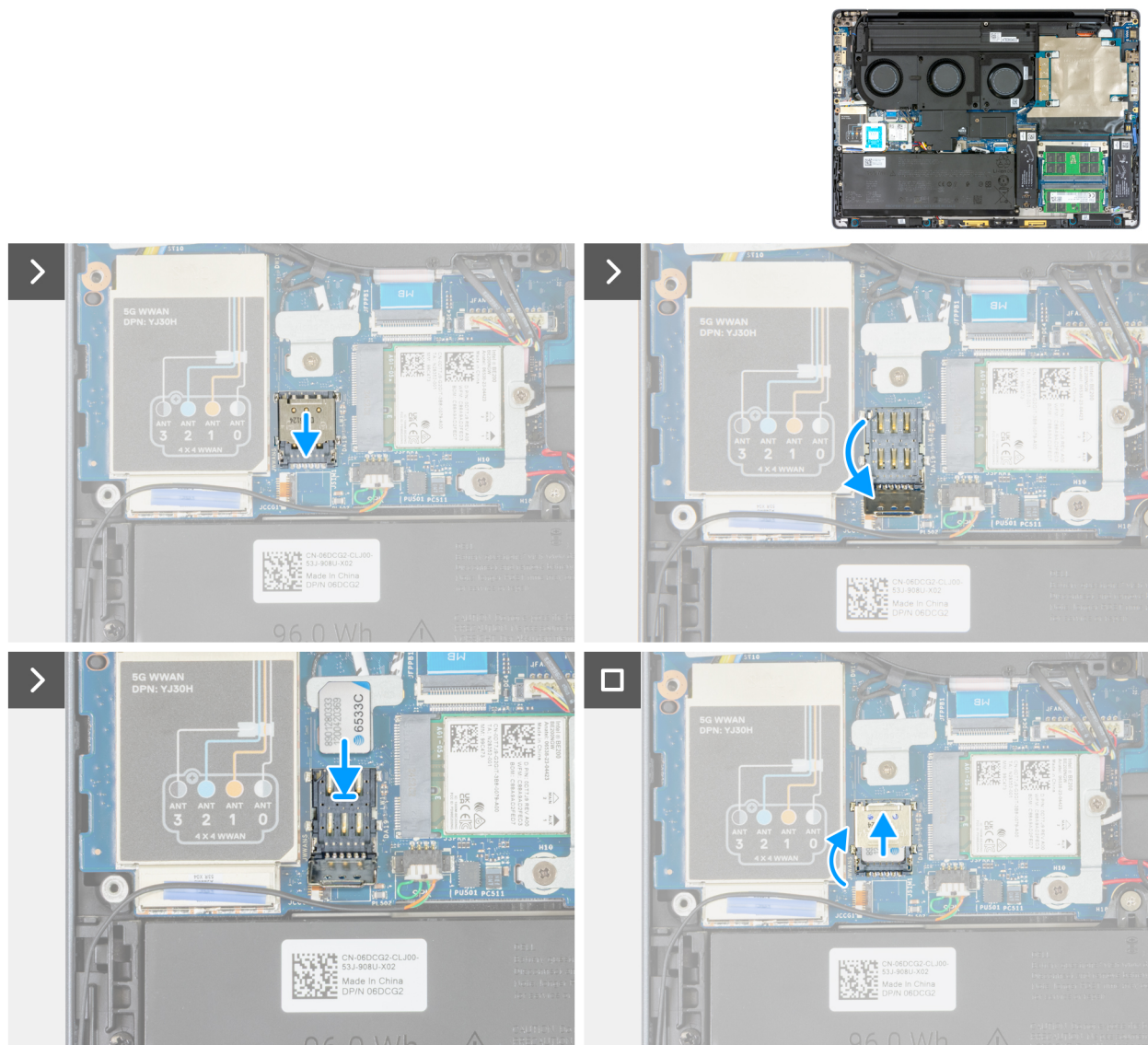
Afbeelding 49. De SIM-kaart installeren
