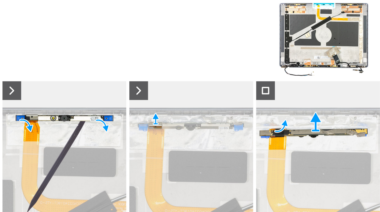
Afbeelding 103. De cameramodule verwijderen
