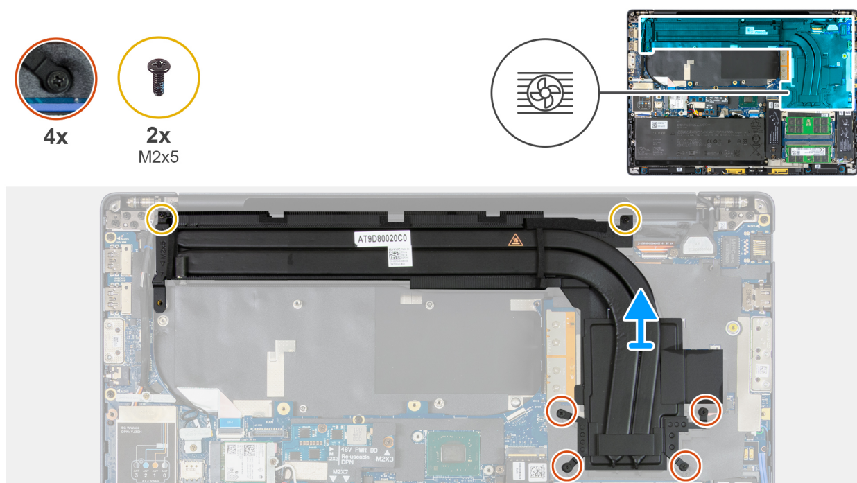
Abbeelding 73. De koelplaat verwijderen voor computers die worden geleverd met een geïntegreerde grafische kaart
