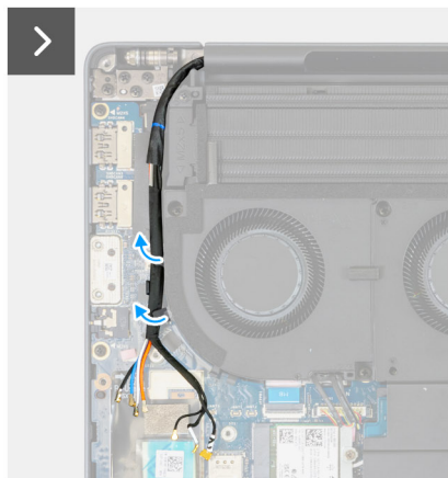
Afbeelding 63. De beeldscherm eenheid verwijderen
