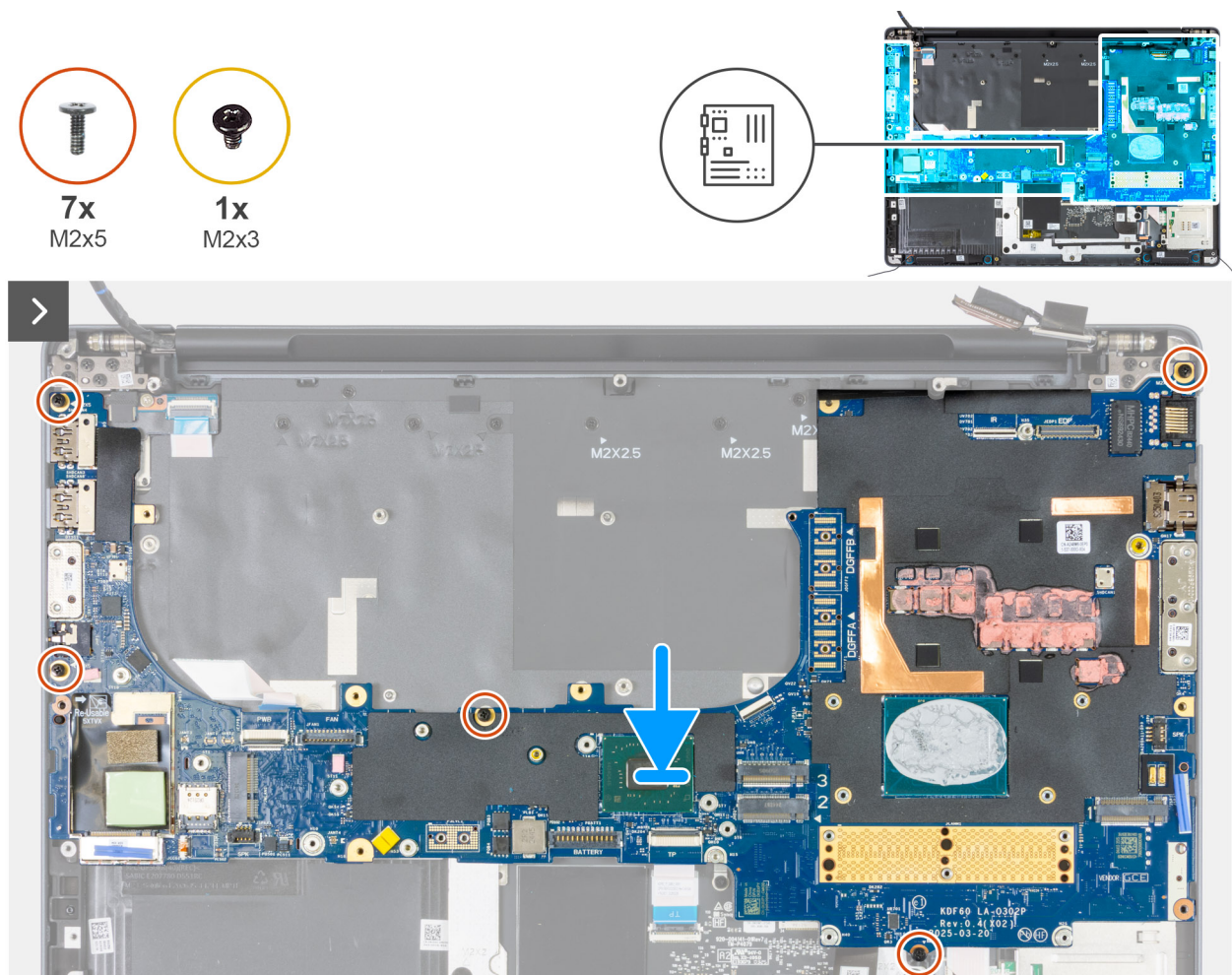
Afbeelding 115. De systeemkaart plaatsen
