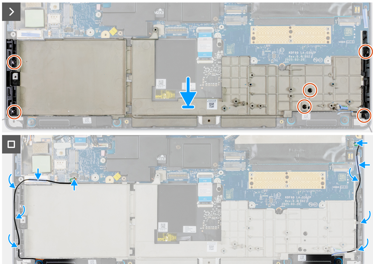
Afbeelding 80. Het binnenframe installeren
