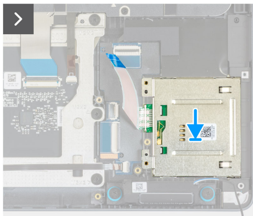
Abbildung 124. Installieren des Smartcardlesegeräts
