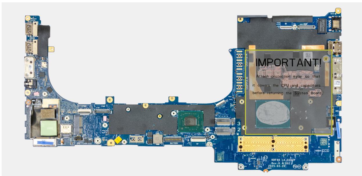
Abbildung 113. Vorbereiten der defekten Hauptplatine auf die Rücksendung
