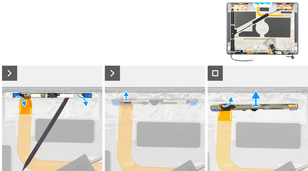
Abbildung 103. Entfernen des Kameramoduls
