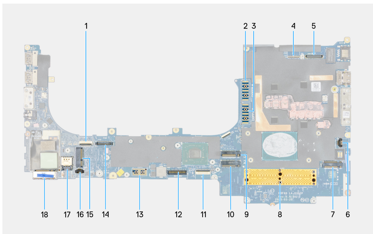
Abbildung 114. Komponenten der Hauptplatine
