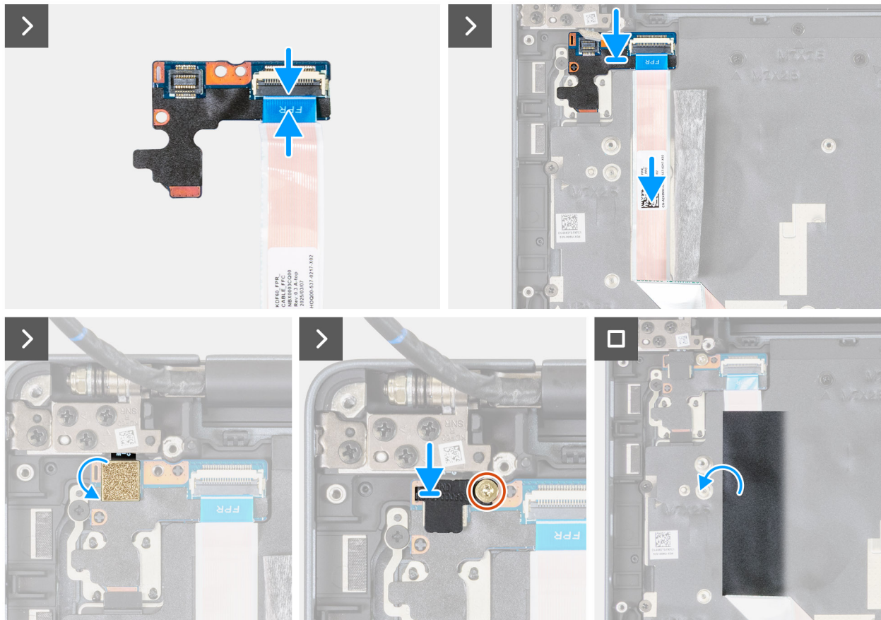
Abbildung 128. Einbauen der Netzschalterplatine
