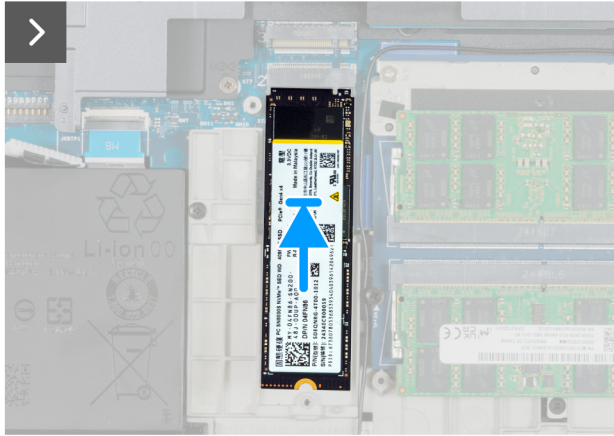
Abbildung 39. Installieren der M.2-2280-SSD in Steckplatz 2 (SSD2)
