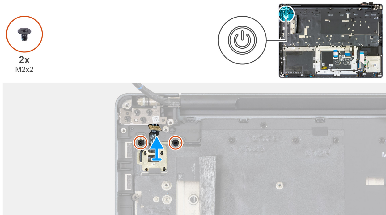
Abbildung 129. Entfernen des Netzschalters
