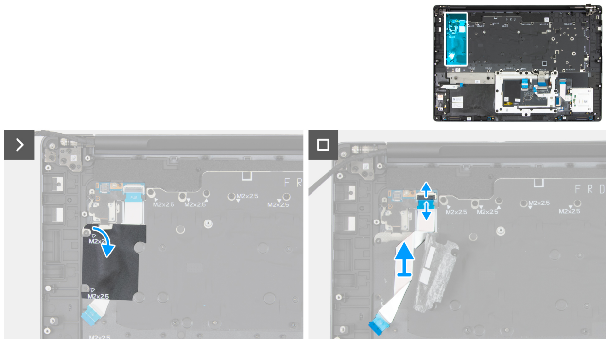
Abbildung 125. Entfernen des Kabels der Netzscharterplatine
