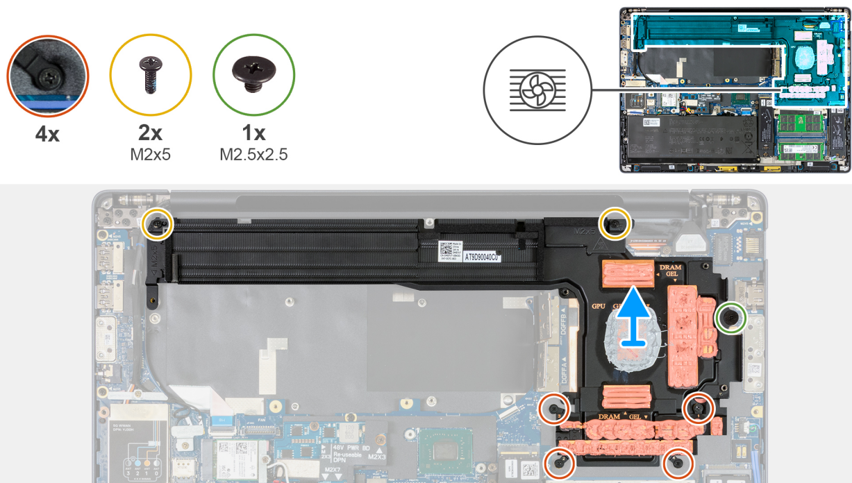
Abbildung 75. Entfernen des Kühlkörpers bei Computern mit separater Grafikkarte
