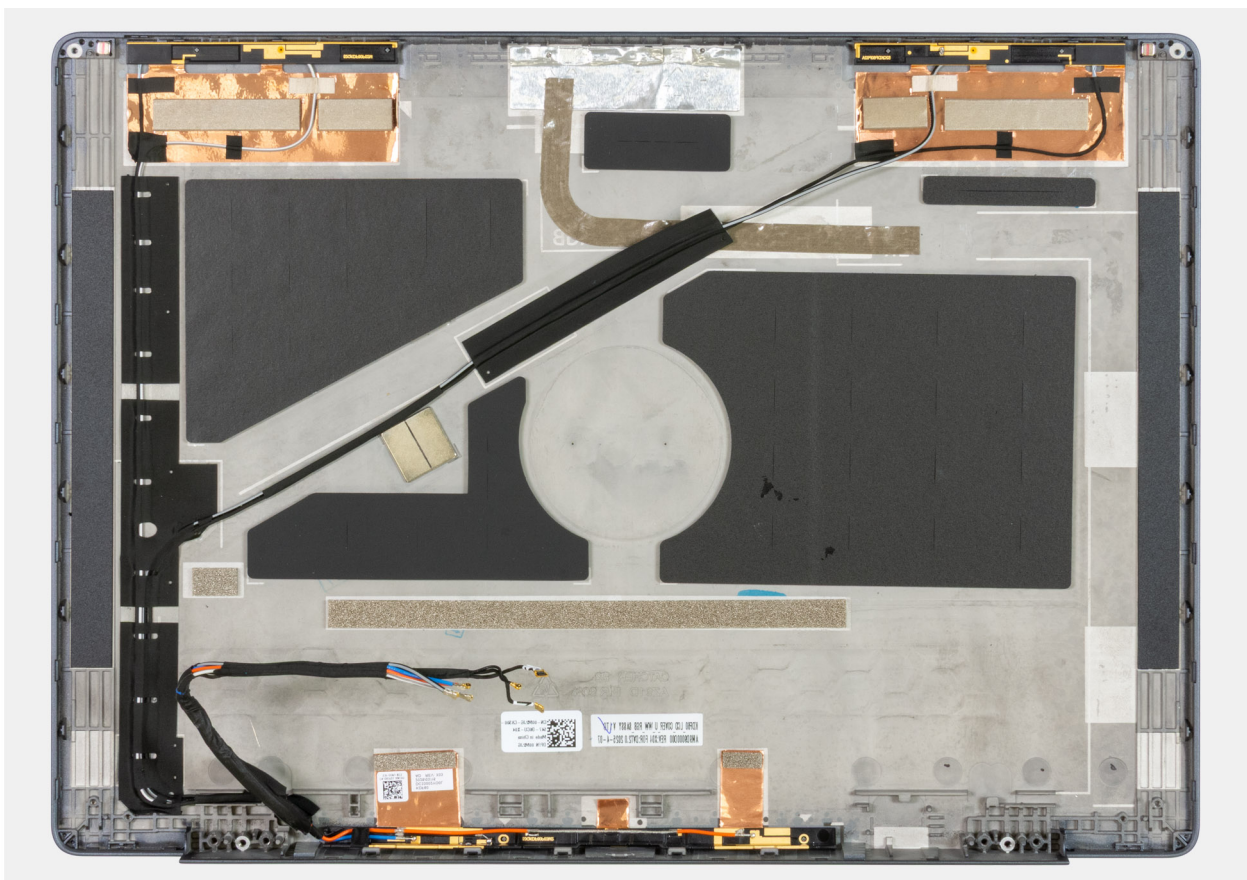
Abbildung 108. Hintere Bildschirmrückabdeckung
