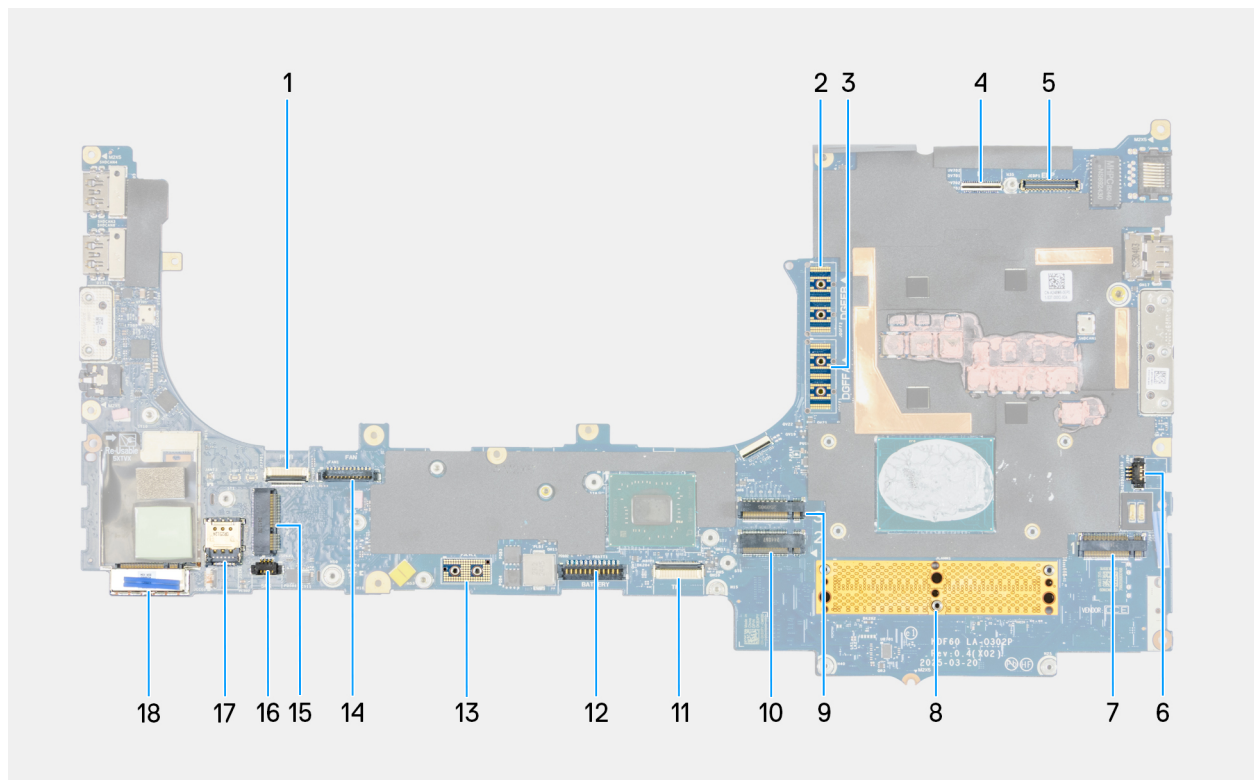
Abbildung 110. Komponenten der Hauptplatine
