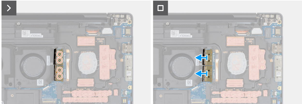
Abbildung 57. Entfernen des separaten FPC-Trägerverbinders
