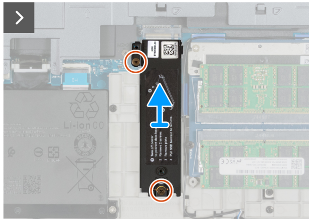
Abbildung 36. Entfernen der M.2-2280-SSD aus Steckplatz 3 (SSD3)
