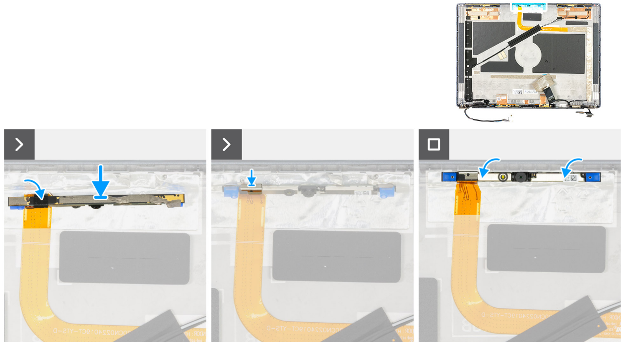
Abbildung 104. Installieren des Kameramoduls
