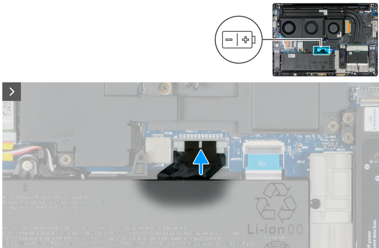
Abbildung 27. Verbinden des Akkukabels
