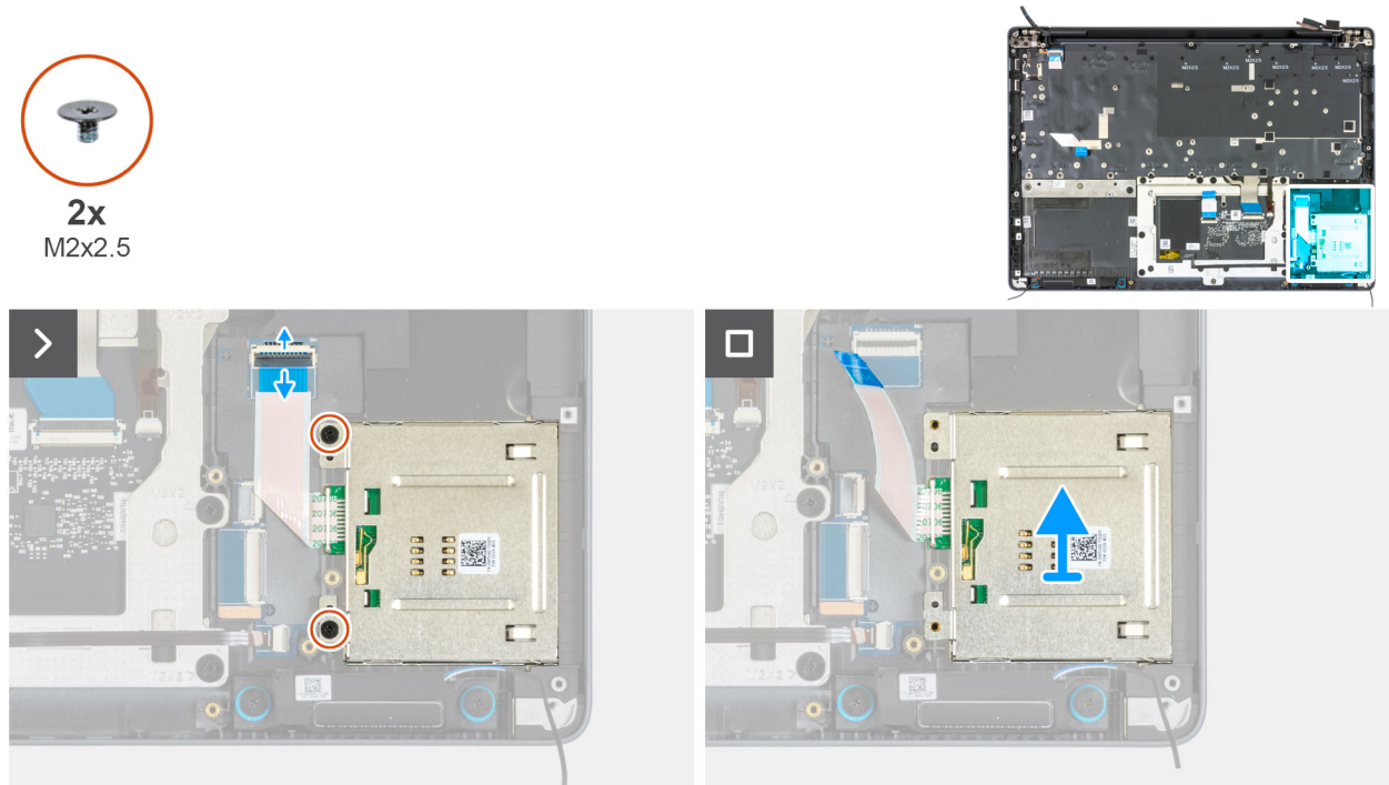
Abbildung 123. Entfernen des Smartcardlesegeräts
