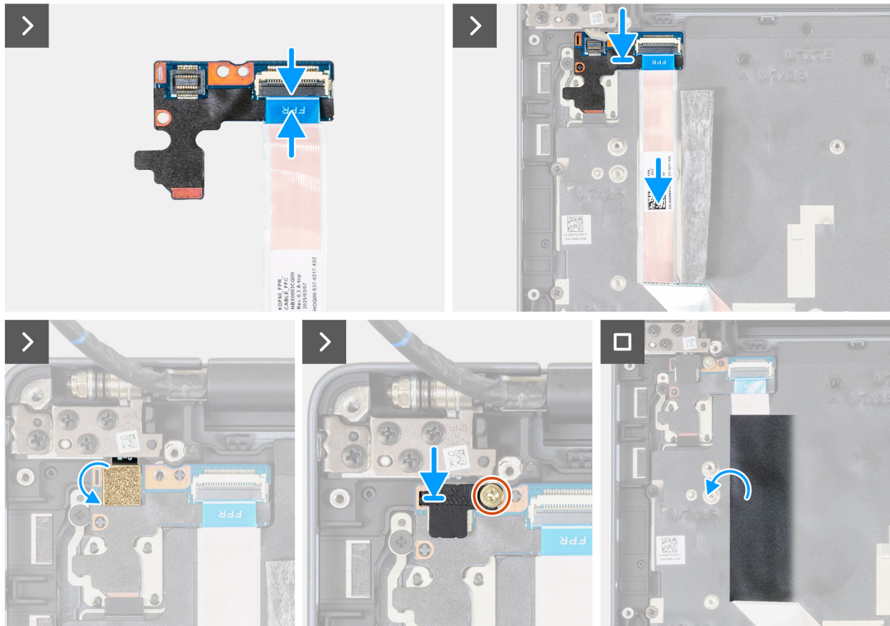
Figure 128. Installation de la carte du bouton d'alimentation
