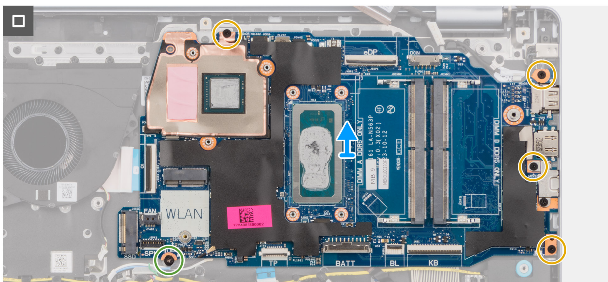
Ilustración 82. Extracción de la tarjeta madre
