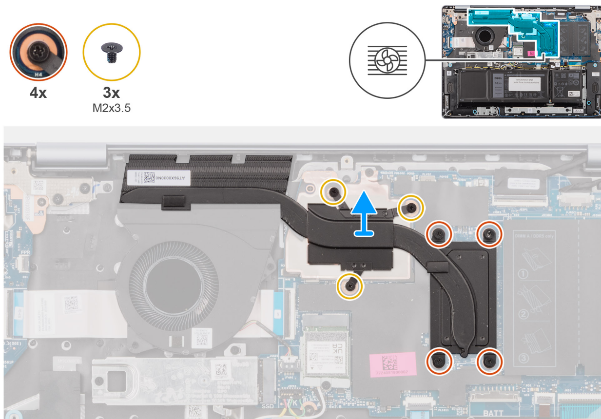
Ilustración 42. Extracción del disipador de calor (en computadoras que se envían con tarjeta de gráficos discretos)
