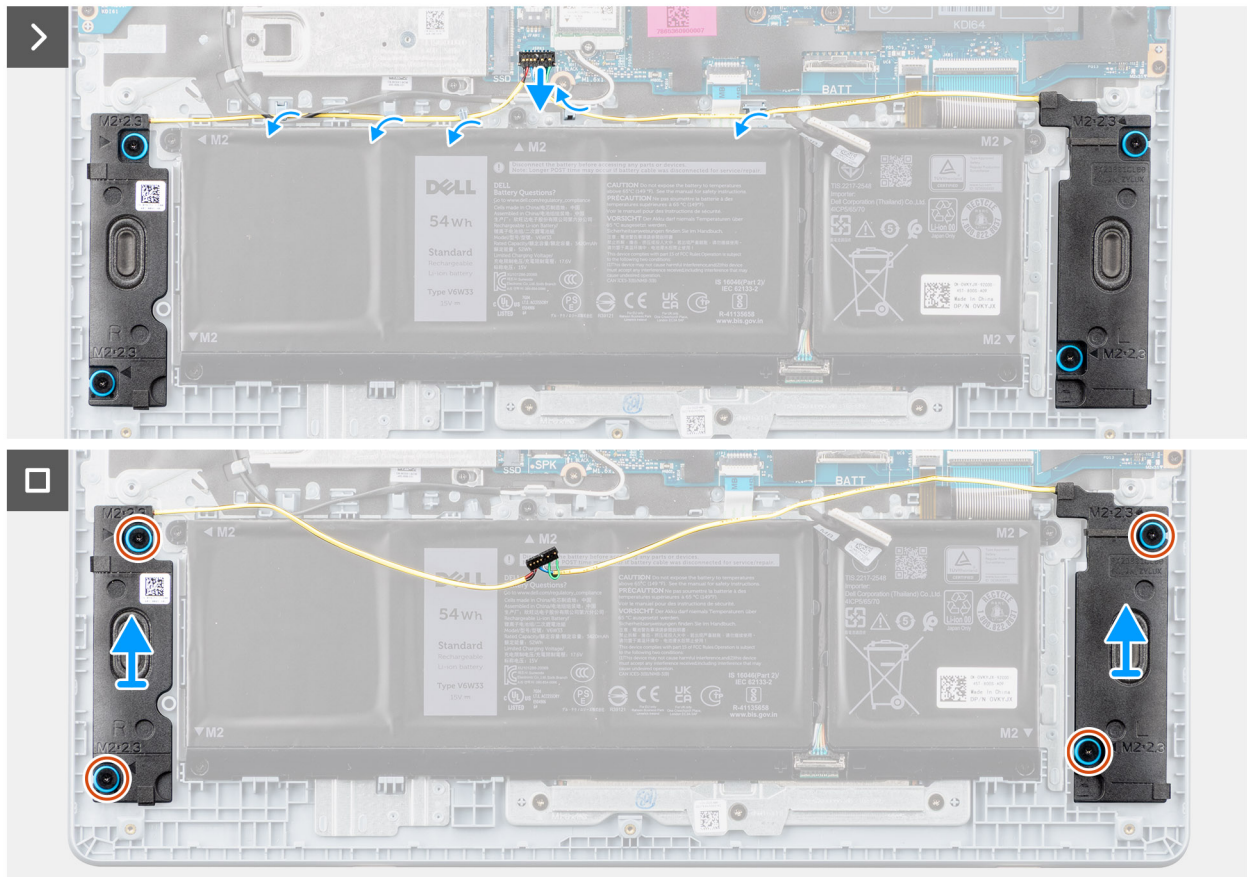
Ilustración 33. Extracción de los parlantes
