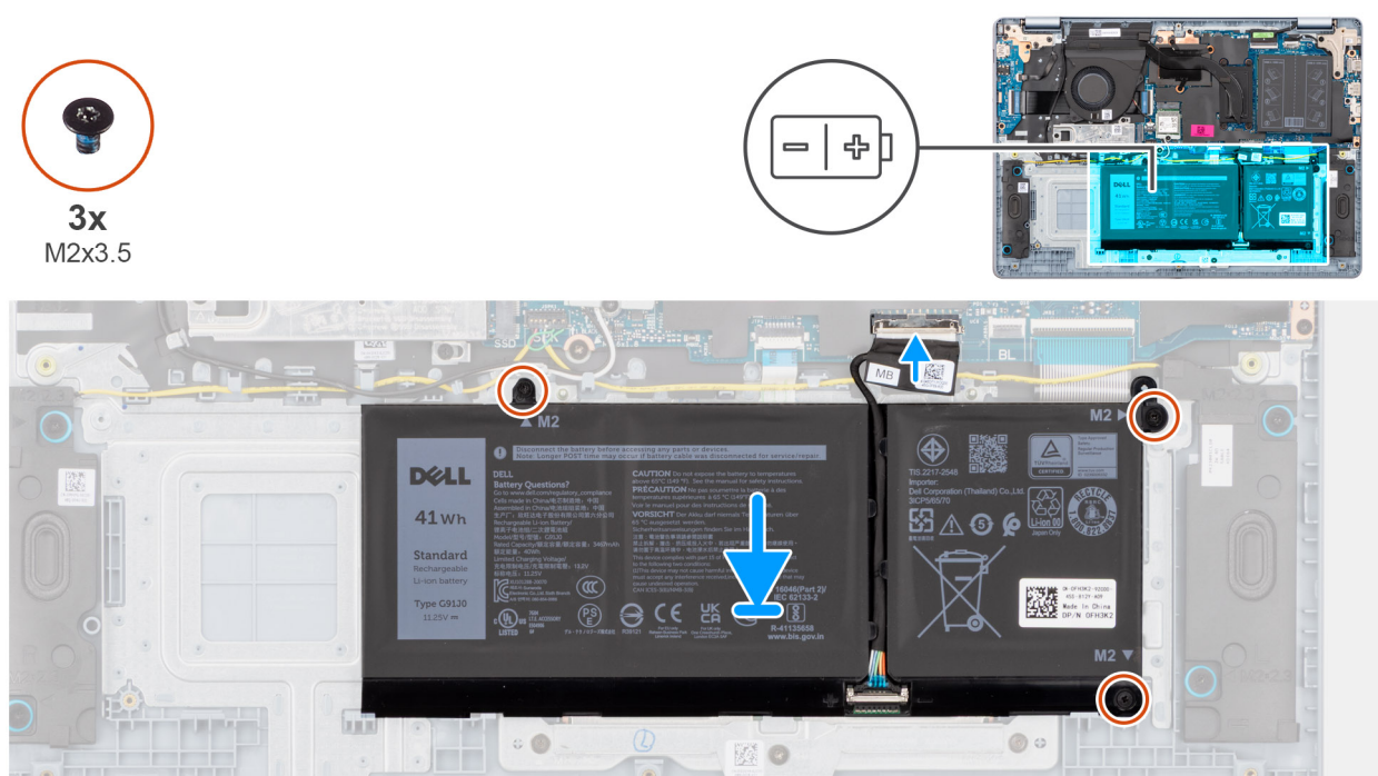
Ilustración 17. Instalación de la batería de 3 celdas
