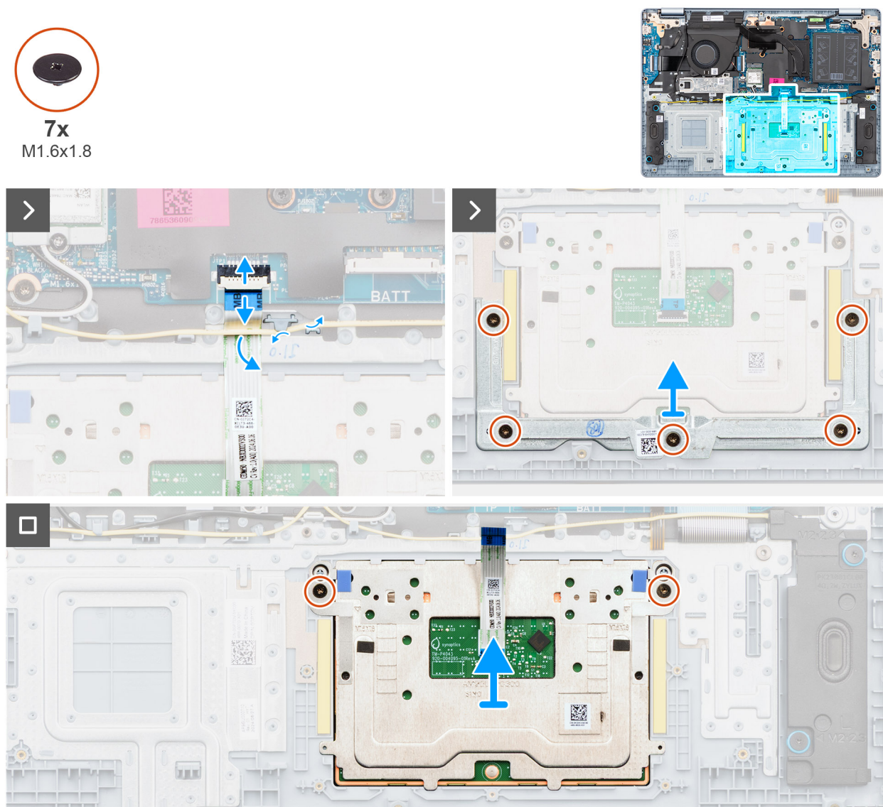
Ilustración 44. Extracción del panel táctil
