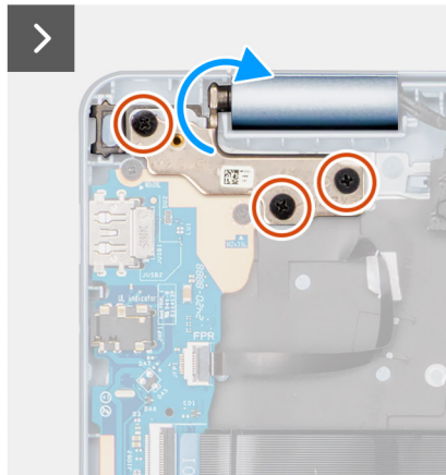
Ilustración 50. Extracción del ensamblaje de la pantalla
