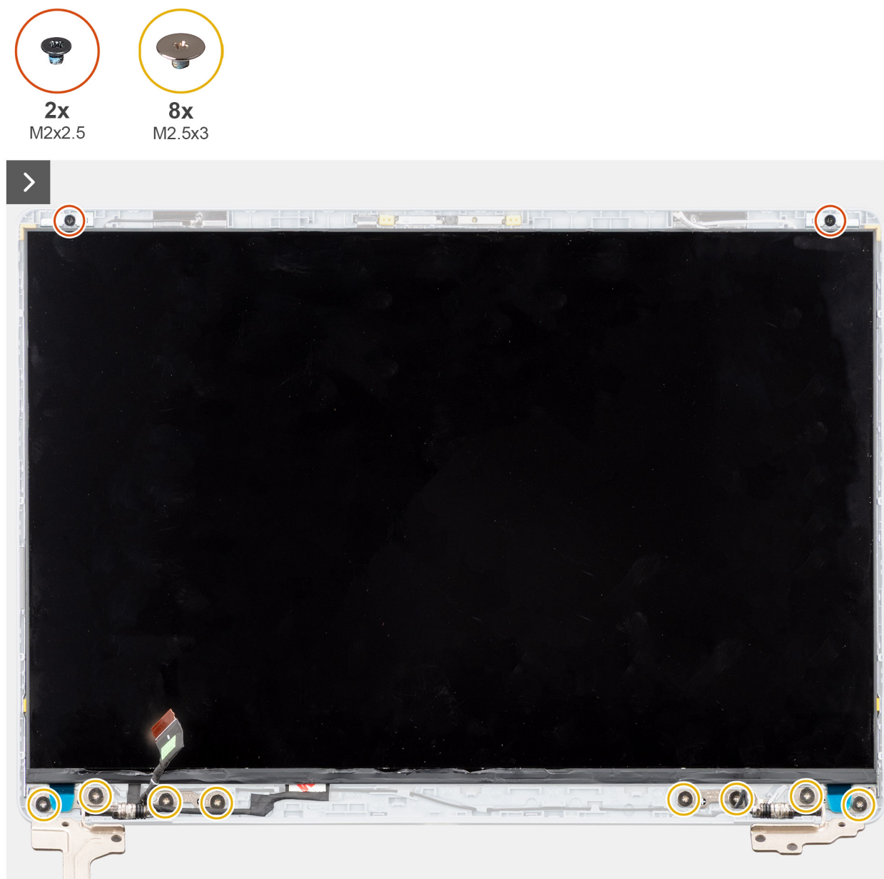
Ilustración 61. Extracción del panel de pantalla
