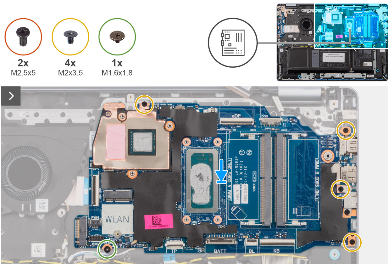
Ilustración 85. Instalación de la tarjeta madre
