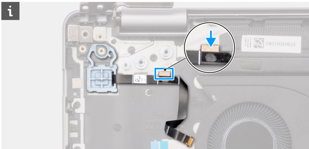
Ilustración 76. Adherir el cable del lector de huellas digitales al ensamblaje del teclado y el reposamanos
