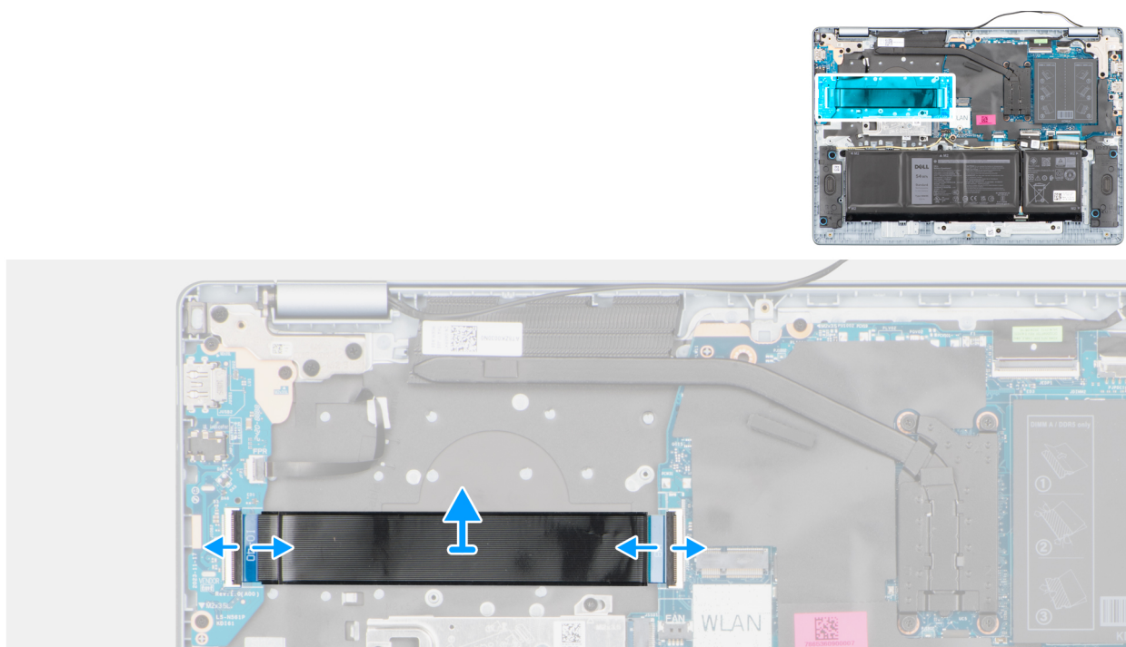
Ilustración 46. Extracción del cable de la placa de I/O
