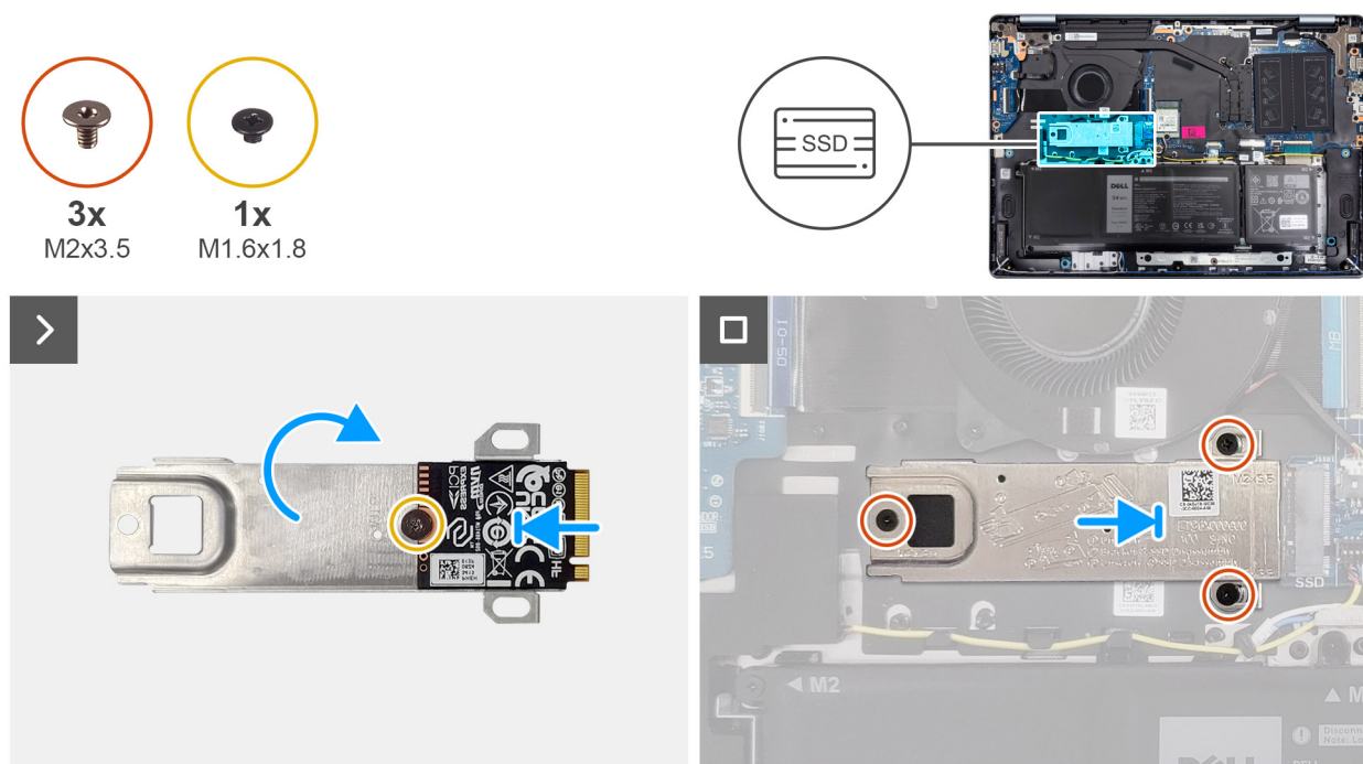
Ilustración 29. Instalación de la unidad de estado sólido
