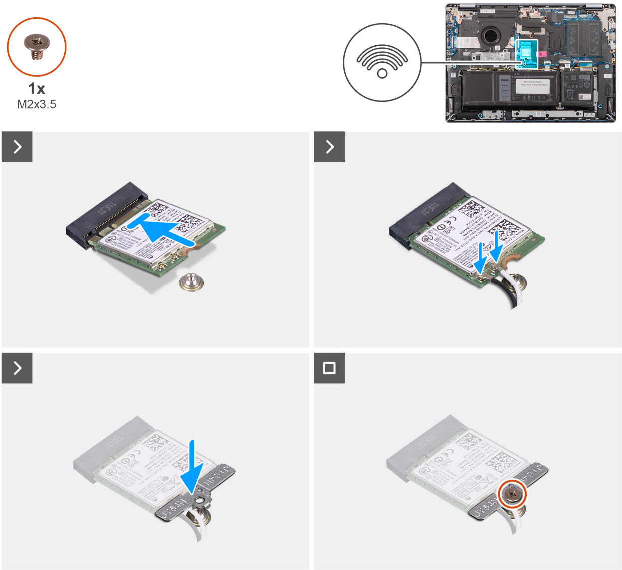
Ilustración 31. Instalación de la tarjeta inalámbrica
