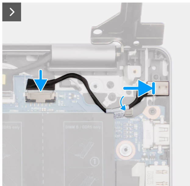
Ilustración 78. Instalación del puerto del adaptador de alimentación
