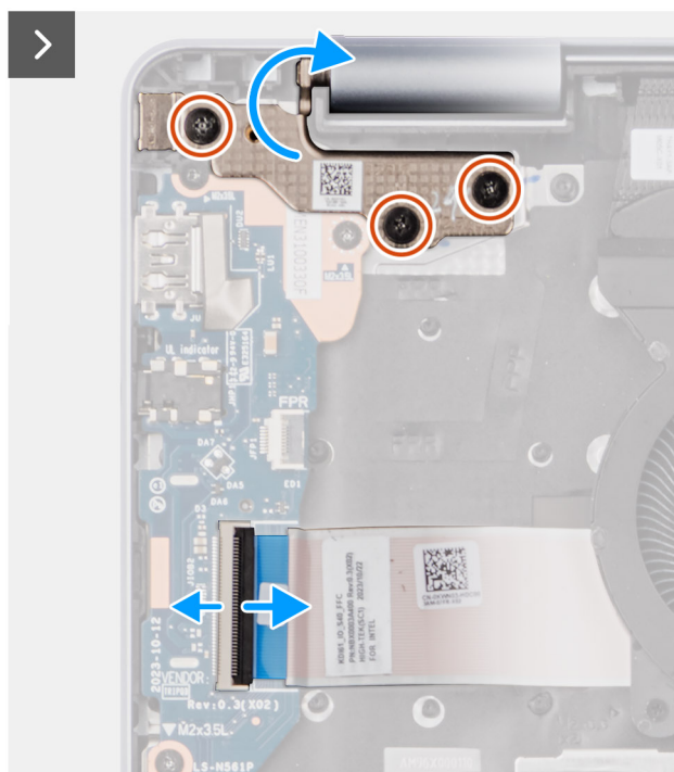
Ilustración 48. Extracción de la placa de I/O
