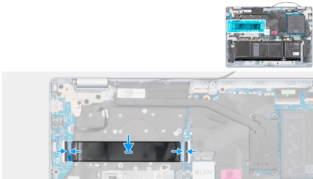
Ilustración 47. Instalación del cable de la placa de I/O
