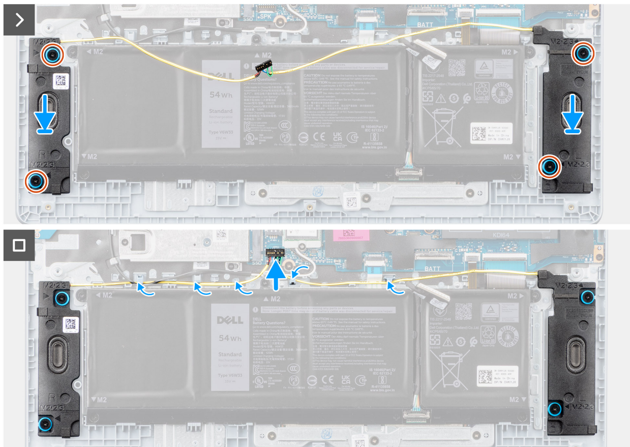
Ilustración 35. Instalación de los parlantes
