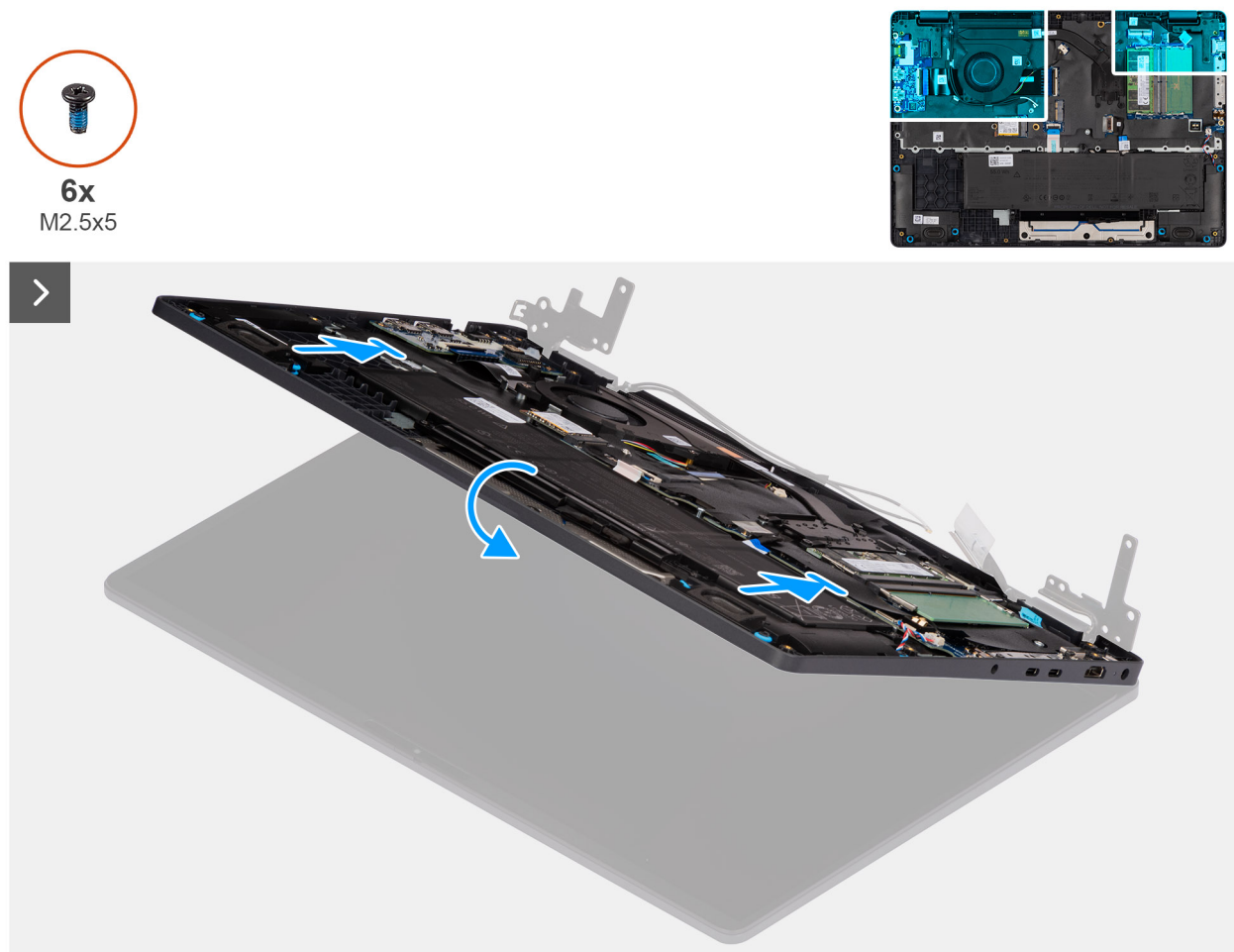
Figura 96. Installazione del gruppo del display
