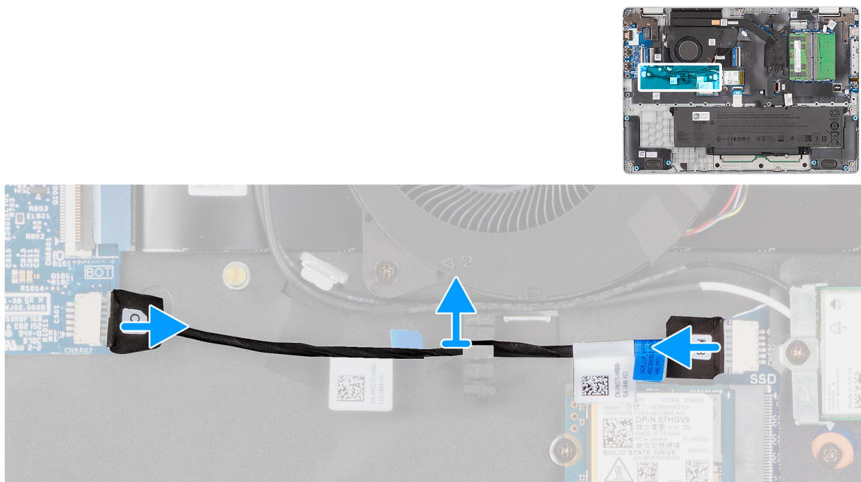
Figura 45. Rimozione del cavo vPro
