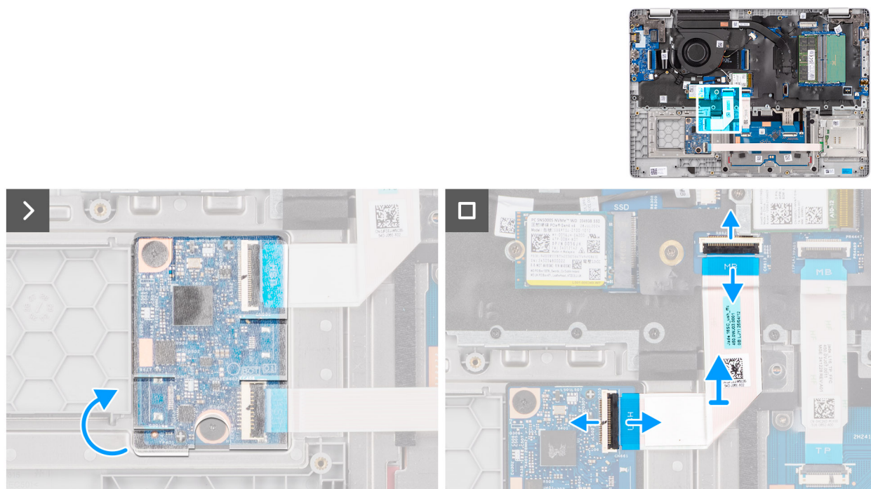
Figura 35. Rimozione dell'FPC della scheda USH
