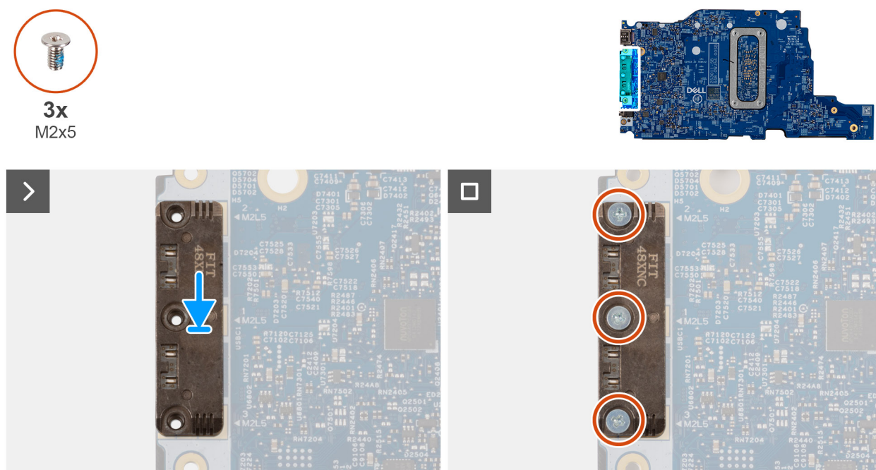
Figura 78. Installazione del modulo USB Type-C
