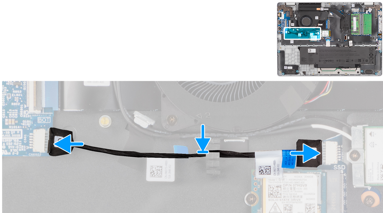
Figura 46. Installazione del cavo vPro
