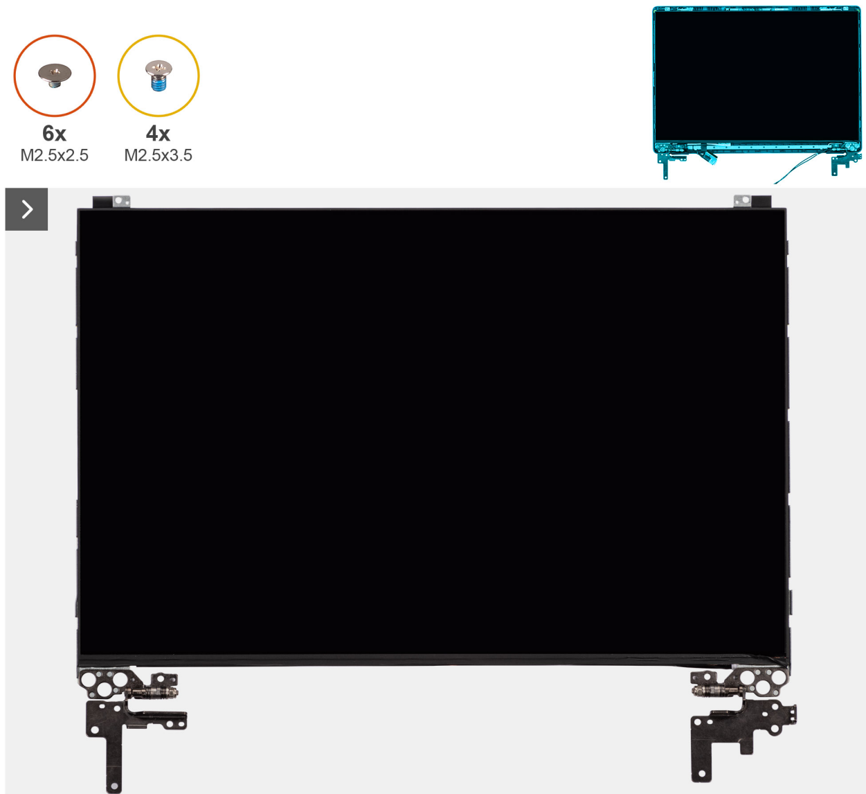
Figura 109. Installazione del gruppo del pannello del display
