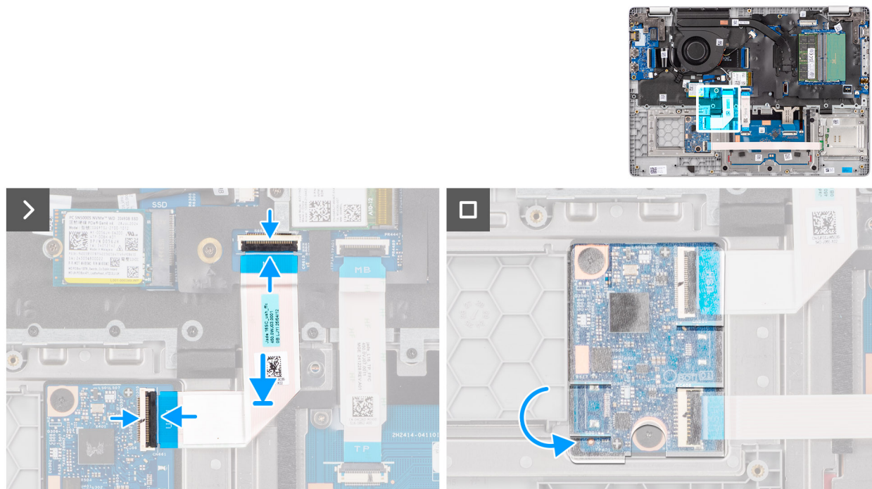
Figura 36. Installazione dell FPC della scheda USH
