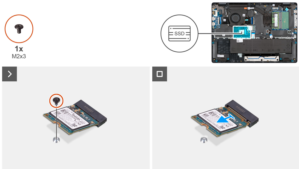
Figura 23. Rimozione dell'SSD
