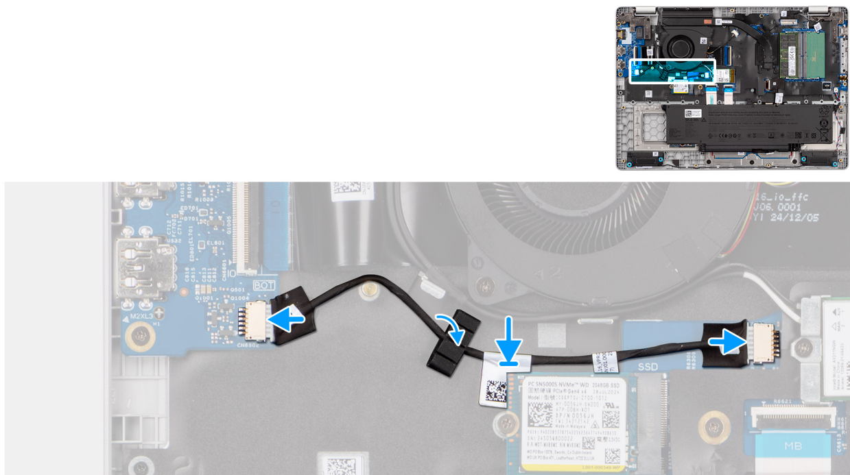
Figura 48. Installazione del cavo vPro
