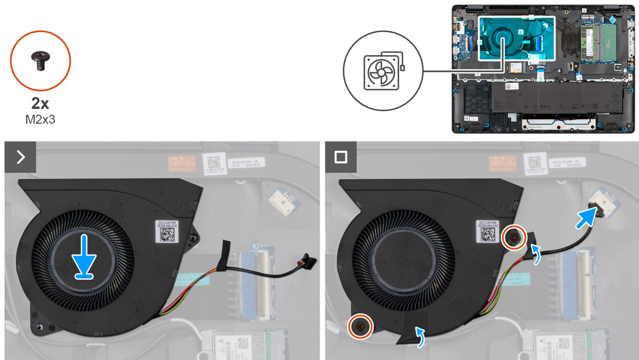
Figura 34. Installazione della ventola
