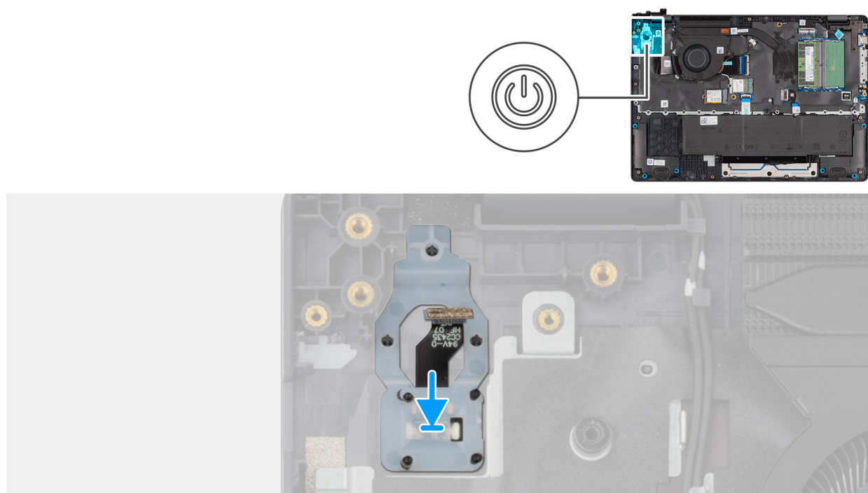
Figura 56. Installazione del pulsante di accensione con lettore di impronte digitali
