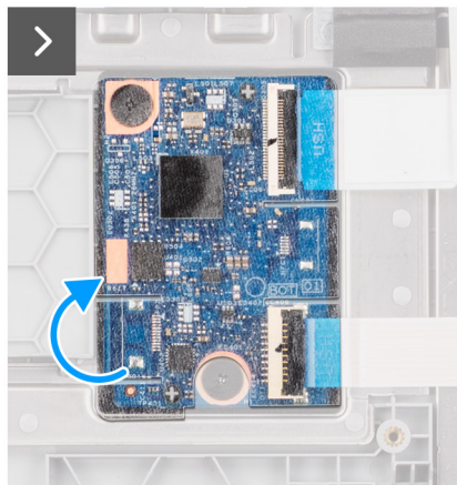
Figura 37. Rimozione della scheda USH
