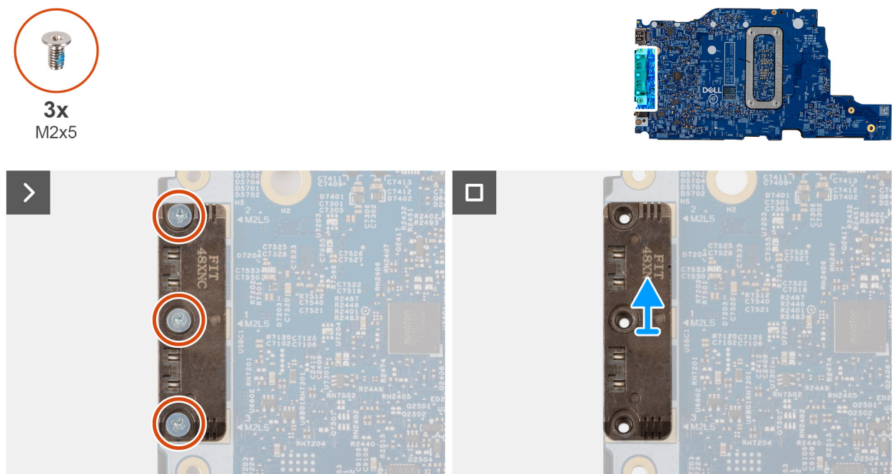
Figura 77. Rimozione del modulo USB Type-C
