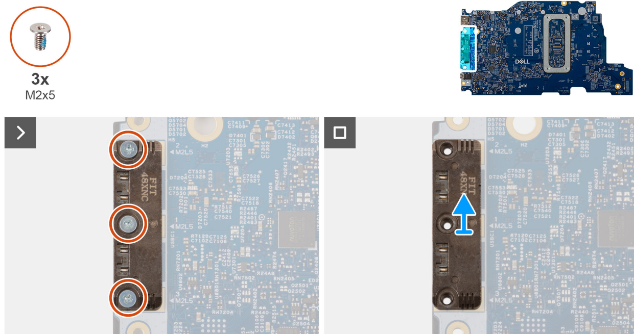
Figura 75. Rimozione del modulo USB Type-C
