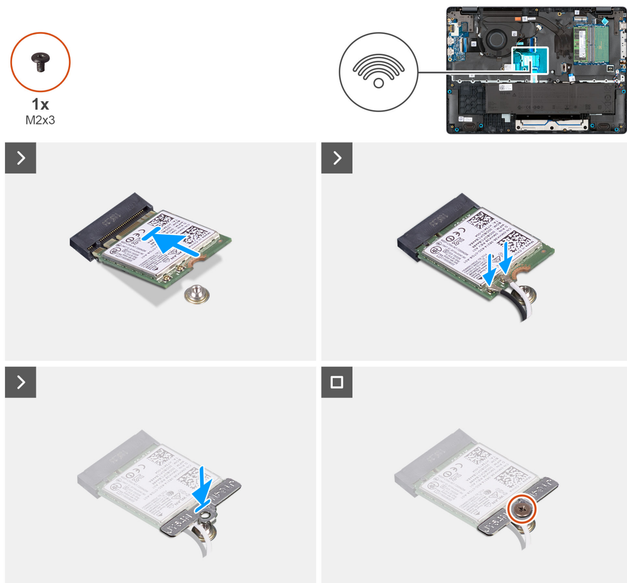
Figura 26. Installazione della scheda wireless
