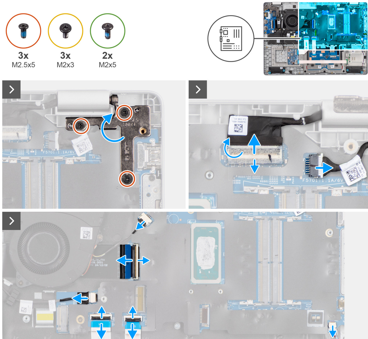
Figura 70. Rimozione della scheda di sistema
