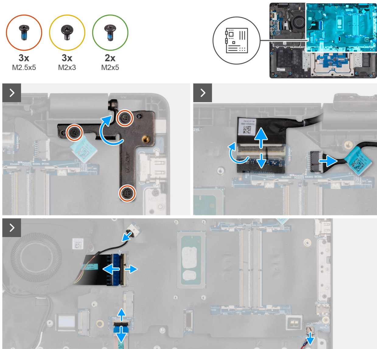
Figura 58. Rimozione della scheda di sistema
