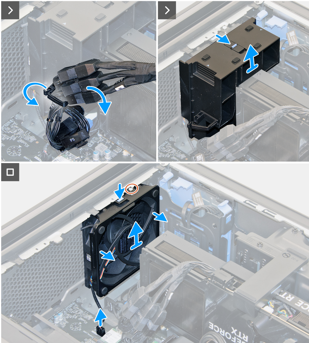
Abbildung 41. Entfernen des unteren vorderen Gehäuselüfters
