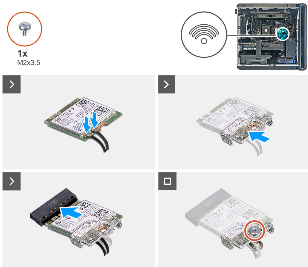
Abbildung 40. Installieren der Wireless-Karte
