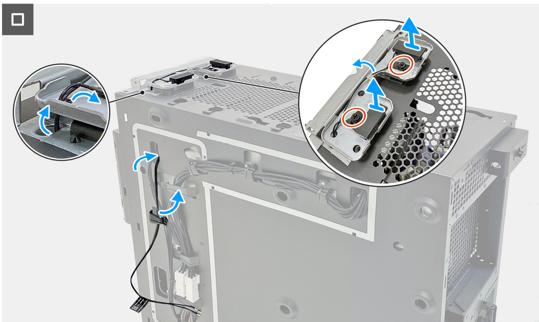
Abbildung 57. Entfernen der Antenne
