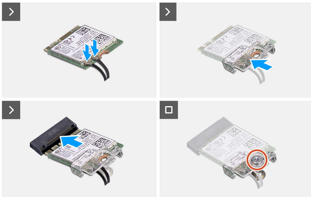
Abbildung 40. Installieren der Wireless-Karte
