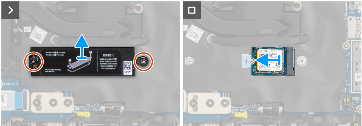
Figure 33. Retrait du disque SSD M.2 2230
