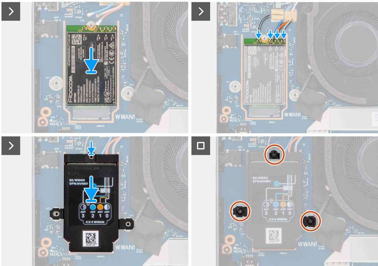
Figure 32. Installation de la carte WWAN
