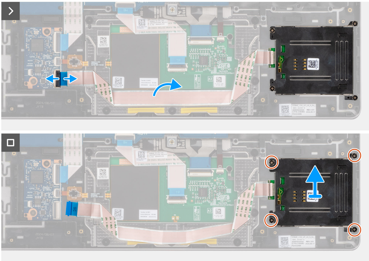
Figure 45. Retrait du lecteur de carte à puce
