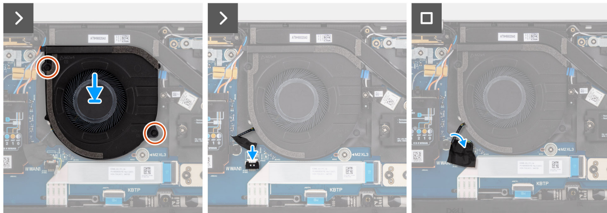
Figure 40. Installation du ventilateur
