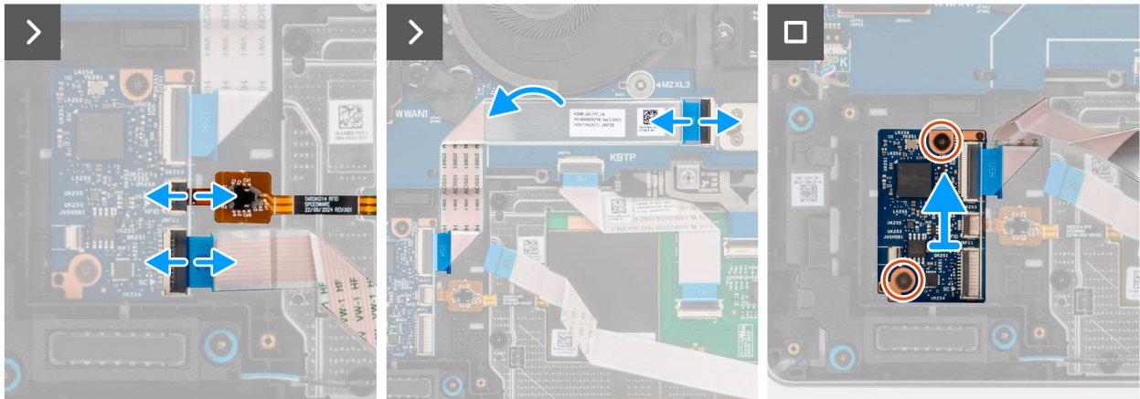
Figure 43. Retrait de la carte USH
