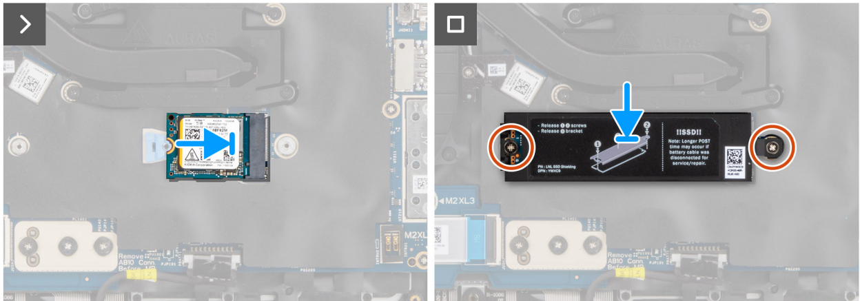
Figure 34. Installation du disque SSD M.2 2230
