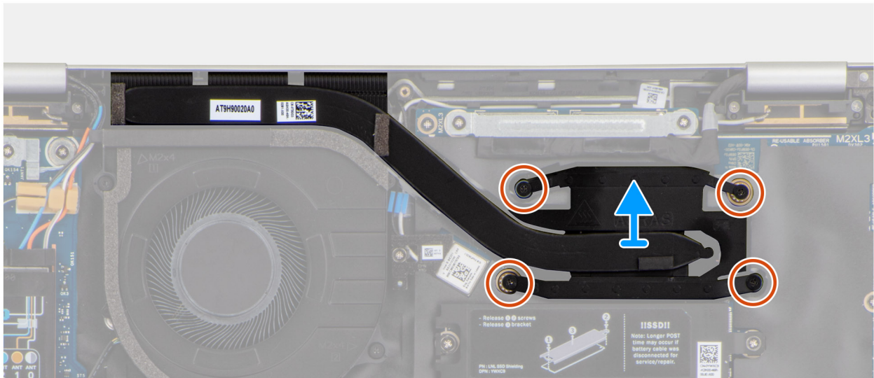
Figure 41. Retrait du dissipateur de chaleur
