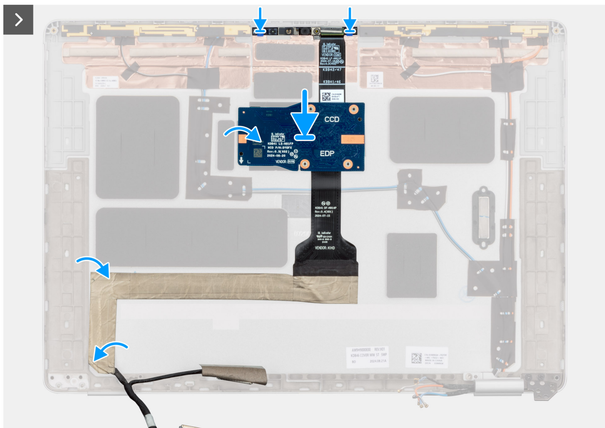
Figure 76. Installation du câble de la caméra et de l'écran
