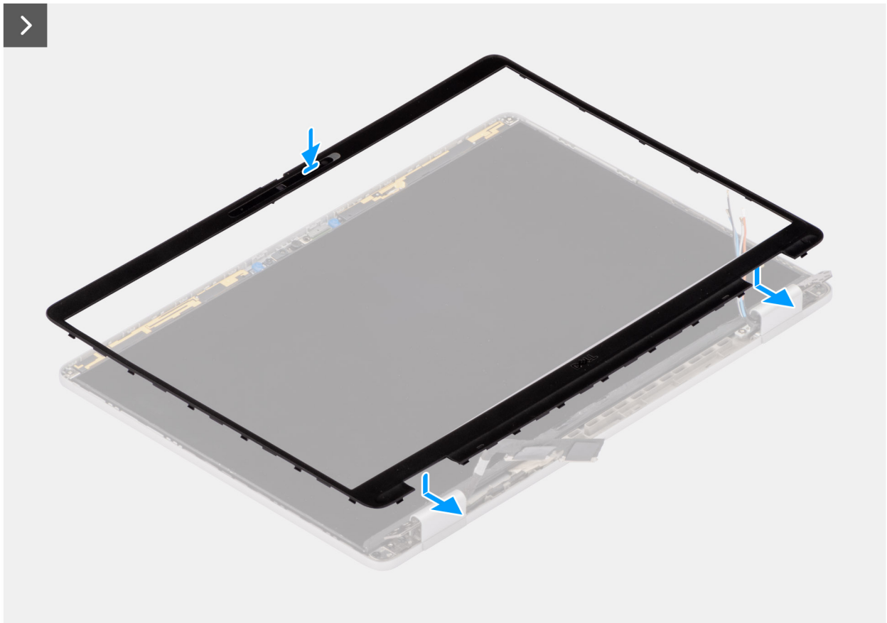
Figure 66. Installation de la bordure d'écran
