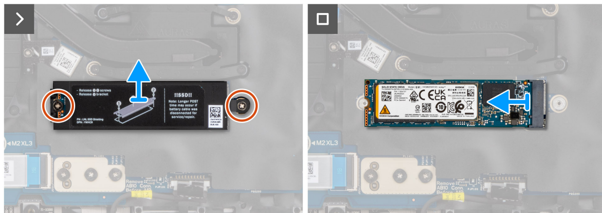
Figure 35. Retrait du disque SSD M.2 2280
