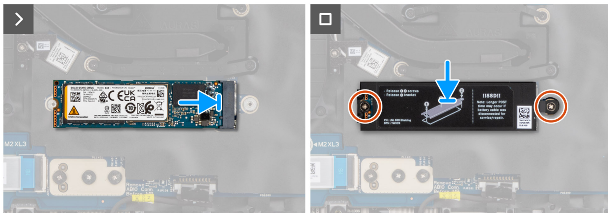
Figure 36. Installation du disque SSD M.2 2280
