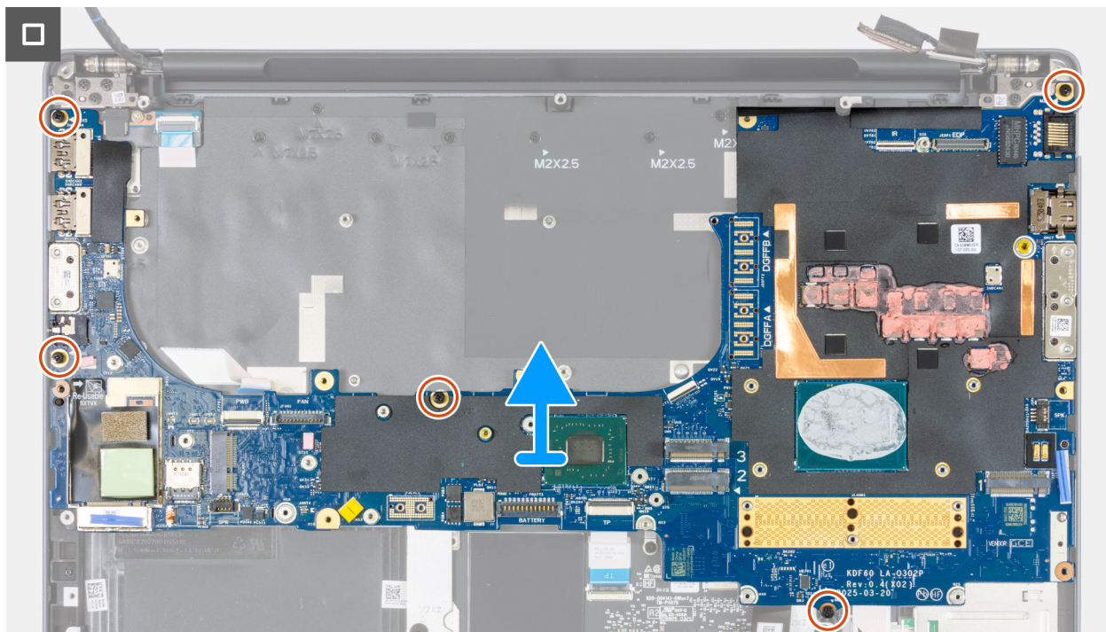
Abbildung 112. Entfernen der Systemplatine
