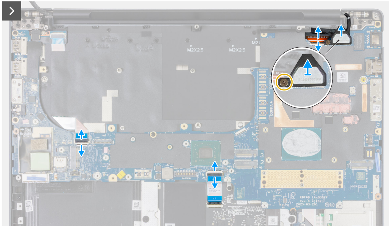
Abbildung 111. Entfernen der Systemplatine
