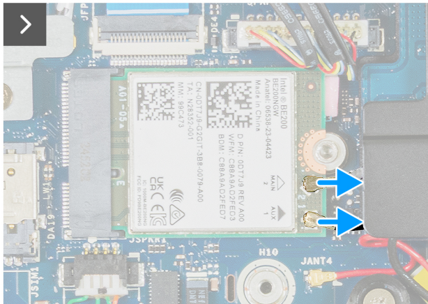
Abbildung 46. Entfernen der WLAN-Karte
