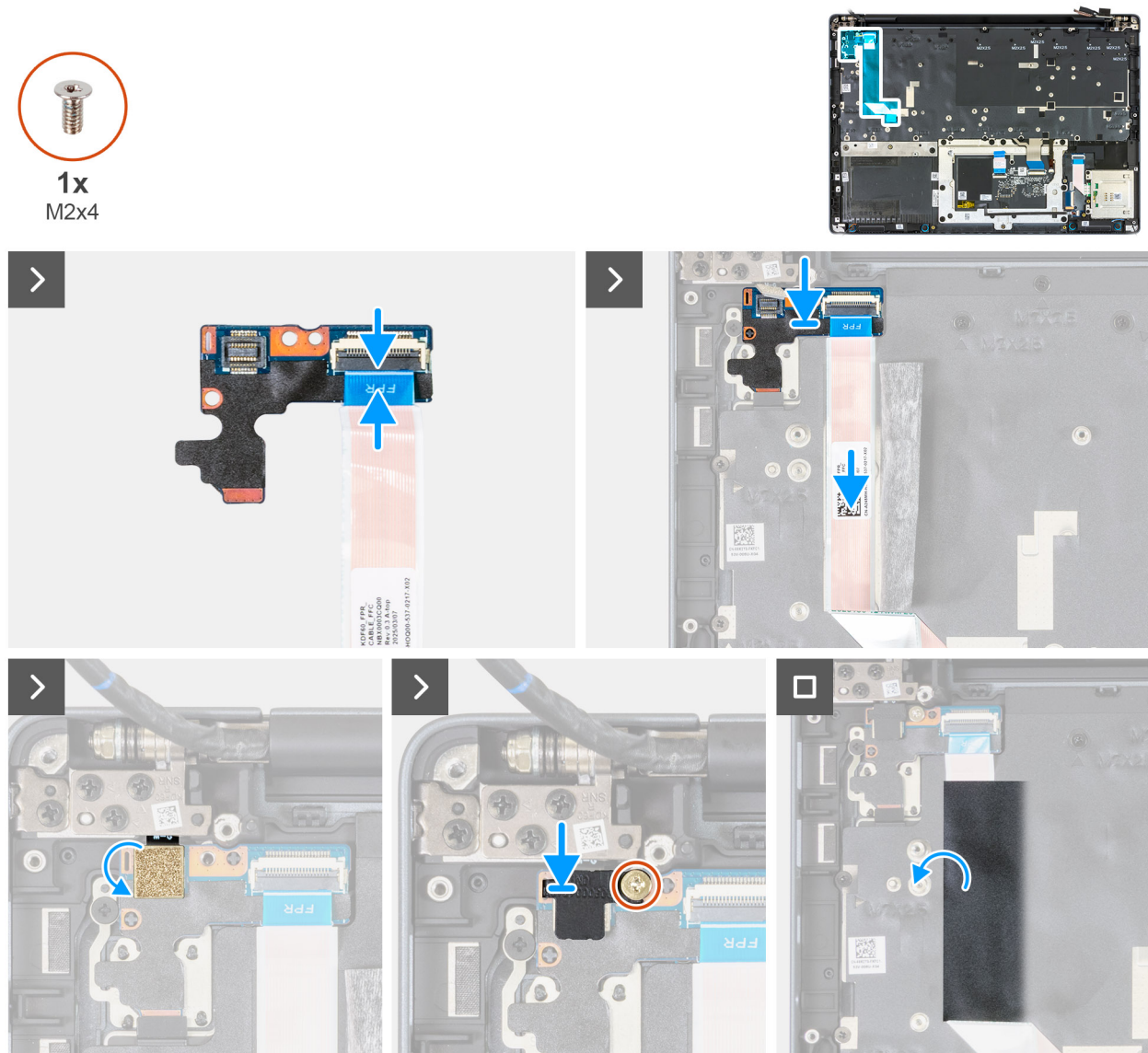
Abbildung 128. Einbauen der Netzschalterplatine
