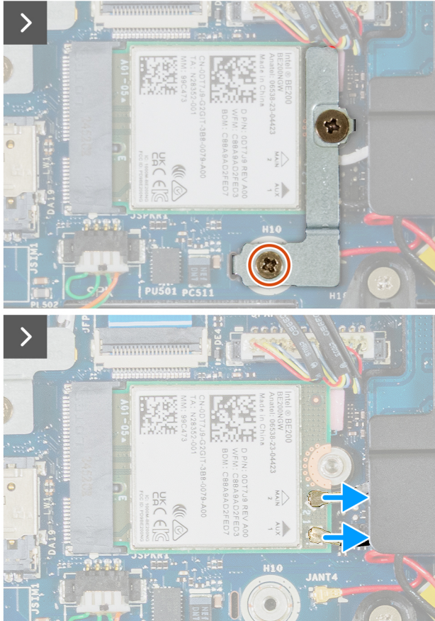
Abbildung 46. Entfernen der WLAN-Karte
