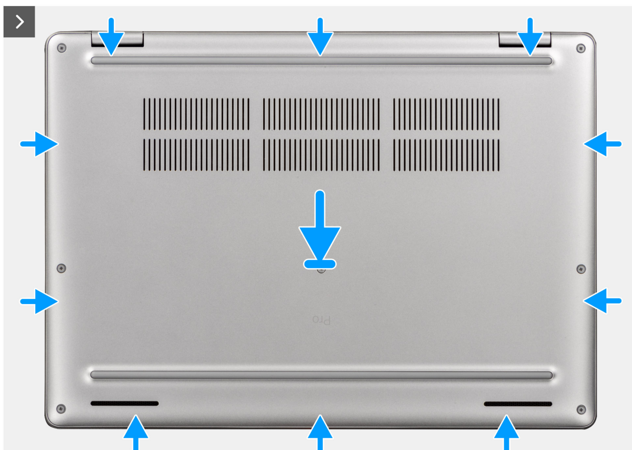
Afbeelding 26. De onderplaat installeren
