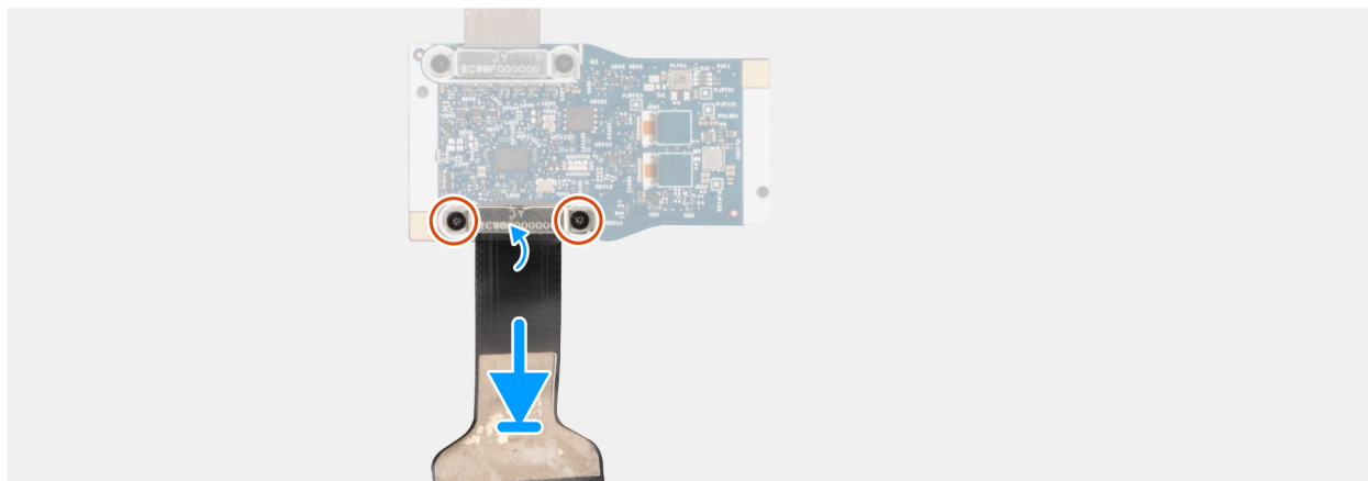
Afbeelding 91. De beeldschermkabel voor de MIPI-camera installeren
