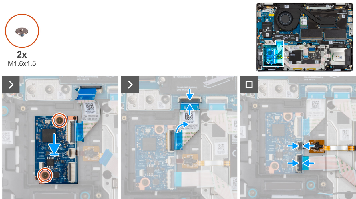
Afbeelding 47. De USH-kaart plaatsen
