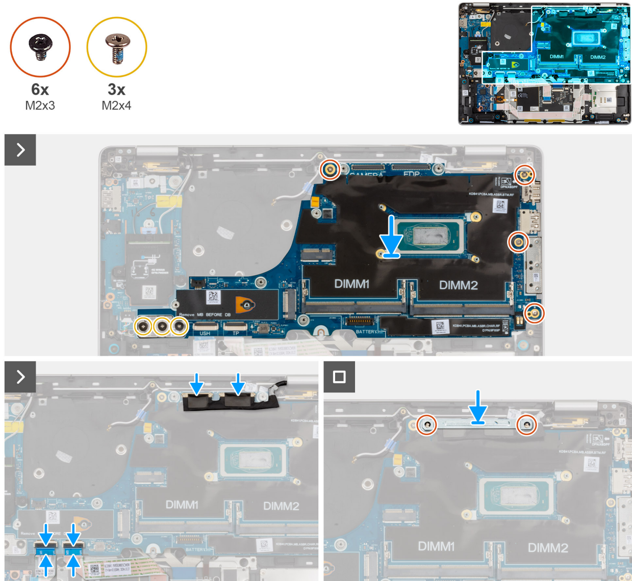
Afbeelding 53. De systeemkaart installeren
