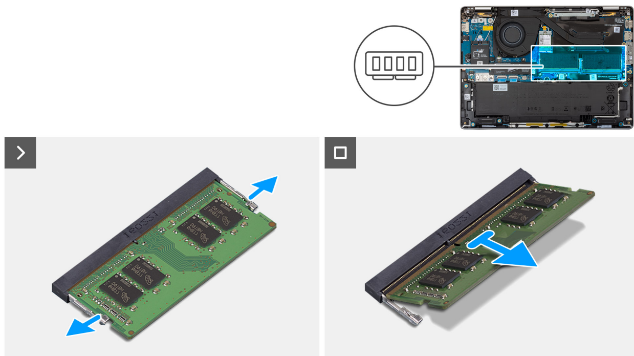
Afbeelding 32. De geheugenmodule verwijderen
