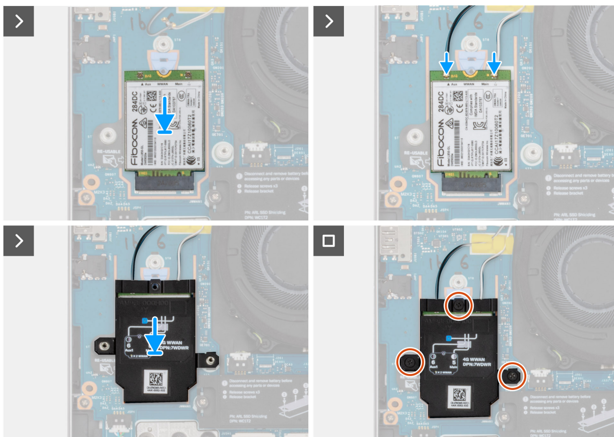
Afbeelding 35. De WWAN-kaart installeren
