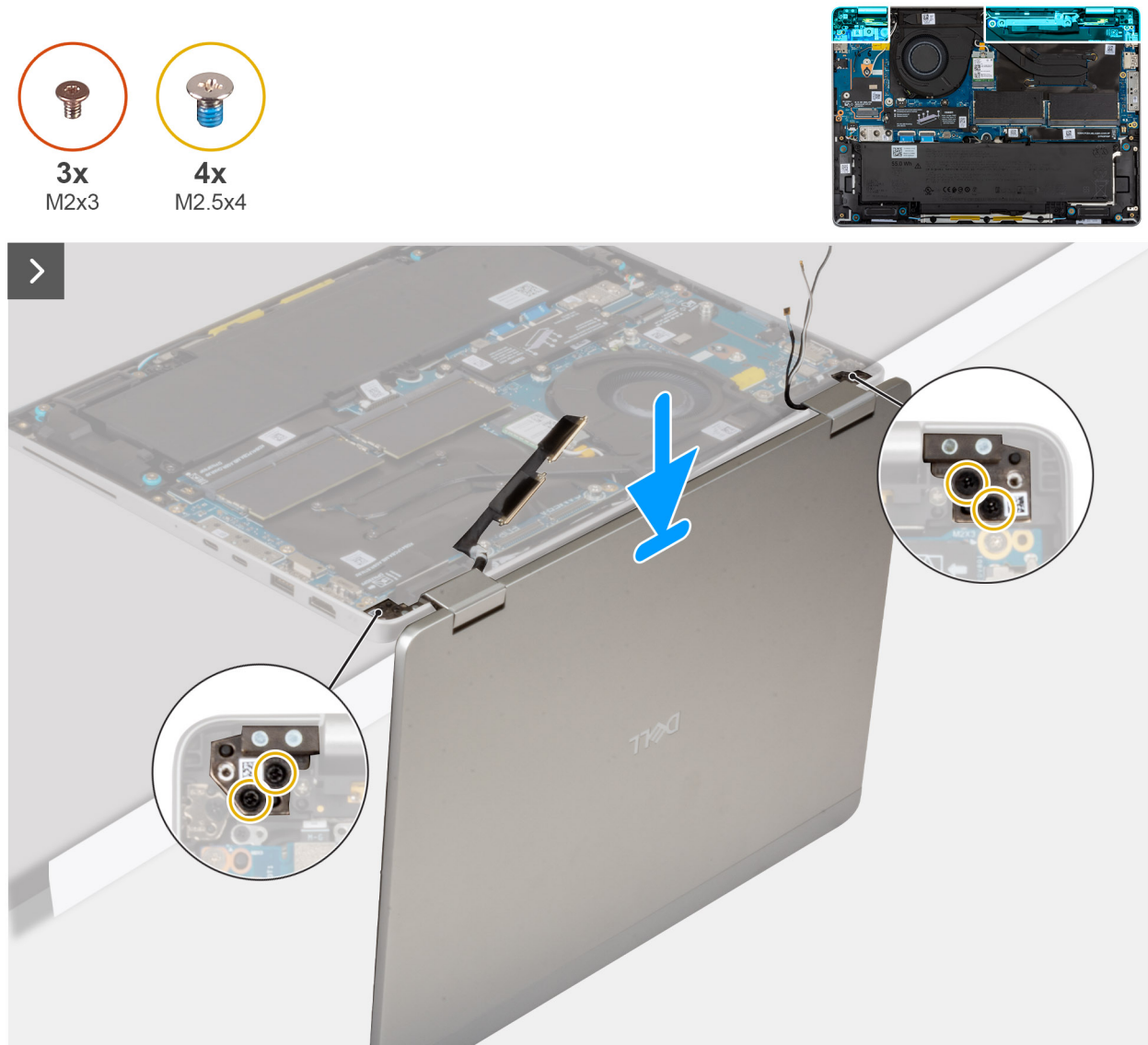
Afbeelding 66. De beeldschermeenheid installeren
