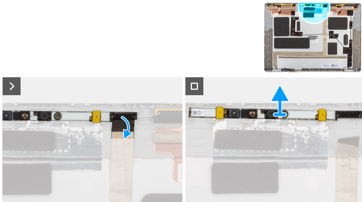
Afbeelding 82. De RGB/IR-camera verwijderen
