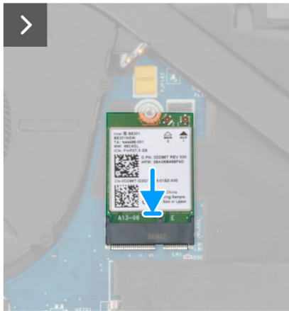
Afbeelding 41. De WLAN-kaart plaatsen
