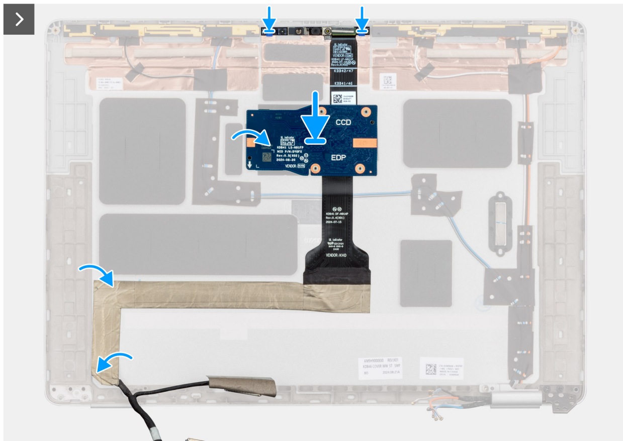
Afbeelding 86. De beeldschermkabel installeren
