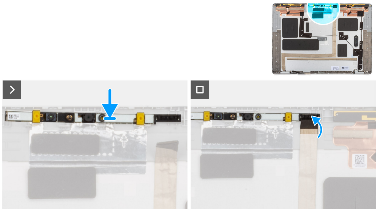
Afbeelding 83. De RGB/IR-camera installeren
