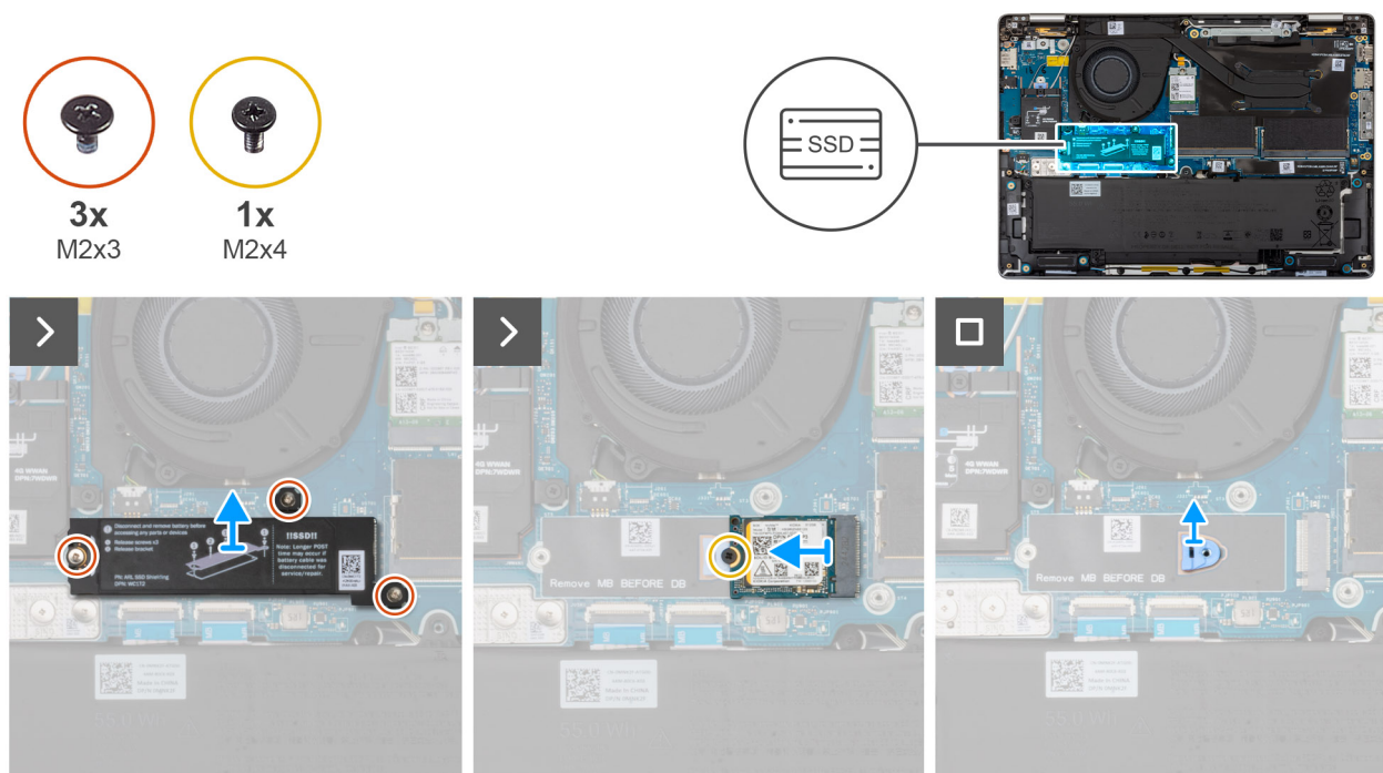
Afbeelding 36. De M.2 2230 SSD verwijderen
