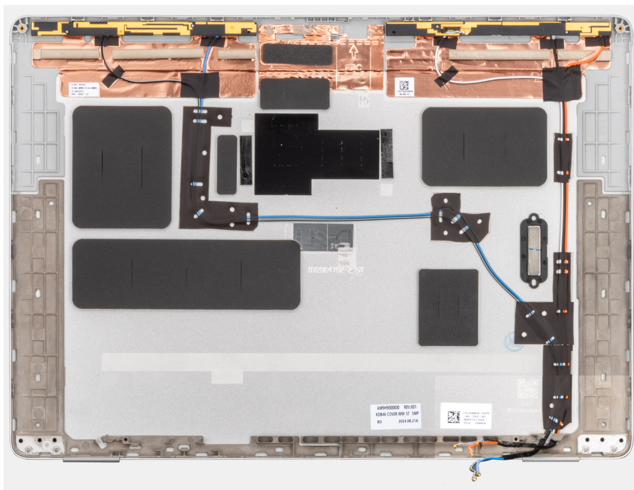
Afbeelding 97. Achterplaat van het beeldscherm en de antenne-eenheid
