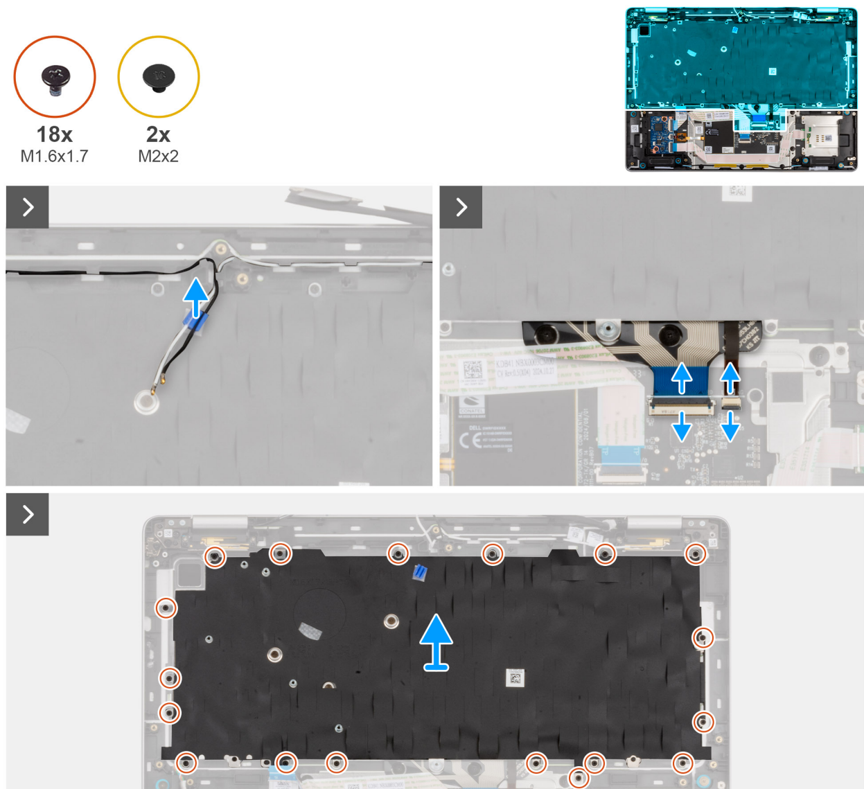
Afbeelding 98. Het toetsenbord verwijderen
