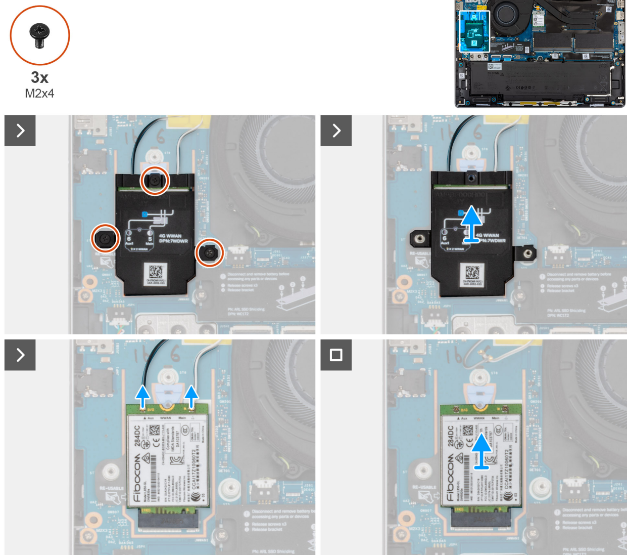
Afbeelding 34. De WWAN-kaart verwijderen
