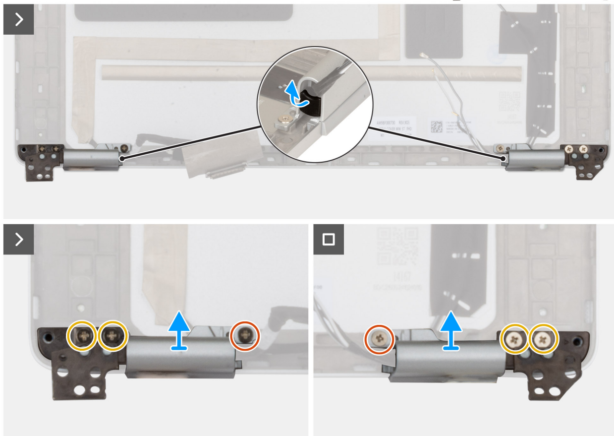
Afbeelding 80. De beeldschermcharnierkappen verwijderen
