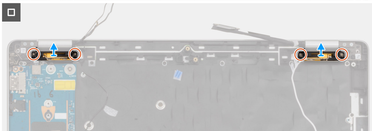
Afbeelding 55. De WLAN-antennemodule verwijderen
