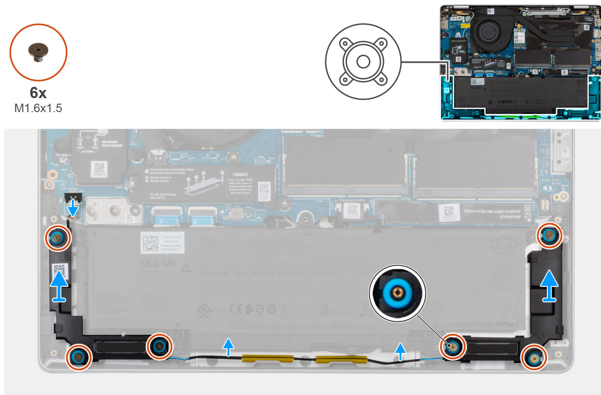
Afbeelding 42. De luidsprekers verwijderen
