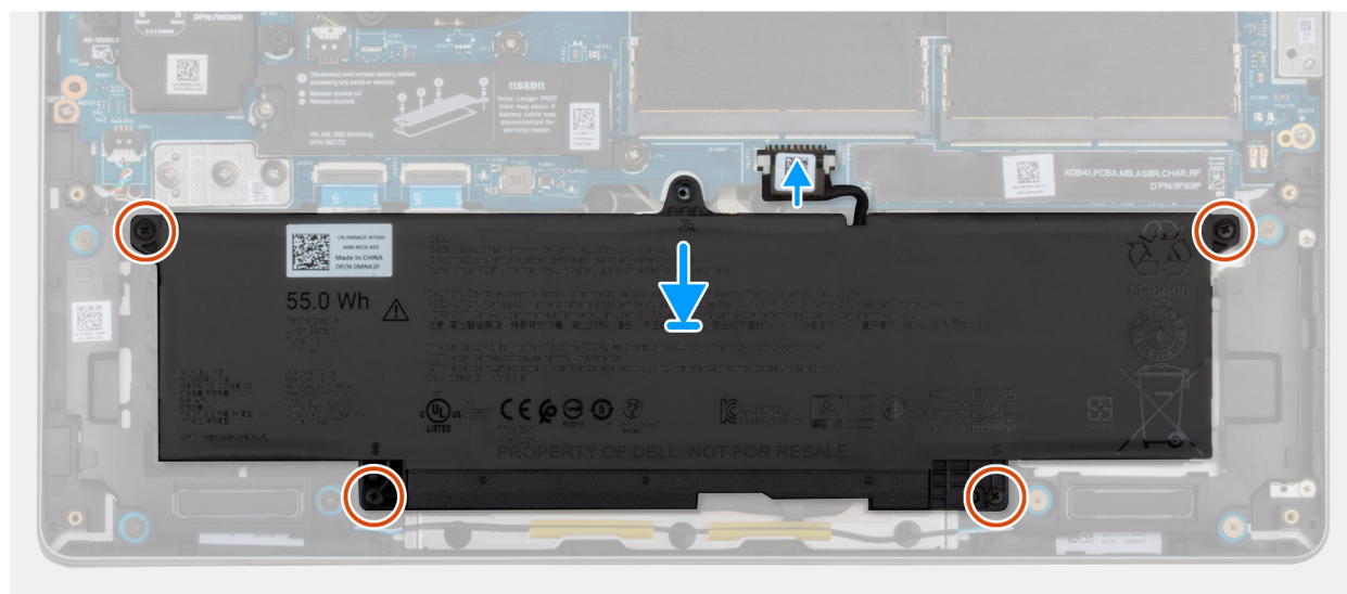
Afbeelding 29. De batterij installeren
