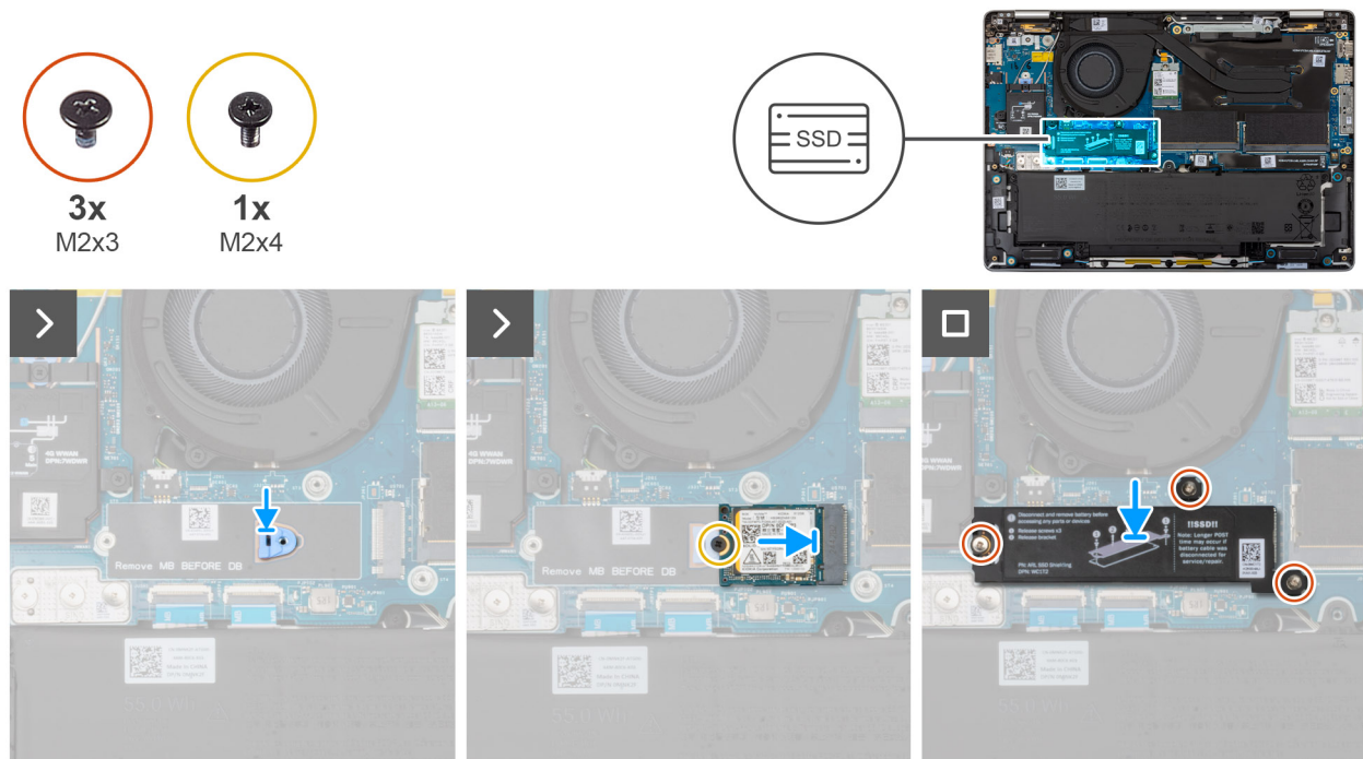
Afbeelding 37. De M.2 2230 SSD installeren
