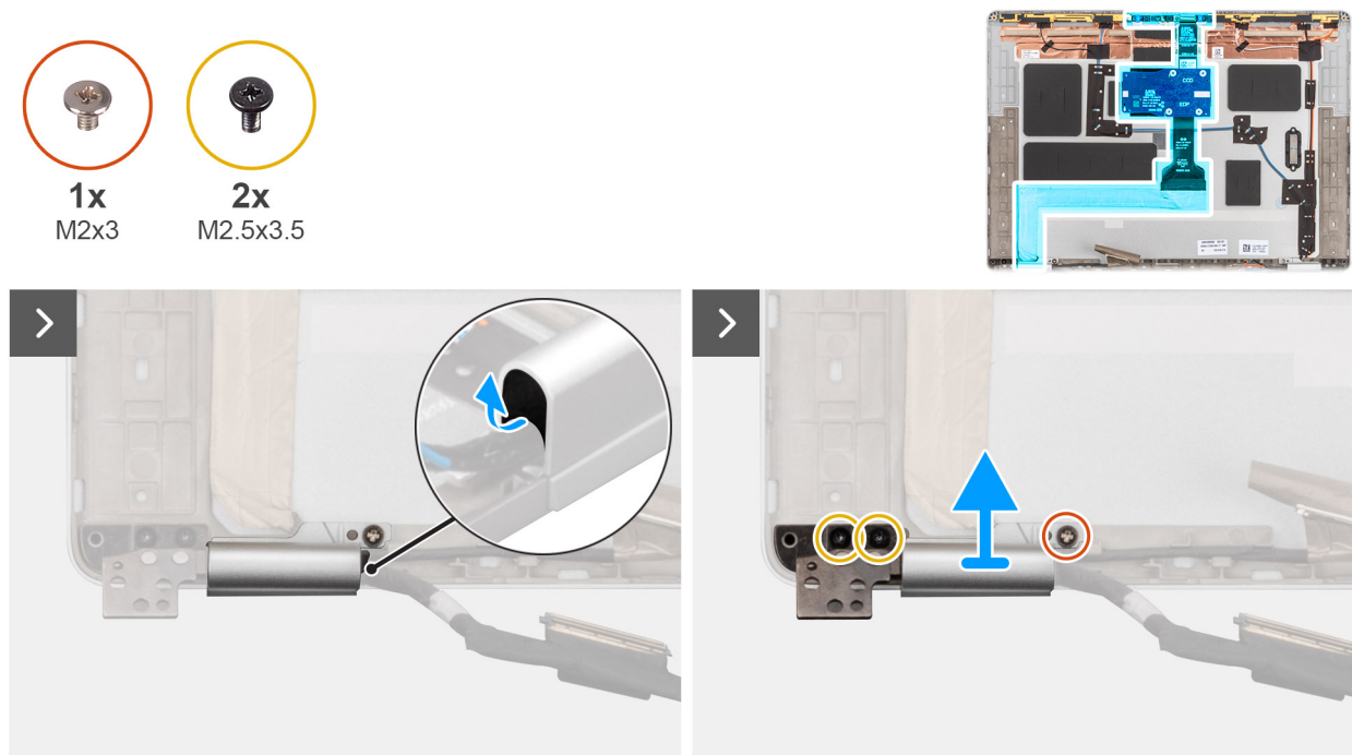
Afbeelding 84. De beeldschermkabel verwijderen
