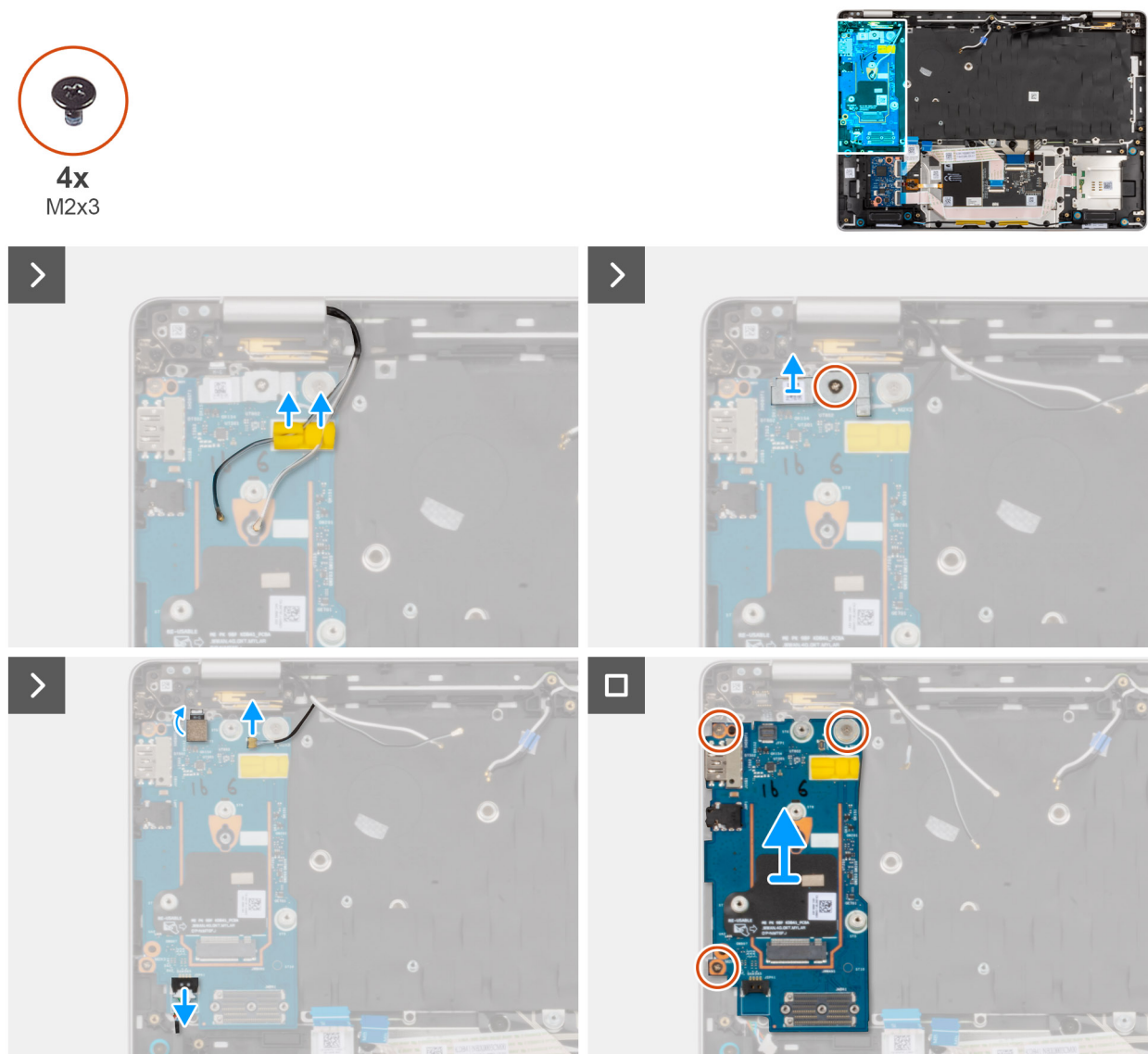
Afbeelding 60. De I/O-kaart verwijderen
