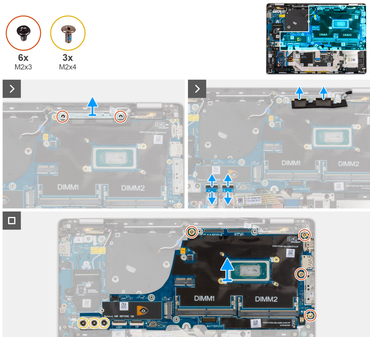
Afbeelding 51. De systeemkaart verwijderen
