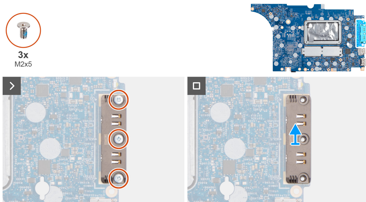
Figur 92. Ta bort USB Type-C-modulen
