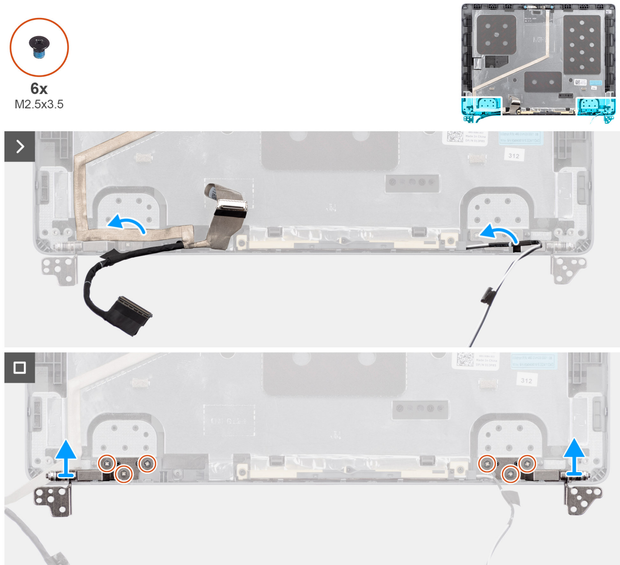
Figur 66. Ta bort bildskärmsgångjärnen
