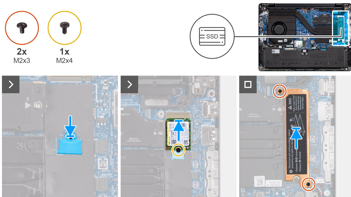
Figur 23. Installera M.2 2230 SSD-disken
