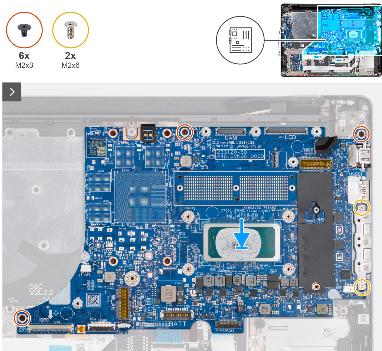
Figur 81. Installera moderkortet
