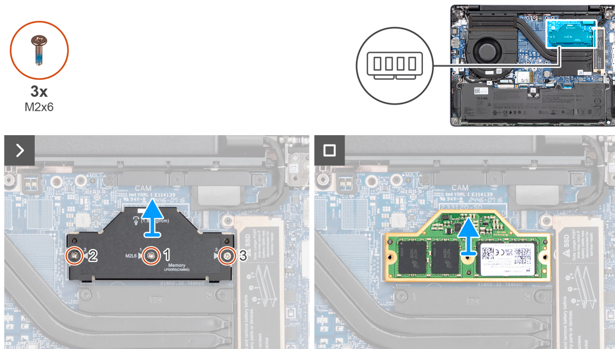
Figur 20. Ta bort minnesmodulen
