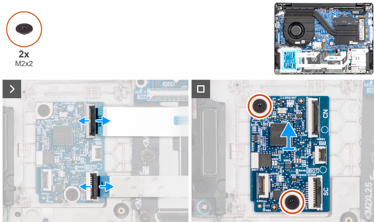
Figur 35. Ta bort USH-kortet
