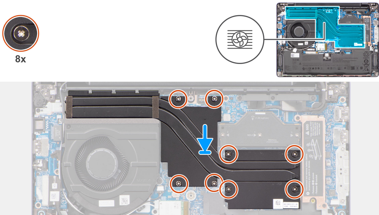
Figur 42. Installera kylflänsen
