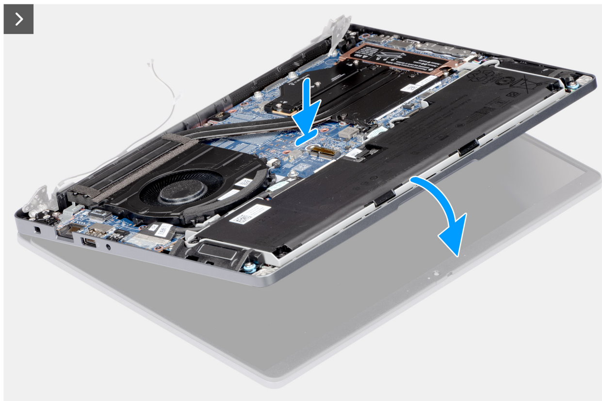
Figur 50. Installera bildskärmsenheten
