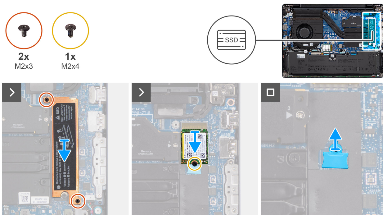
Figur 22. Ta bort M.2 2230 SSD-disken
