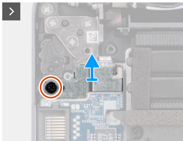
Figur 43. Ta bort I/O-kortet
