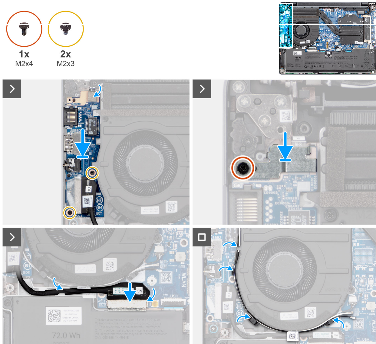
Figur 44. Installera I/O-kortet
