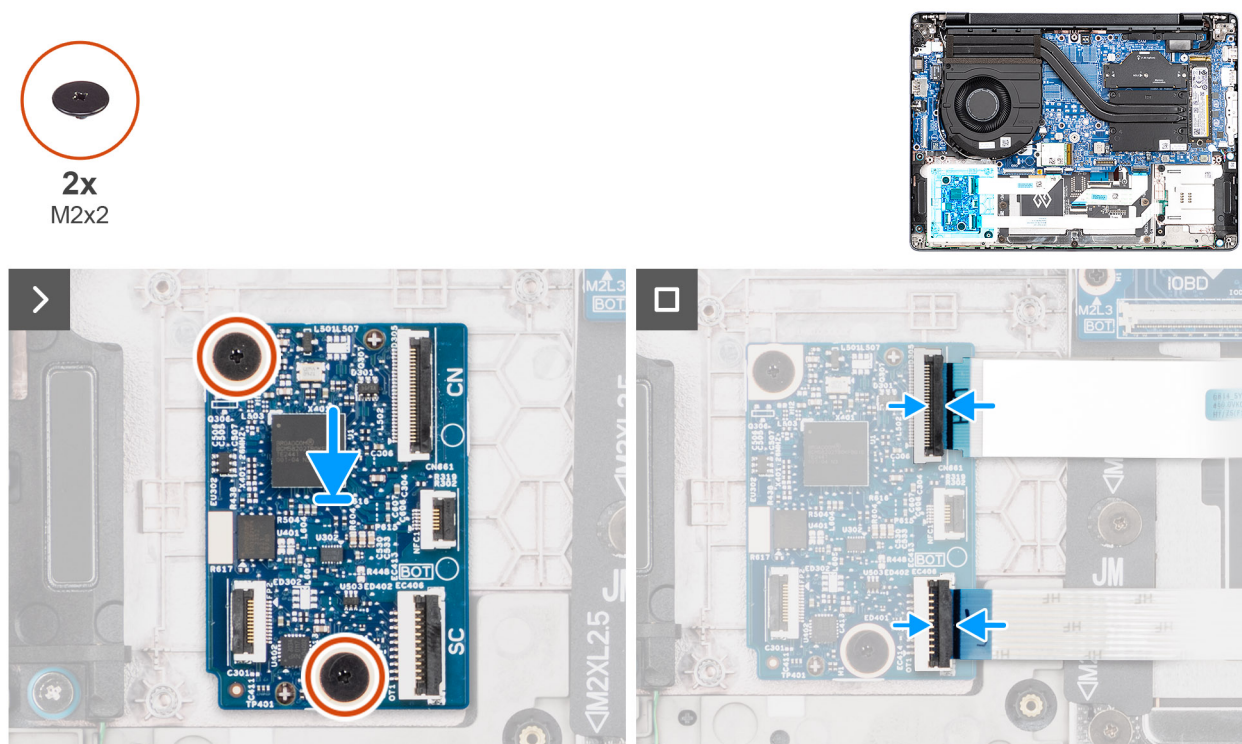
Figur 36. Installera USH-kortet
