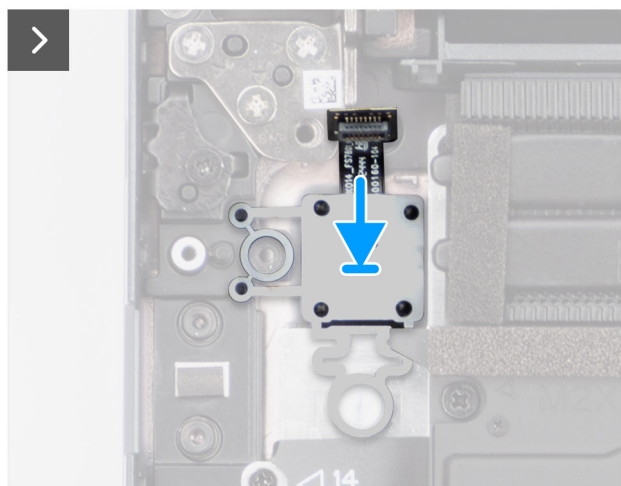
Figur 46. Installera strömbrytaren
