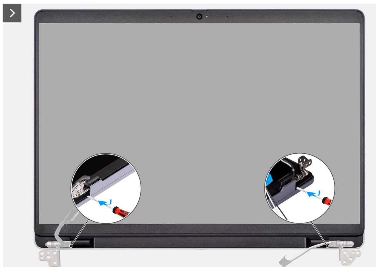
Figur 52. Ta bort bildskärmsramen
