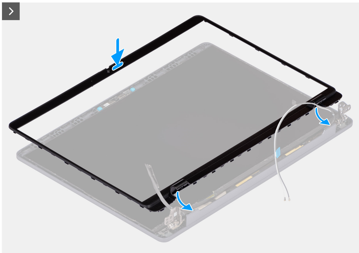
Figur 58. Installera bildskärmsramen
