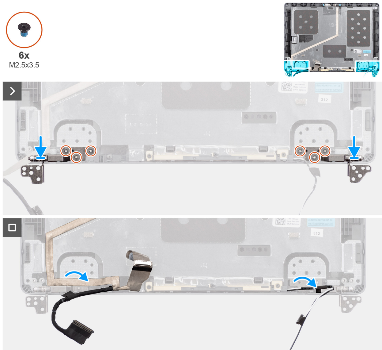
Figur 67. Installera bildskärmsgångjärnen
