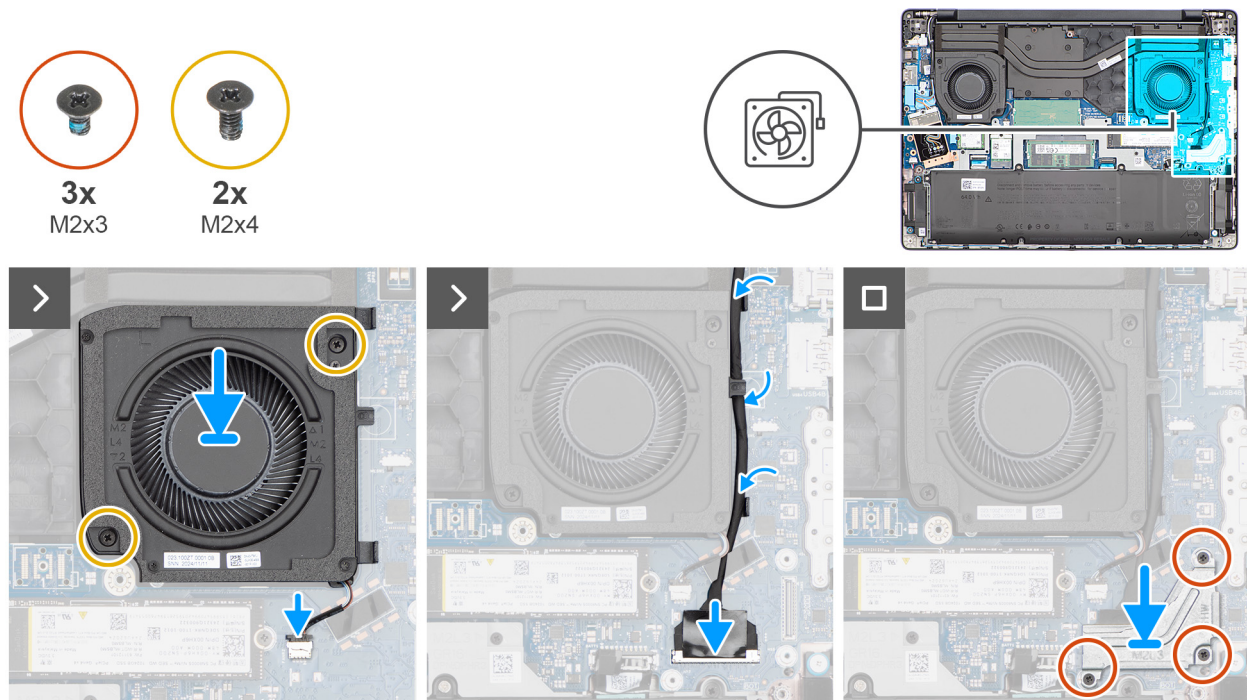
Ilustración 39. Instalación del ventilador izquierdo/de video
