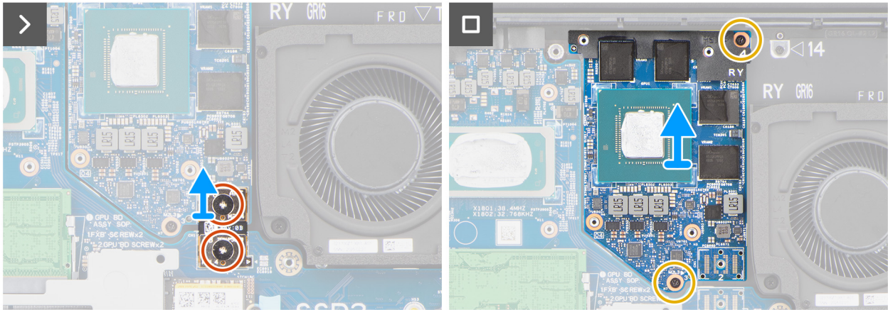
Ilustración 46. Extracción de GPU
