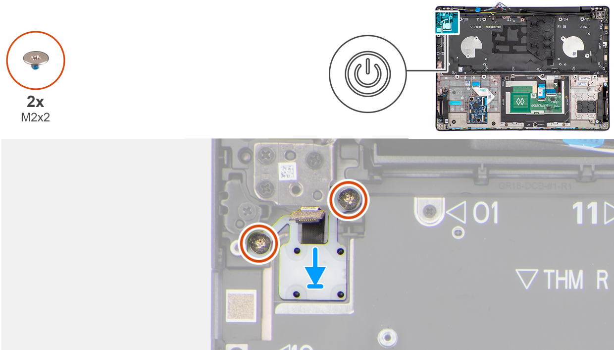
Ilustración 97. Instalación del botón de encendido
