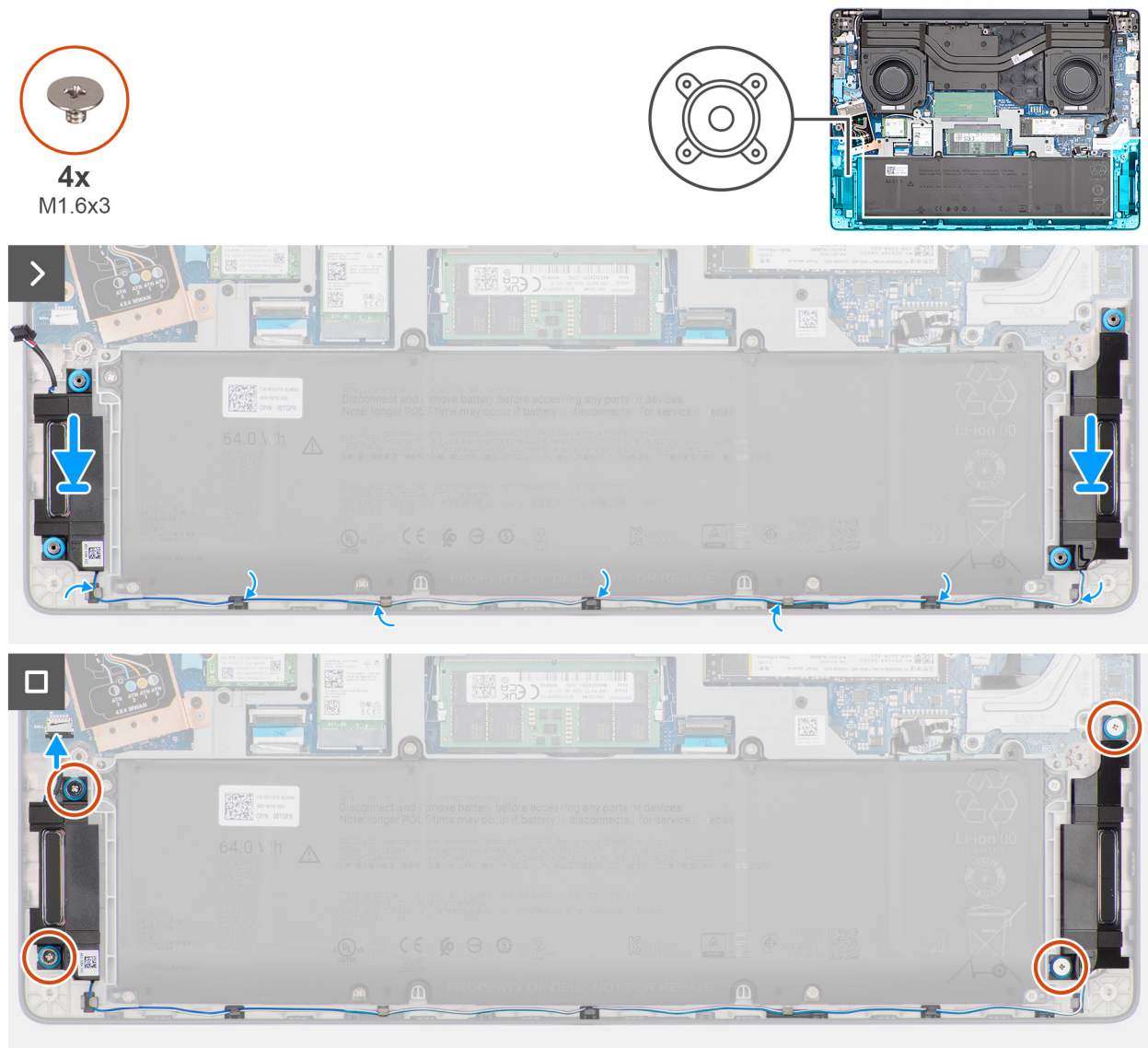
Ilustración 34. Instalación de los parlantes
