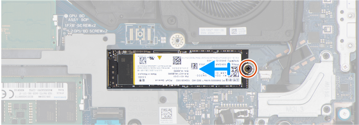
Ilustración 25. Extracción de la unidad de estado sólido M.2 2280
