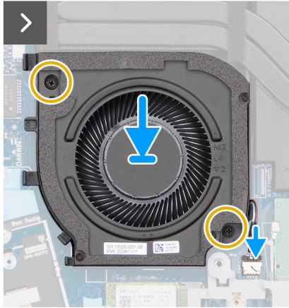
Ilustración 37. Instalación del ventilador derecho/del procesador
