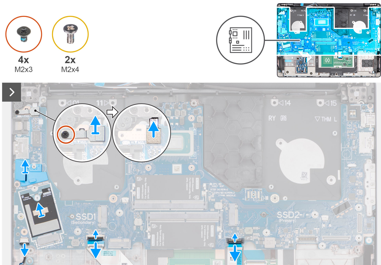
Ilustración 83. Extracción de la tarjeta madre
