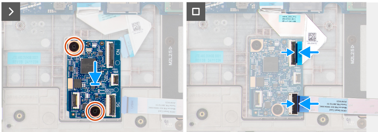
Ilustración 51. Instalación de la placa USH
