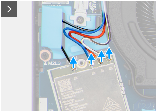
Ilustración 29. Extracción del módulo de WWAN
