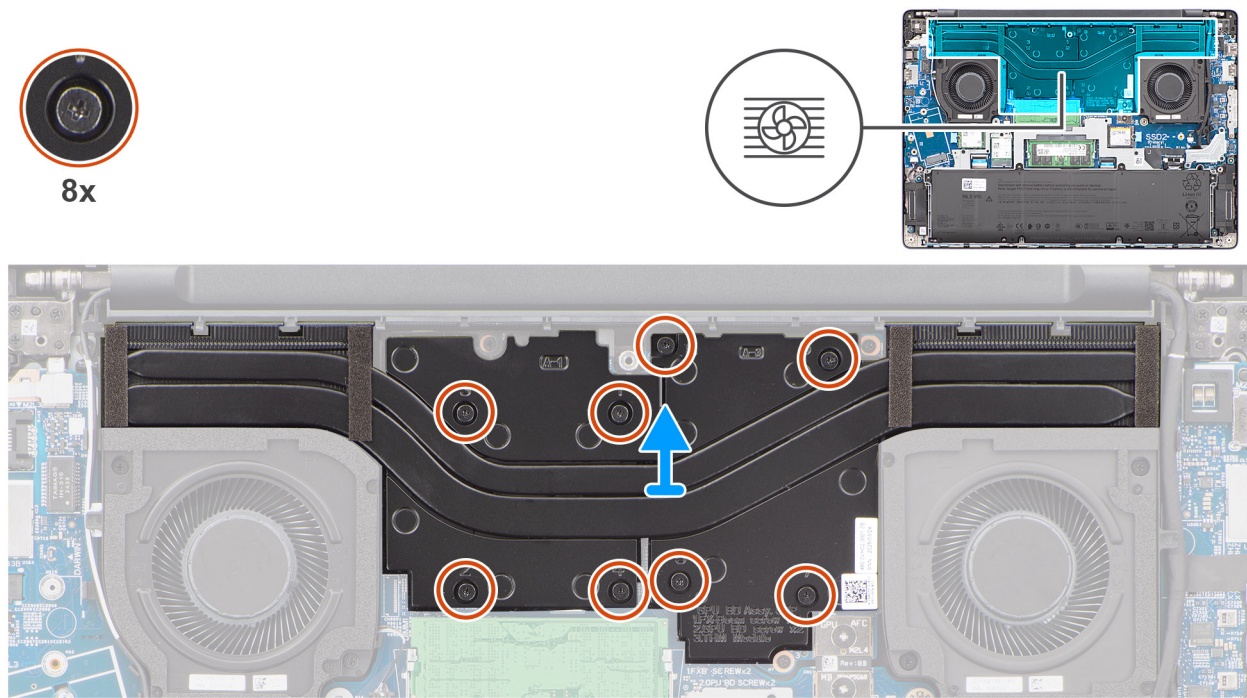
Ilustración 42. Extracción del disipador de calor
