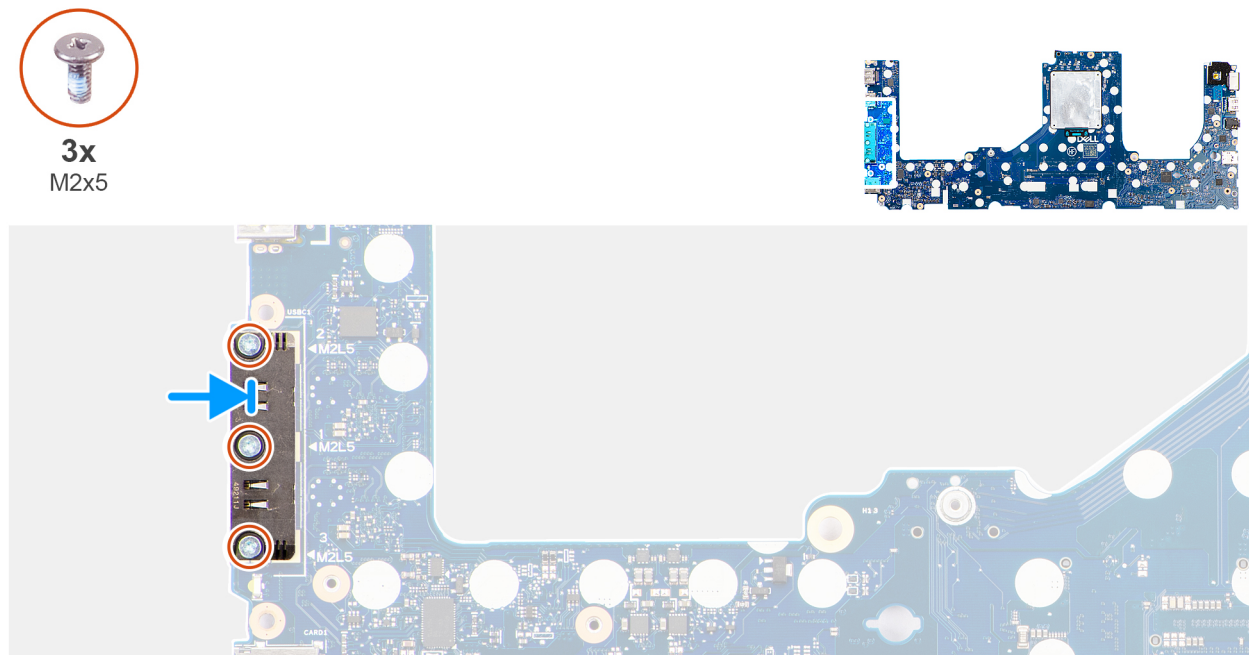
Ilustración 95. Instalación del módulo USB Type-C
