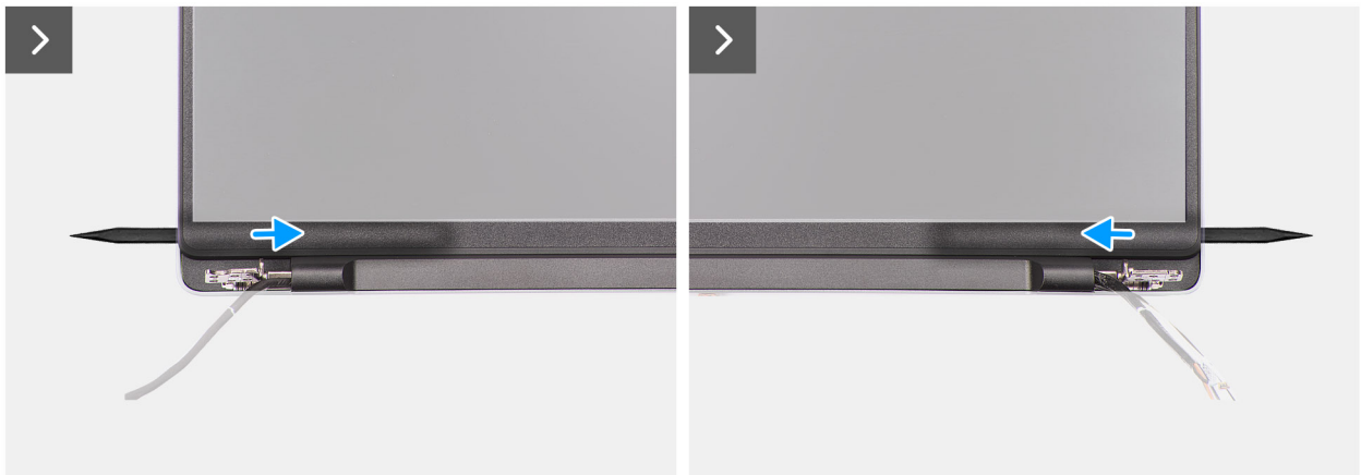
Ilustración 64. Extracción del embellecedor de la pantalla
