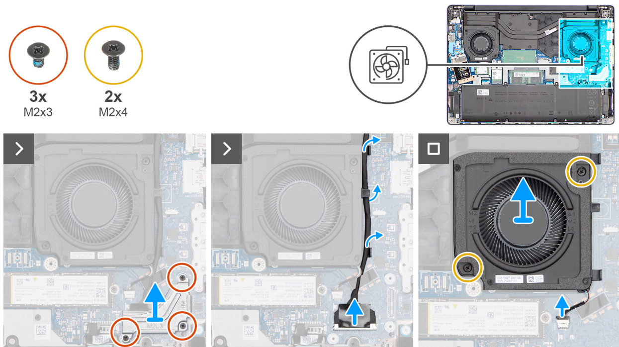
Ilustración 38. Extracción del ventilador izquierdo/de video
