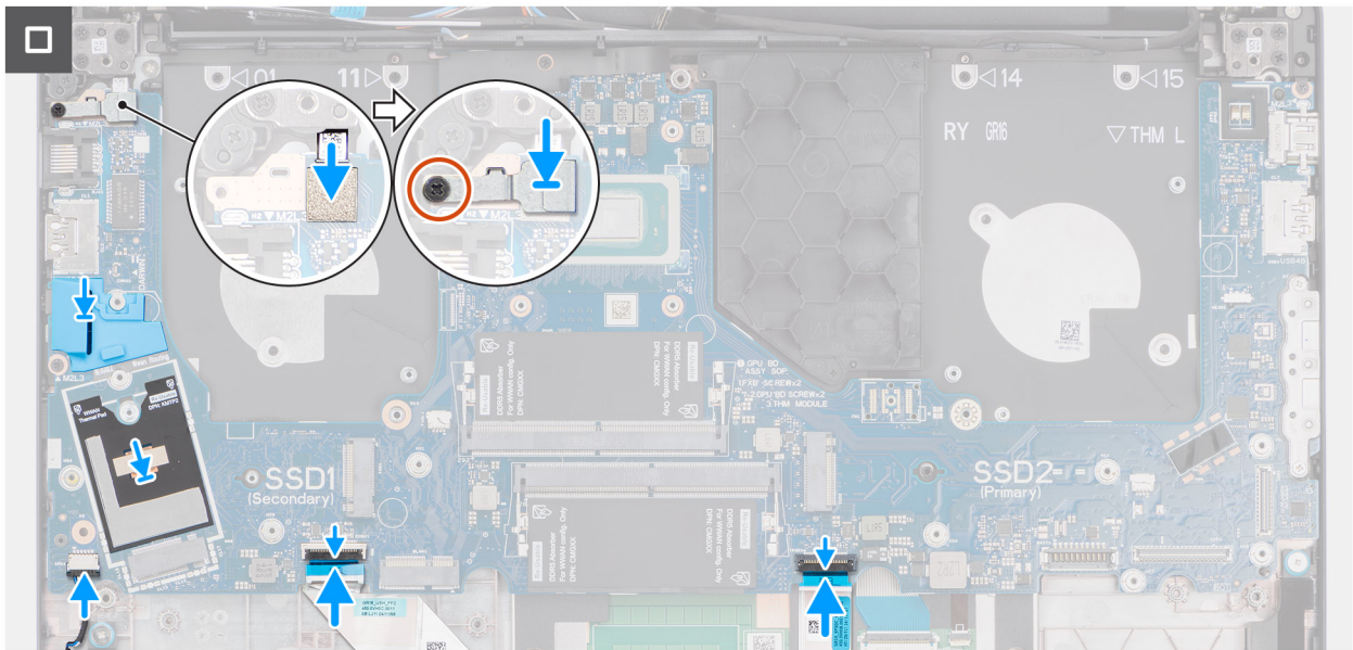
Ilustración 87. Instalación de la tarjeta madre
