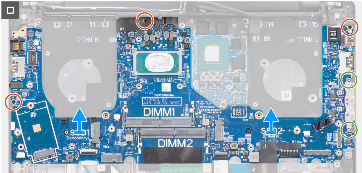
Ilustración 90. Extracción de la tarjeta madre
