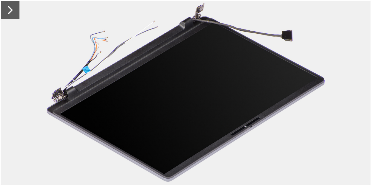
Ilustración 57. Instalación del ensamblaje de la pantalla
