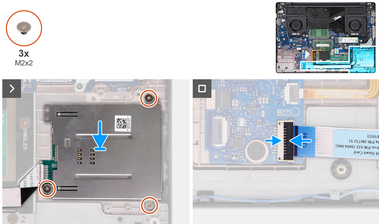
Ilustración 53. Instalación del lector de tarjetas inteligentes
