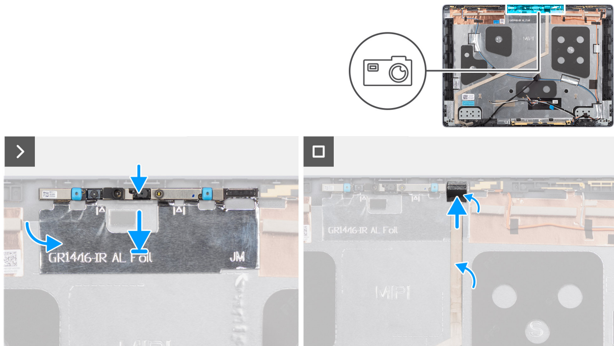
Ilustración 79. Instalación de la cámara
