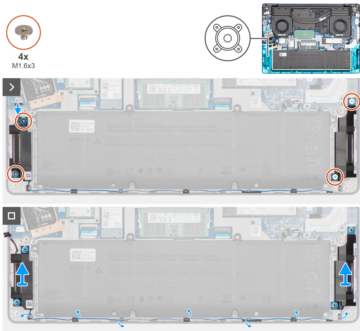
Ilustración 33. Extracción de los parlantes
