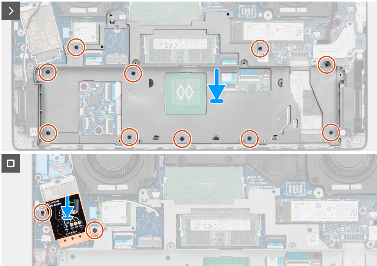
Ilustración 49. Instalación del compartimento de la batería
