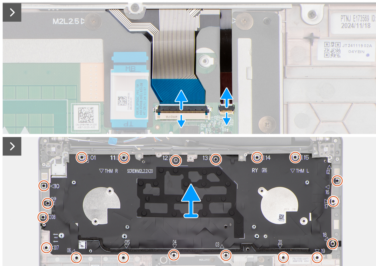
Ilustración 98. Extracción del teclado
