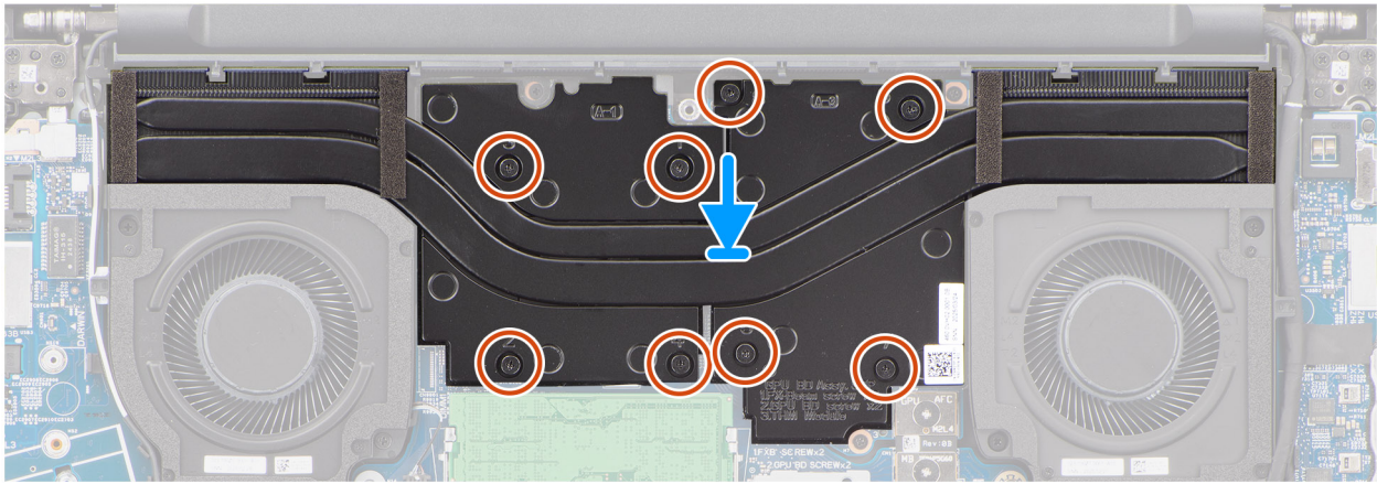
Ilustración 43. Instalación del disipador de calor
