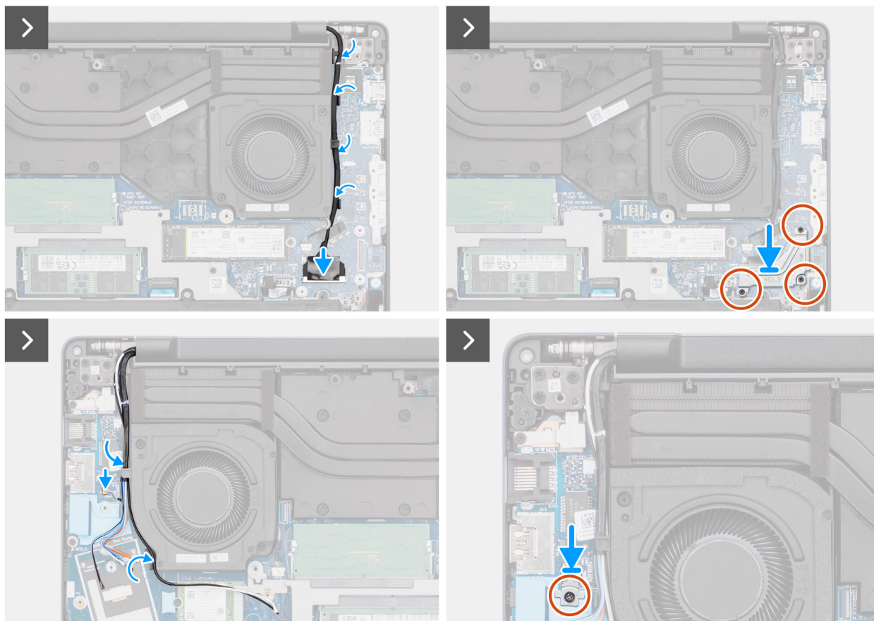
Ilustración 59. Instalación del ensamblaje de la pantalla
