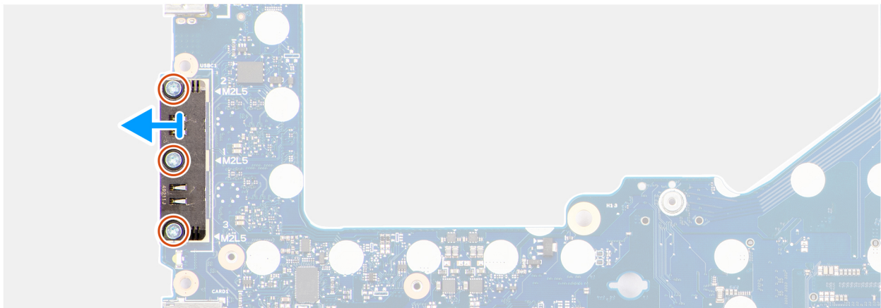
Ilustración 94. Extracción del módulo USB Type-C
