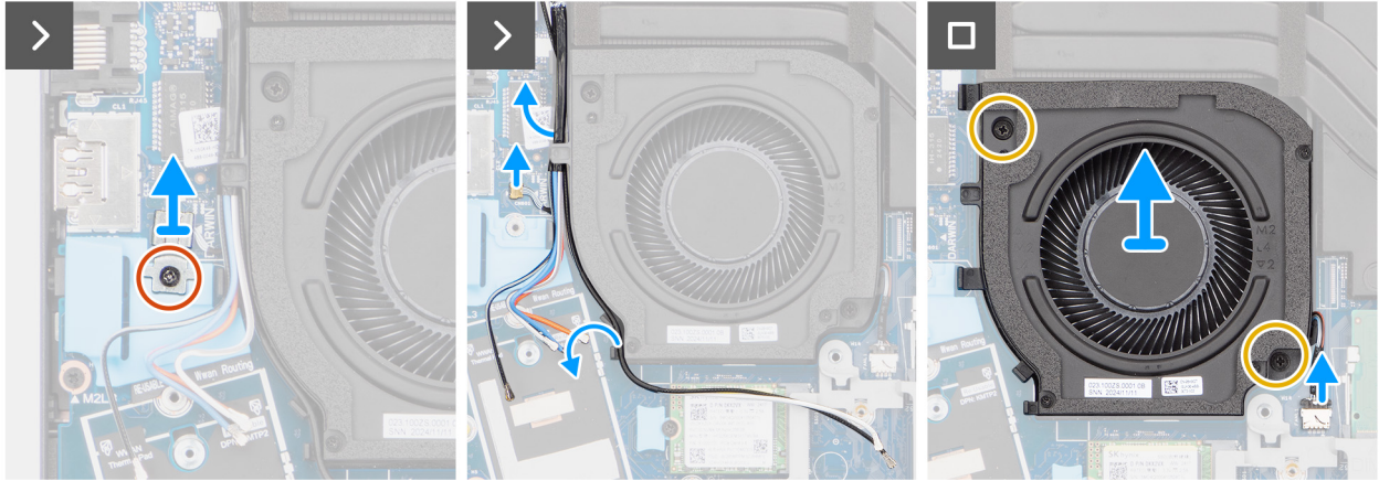
Ilustración 36. Extracción del ventilador derecho/del procesador
