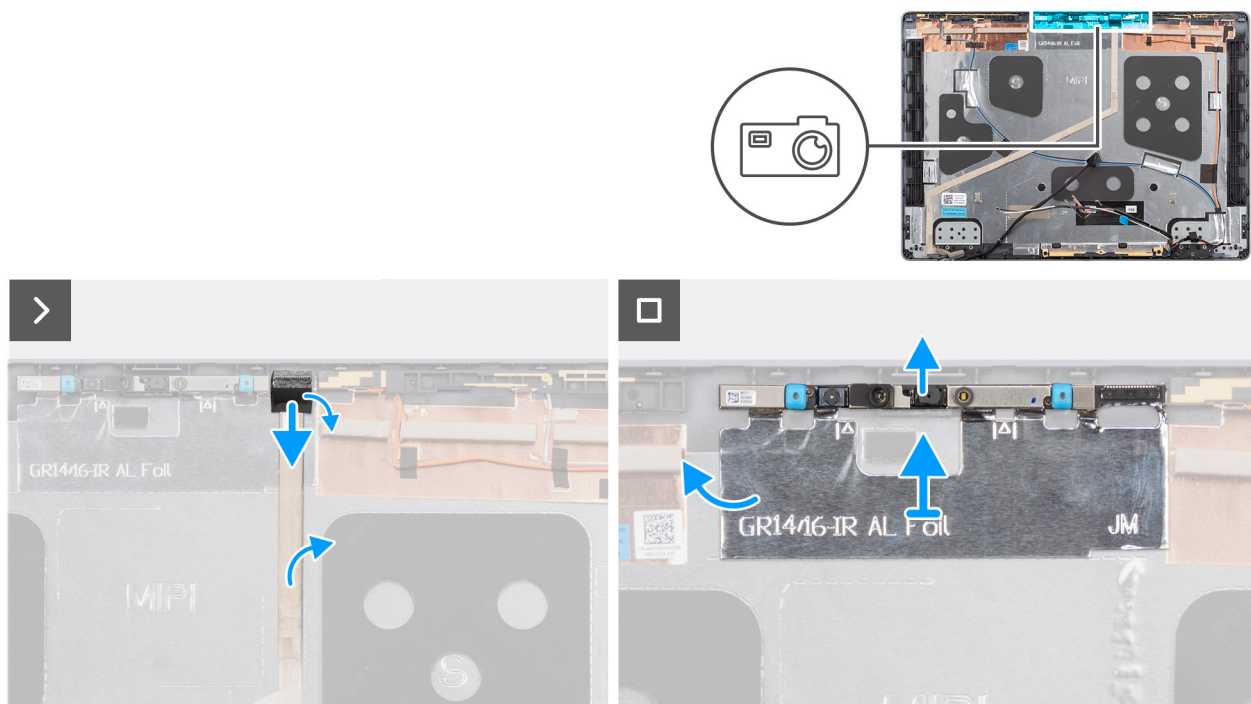
Ilustración 78. Extracción de la cámara
