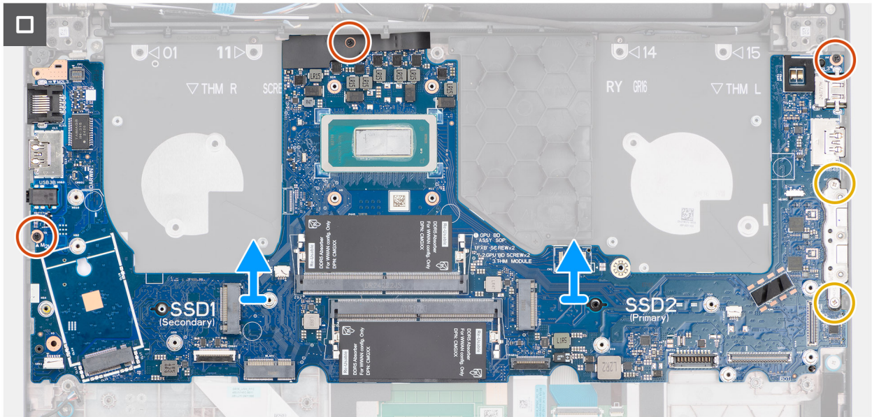
Ilustración 84. Extracción de la tarjeta madre
