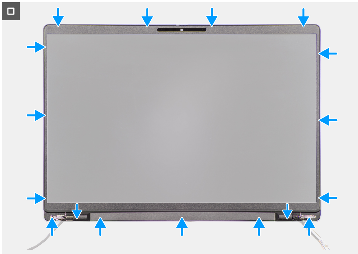
Ilustración 67. Instalación del bisel de la pantalla
