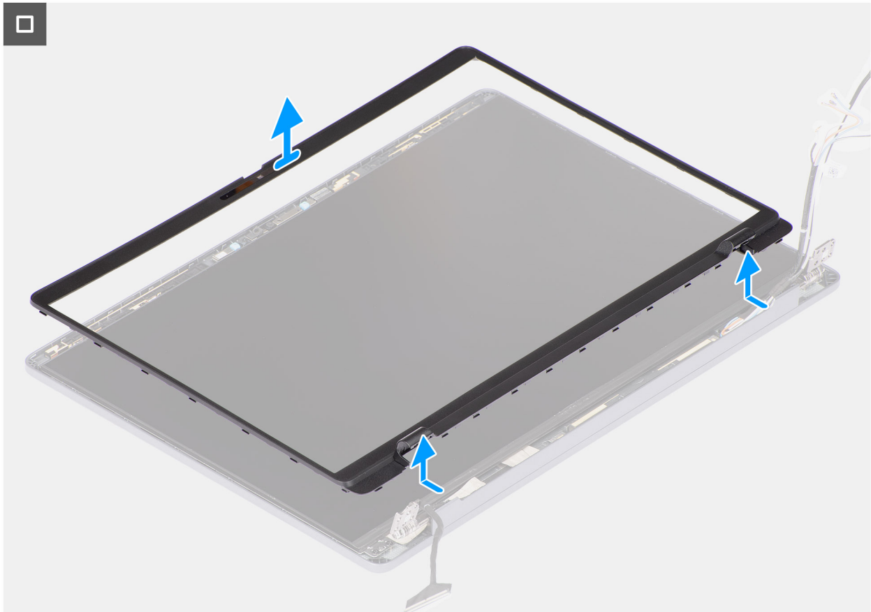
Ilustración 65. Extracción del embellecedor de la pantalla
