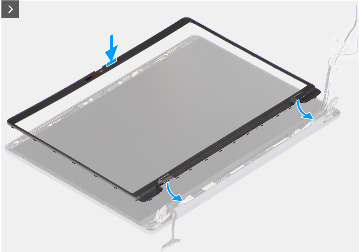
Ilustración 66. Instalación del bisel de la pantalla
