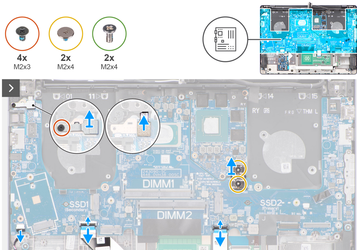
Ilustración 89. Extracción de la tarjeta madre
