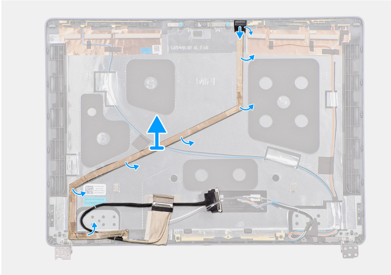
Ilustración 76. Extracción del cable de pantalla
