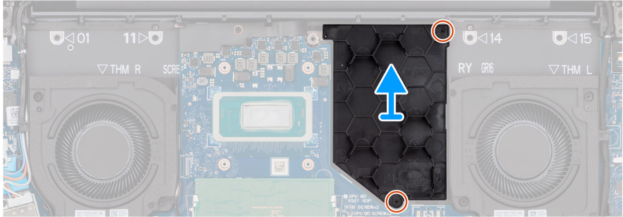
Ilustración 44. Extracción de la pieza de relleno de GPU
