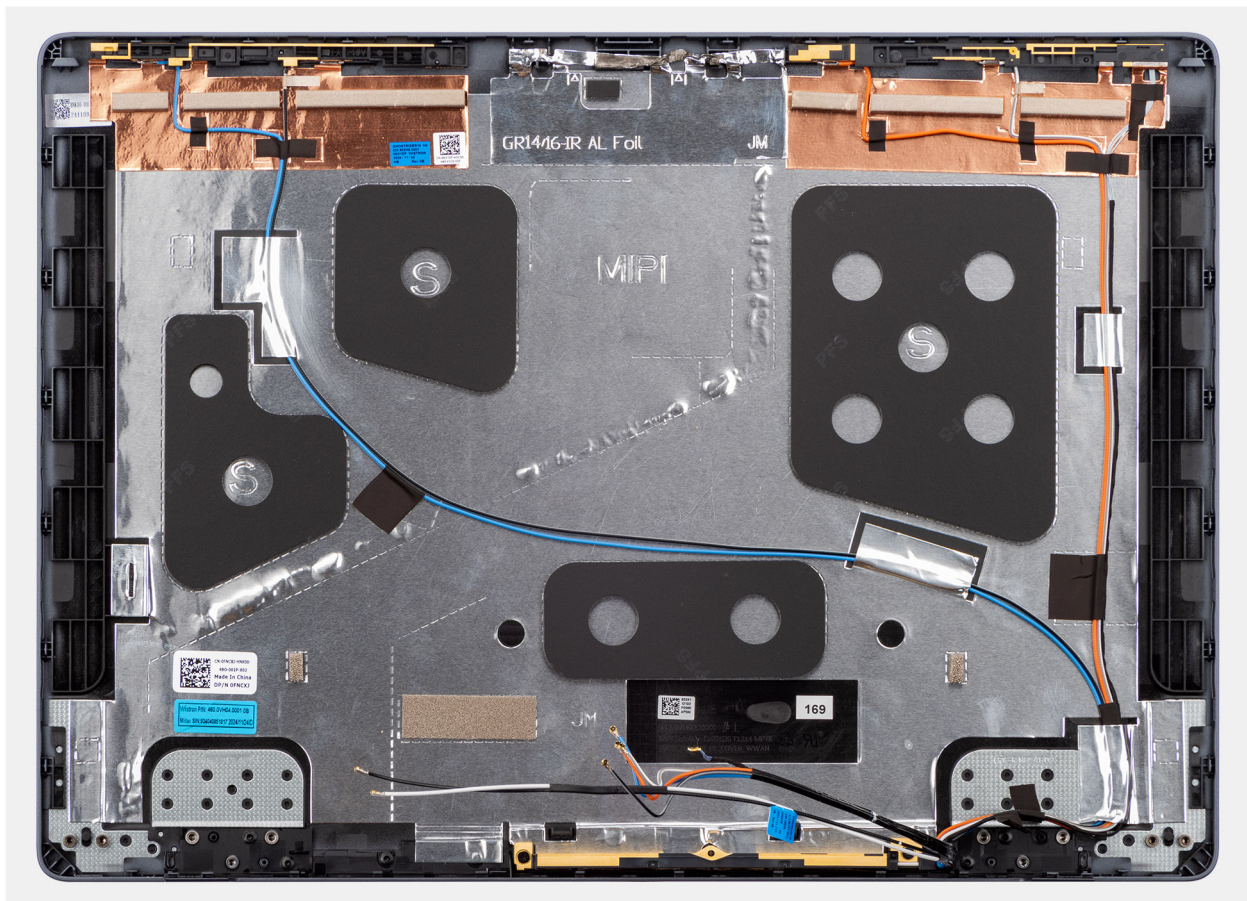
Ilustración 80. Ensamblaje de la antena y la cubierta posterior de la pantalla
