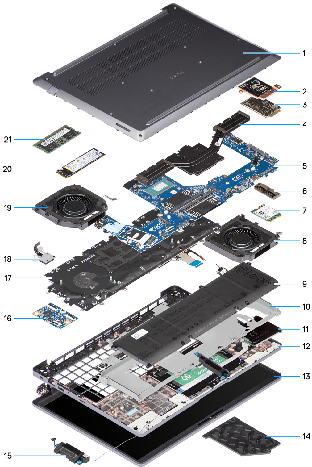
Ilustración 11. Componentes principales de la Dell Pro Max 16 MC16250
