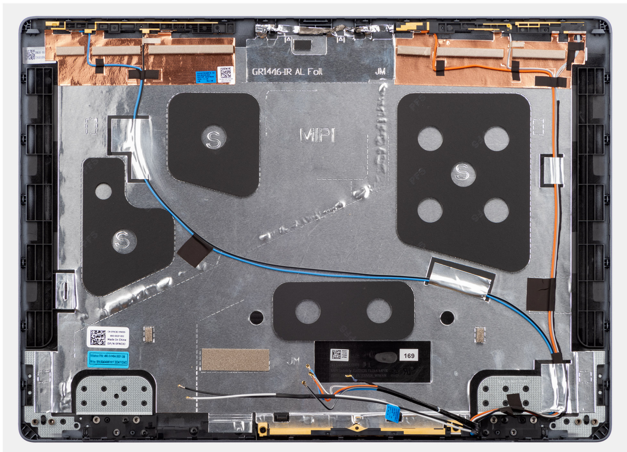
Ilustración 81. Ensamblaje de la antena y la cubierta posterior de la pantalla
