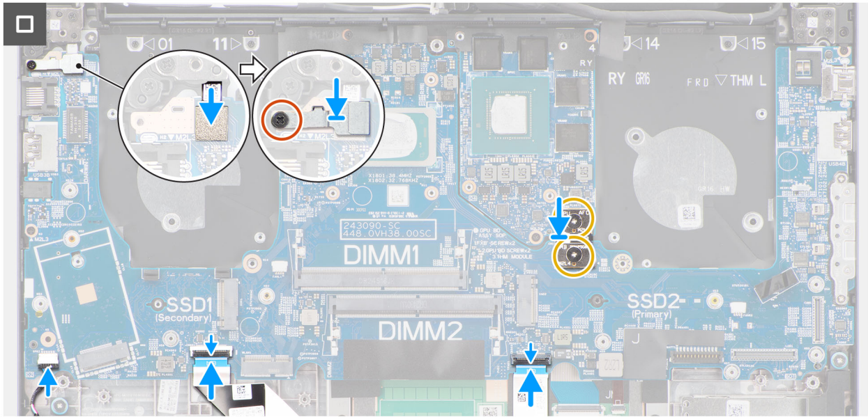
Ilustración 93. Instalación de la tarjeta madre
