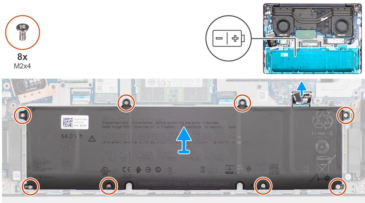
Ilustración 17. Extracción de la batería
