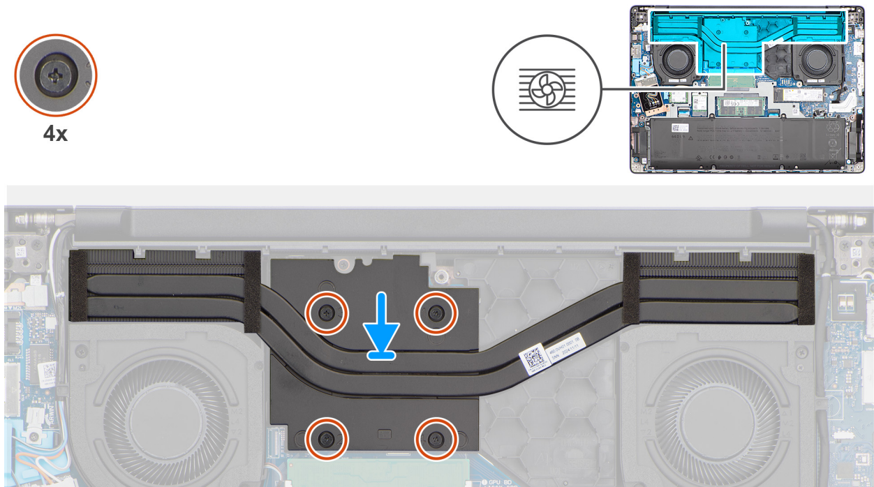
Ilustración 41. Instalación del disipador de calor
