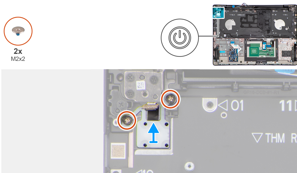
Ilustración 96. Extracción del botón de encendido
