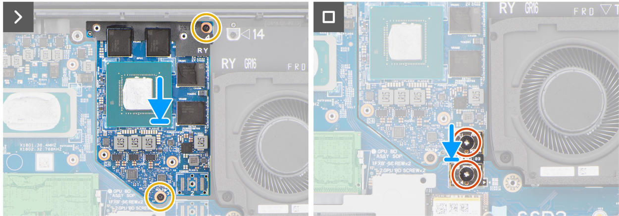
Ilustración 47. Instalación de GPU
