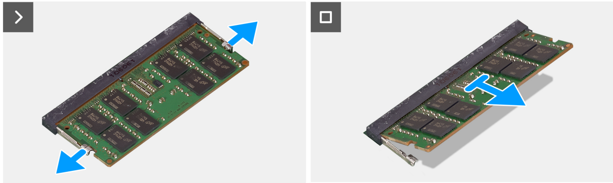
Ilustración 21. Extracción del módulo de memoria
