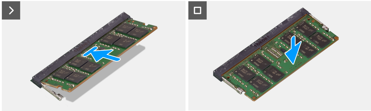
Ilustración 22. Instalación del módulo de memoria
