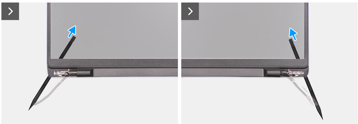
Ilustración 61. Extracción del embellecedor de la pantalla
