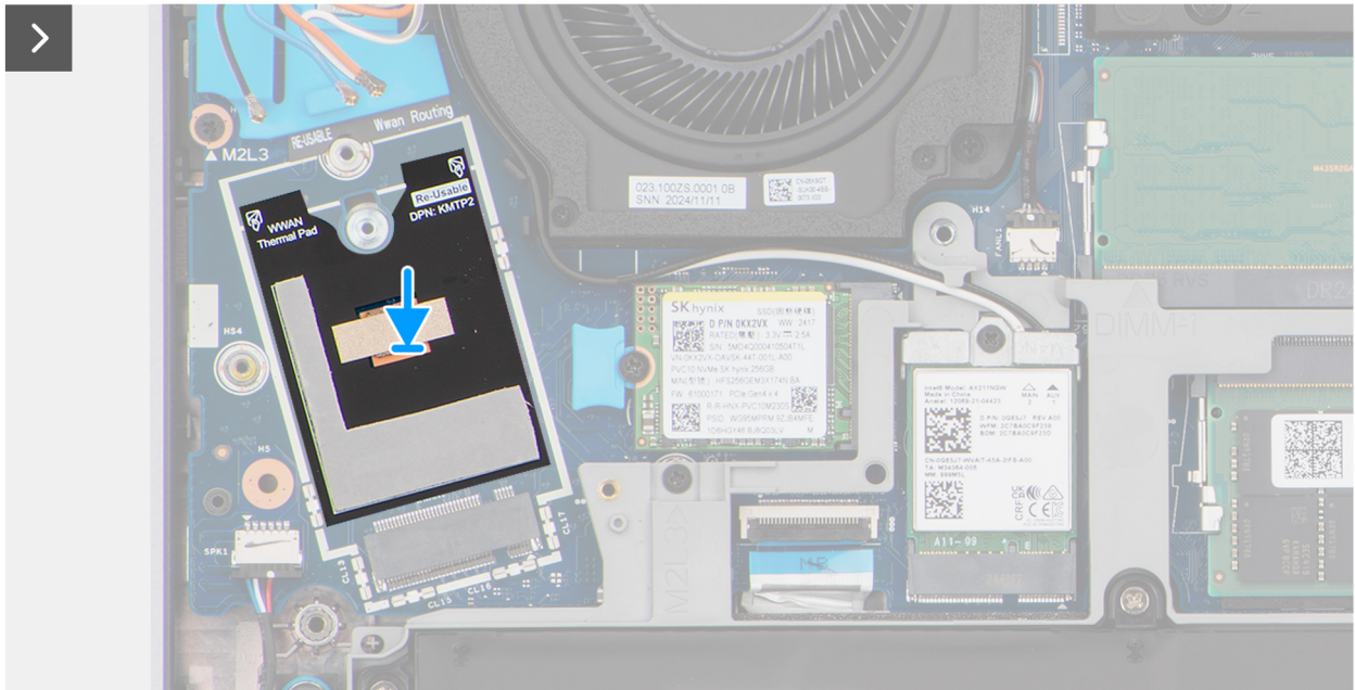
Ilustración 31. Instalación del módulo de WWAN
