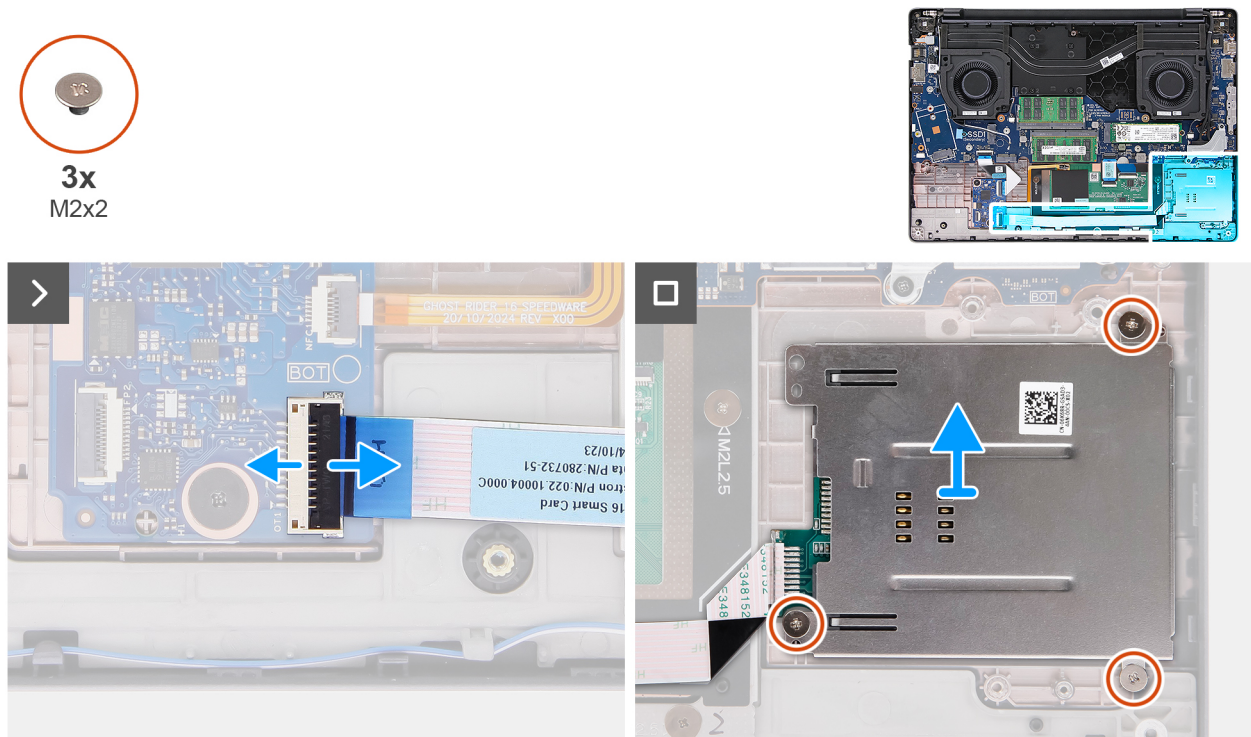
Ilustración 52. Extracción del lector de tarjetas inteligentes
