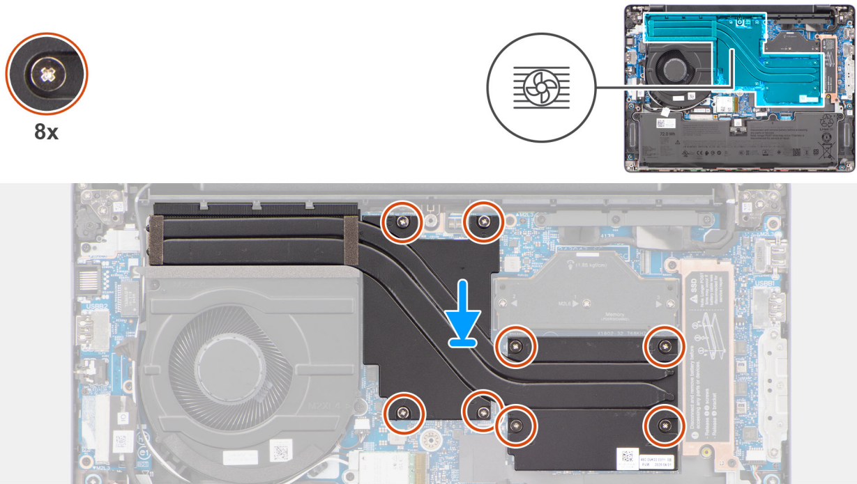
Ilustración 42. Instalación del disipador de calor
