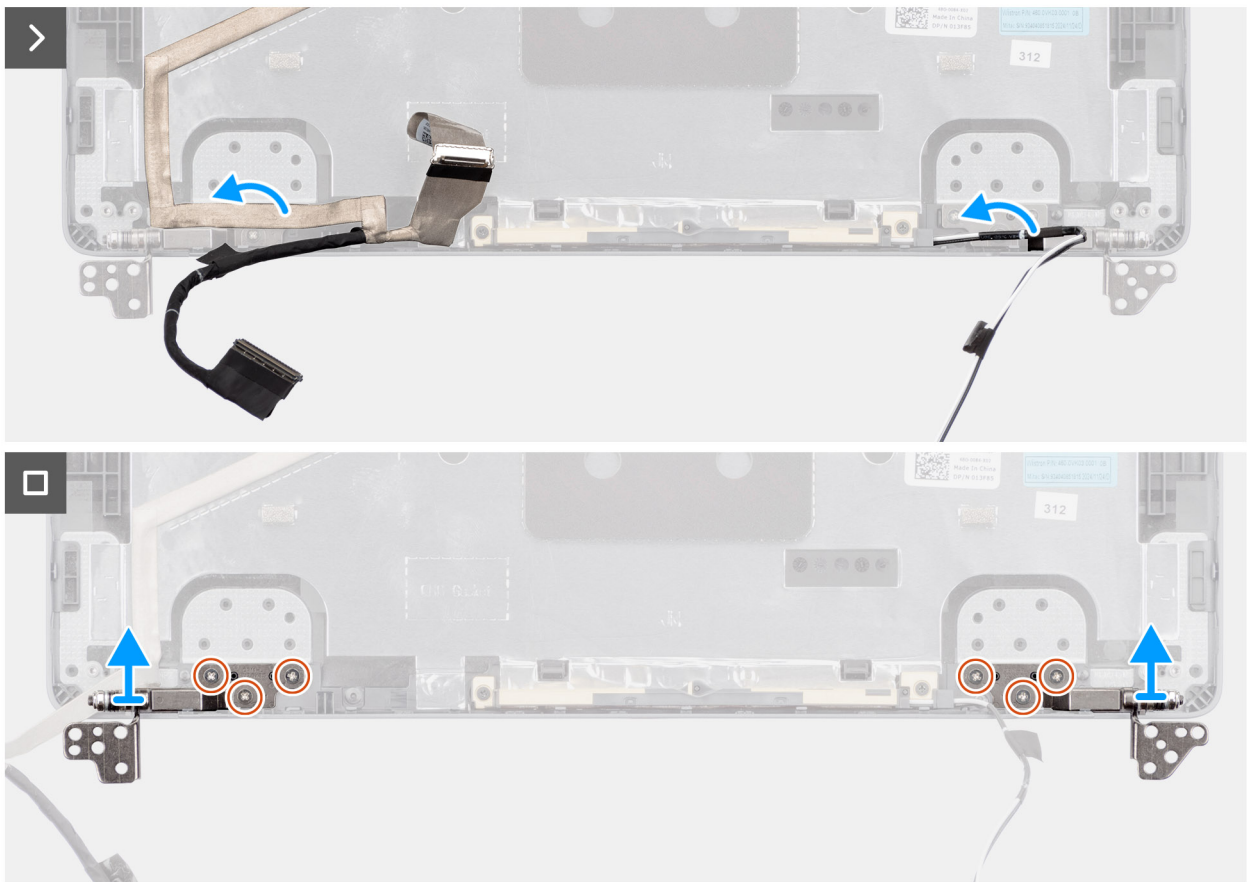
Ilustración 66. Removing the display hinges
