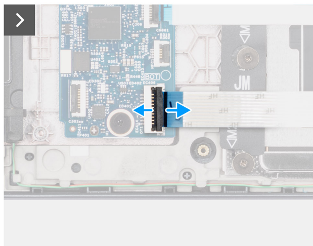
Ilustración 37. Extracción del lector de tarjetas inteligentes
