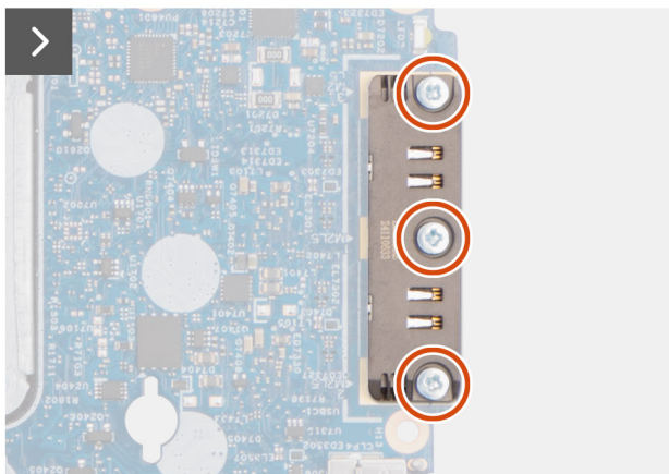
Ilustración 92. Removing the USB Type-C module
