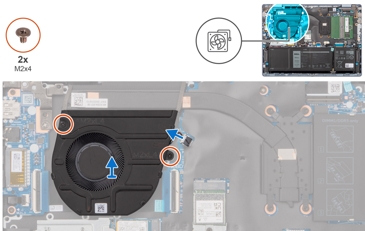
Figure 27. Removing the fan
