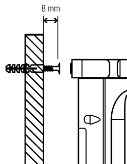
Fig. 3. Detalle montaje en pared.
