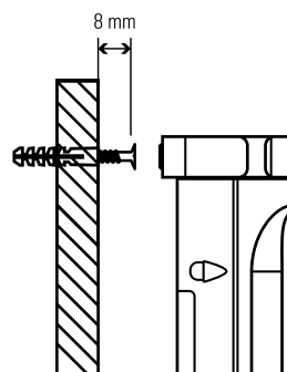
Fig. 3. Montage mural.
