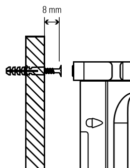
Fig. 3. Detail der Wandmontage.
