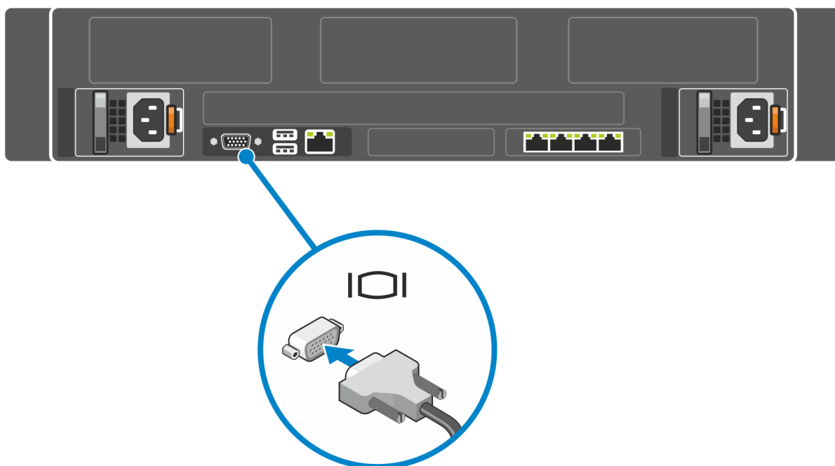
Abbildung 3. Bildschirmanschluss
