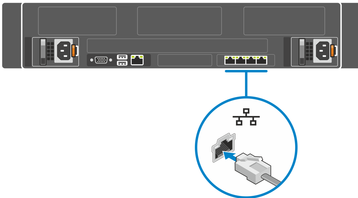
Abbildung 2. Netzwerkport
