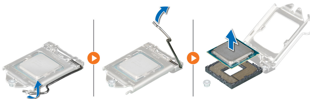
Figure 45. Retrait du processeur
