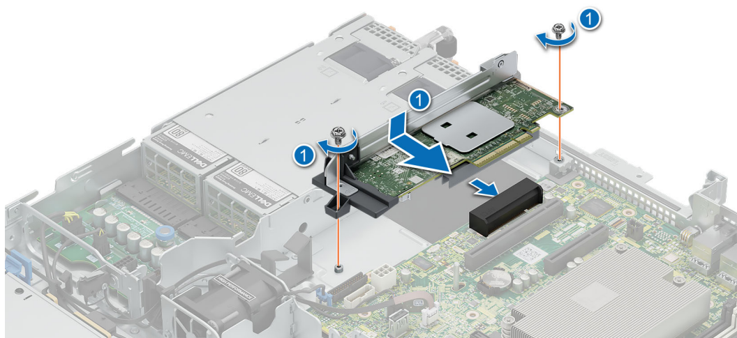
Figure 66. Installation de la carte PERC interne
