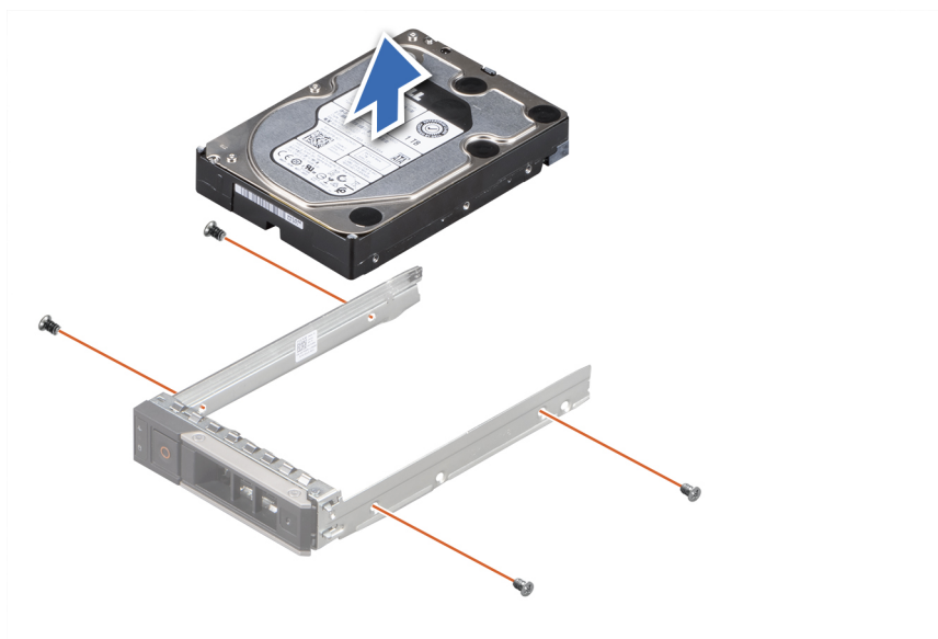
Figure 36. Retrait d'un disque dur installé de son support
