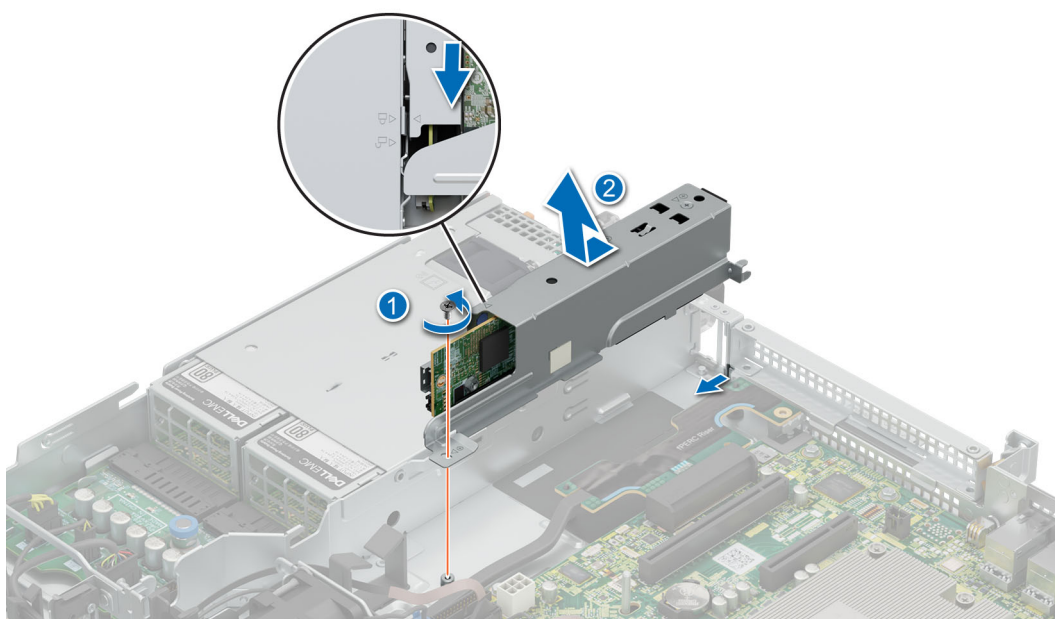
Figure 56. Retrait du bâti du module BOSS N1
