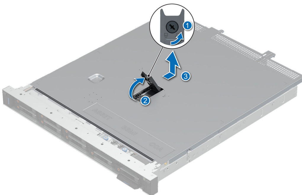
Figure 16. Retrait du capot du système
