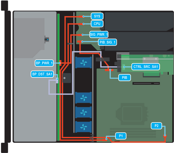
Figure 30. Configuration 2 : 4 disques SAS/SATA de 3,5 pouces et carte PERC interne
