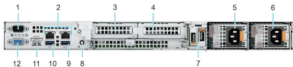
Figure 3. Vue arrière du système
