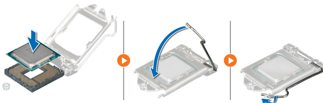
Figure 46. Installation du clip de fixation
