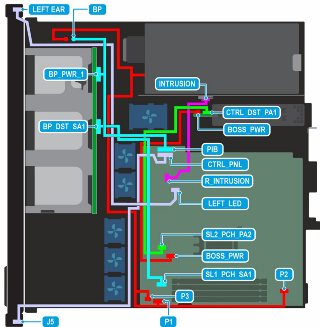
Ilustración 45. Configuración 6: cuatro unidades SATA de 2,5 pulgadas con PSU cableada y BOSS-N1 (opcional)
