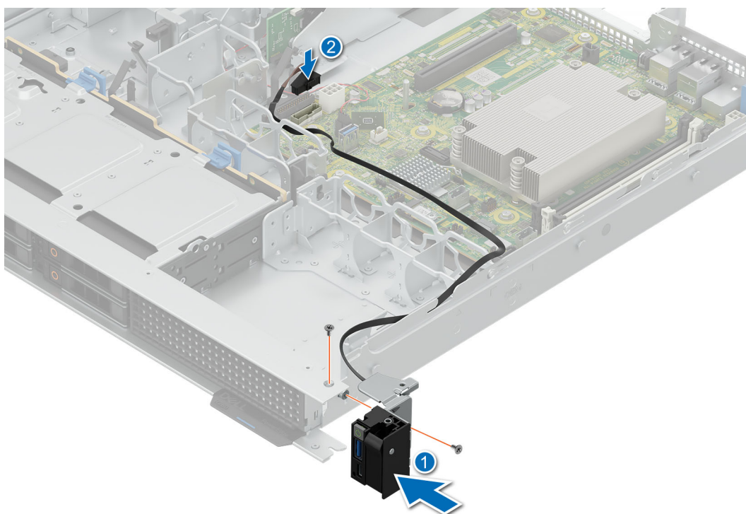
Ilustración 95. Instalación del panel de control derecho
