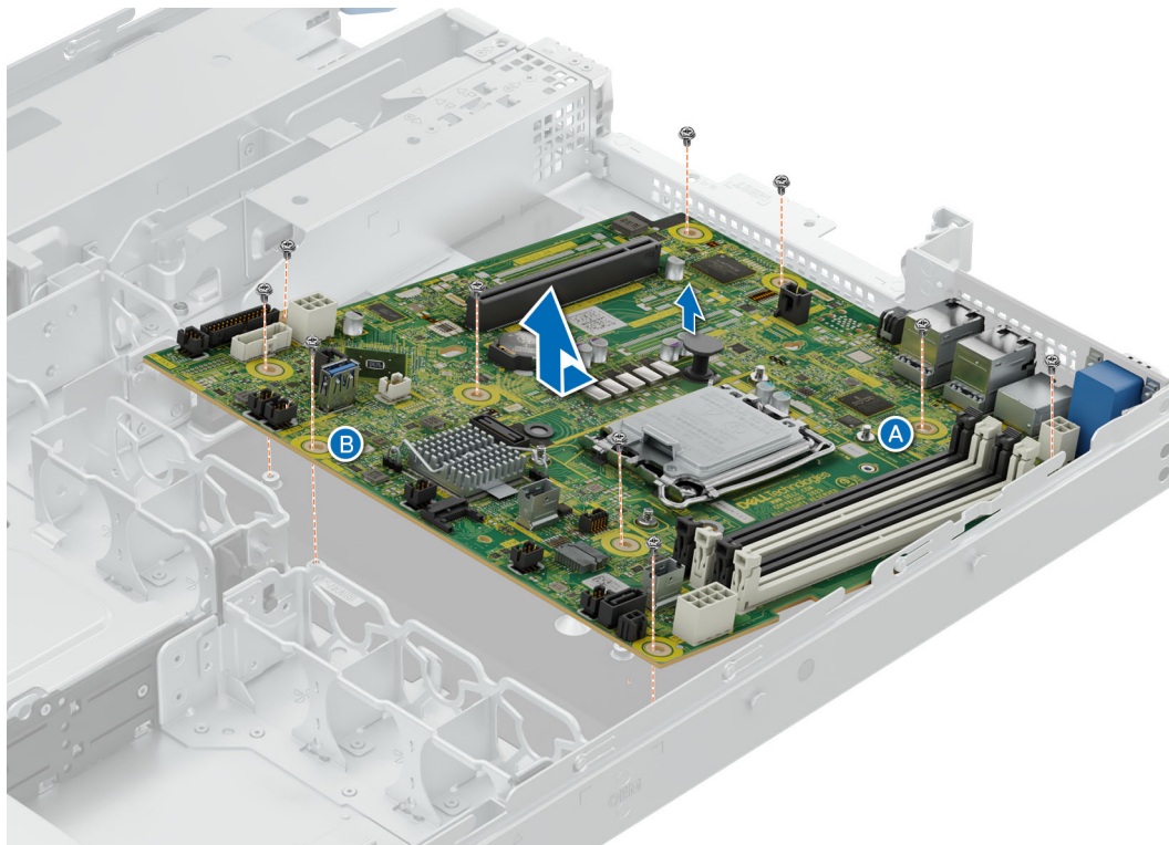
Ilustración 91. Extracción de la tarjeta madre
