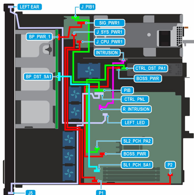
Ilustración 46. Configuración 7: cuatro unidades SATA de 2,5 pulgadas con PSU no cableada y BOSS-N1 (opcional)
