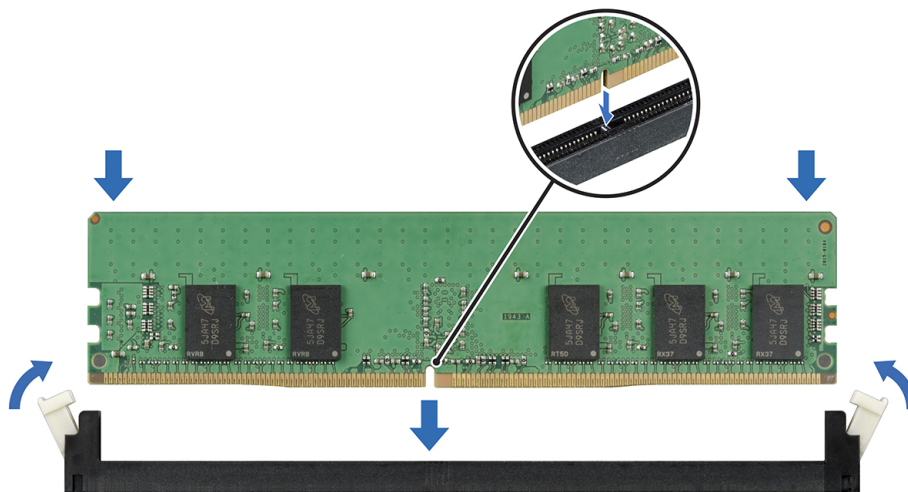
Ilustración 57. Instalación de un módulo de memoria
