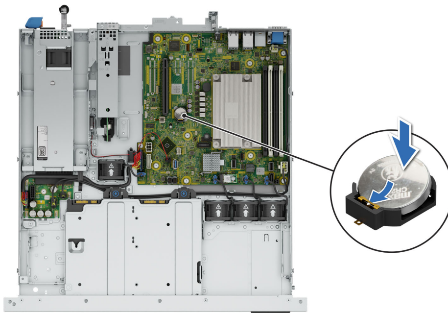
Ilustración 82. Instalación de la batería del sistema
