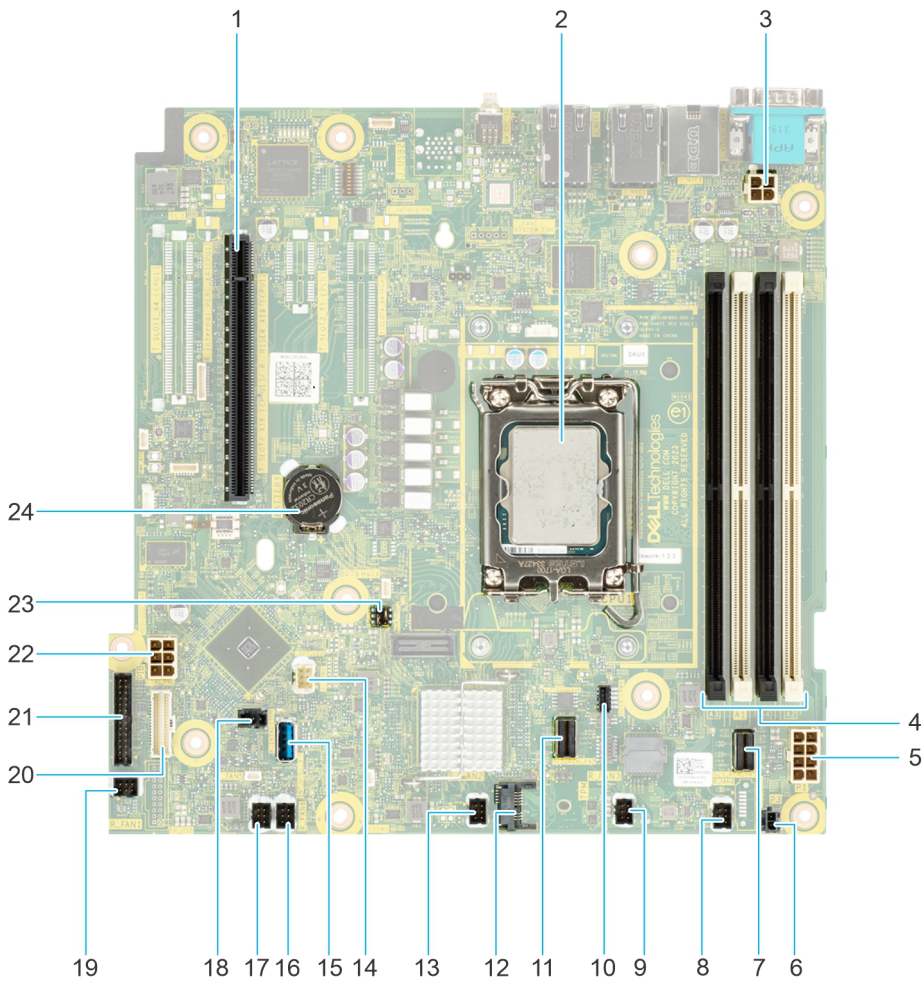
Ilustración 100. Puentes y conectores de la tarjeta madre del sistema
