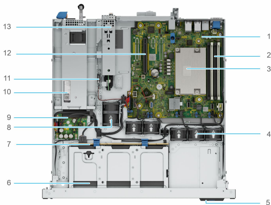
Ilustración 9. Vista interior del sistema con PSU no cableada y unidades de 2,5 pulgadas sin cubierta para flujo de aire y tarjeta elevadora
