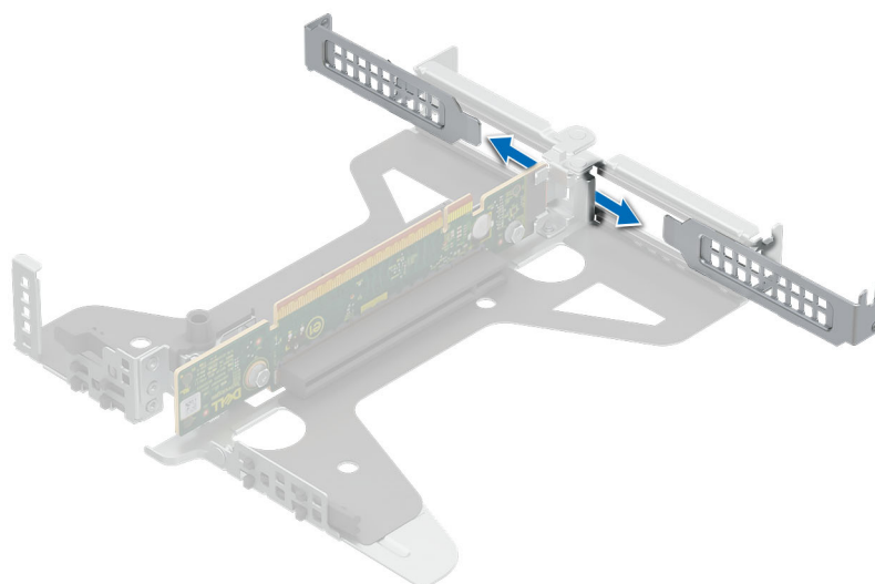
Ilustración 68. Extracción del soporte de relleno de la tarjeta elevadora
