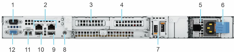
Ilustración 6. Vista posterior del sistema con PSU no cableada
