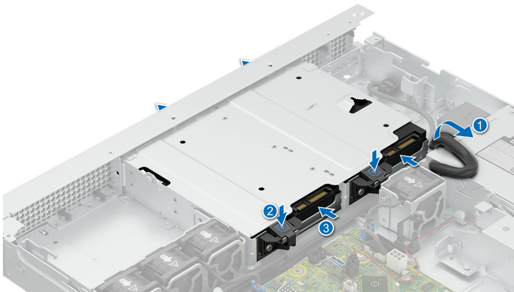
Ilustración 53. Extracción del disco duro cableado de 3,5 pulgadas
