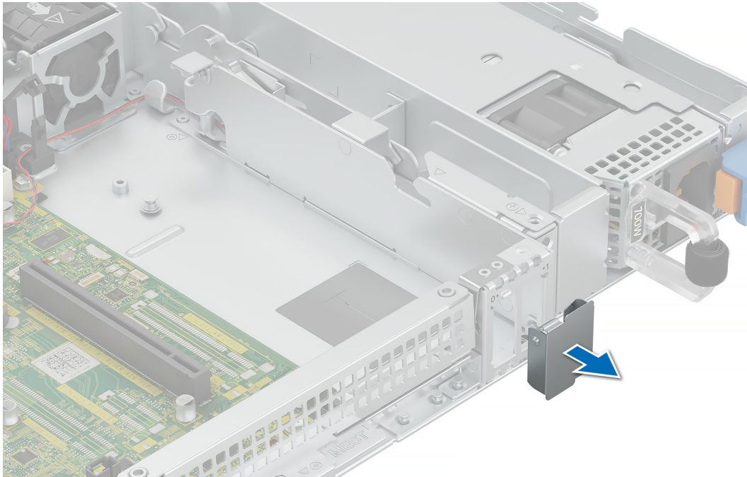
Ilustración 71. Extracción del panel de relleno de BOSS N1
