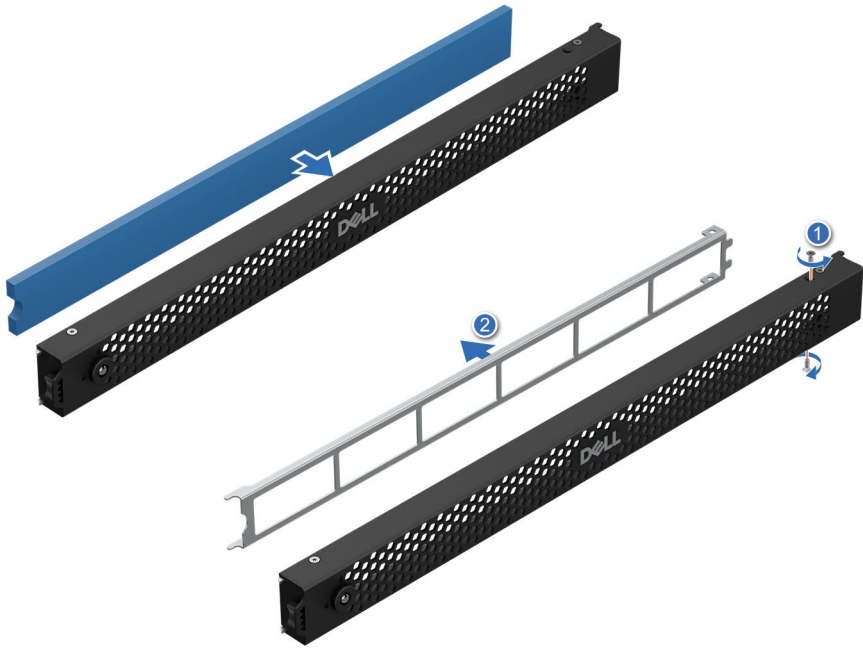
Ilustración 98. Instalación del filtro
