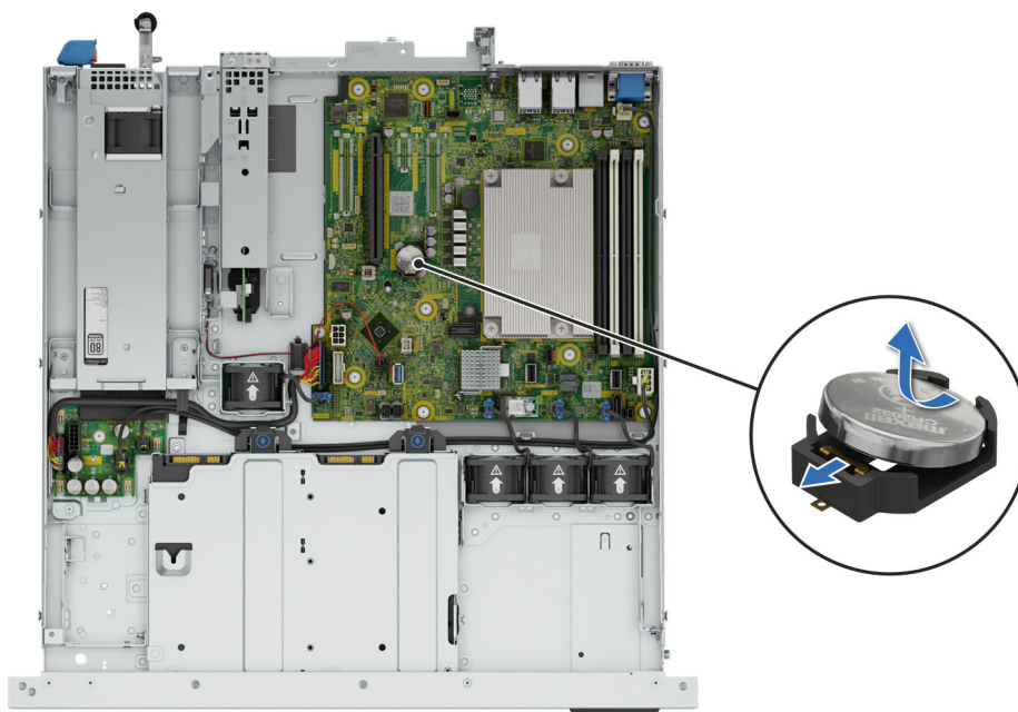
Ilustración 81. Extracción de la batería del sistema
