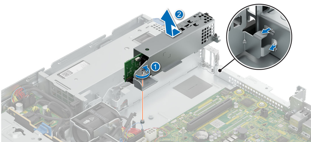
Ilustración 74. Extracción de la canastilla para BOSS-N1
