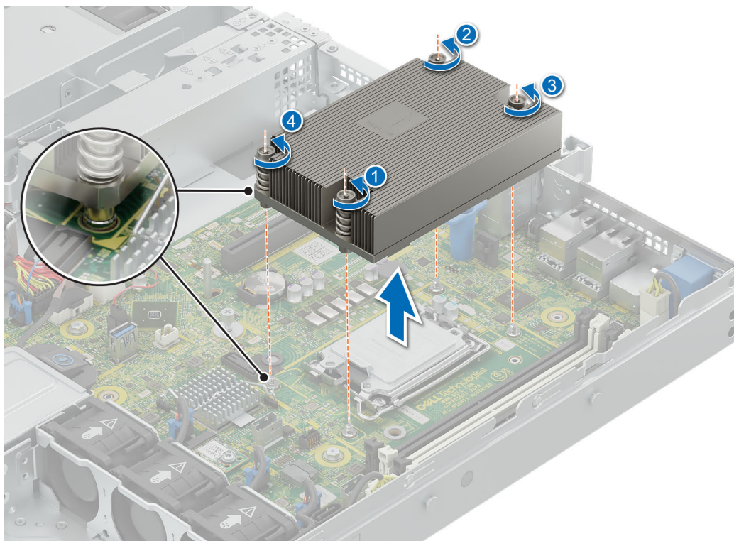
Ilustración 58. Extracción del módulo del disipador de calor
