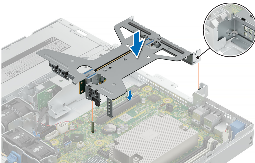
Ilustración 70. Instalación del soporte vertical
