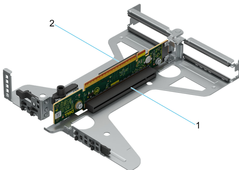
Ilustración 65. Tarjeta elevadora de mariposa
