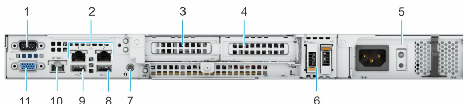
Ilustración 7. Vista posterior del sistema con PSU cableada
