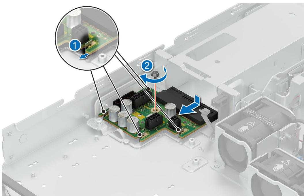
Ilustración 90. Instalación de la PIB
