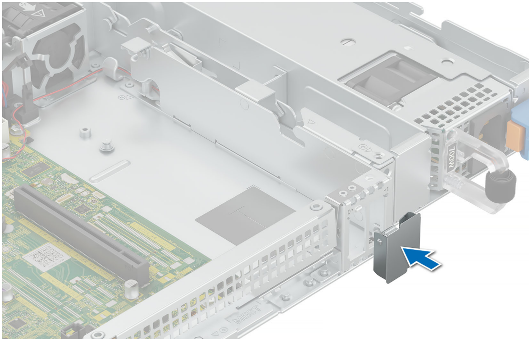
Ilustración 72. Instalación del panel de relleno de BOSS N1
