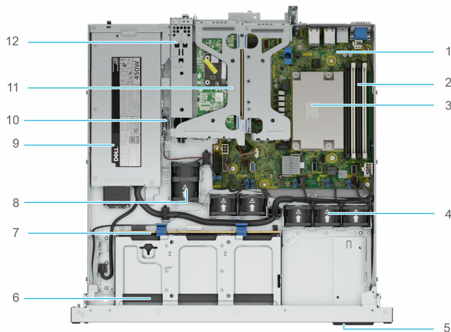
Ilustración 10. Vista interior del sistema con PSU cableada y unidades de 2,5 pulgadas sin cubierta para flujo de aire
