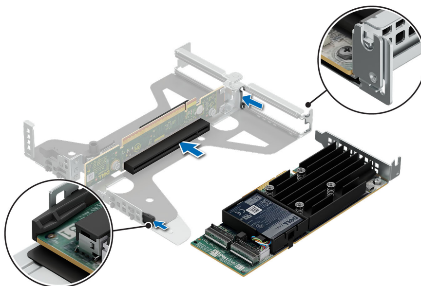
Ilustración 69. Instalación de una tarjeta de expansión en la tarjeta elevadora
