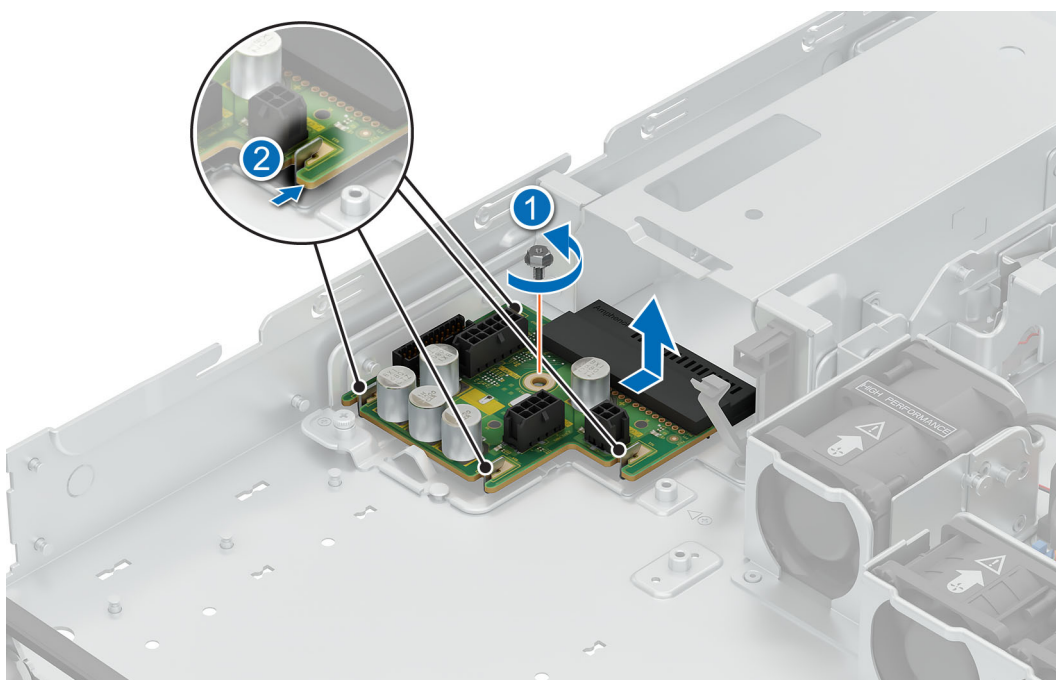
Ilustración 89. Extracción de la PIB
