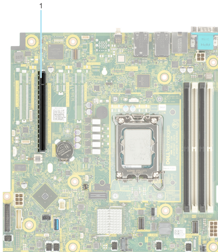
Ilustración 64. Conectores de la ranura de tarjeta elevadora para tarjetas de expansión
