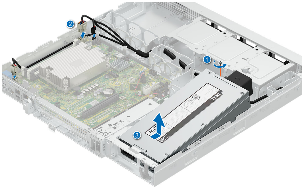
Figure 85. Retrait d'un bloc d'alimentation câblé
