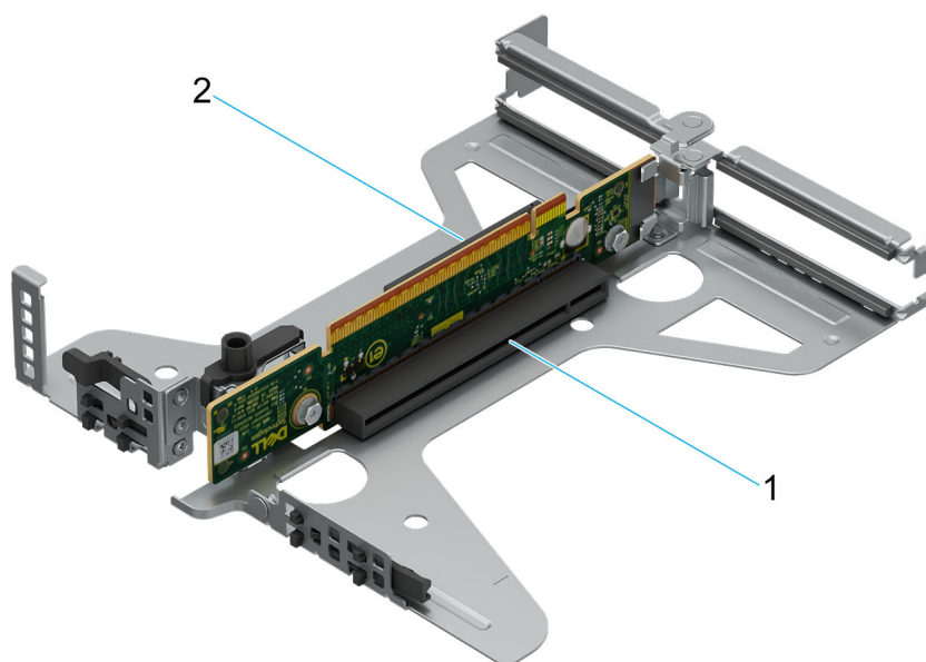
Figure 65. Carte de montage papillon
