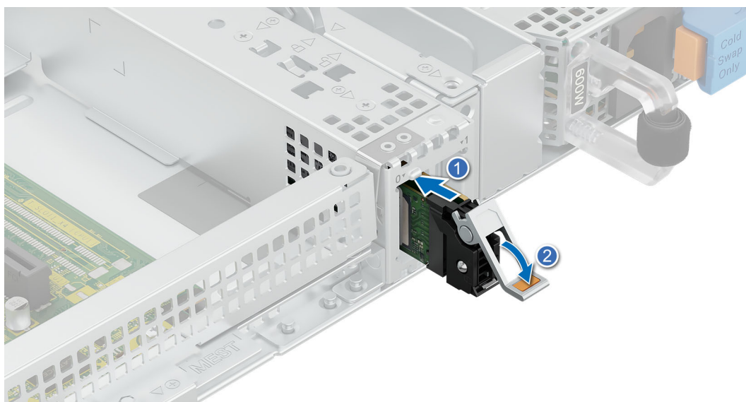
Figure 80. Installation du module BOSS-N1 M.2
