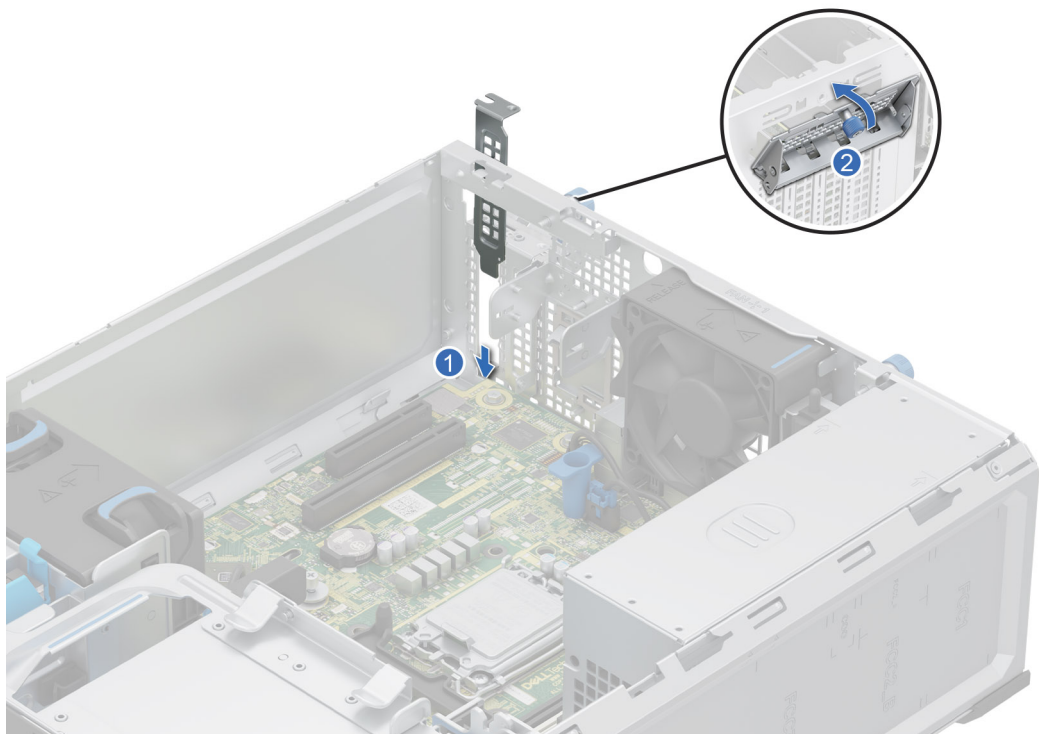
Abbildung 46. Einsetzen des Metallabdeckblechs
