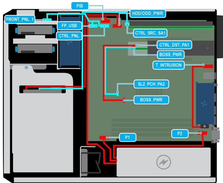
Abbildung 33. Kabelführung – 3 x 3,5-Zoll-PERC-SATA-Laufwerke
