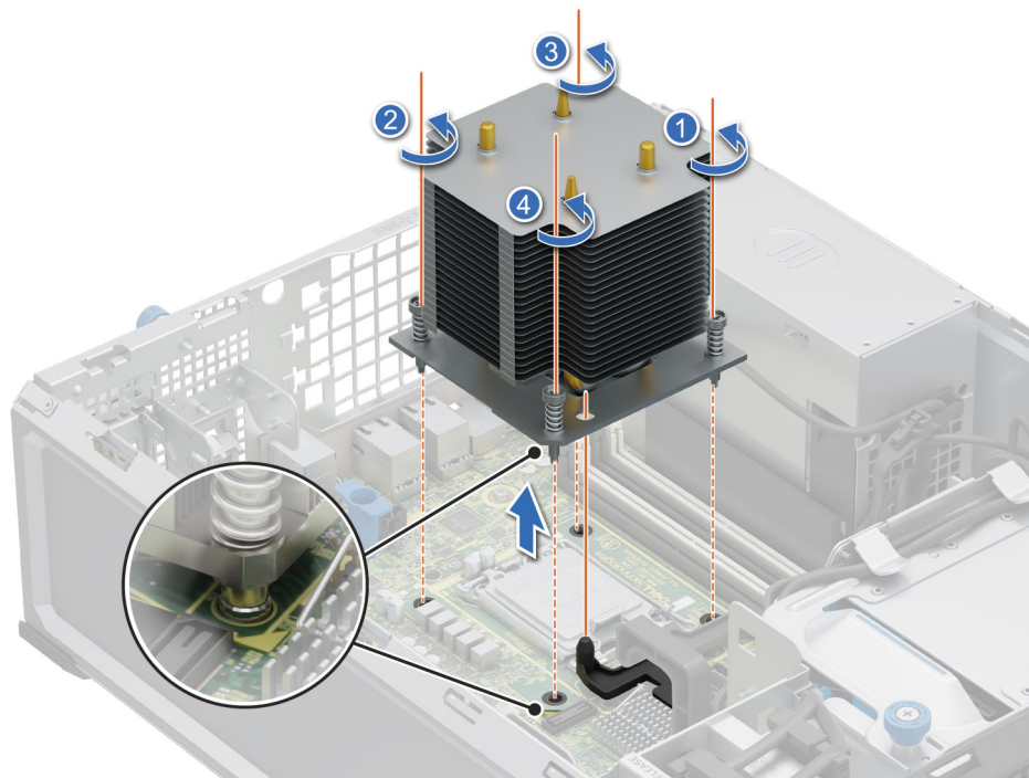
Abbildung 39. Entfernen des Kühlkörpers
