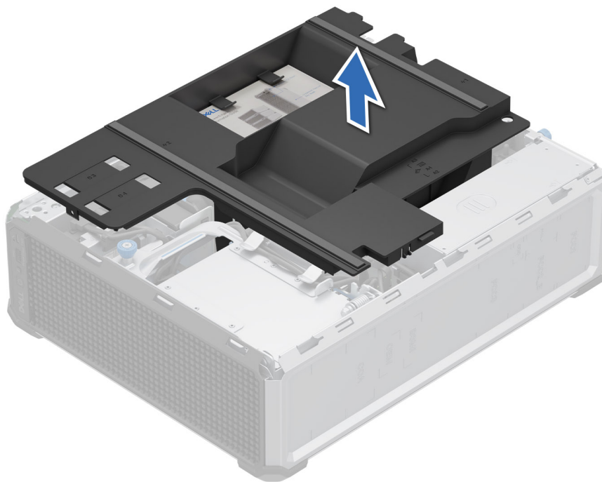
Abbildung 16. Entfernen des Luftkanals
