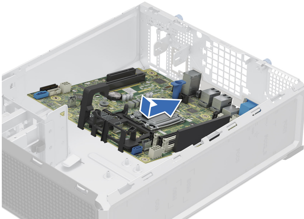
Abbildung 65. Einbauen der Systemplatine
