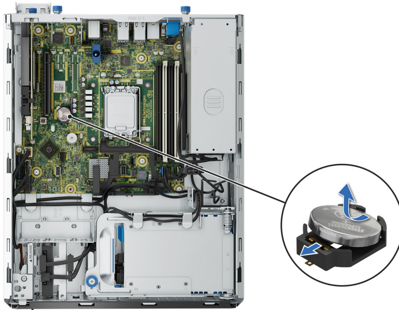
Abbildung 61. Entfernen der Systembatterie
