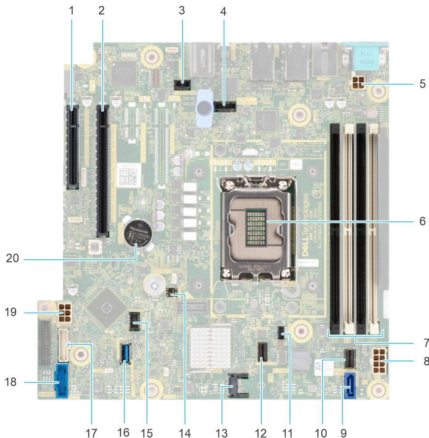
Abbildung 74. Layout der Systemplatine
