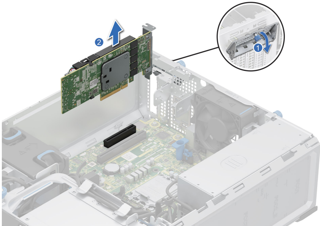
Abbildung 45. Entfernen einer Erweiterungskarte
