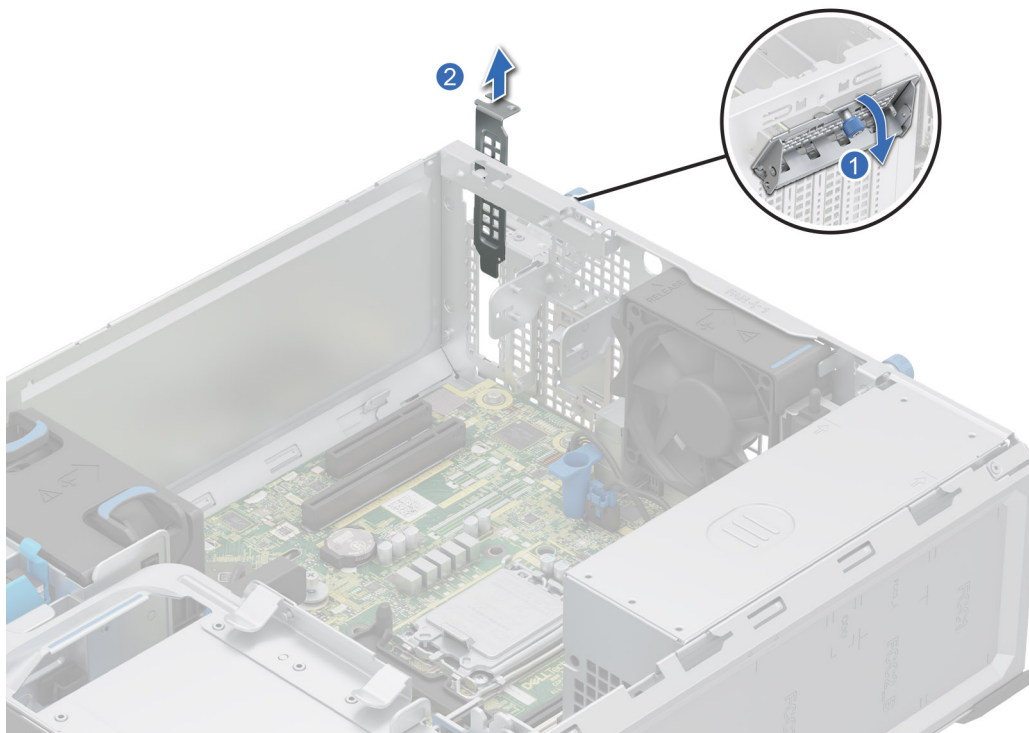
Abbildung 47. Entfernen des Metallabdeckblechs
