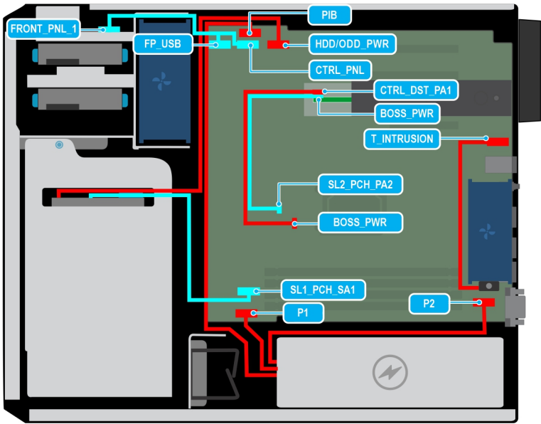
Abbildung 32. Kabelführung – 3 x 3,5-Zoll-Chip-SATA-Laufwerke
