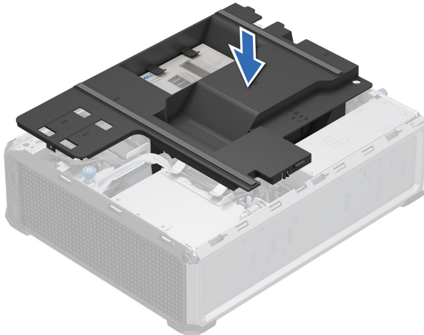
Abbildung 17. Installieren des Luftkanals
