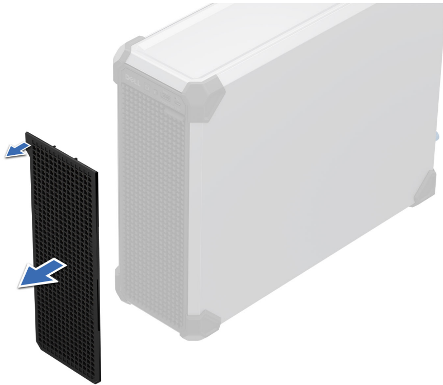
Abbildung 12. Entfernen der Frontverkleidung
