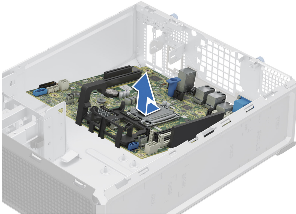
Abbildung 64. Entfernen der Hauptplatine
