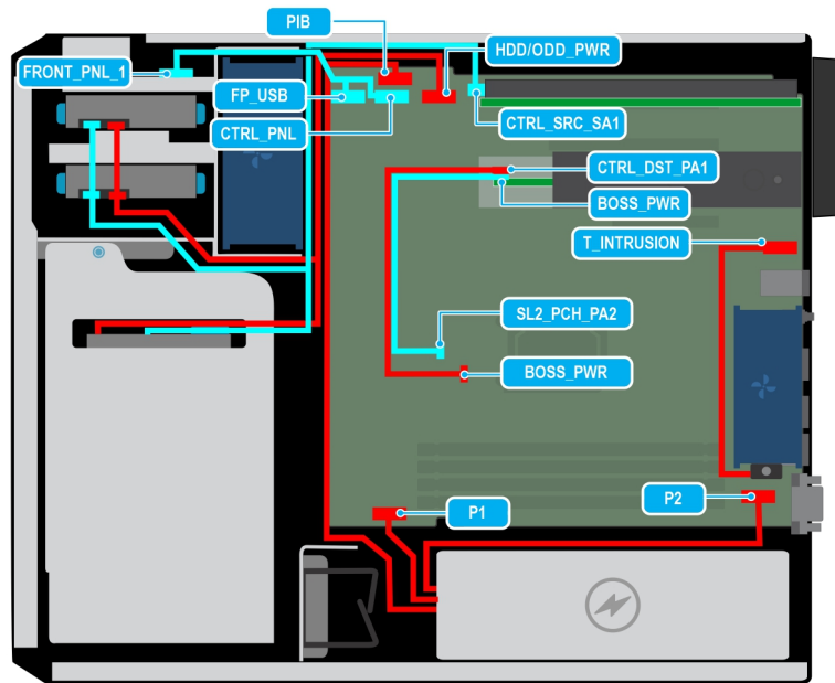
Abbildung 35. Kabelführung – 3 x 3,5-Zoll- + 2 x 2,5-Zoll- PERC-SATA-Laufwerke
