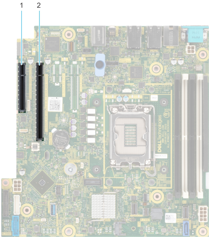
Abbildung 44. PCIe-Steckplätze auf der Systemplatine
