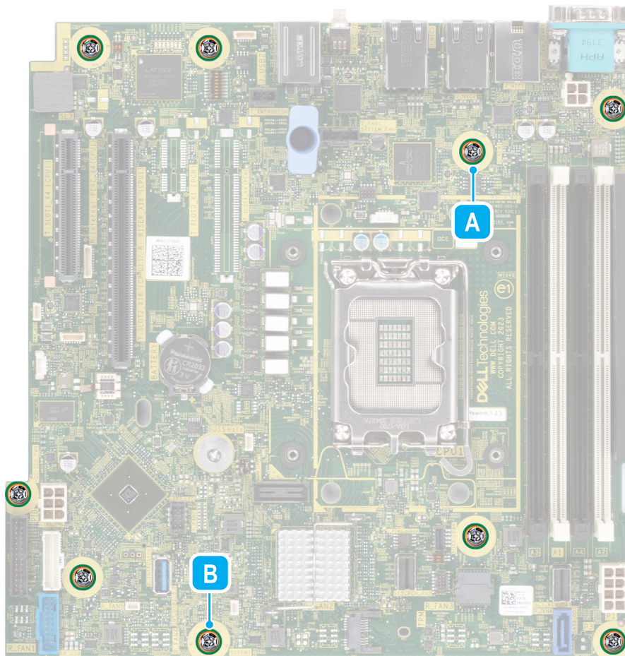
Abbildung 66. Position der Schrauben der Systemplatine
