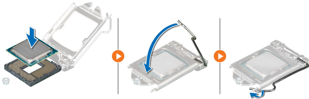
Abbildung 41. Einbauen des Prozessors
