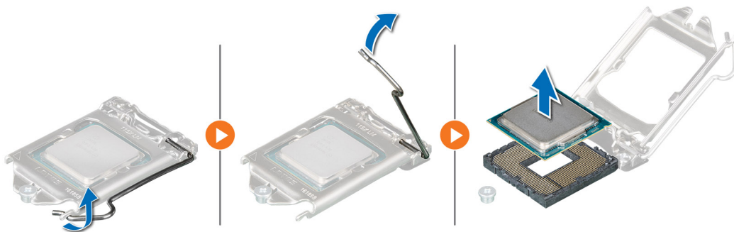
Abbildung 40. Entfernen des Prozessors
