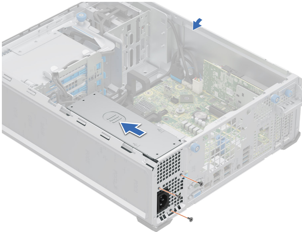
Abbildung 59. Entfernen eines verkabelten Netzteils
