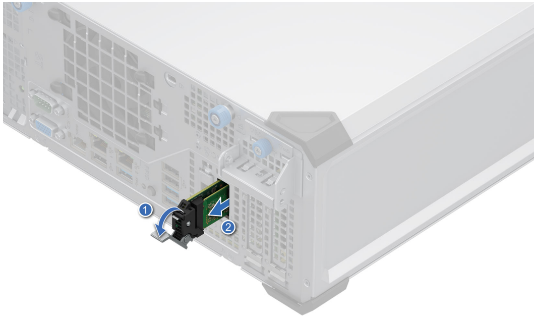
Abbildung 53. Entfernen des BOSS-N1-Kartenträgers
