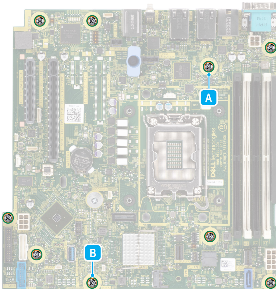
Abbildung 63. Position der Schrauben der Systemplatine
