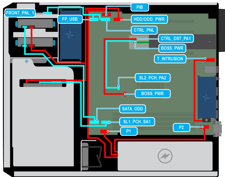
Abbildung 34. Kabelführung – 3 x 3,5-Zoll- + 2 x 2,5-Zoll-Chip-SATA-Laufwerke
