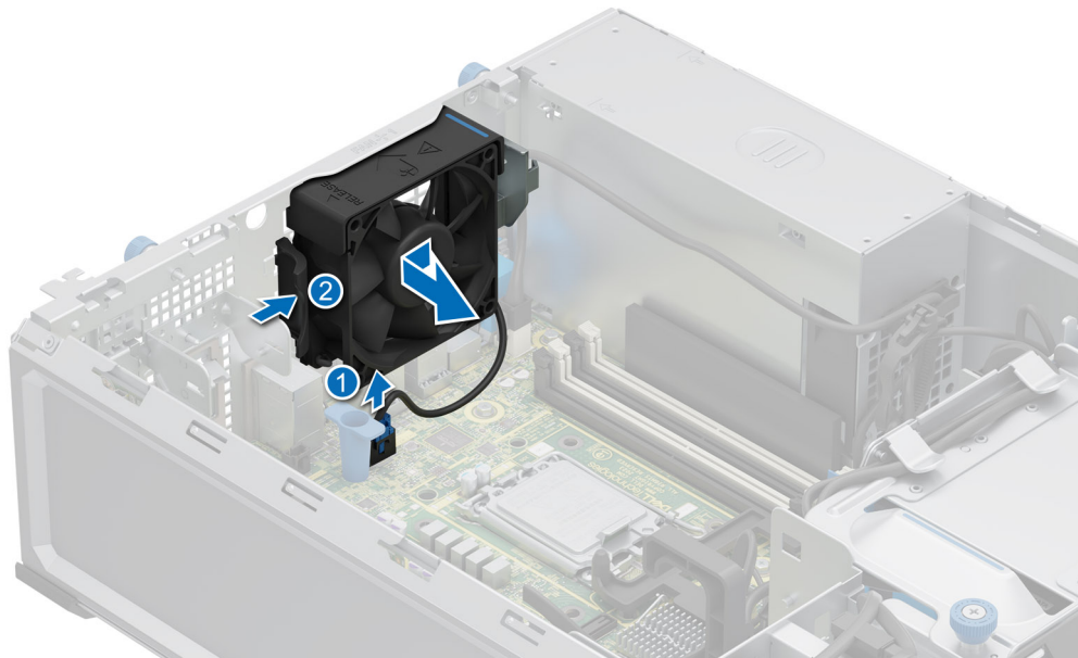
Abbildung 28. Kühlungsüfter entfernen
