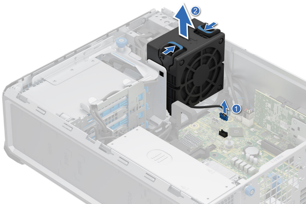
Abbildung 29. Entfernen des Hochleistungs-PCI-Lüfters (HPR)
