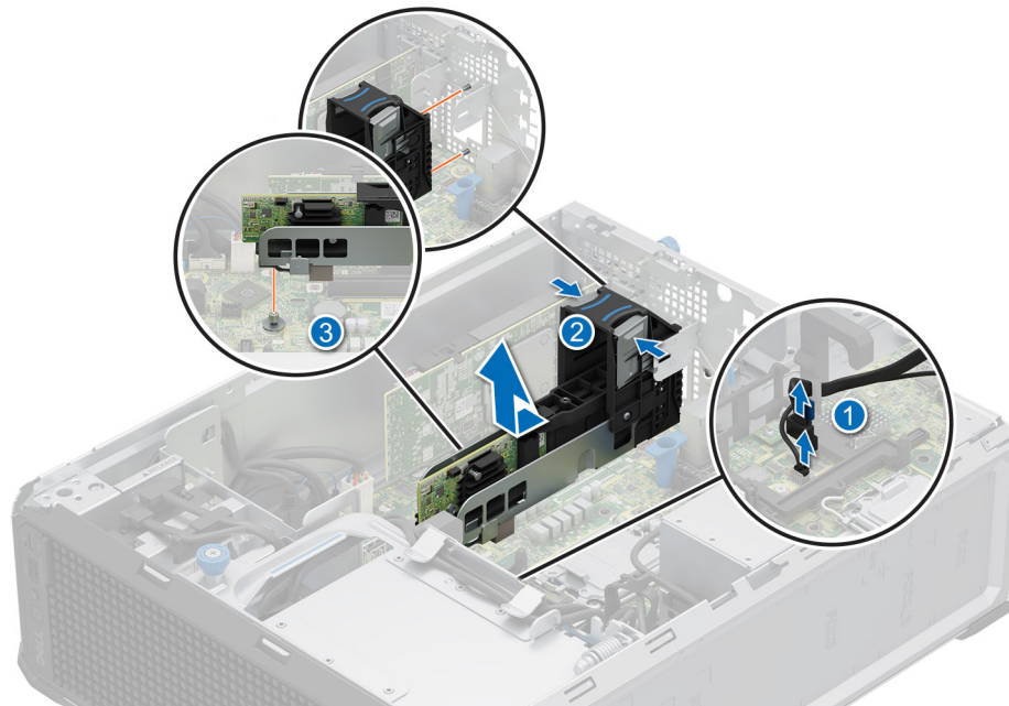
Abbildung 49. Entfernen des BOSS-N1-Moduls
