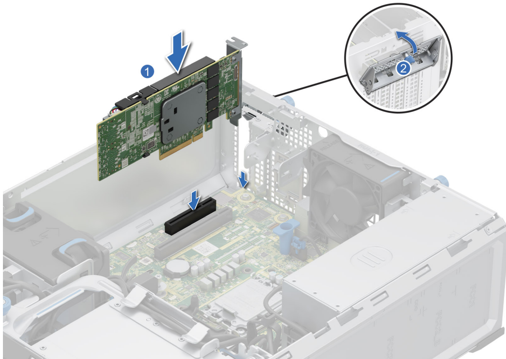
Abbildung 48. Installieren einer Erweiterungskarte
