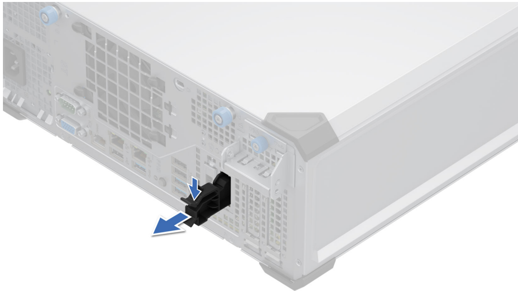
Abbildung 51. Entfernen des Platzhalters für das BOSS-N1-Modul
