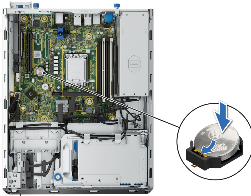
Abbildung 62. Installieren der Systembatterie
