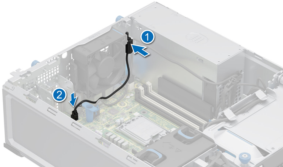
Abbildung 19. Installieren des Schutzschaltermoduls
