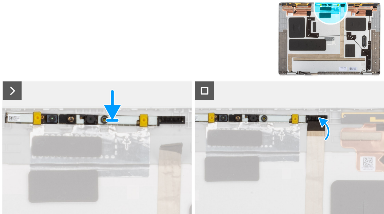
Abbildung 83. Installieren der RGB/IR-Kamera
