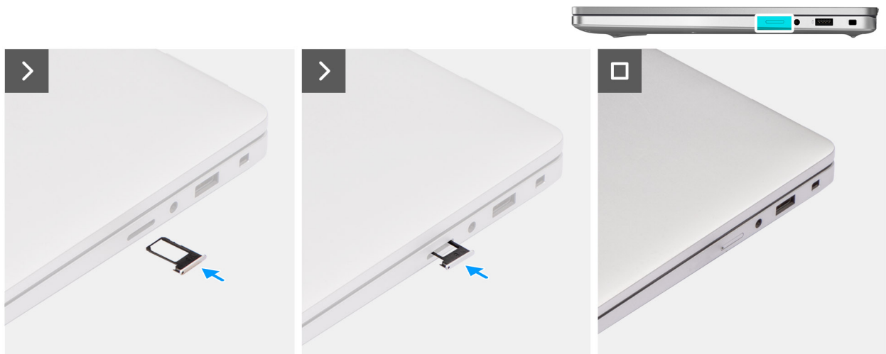
Abbildung 21. Installieren des SIM-Kartenfachs
