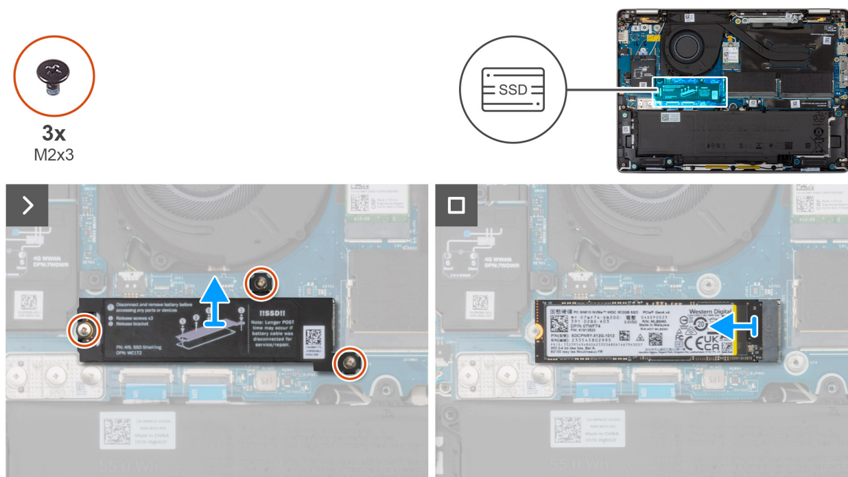
Abbildung 38. Entfernen der M.2-2280-SSD
