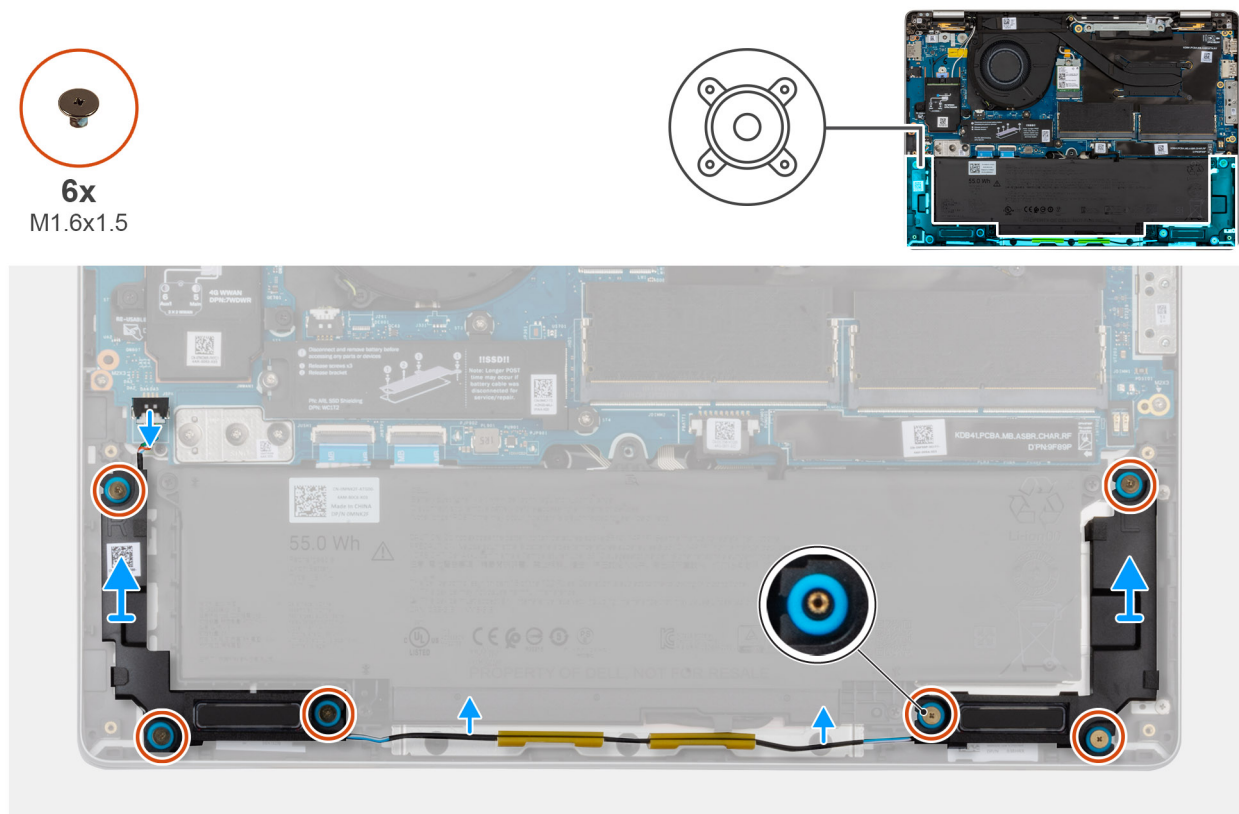
Abbildung 42. Entfernen der Lautsprecher
