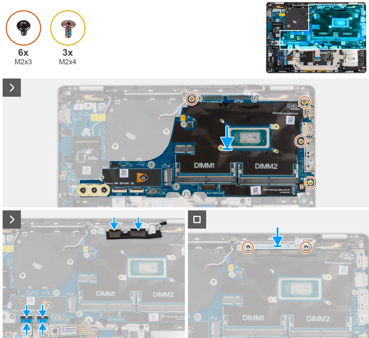
Abbildung 53. Einbauen der Systemplatine
