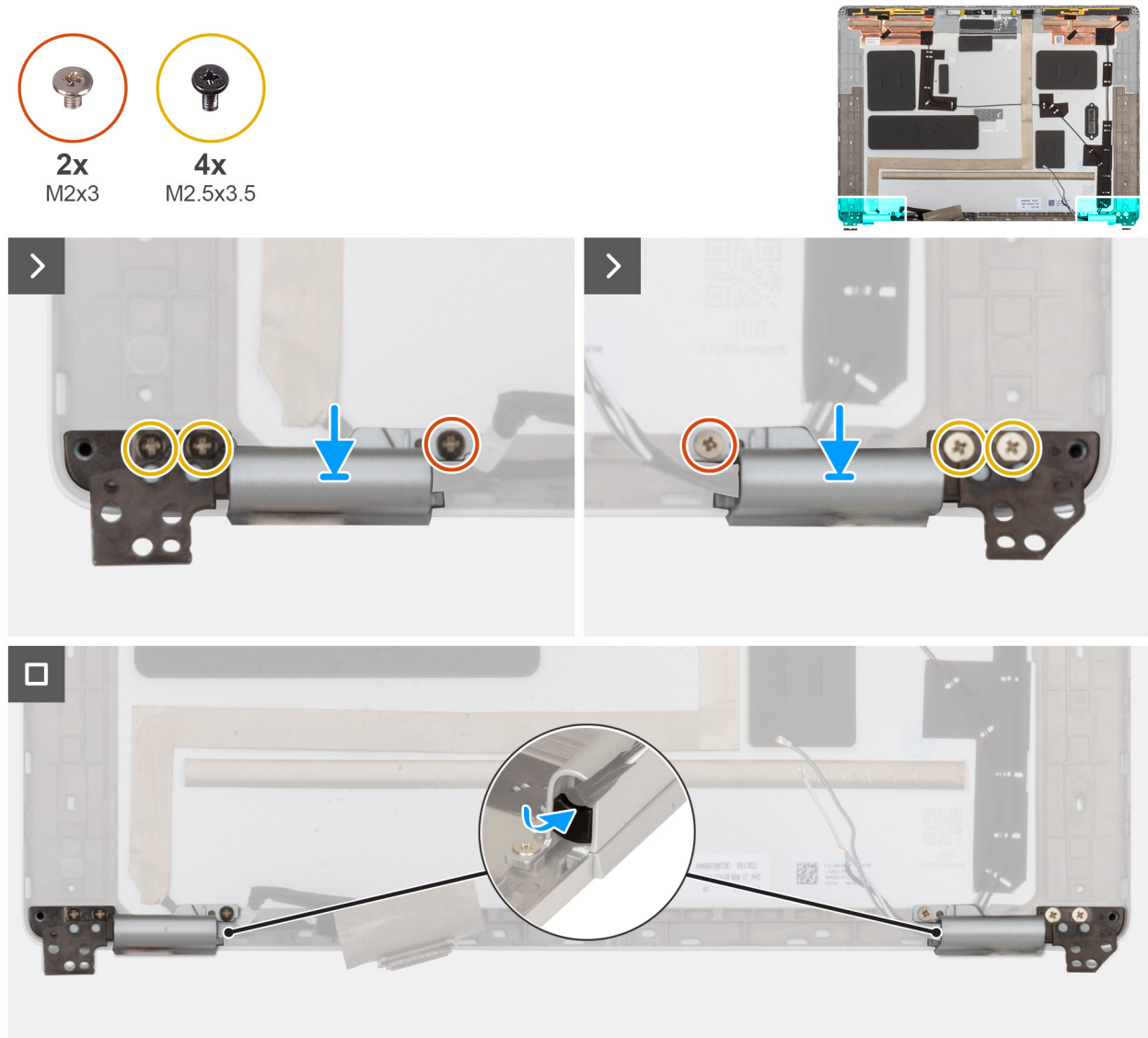
Abbildung 81. Einbauen der Bildschirmscharnierabdeckungen
