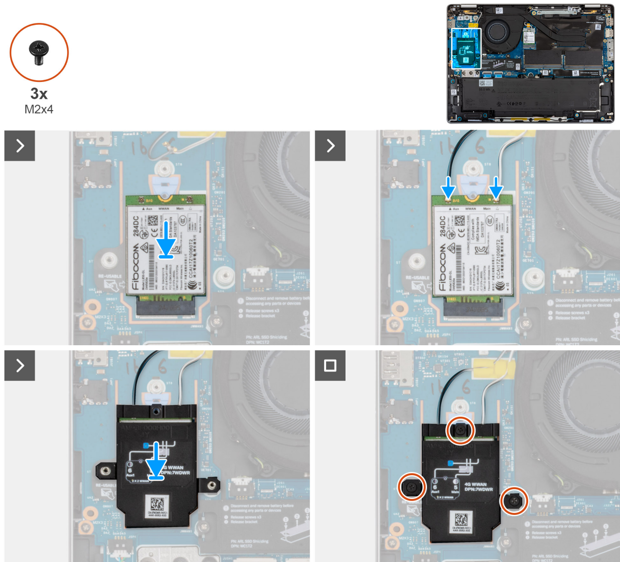
Abbildung 35. Einbauen der WWAN-Karte
