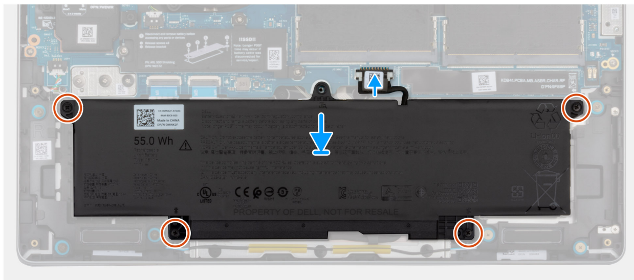
Abbildung 29. Einsetzen des Akkus
