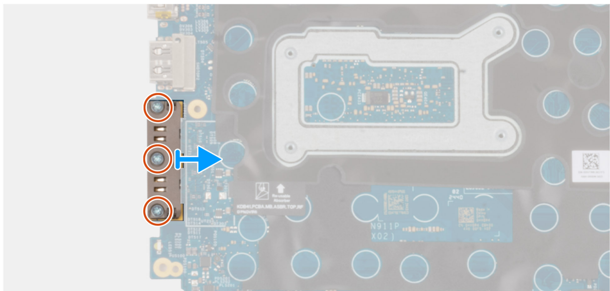
Abbildung 58. Entfernen des USB-Type-C-Anschlussmoduls
