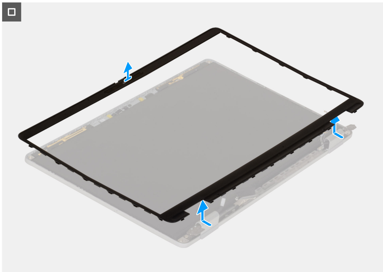
Abbildung 72. Entfernen der Bildschirmblende
