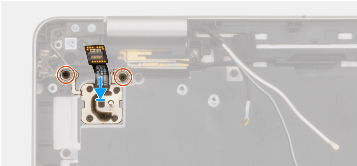
Abbildung 63. Installieren des Netzschalters mit optionalem Fingerabdruck-Lesegerät
