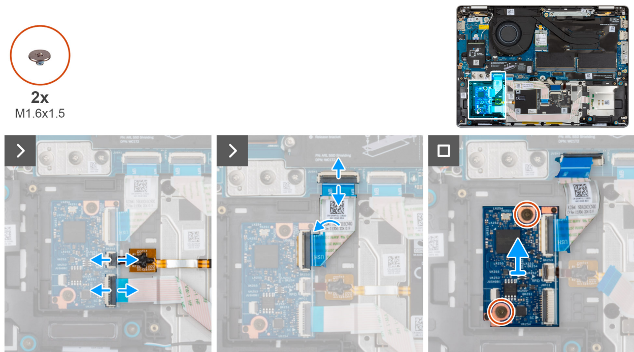
Abbildung 46. Entfernen der USH-Platine
