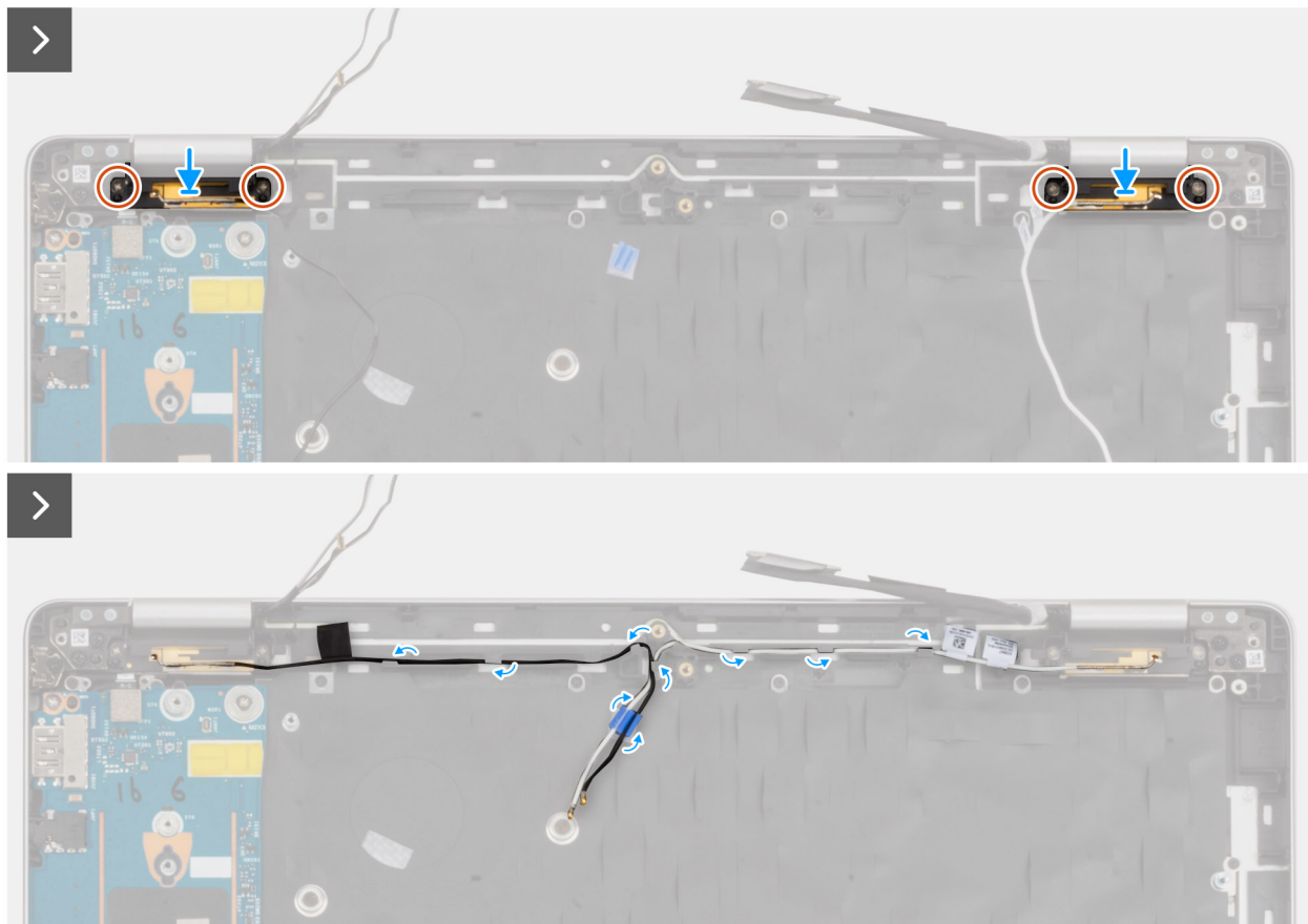
Abbildung 56. Einbauen des WLAN-Antennenmoduls
