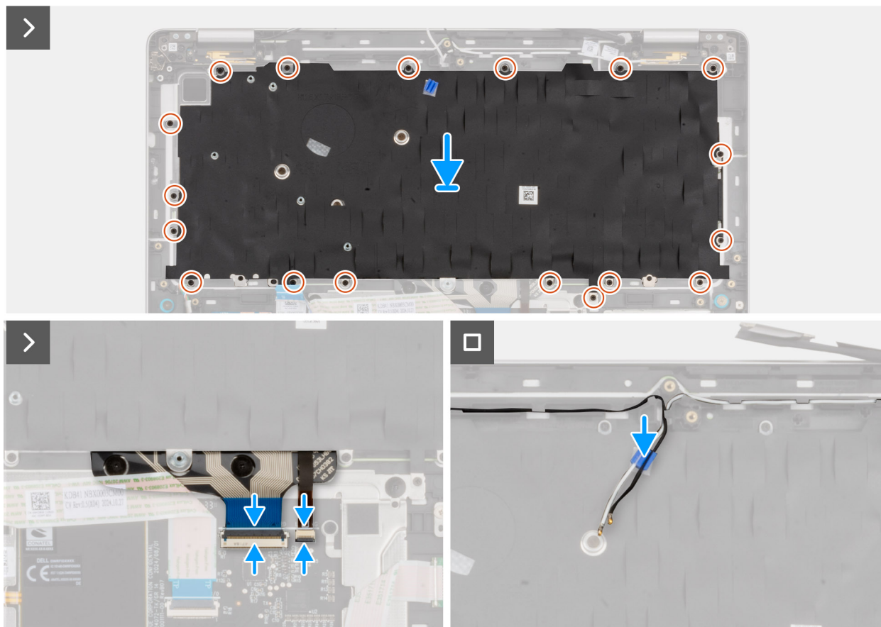
Abbildung 101. Einbauen der Tastatur
