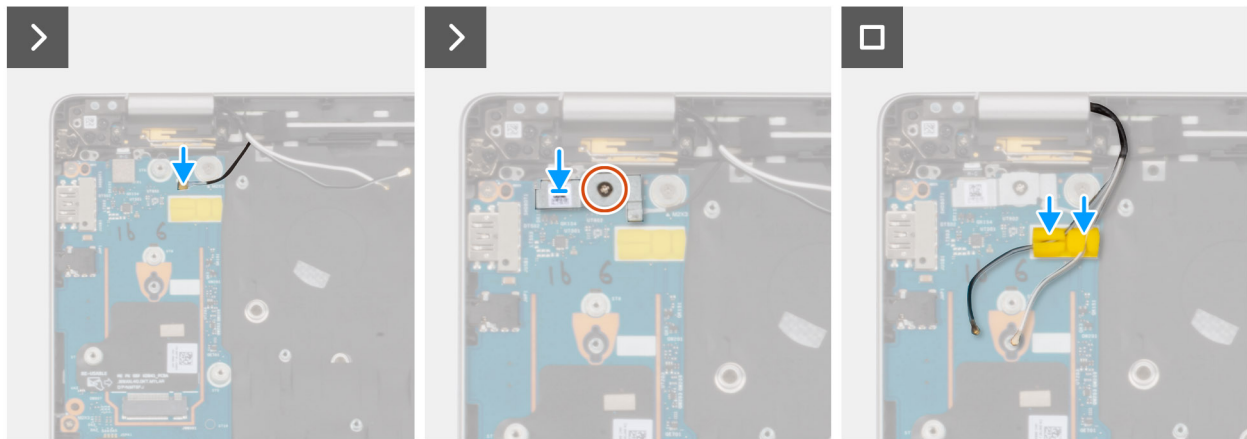
Abbildung 57. Einbauen des WLAN-Antennenmoduls
