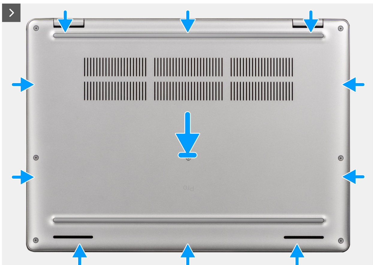
Abbildung 26. Anbringen der Bodenabdeckung
