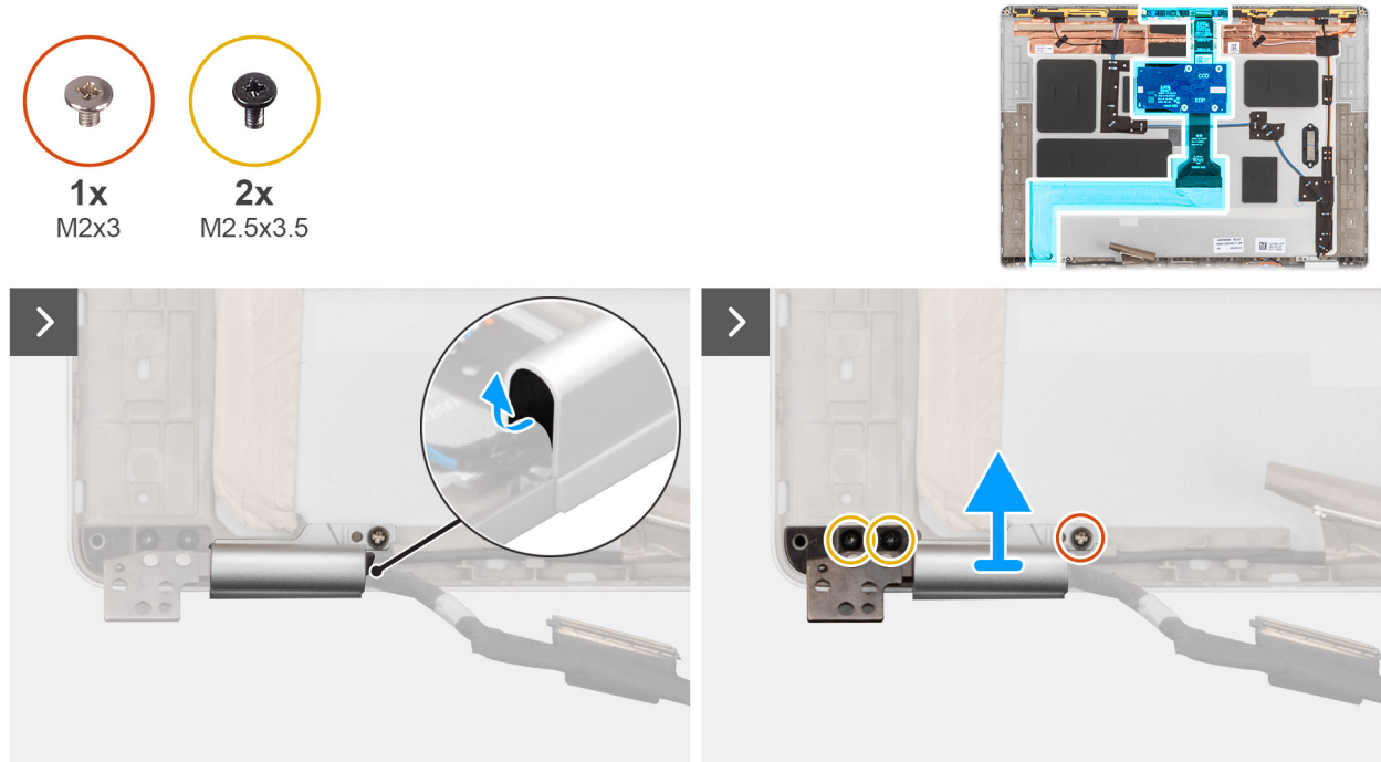
Abbildung 84. Entfernen des Bildschirmkabels
