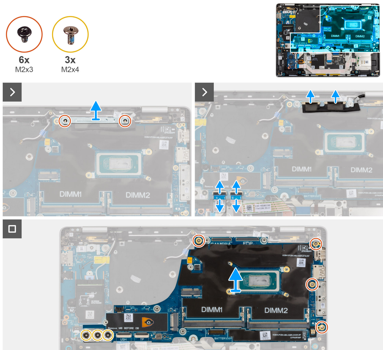
Abbildung 51. Entfernen der Systemplatine
