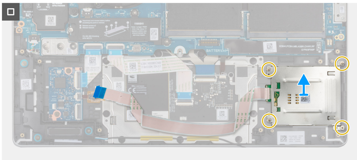
Abbildung 48. Entfernen des Smartcardlesegeräts
