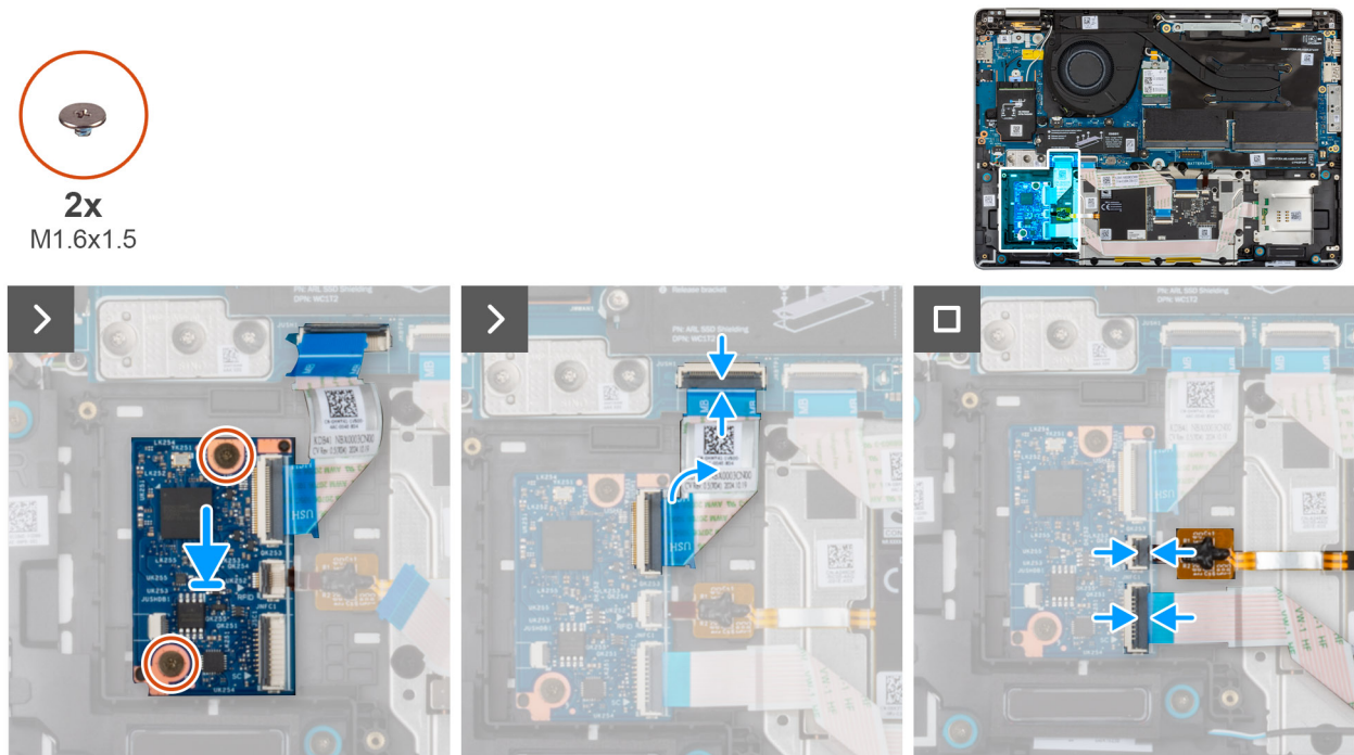
Abbildung 47. Einbauen der USH-Platine
