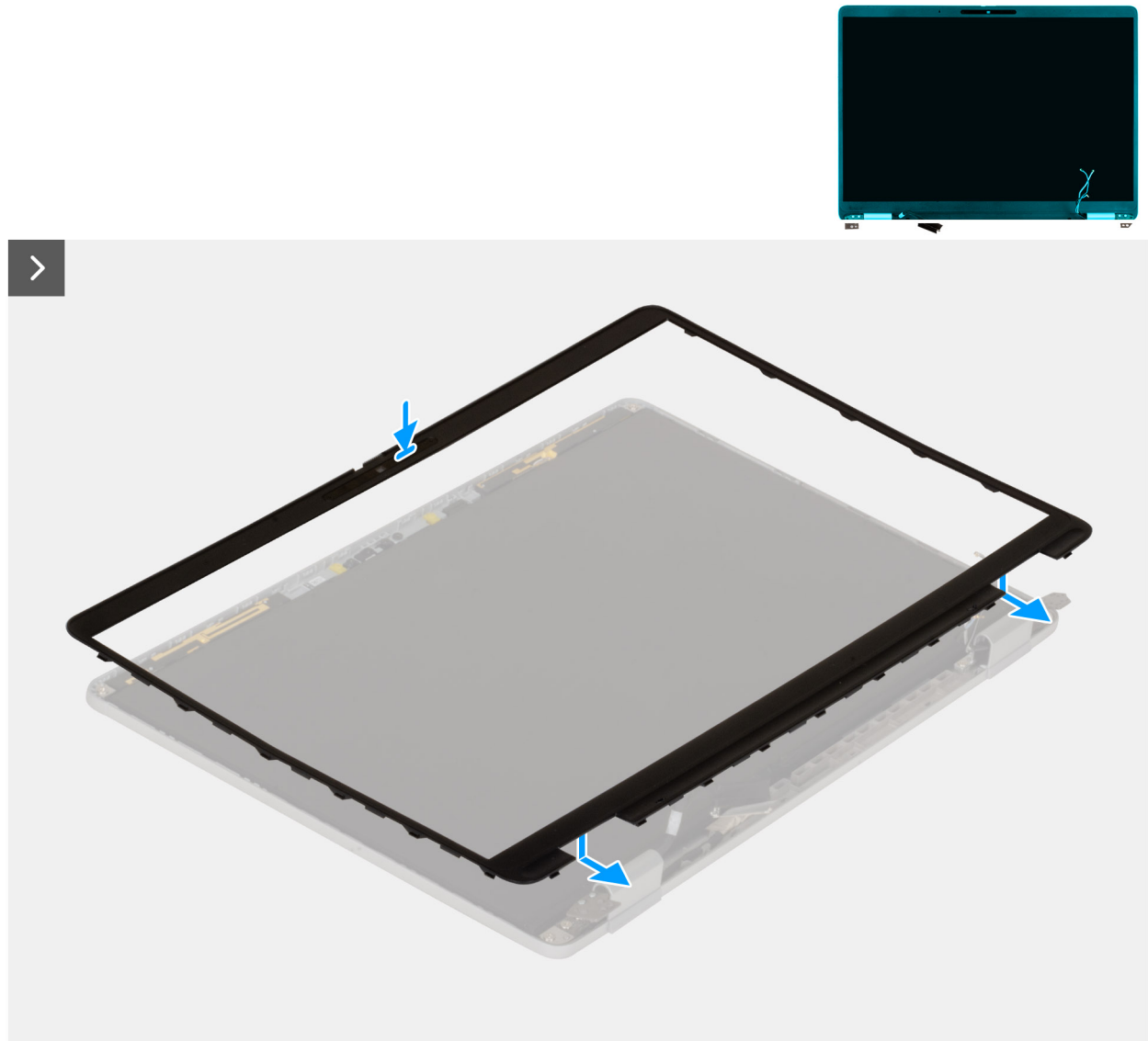
Abbildung 73. Einbauen der Bildschirmblende
