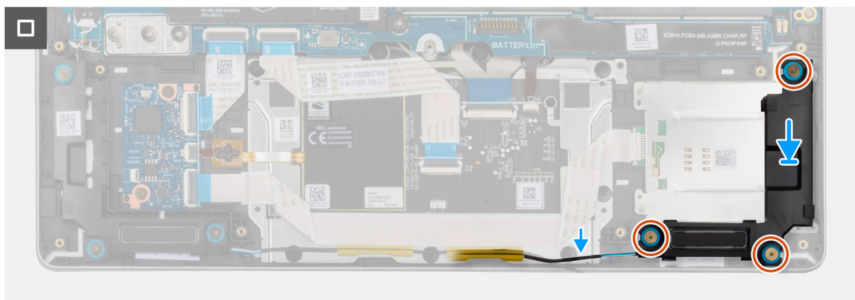
Abbildung 49. Installieren des Smartcardlesegeräts
