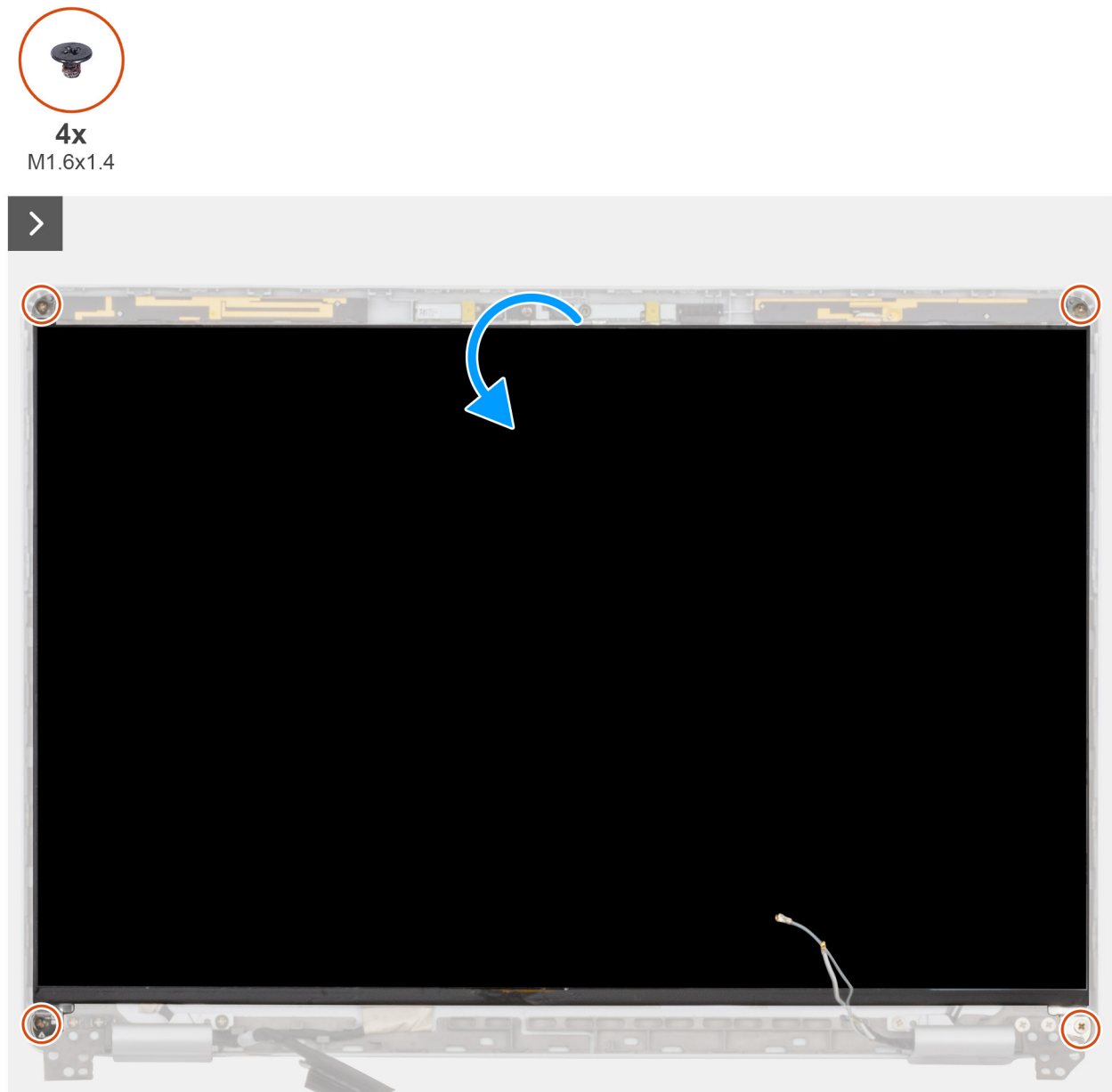
Abbildung 75. Entfernen des Bildschirms
