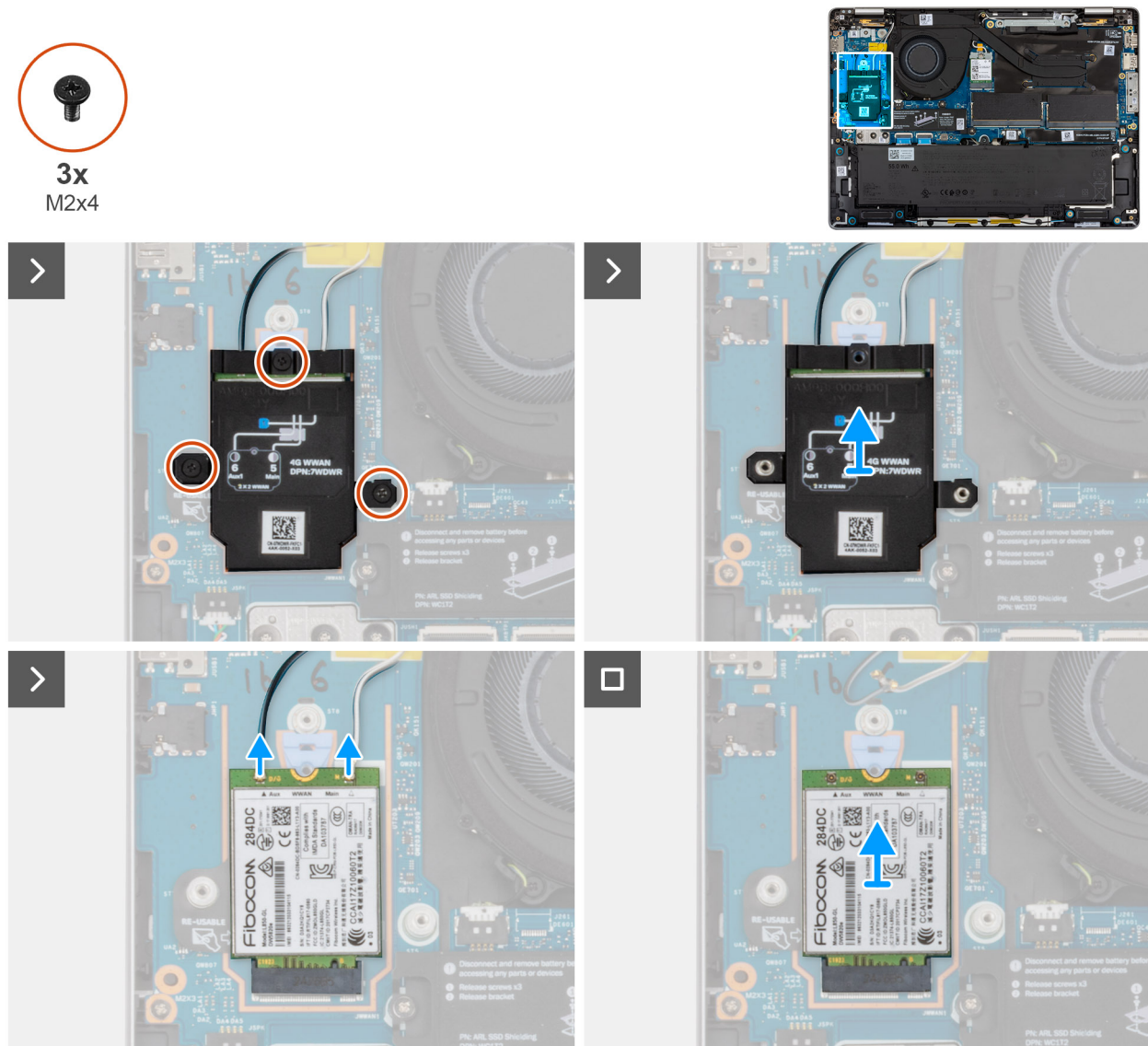
Abbildung 34. Entfernen der WWAN-Karte
