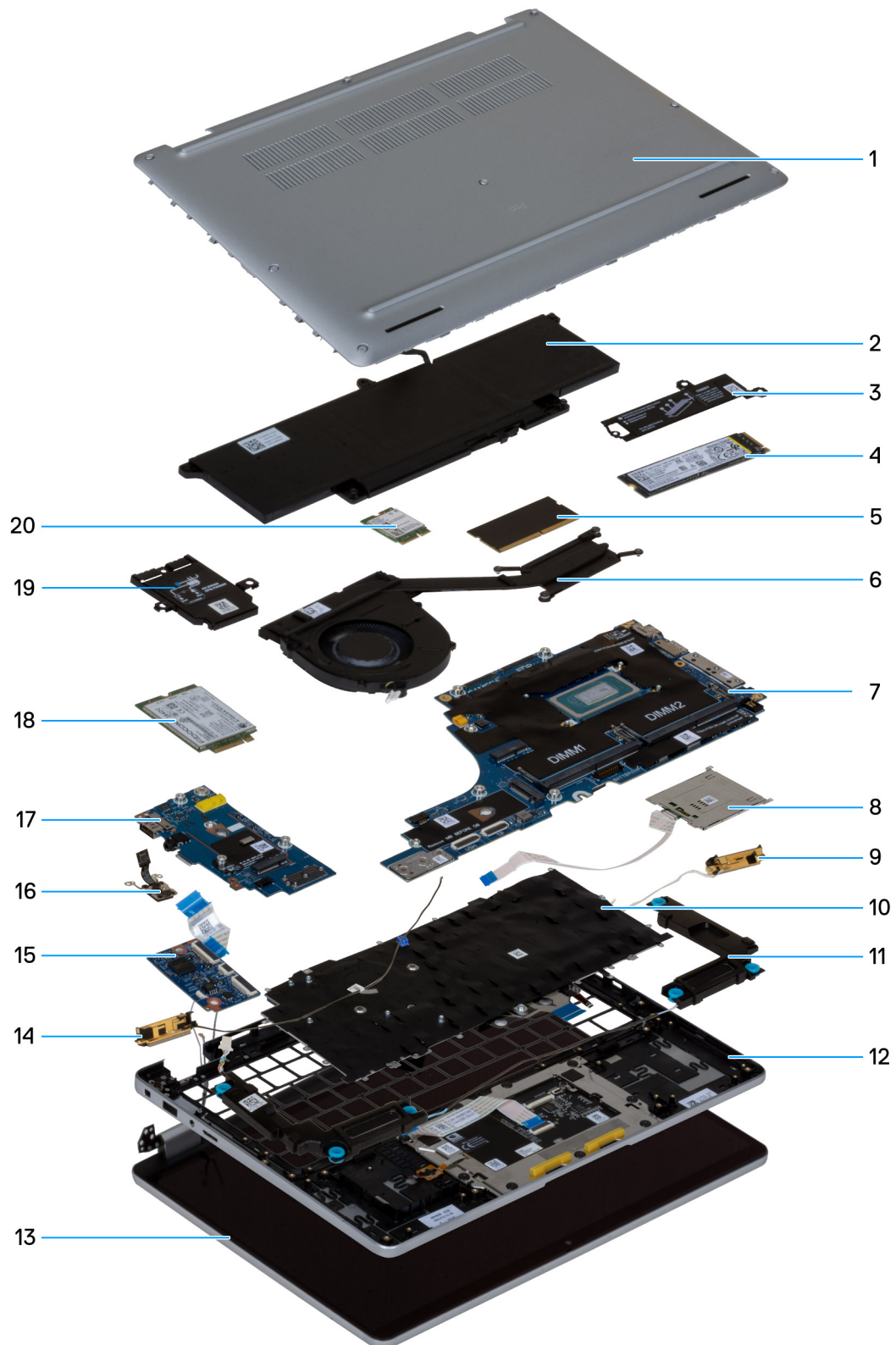
Abbildung 19. Hauptkomponenten von Dell Pro 14 Plus/Dell Pro 14 Plus 2-in-1
