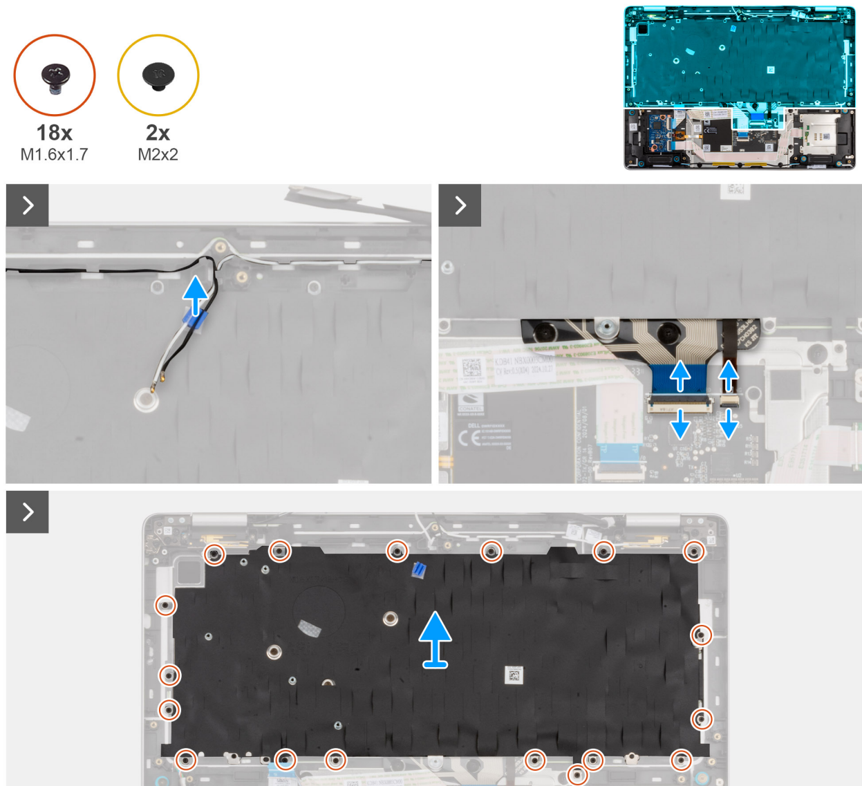
Abbildung 98. Entfernen der Tastatur
