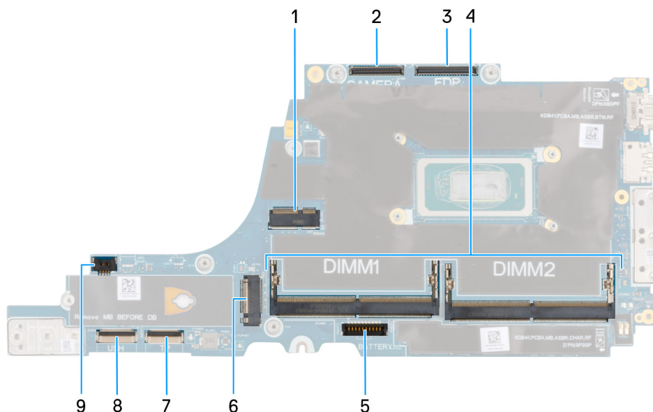
Abbildung 52. Anschlüsse auf der Hauptplatine
