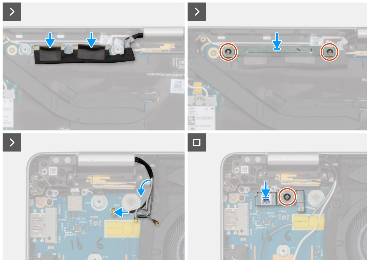
Abbildung 67. Einbauen der Displaybaugruppe
