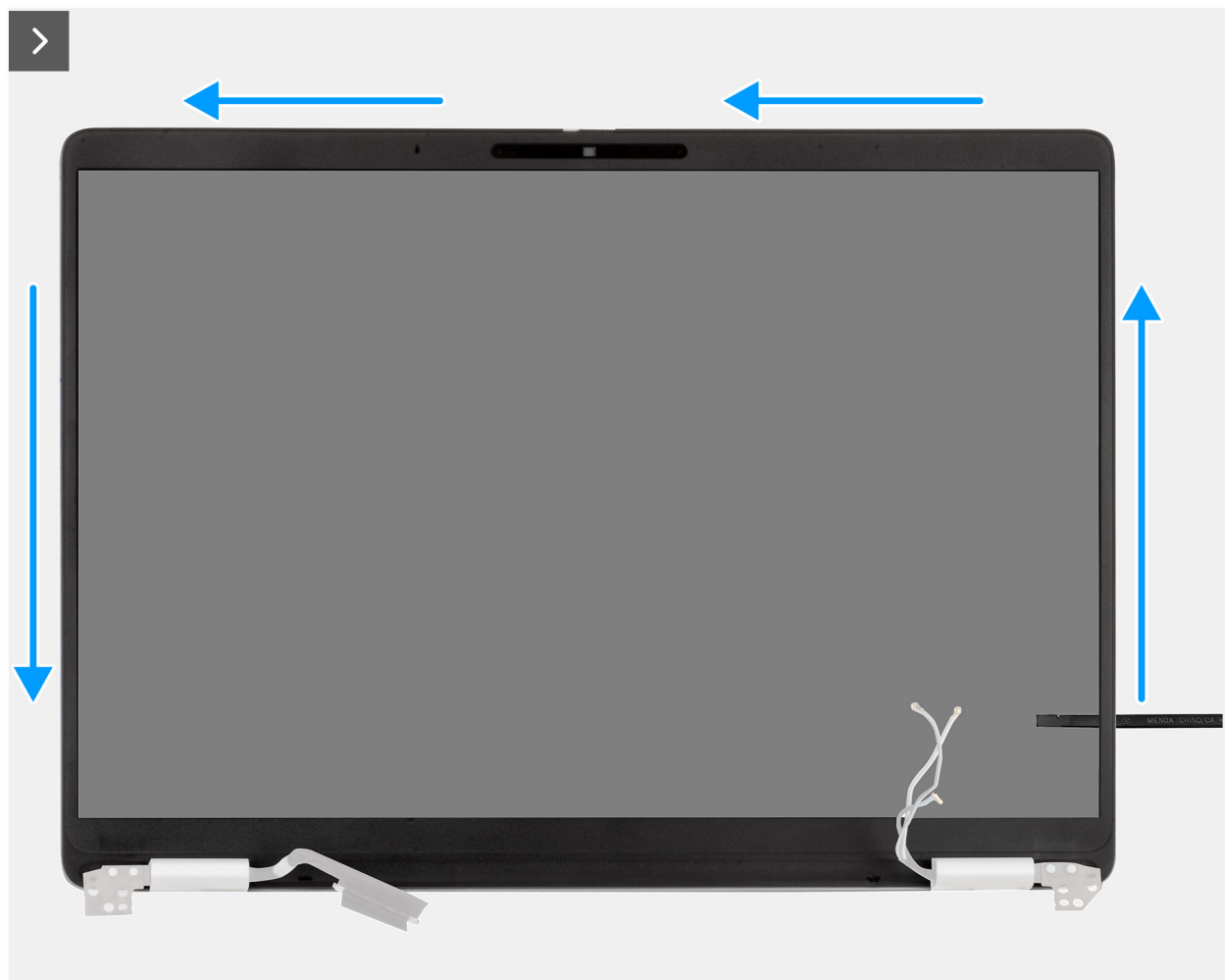
Abbildung 71. Entfernen der Bildschirmblende
