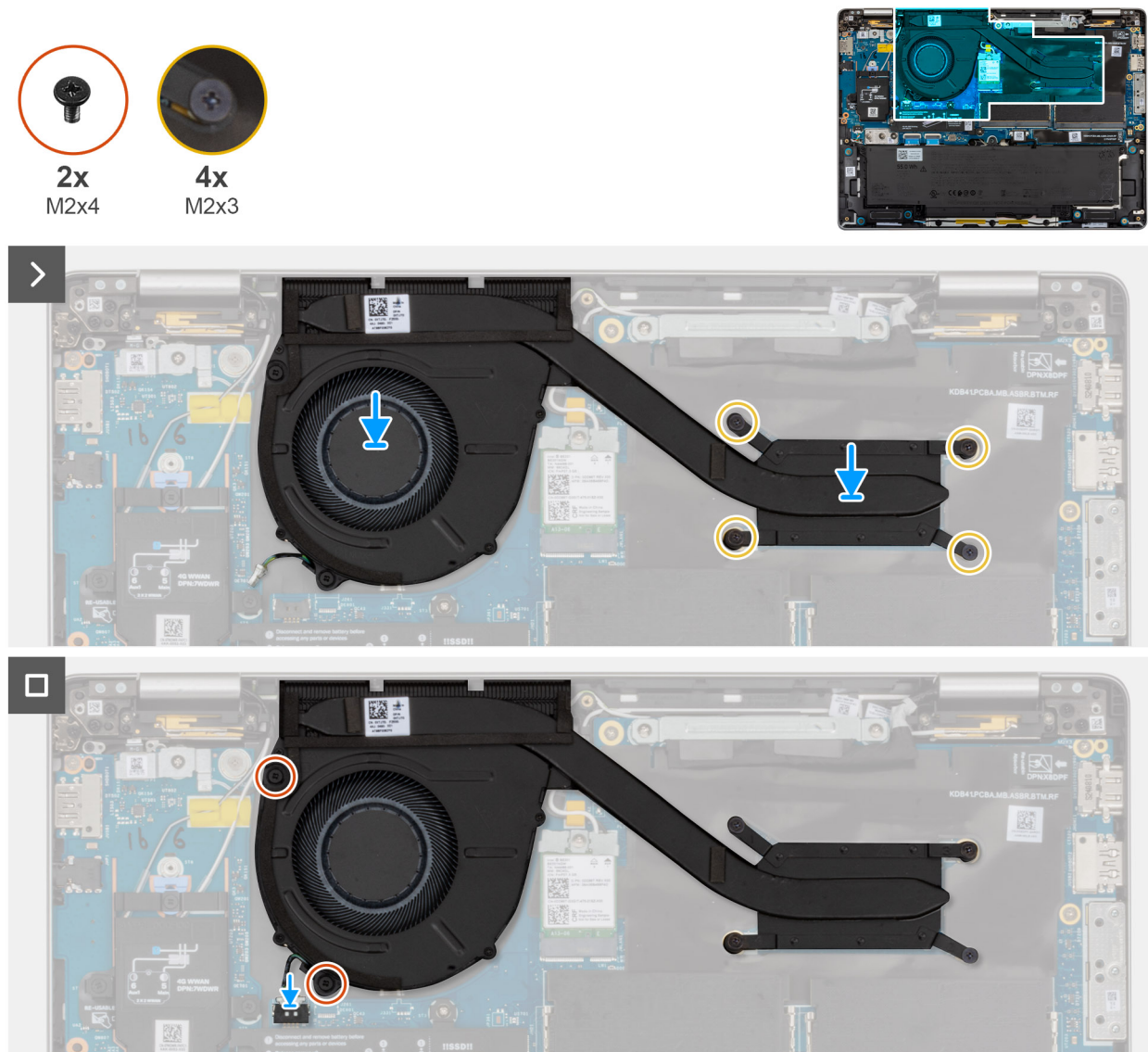
Abbildung 45. Installieren der Lüfter- und Kühlkörperbaugruppe
