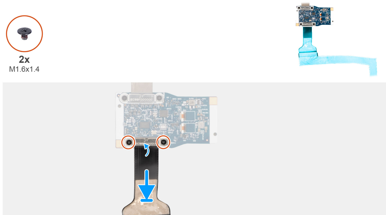
Abbildung 91. Einbauen des Bildschirmkabels für die MIPI-Kamera
