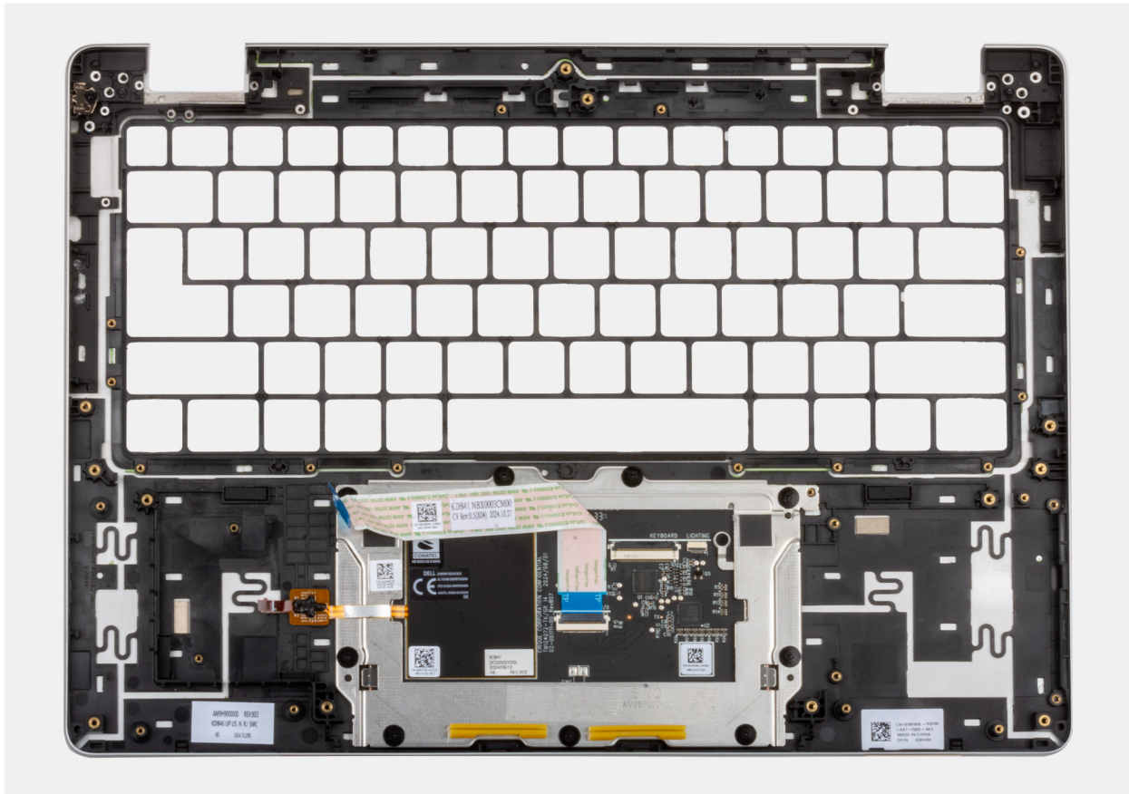
Abbildung 103. Handauflagenbaugruppe
