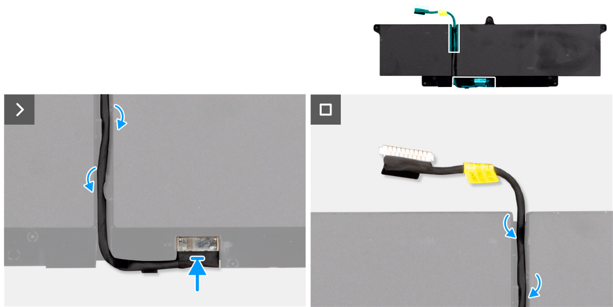
Abbildung 31. Einsetzen des Akkukabels
