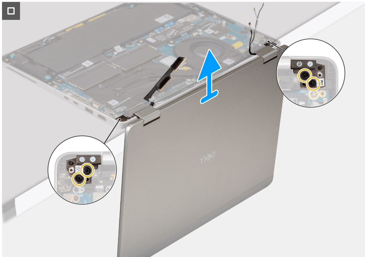
Abbildung 65. Entfernen der Bildschirmbaugruppe
