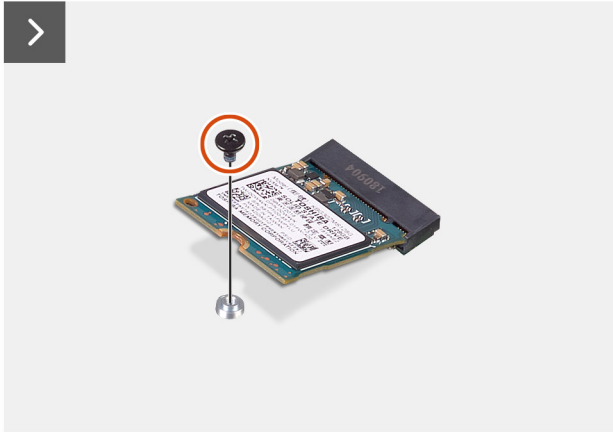
Figure 23. Retrait de la carte SSD
