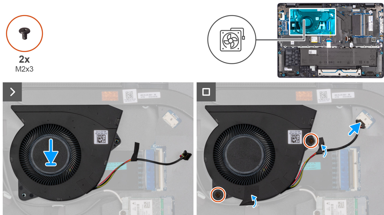
Figure 31. Installation du ventilateur
