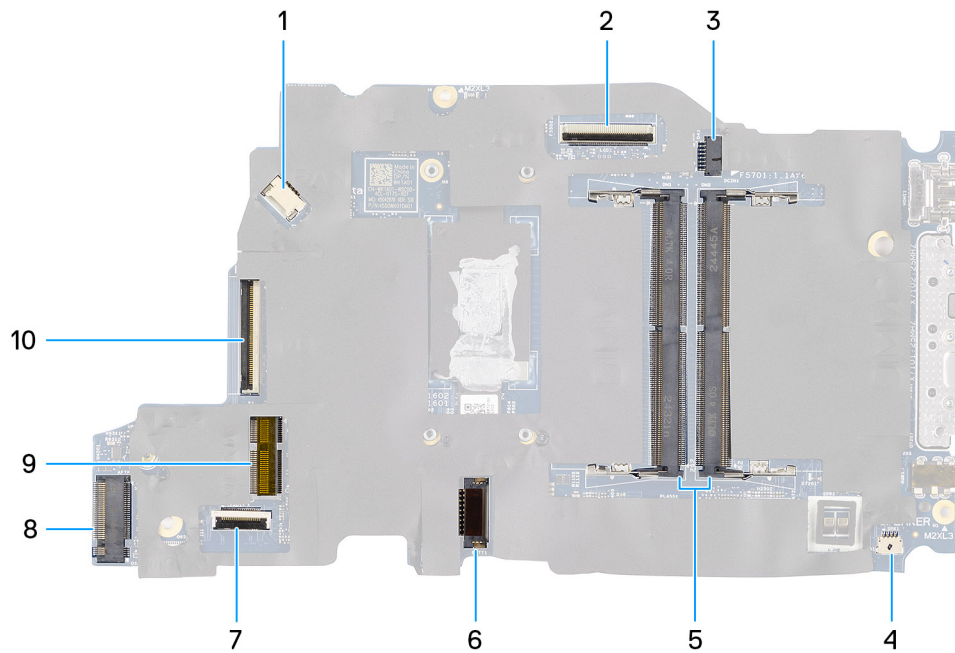
Figure 42. Connecteurs de la carte système
