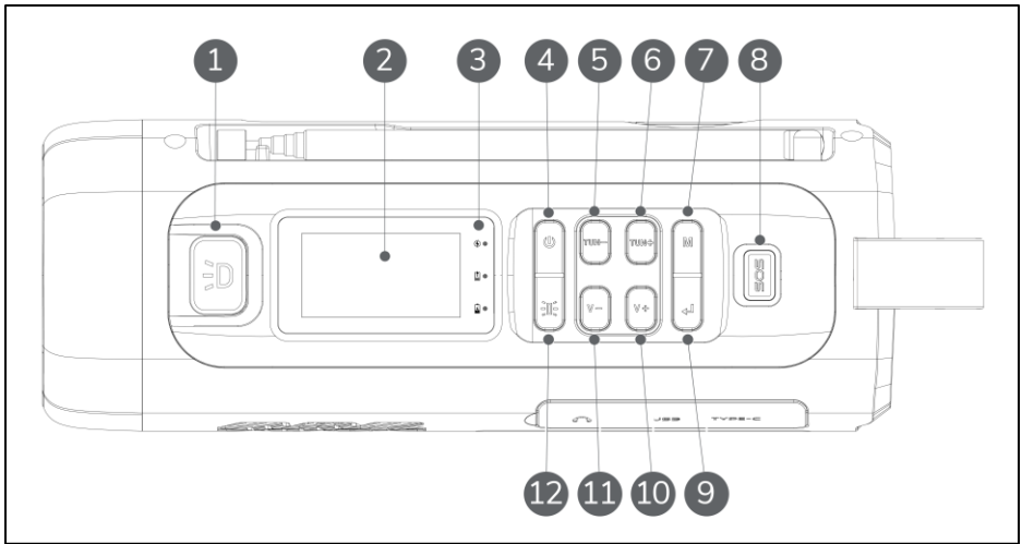
Figuur 6: Bovenaanzicht
