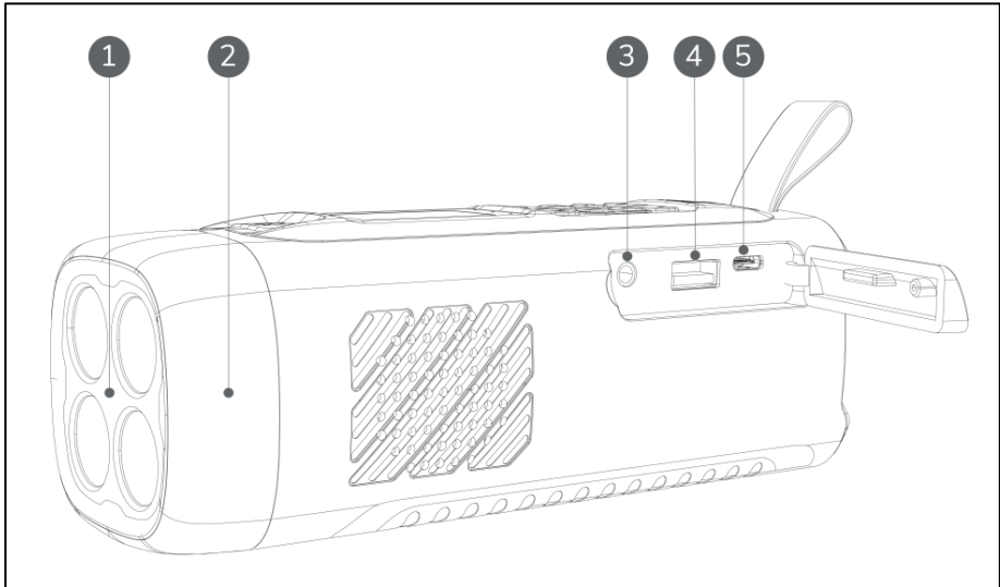
Figura 13: Vista frontal
