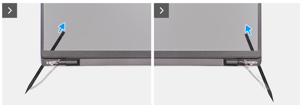
Obrázek 61. Demontáž čelního krytu displeje
