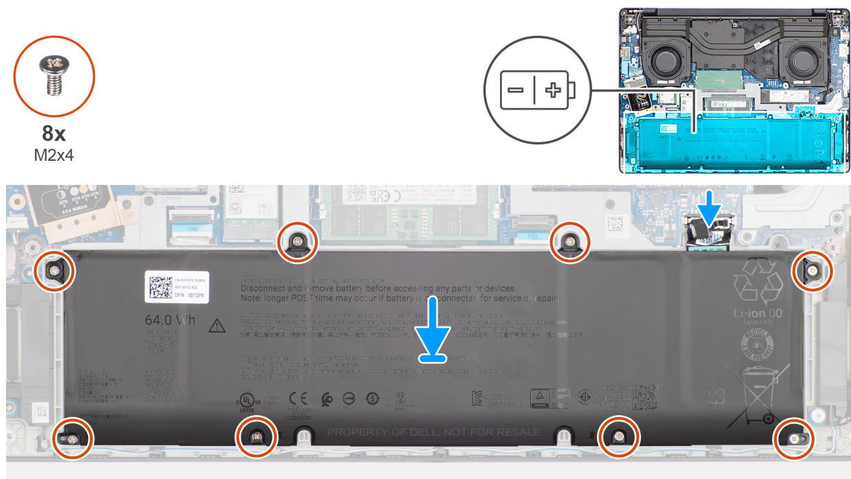
Obrázek 18. Vložení baterie
