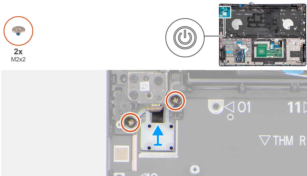
Obrázek 96. Demontáž vypínače
