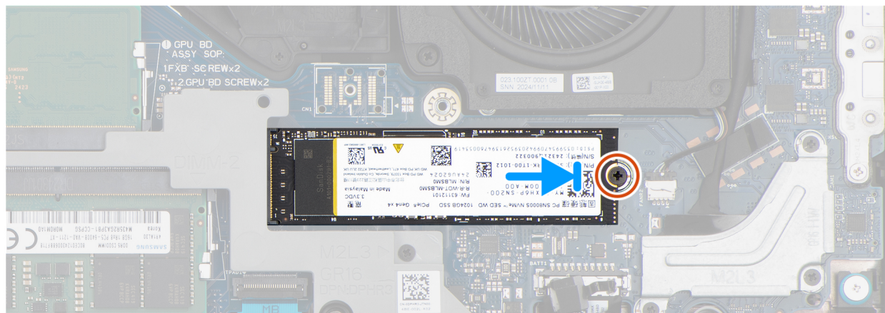
Obrázek 26. Instalace disku SSD M.2 2280
