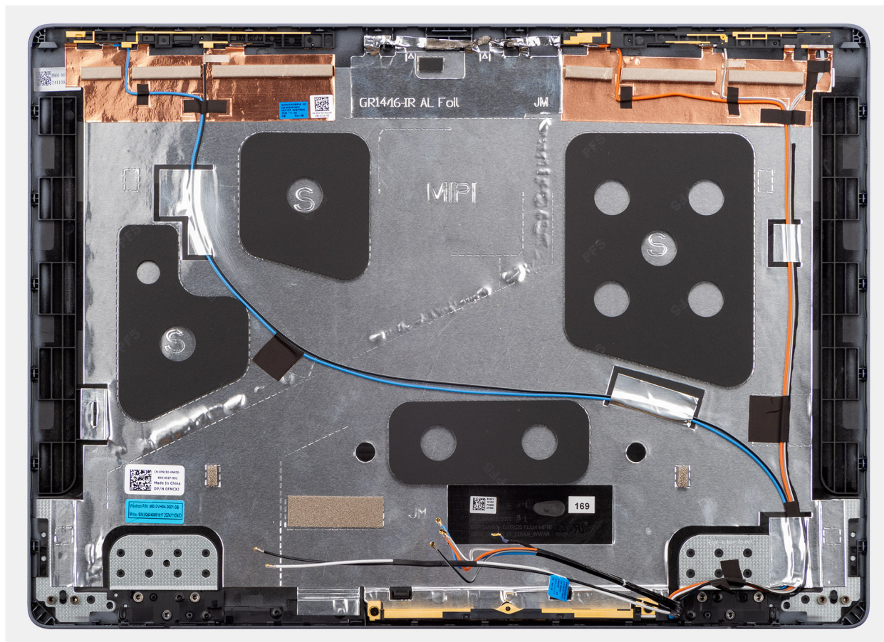
Obrázek 81. Zadní kryt displeje a sestava antény
