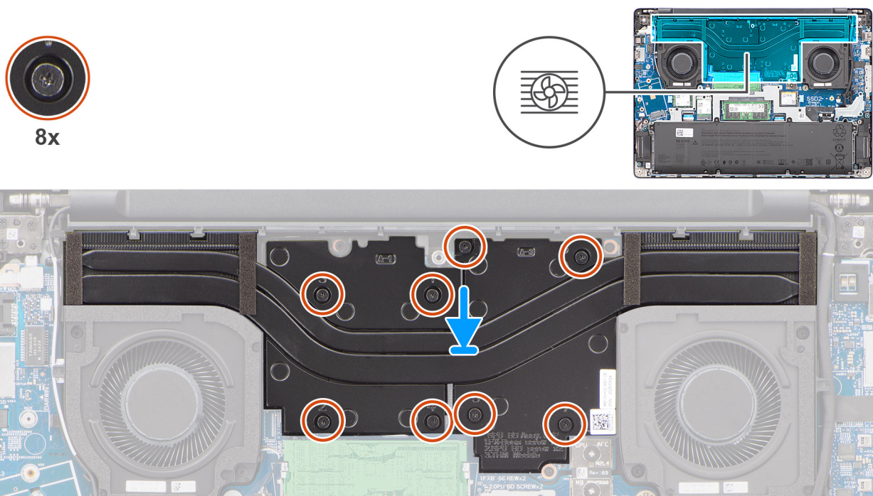
Obrázek 43. Montáž chladiče
