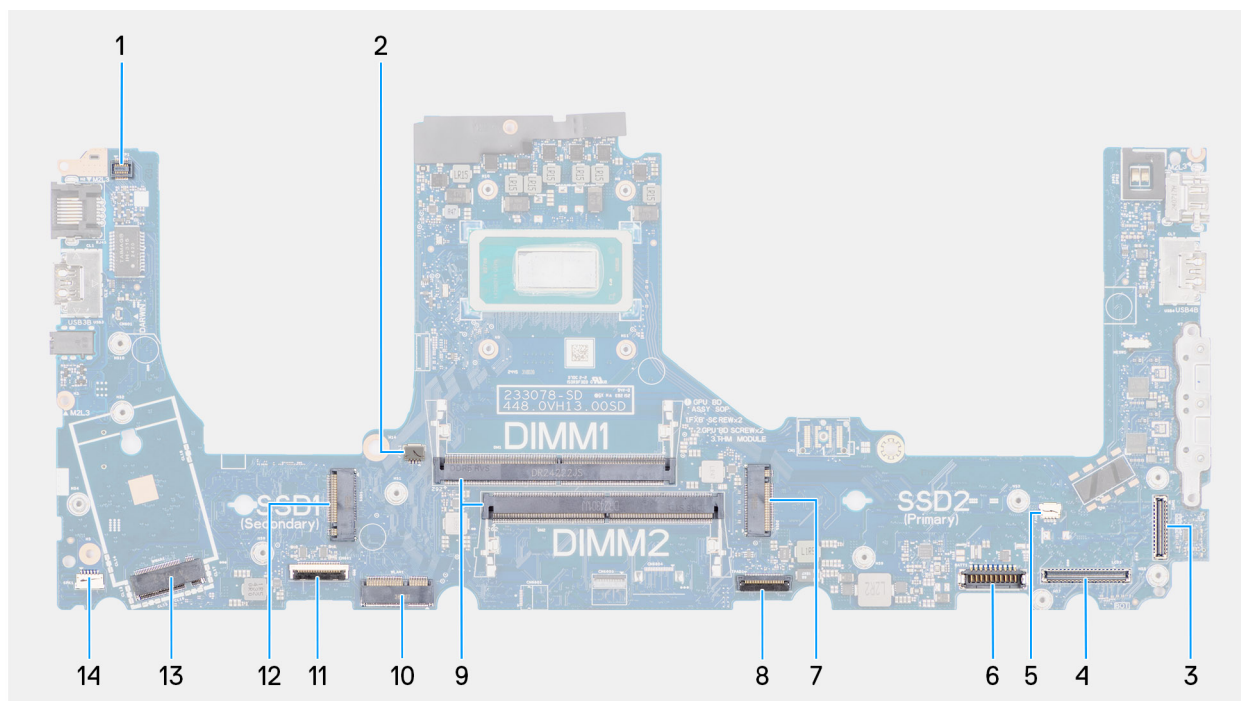
Obrázek 82. Konektory základní desky
