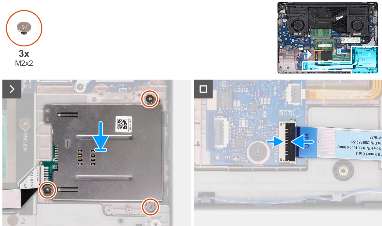
Obrázek 53. Montáž čtečky čipových karet
