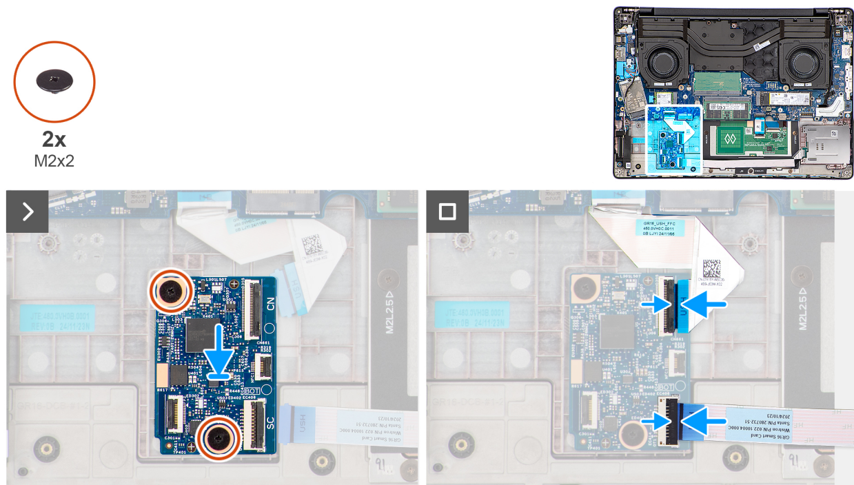
Obrázek 51. Montáž desky USH
