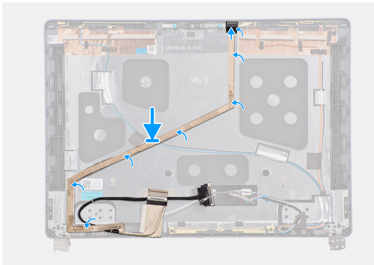
Obrázek 77. Vložení kabelu displeje
