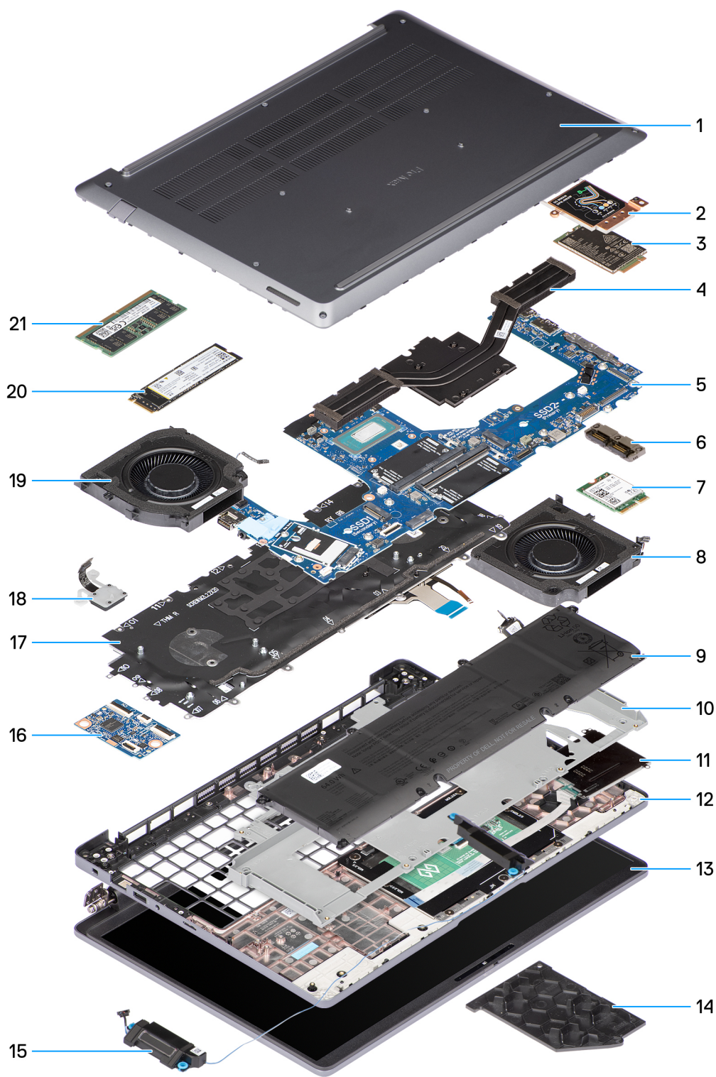
Obrázek 11. Hlavní komponenty počítače Dell Pro Max 16 MC16250
