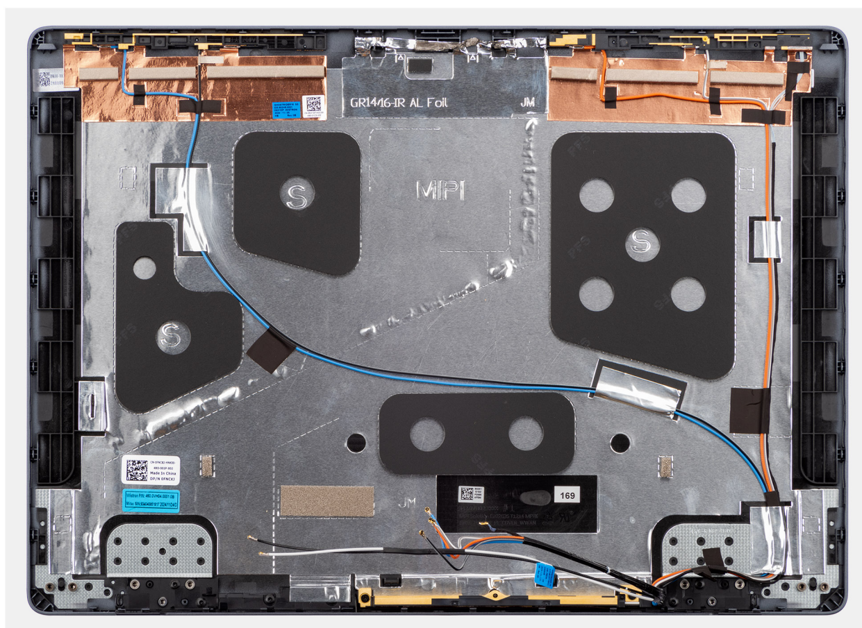
Obrázek 80. Zadní kryt displeje a sestava antény
