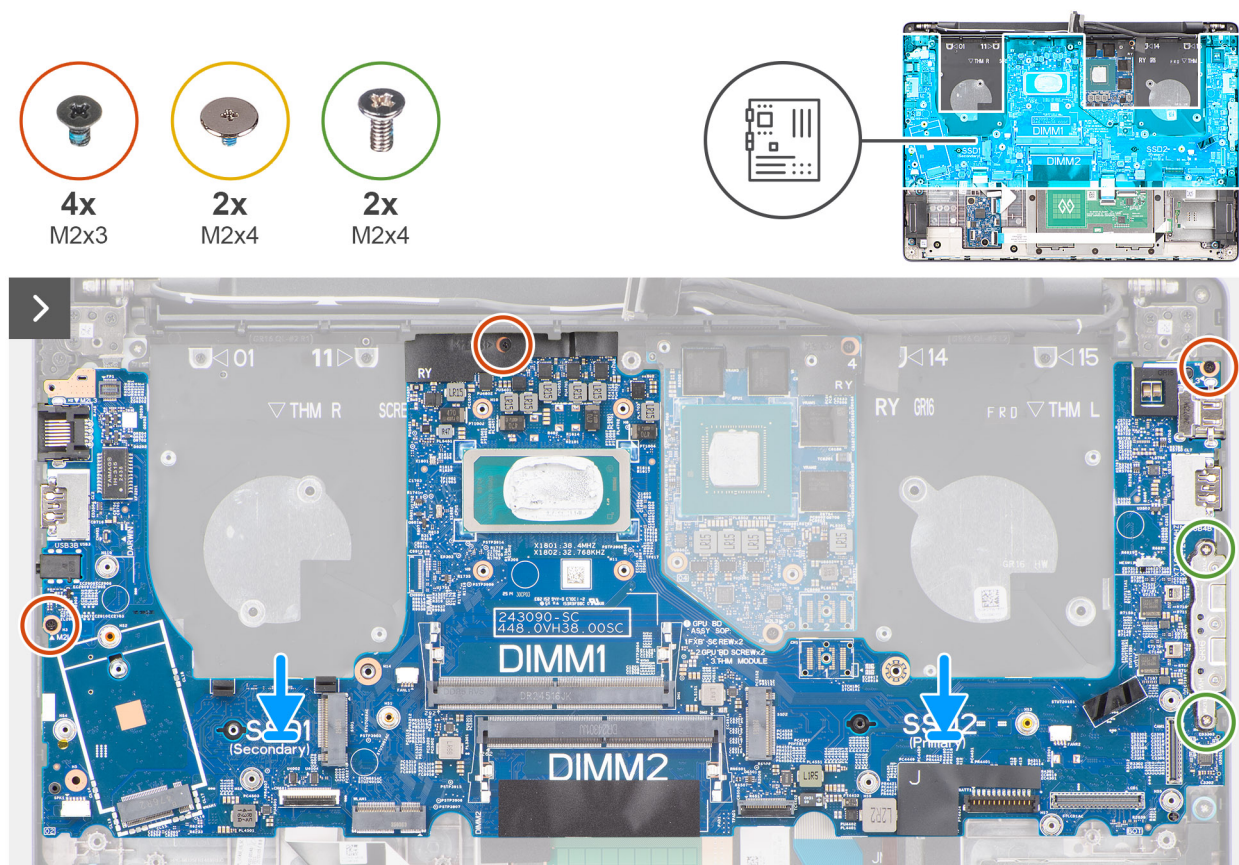
Obrázek 92. Montáž základní desky
