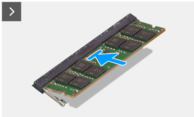
Obrázek 22. Vložení paměťového modulu
