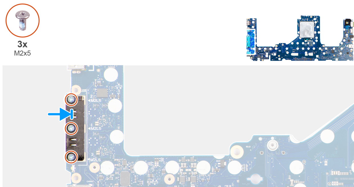
Obrázek 95. Montáž modulu USB Type-C
