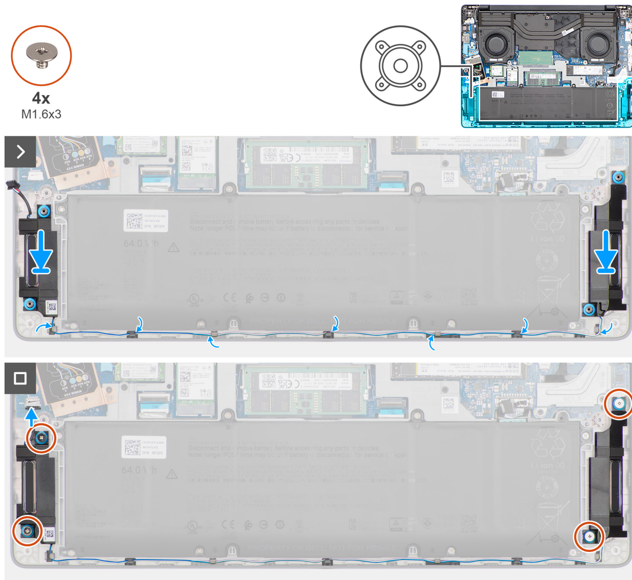
Obrázek 34. Montáž reproduktorů
