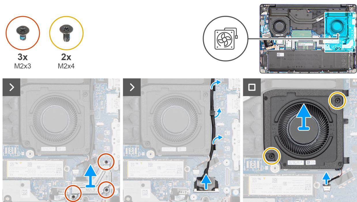
Obrázek 38. Demontáž levého ventilátoru / ventilátoru grafické karty
