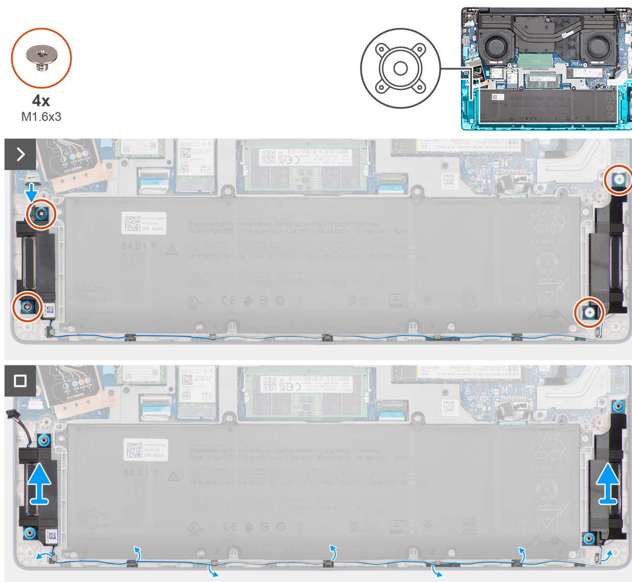
Obrázek 33. Demontáž reproduktorů
