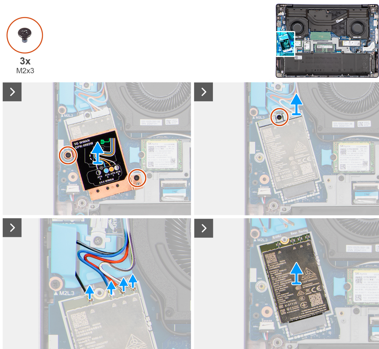
Obrázek 29. Demontáž modulu WWAN
