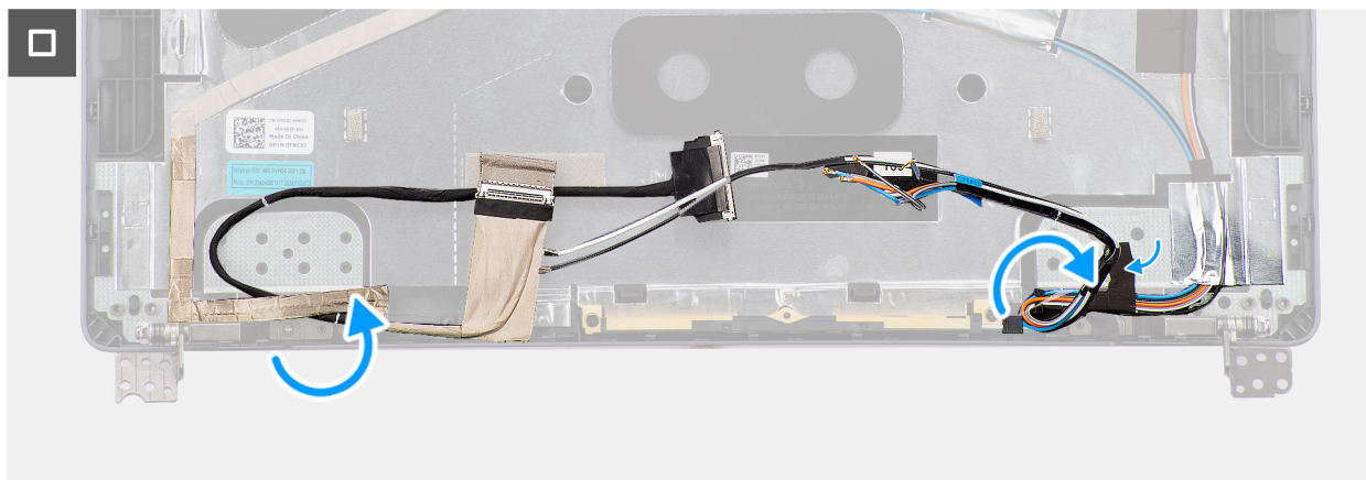
Obrázek 75. Montáž pantů displeje
