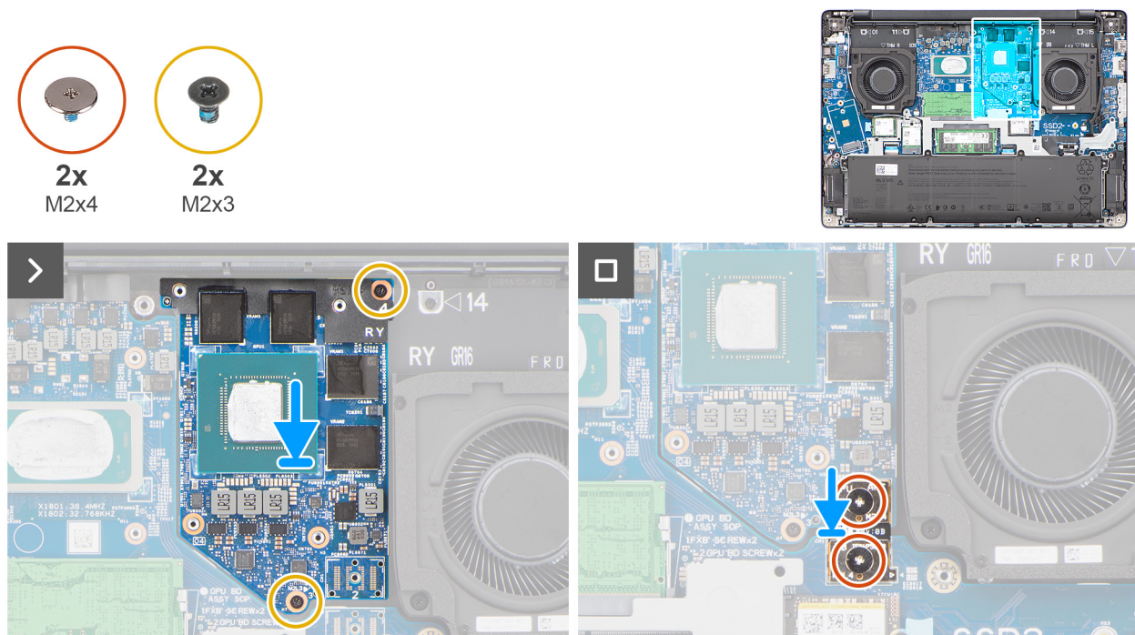
Obrázek 47. Montáž disku GPU
