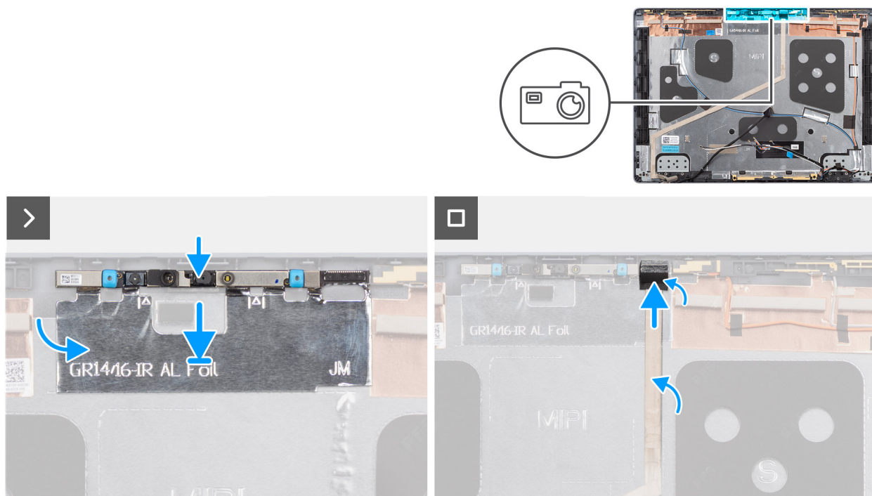
Obrázek 79. Montáž kamery
