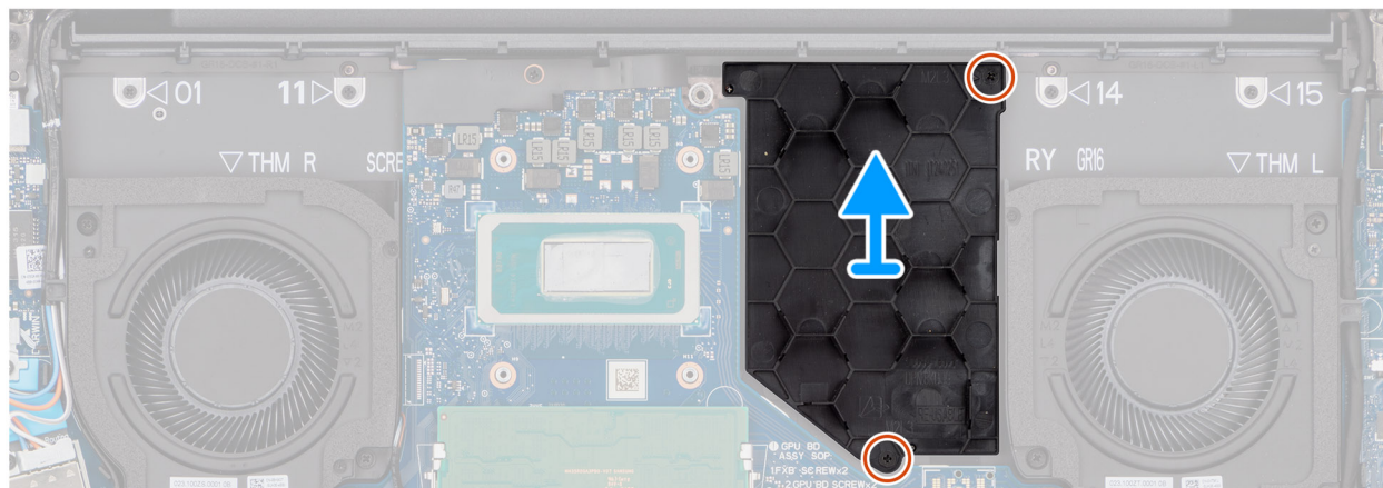
Obrázek 44. Demontáž výplně grafické karty
