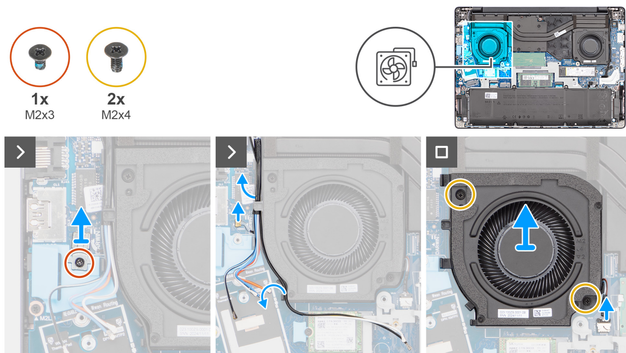
Obrázek 36. Demontáž pravého ventilátoru / ventilátoru procesoru
