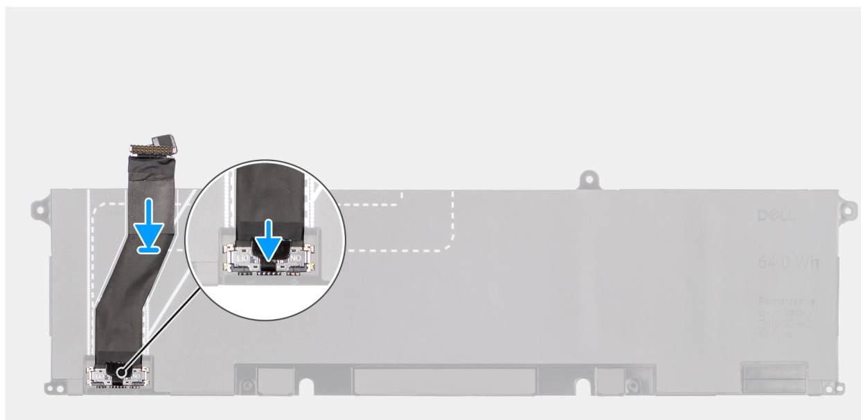
Obrázek 20. Připojení kabelu baterie
