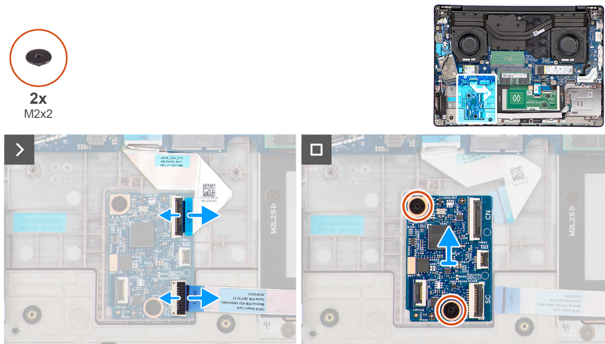
Obrázek 50. Demontáž desky USH
