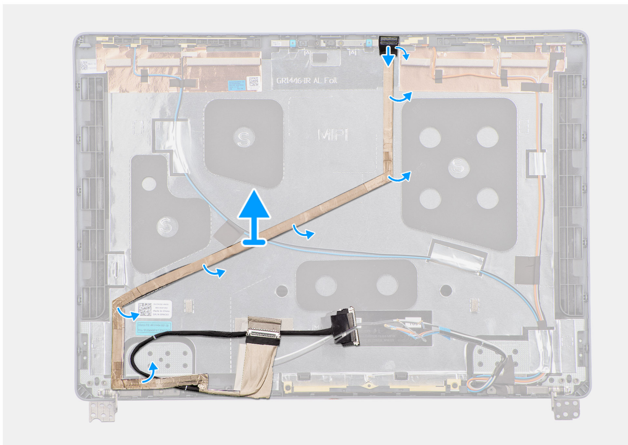
Obrázek 76. Vyjmutí kabelu displeje
