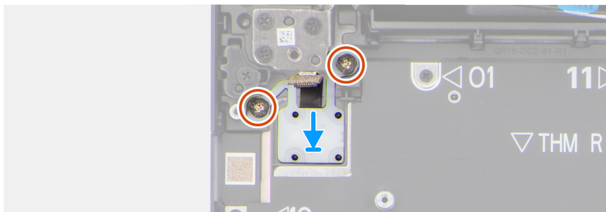
Obrázek 97. Montáž vypínače
