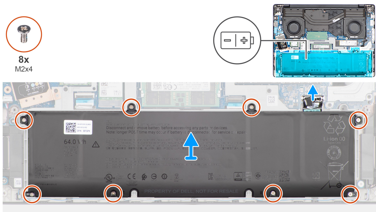
Obrázek 17. Vyjmutí baterie
