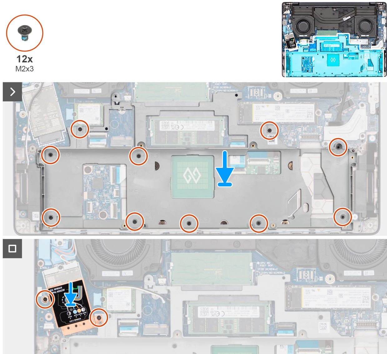
Obrázek 49. Montáž rámu baterie
