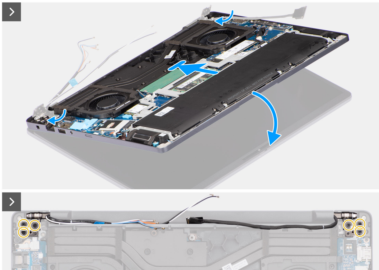
Obrázek 58. Montáž sestavy displeje
