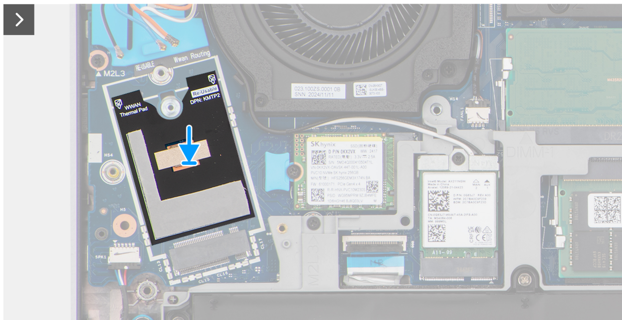
Obrázek 31. Montáž modulu WWAN
