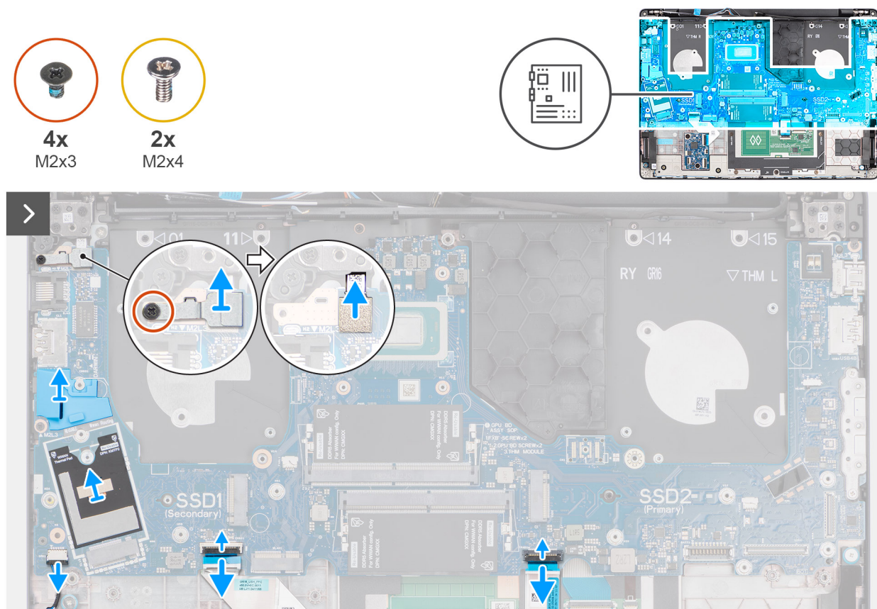
Obrázek 83. Demontáž základní desky
