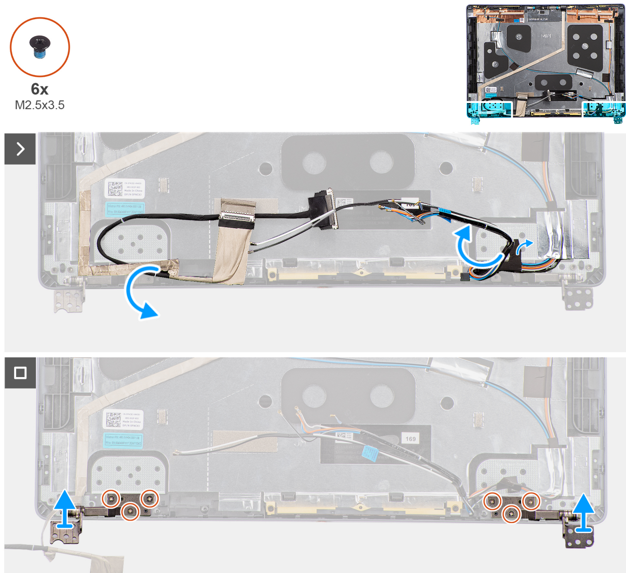
Obrázek 74. Demontáž pantů displeje
