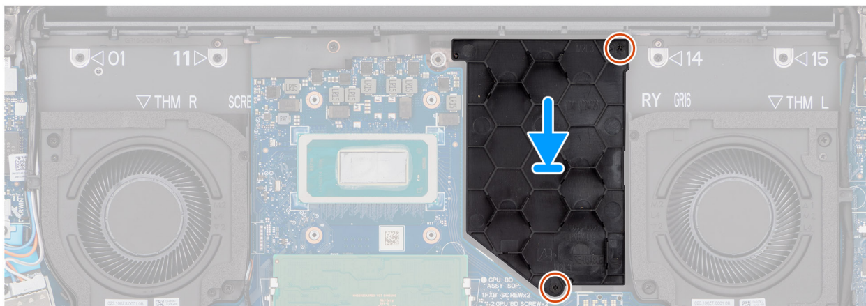
Obrázek 45. Montáž výplně grafické karty
