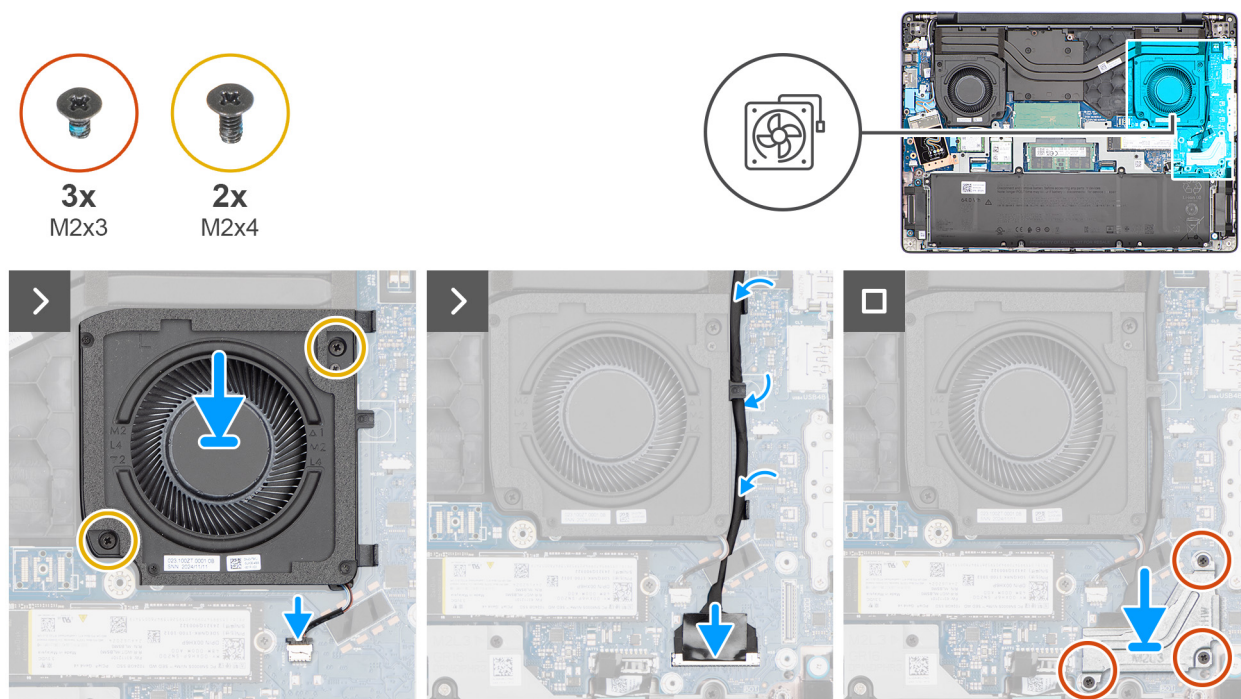
Obrázek 39. Montáž levého ventilátoru / ventilátoru grafické karty
