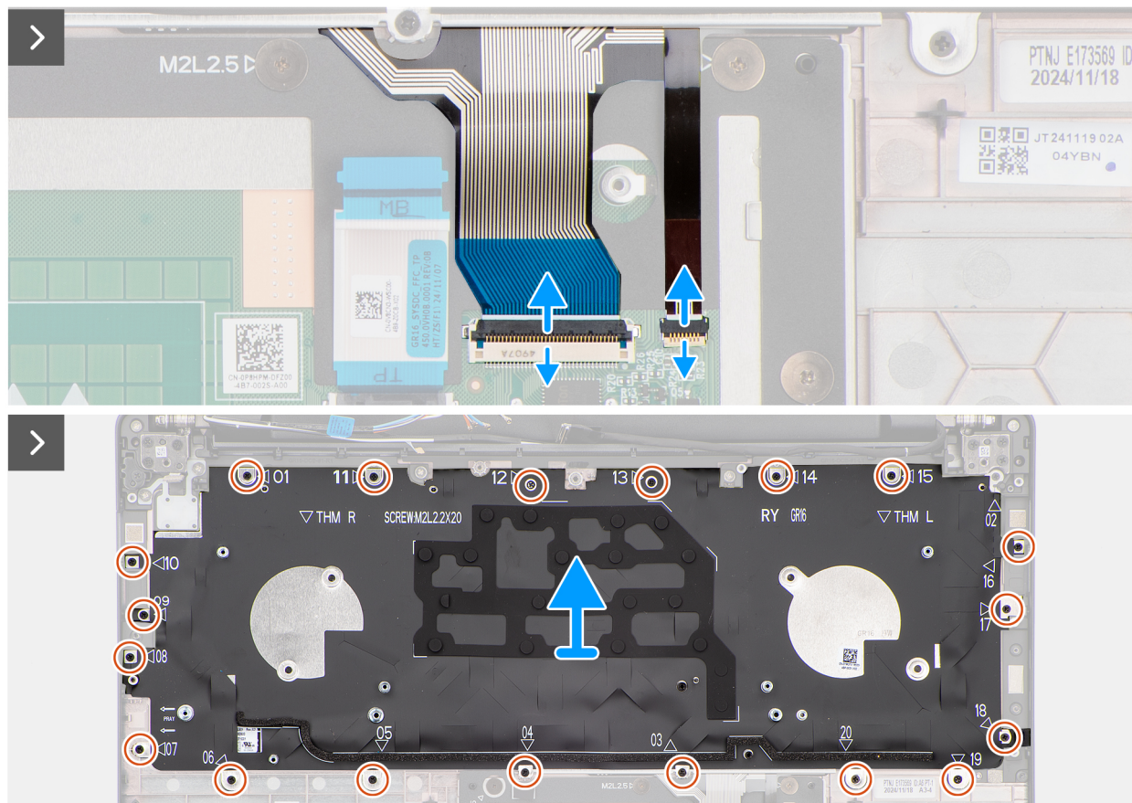
Obrázek 98. Demontáž klávesnice
