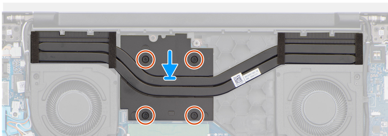
Obrázek 41. Montáž chladiče
