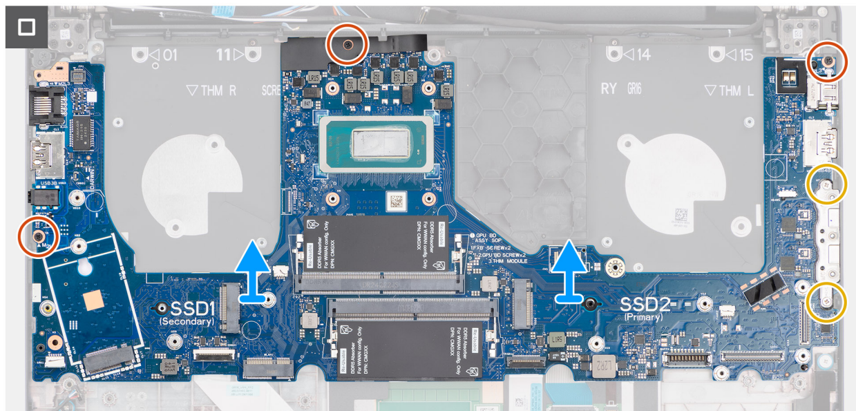
Obrázek 84. Demontáž základní desky
