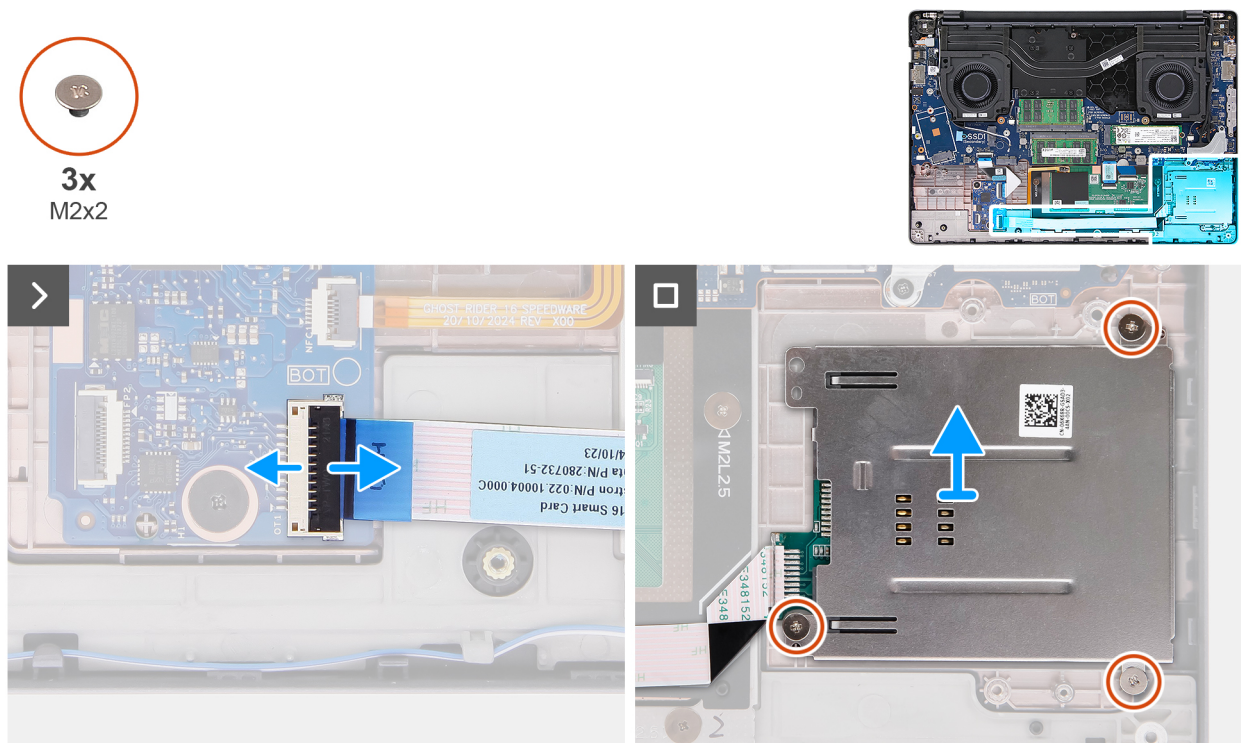
Obrázek 52. Demontáž čtečky čipových karet
