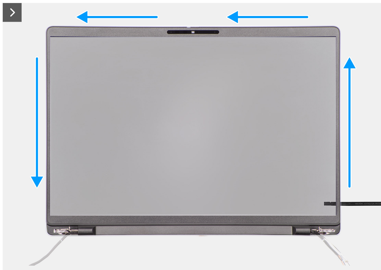
Obrázek 62. Demontáž čelního krytu displeje
