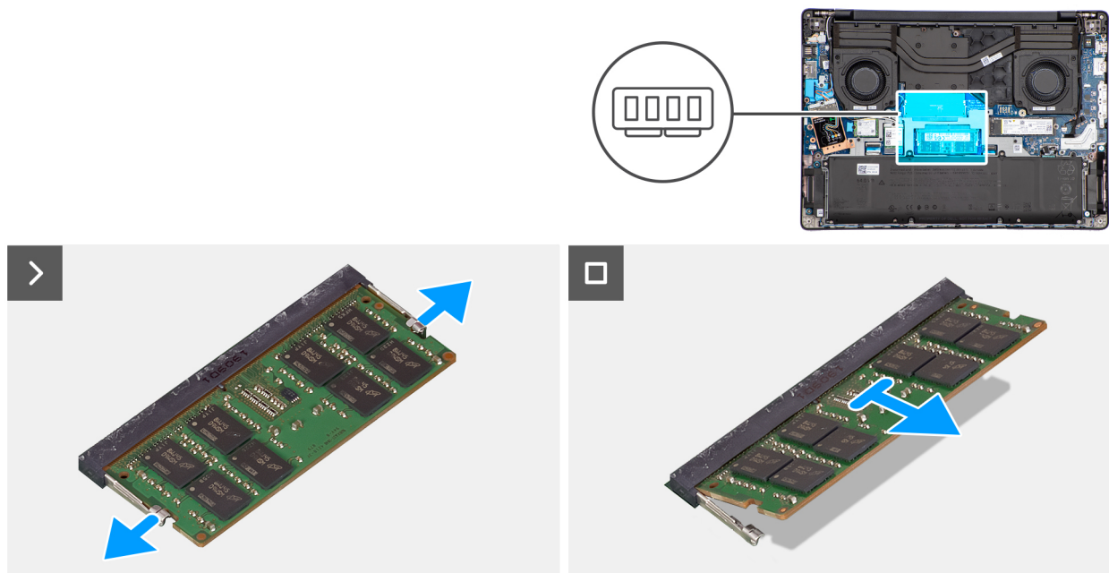
Obrázek 21. Vyjmutí paměťového modulu
