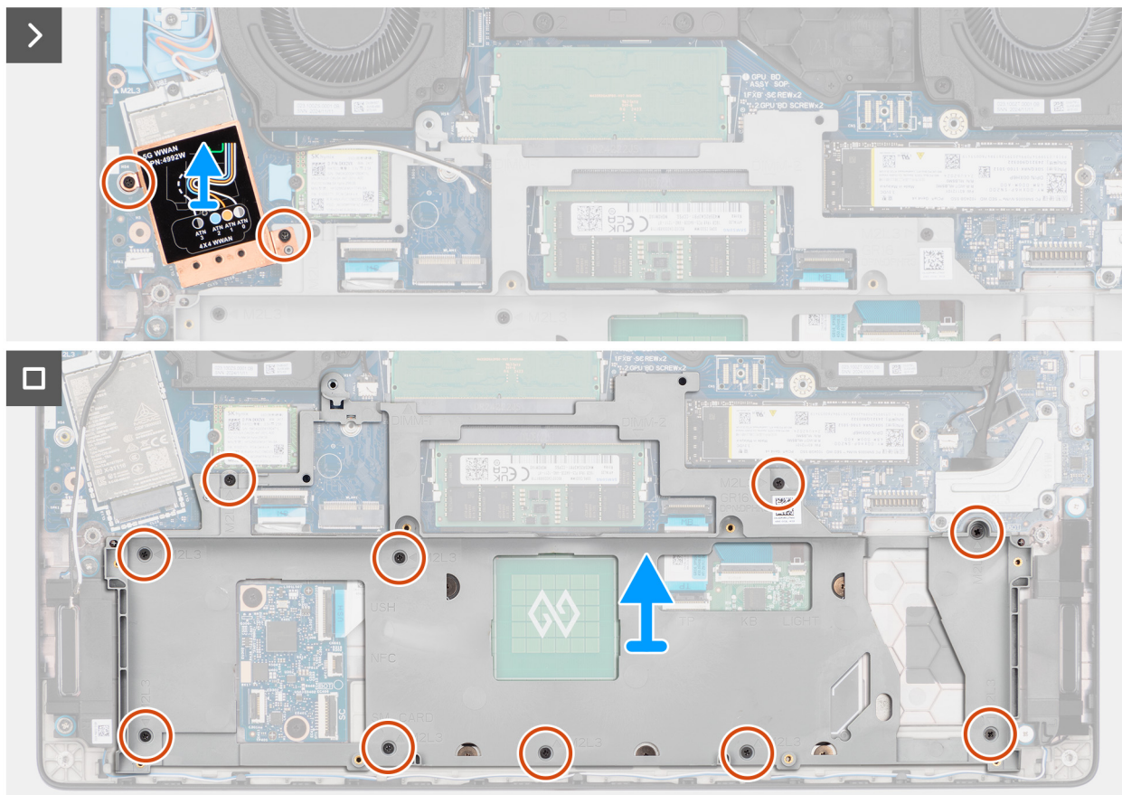
Obrázek 48. Demontáž rámu baterie
