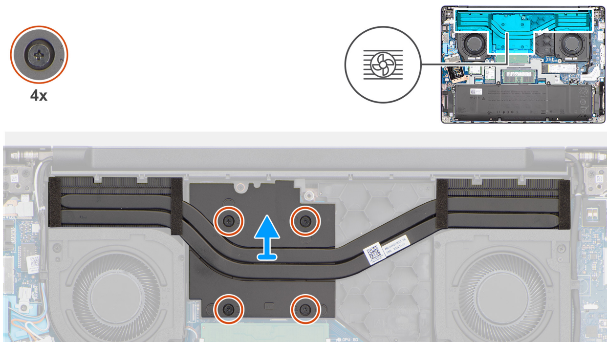
Obrázek 40. Demontáž chladiče
