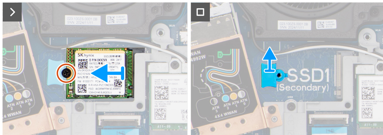
Obrázek 23. Demontáž disku SSD M.2 2230
