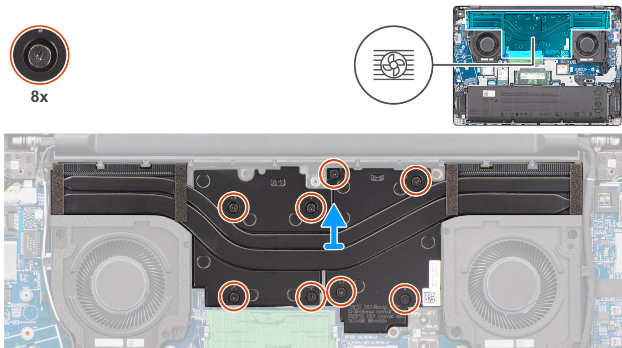
Obrázek 42. Demontáž chladiče
