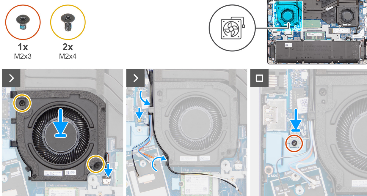
Obrázek 37. Montáž pravého ventilátoru / ventilátoru procesoru
