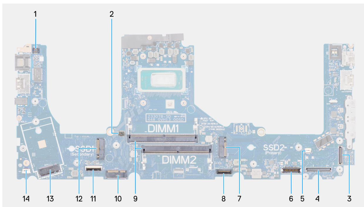
Obrázek 88. Konektory základní desky
