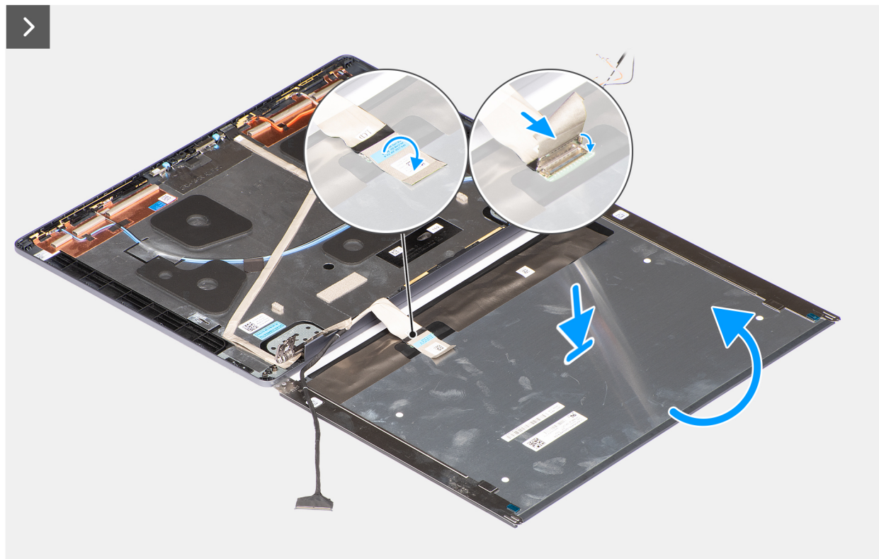
Obrázek 72. Montáž obrazovky displeje
