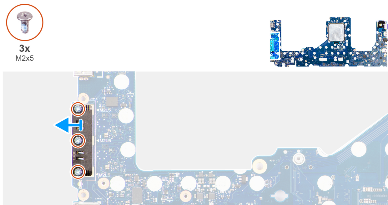
Obrázek 94. Demontáž modulu USB Type-C
