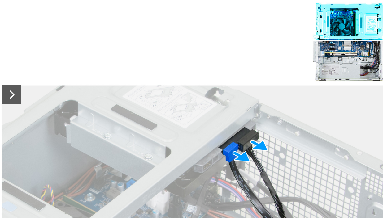
Ilustración 28. Extracción de la bahía de unidad
