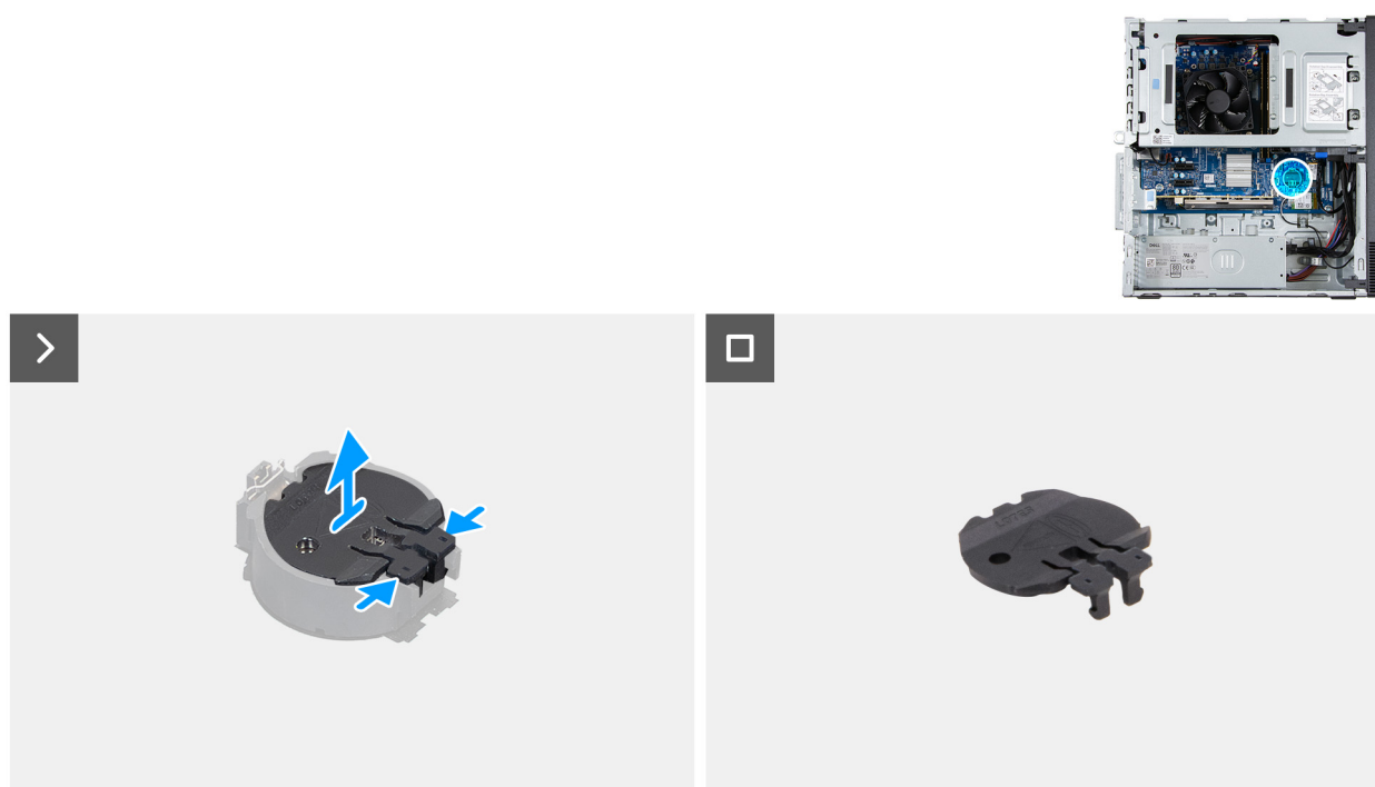
Ilustración 14. Extracción de la cubierta de la batería de tipo botón
