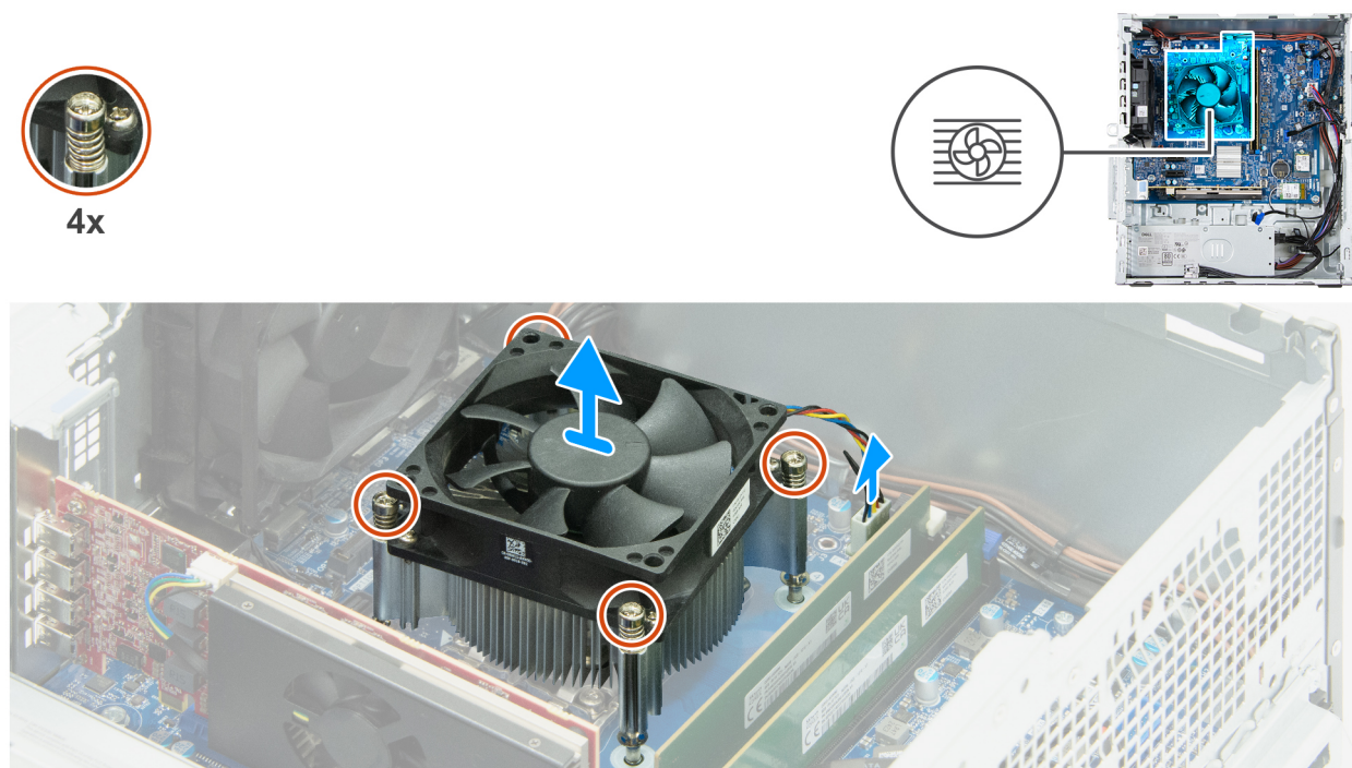
Ilustración 50. Extracción del ensamblaje del disipador de calor y el ventilador del procesador
