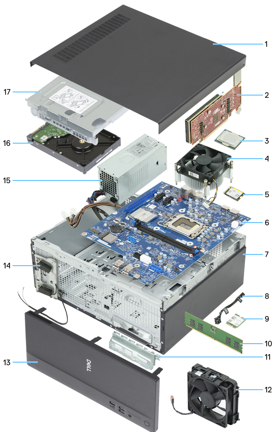
Ilustración 9. Componentes principales de Torre Dell Pro Essential QVT1260
