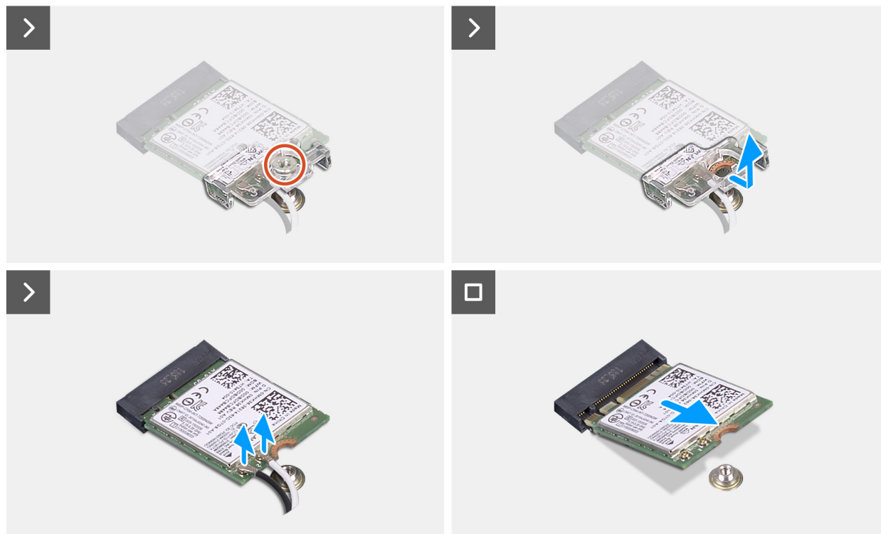
Ilustración 26. Extracción de la tarjeta inalámbrica
