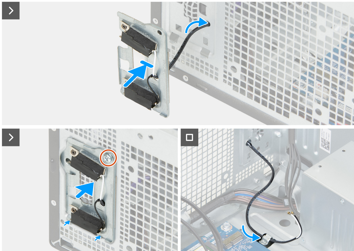
Ilustración 45. Instalación de los módulos de la antena
