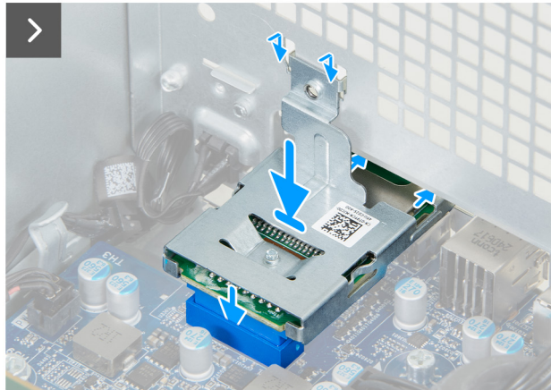
Ilustración 38. Instalación del lector de tarjetas de medios
