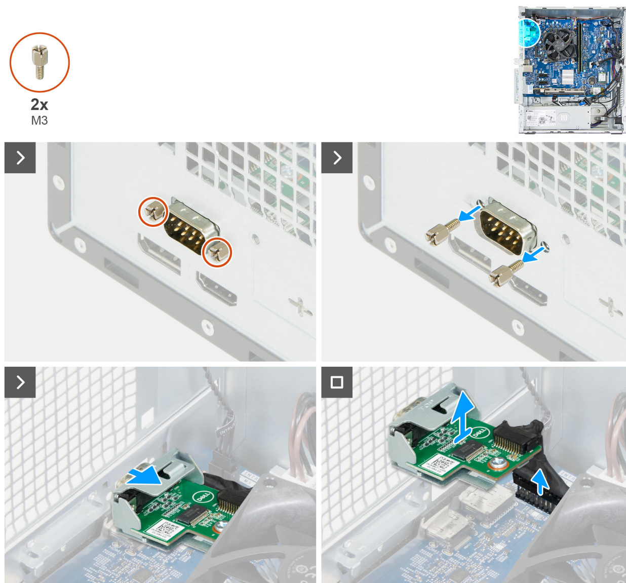
Ilustración 41. Extracción del módulo de puerto serial
