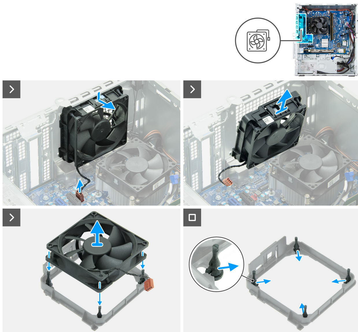
Ilustración 39. Extracción del ventilador
