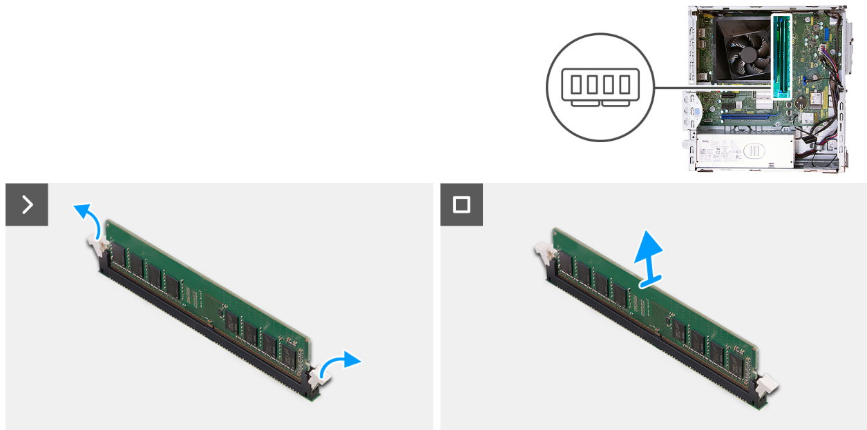
Figure 23. Retrait d'un module de mémoire
