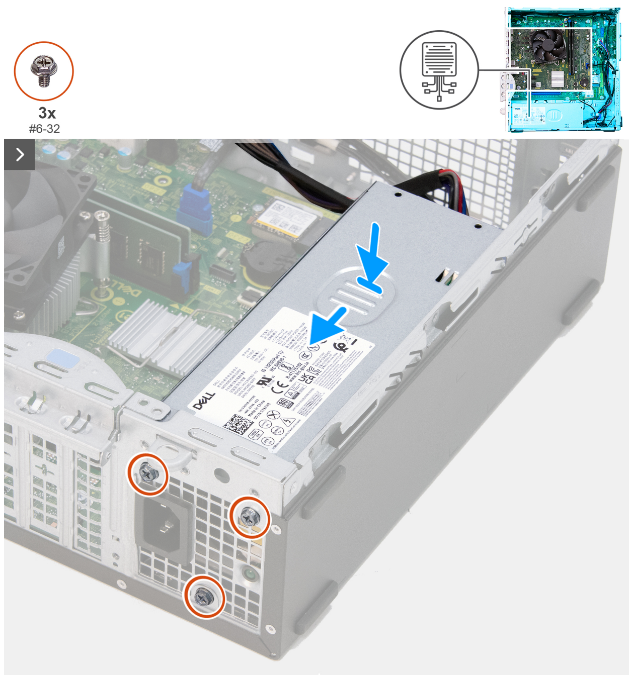
Figure 35. Installation du bloc d'alimentation
