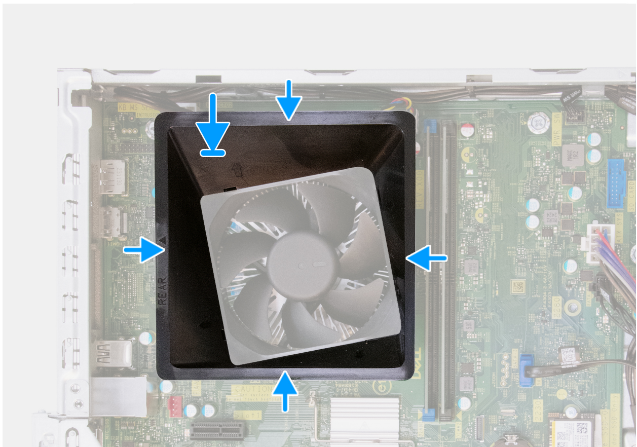
Figure 38. Installation du carénage du ventilateur
