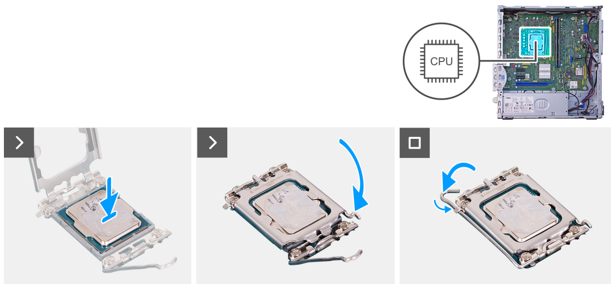
Figure 42. Installation du processeur
