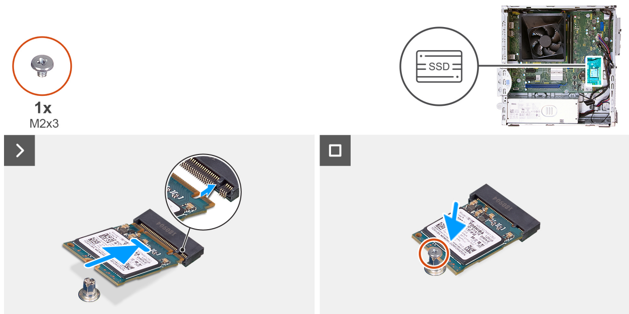
Figure 26. Installation du disque SSD M.2 2230
