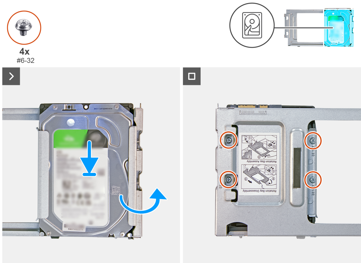
Figure 22. Installation du disque dur
