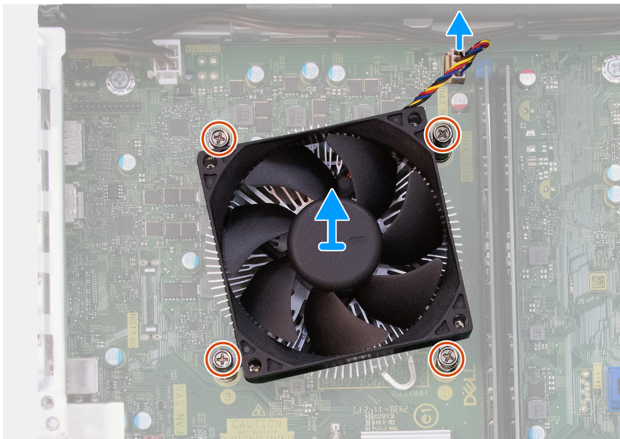
Figure 39. Retrait de l'assemblage de dissipateur de chaleur et ventilateur de processeur
