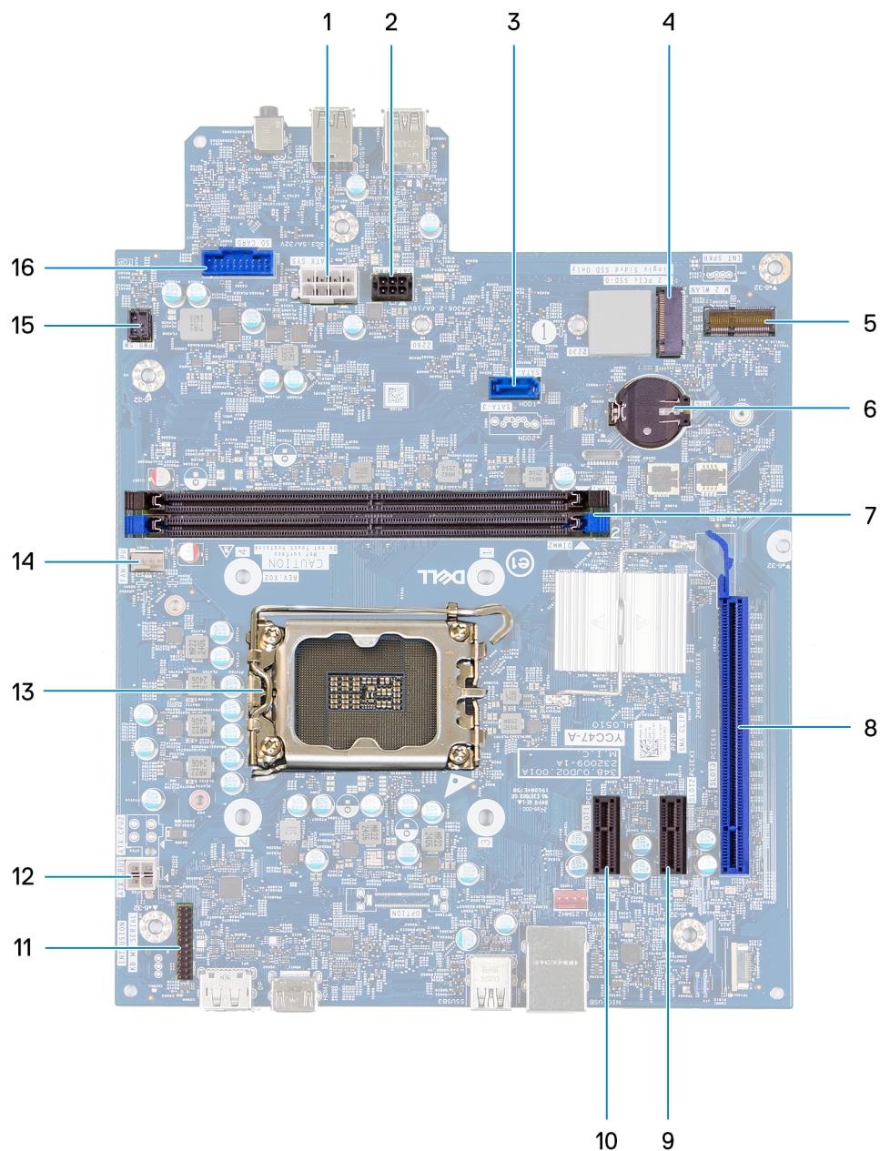
Figure 52. Présentation de la carte système
