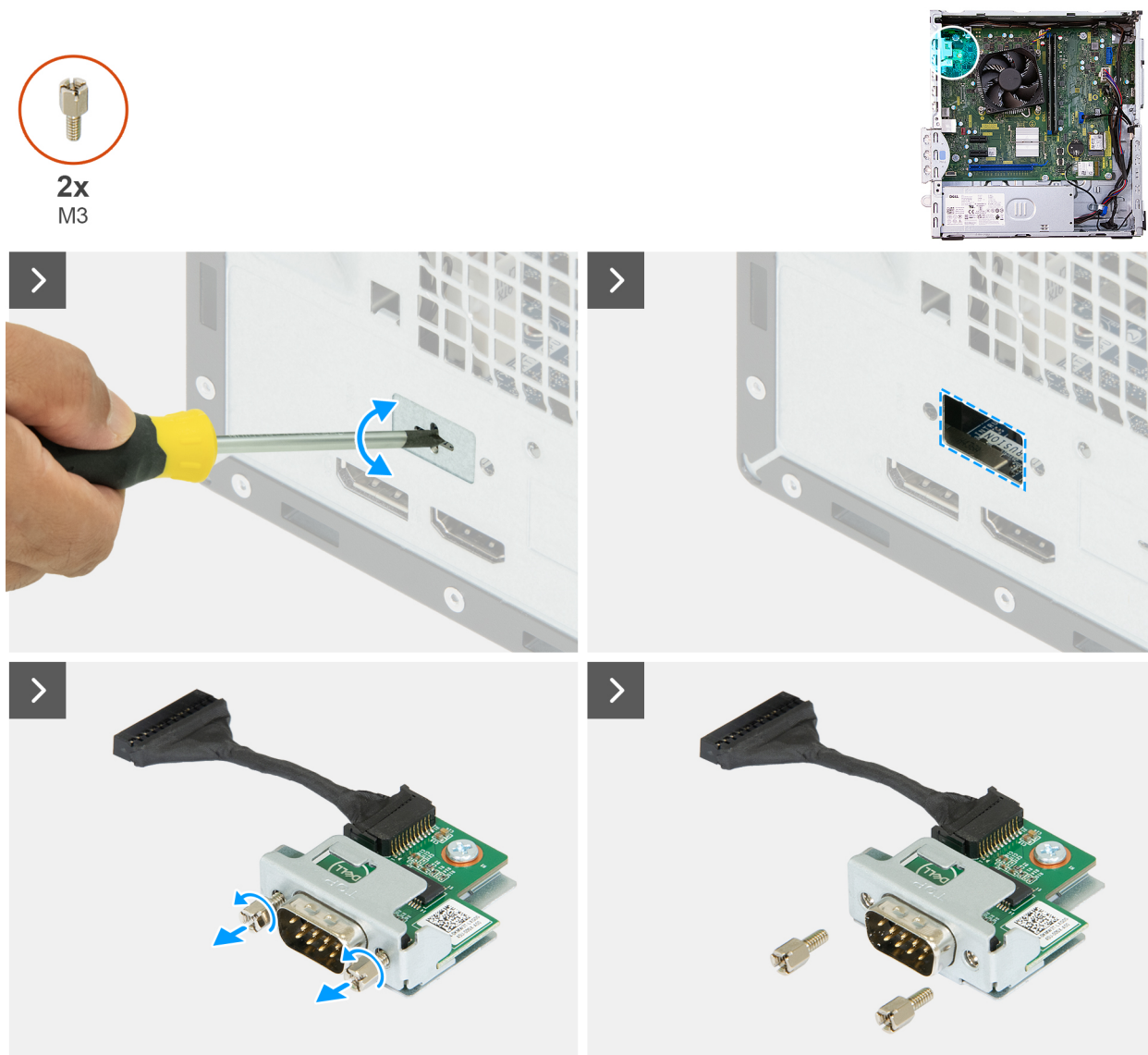
Figure 46. Installation du module de port série
