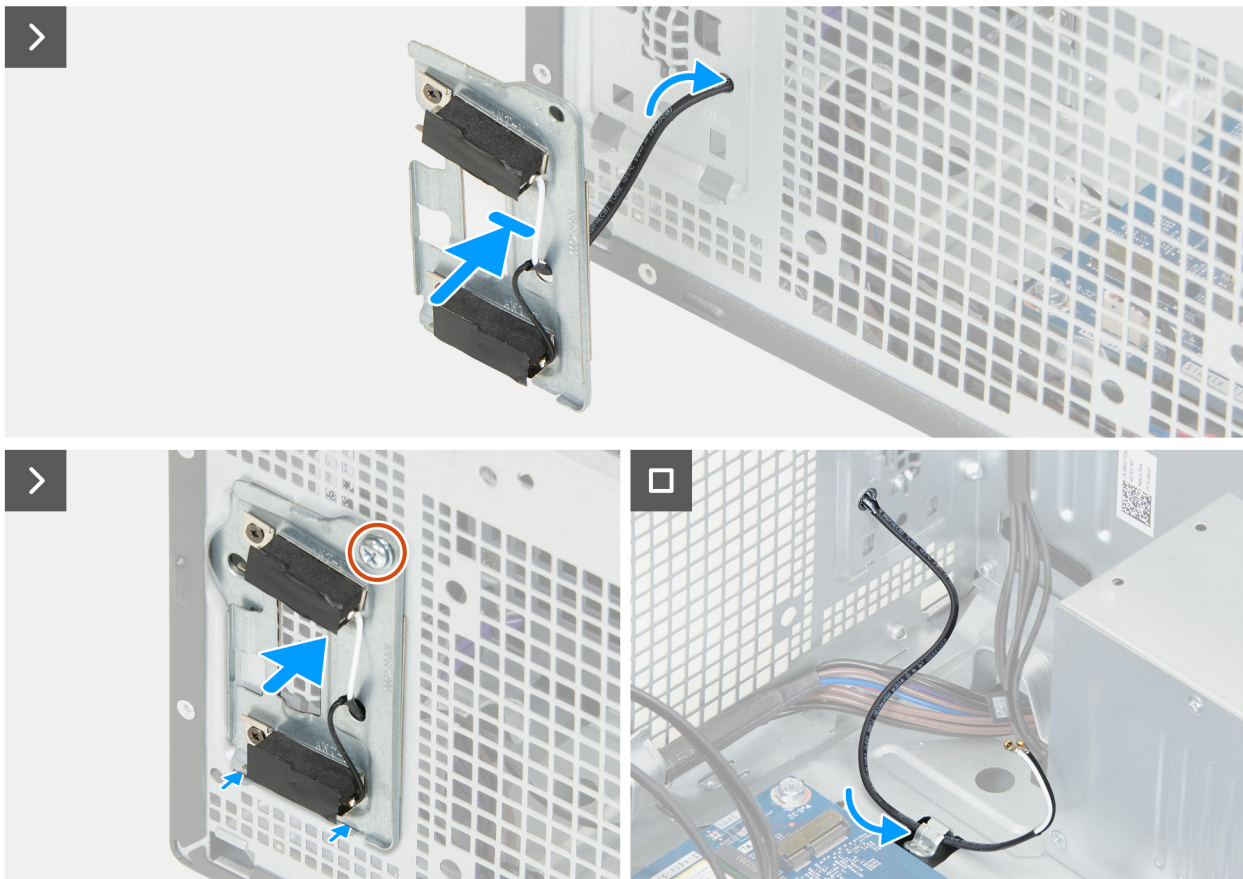
Figure 32. Installation du module d'antenne
