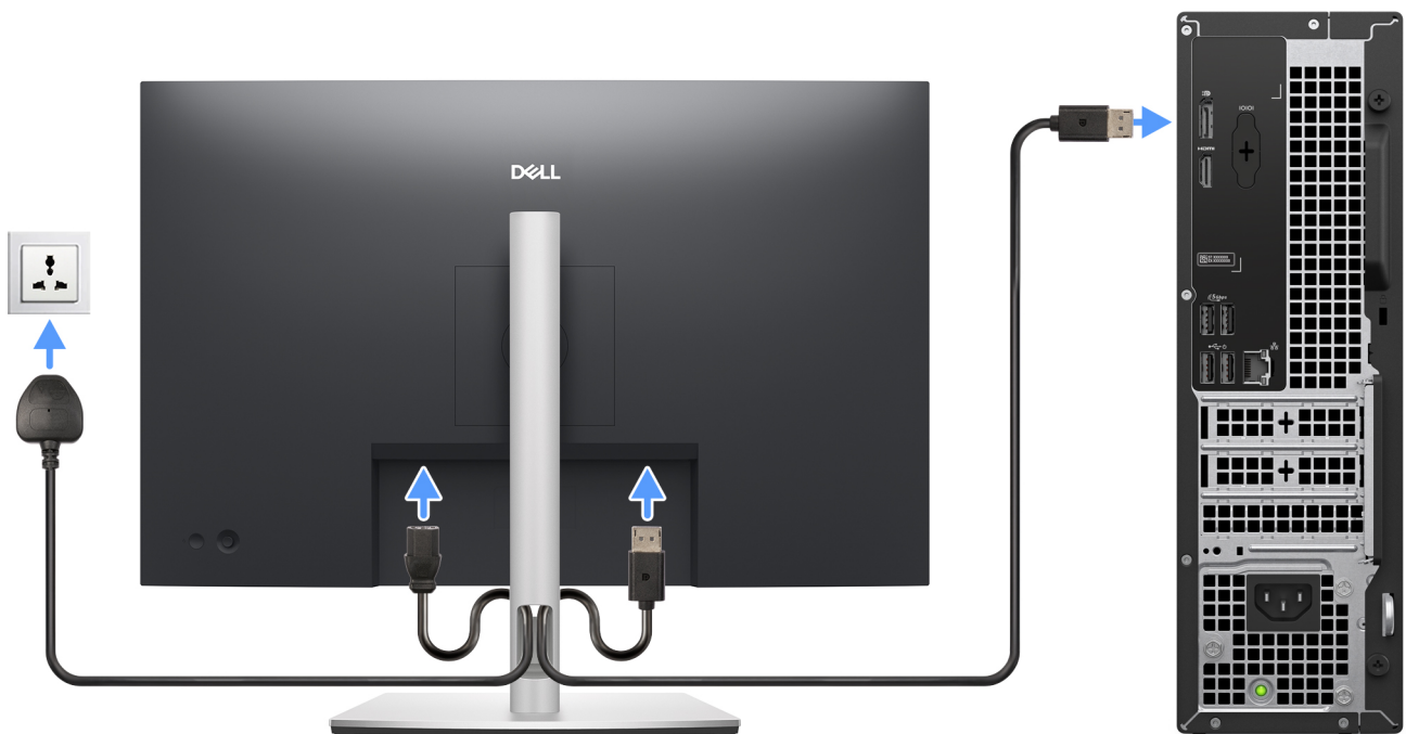
Figure 6. Branchement de l'écran
