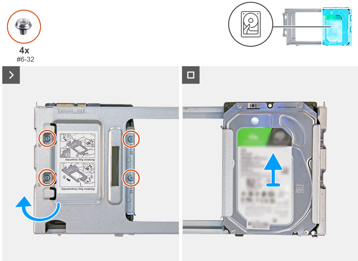
Figure 21. Retrait du disque dur
