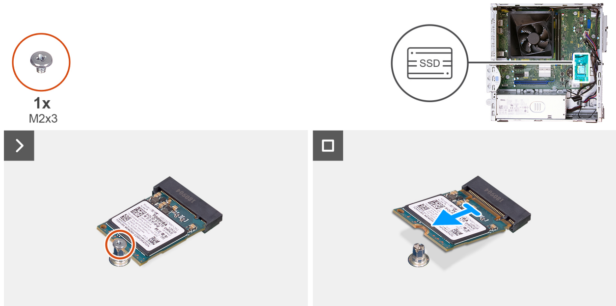
Figure 25. Retrait du disque SSD M.2 2230
