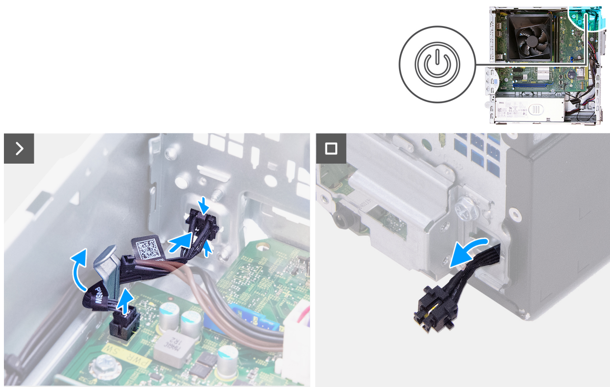
Figure 43. Retrait du bouton d'alimentation
