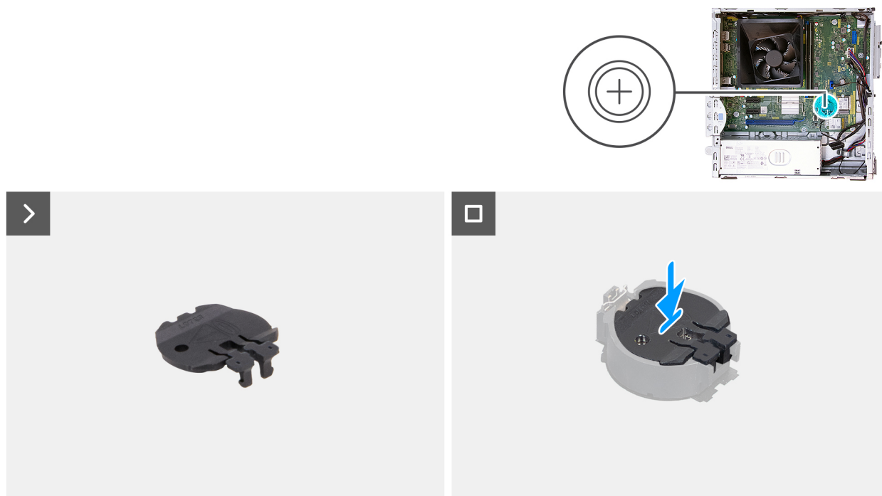
Figure 13. Installation du capot de la pile bouton
