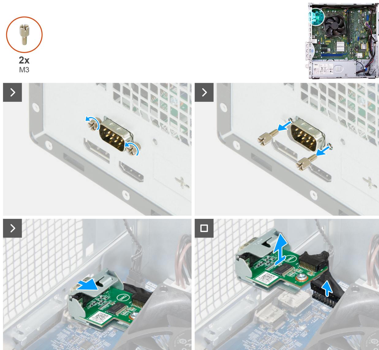
Figure 45. Retrait du module de port série
