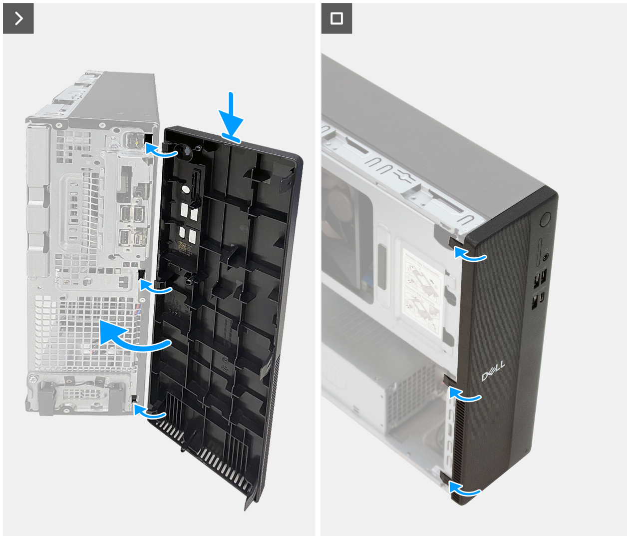
Figure 17. Installation du capot avant
