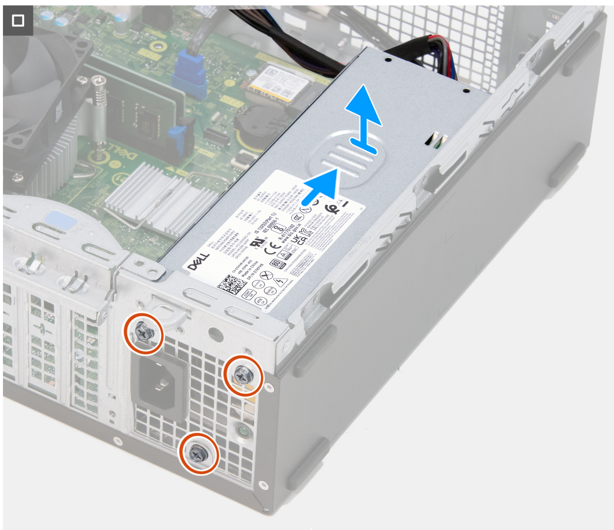
Figure 34. Retrait du bloc d'alimentation
