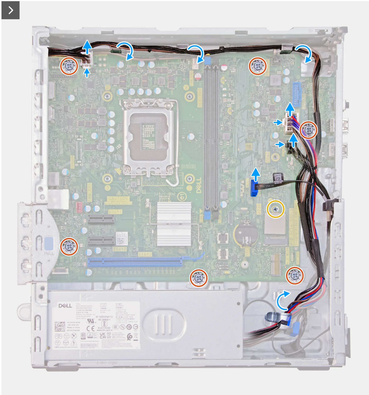
Figure 50. Retrait de la carte système
