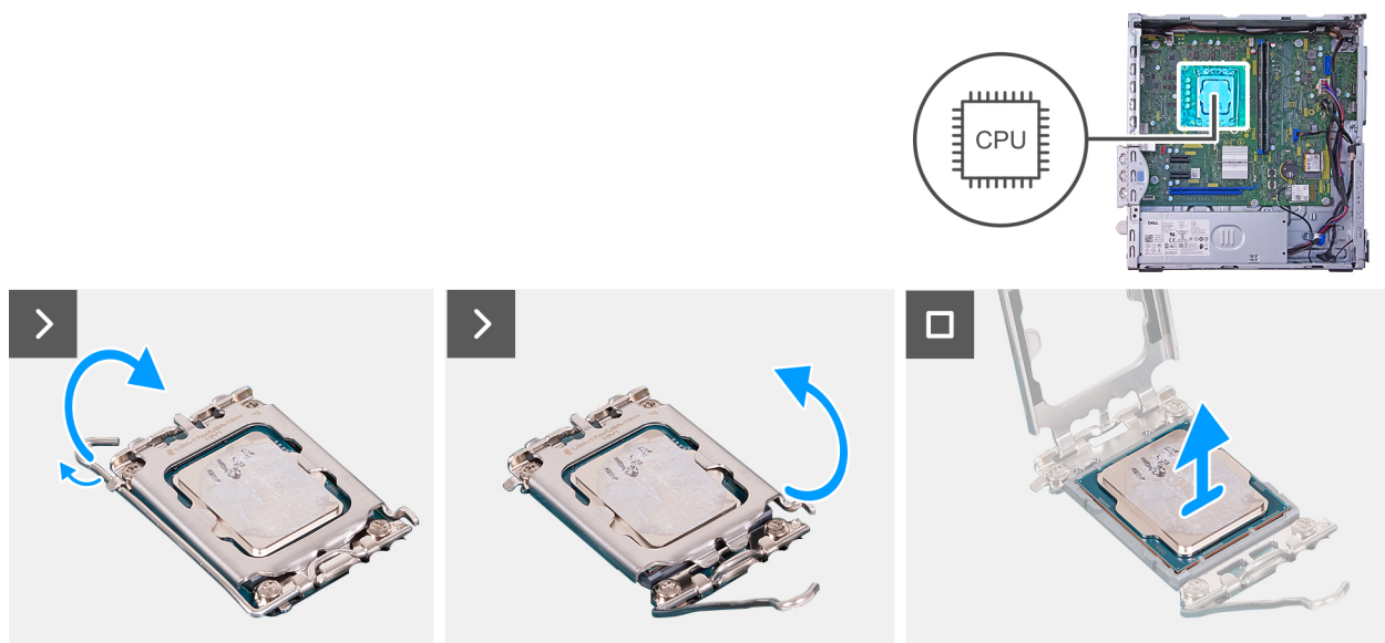
Figure 41. Retrait du processeur
