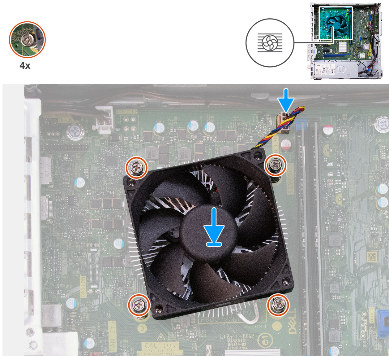
Figure 40. Installation de l'assemblage du ventilateur et du dissipateur de chaleur du processeur
