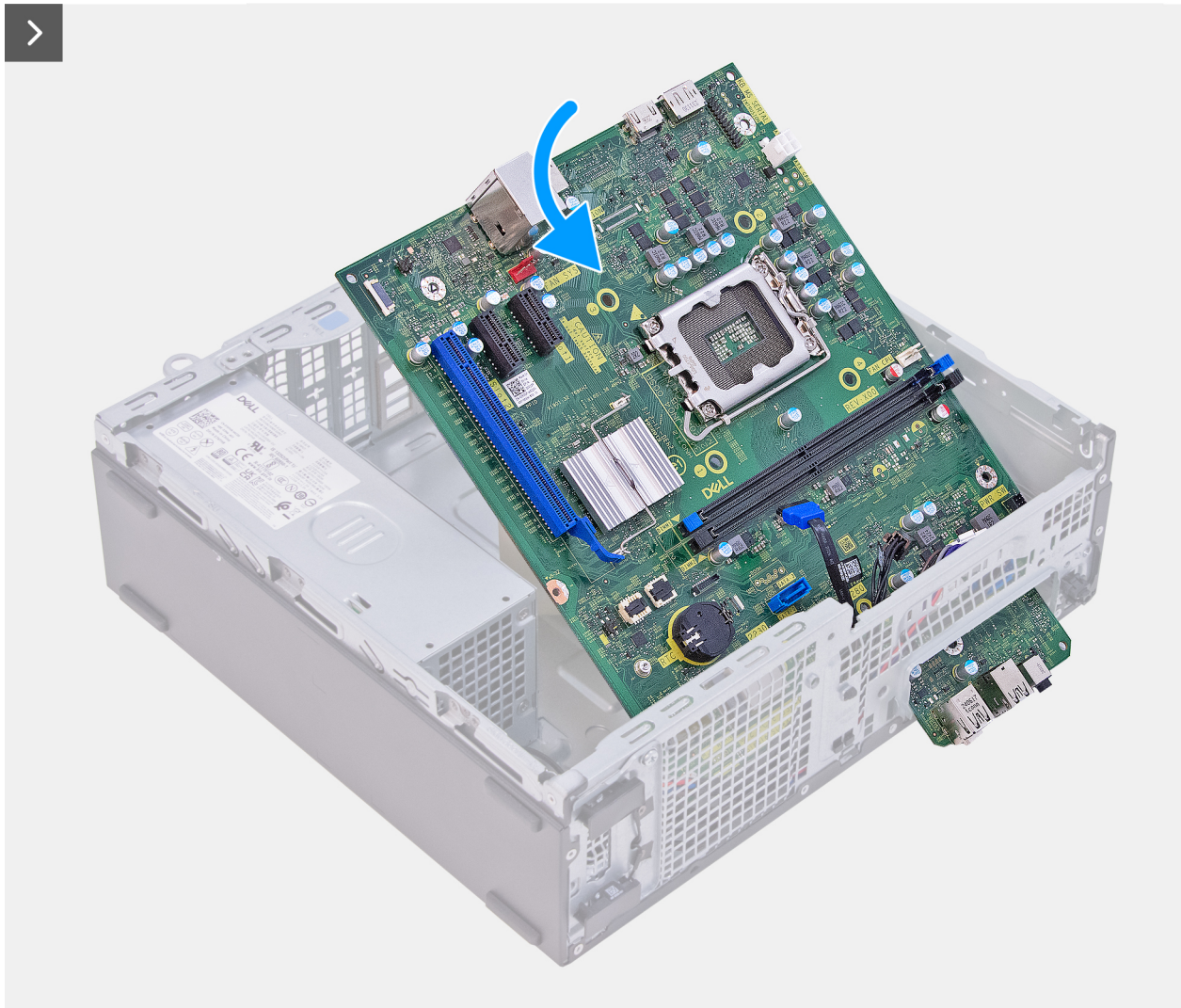
Figure 53. Installation de la carte système
