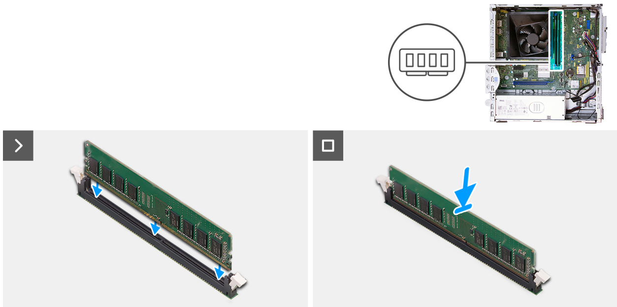
Figure 24. Installation du module de mémoire
