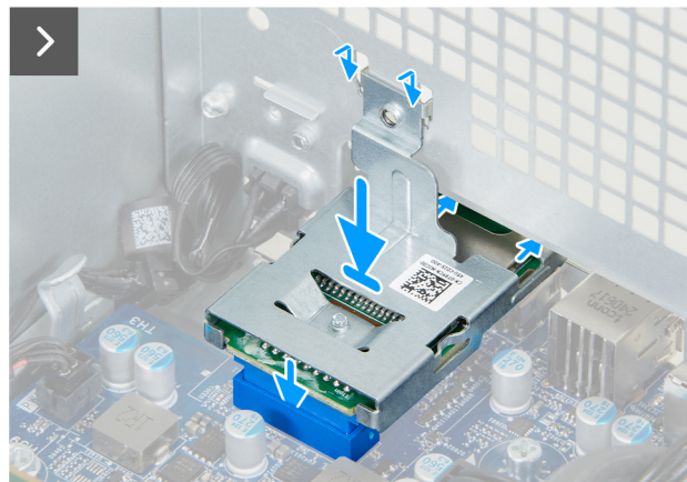
Figure 30. Installation du lecteur de carte média
