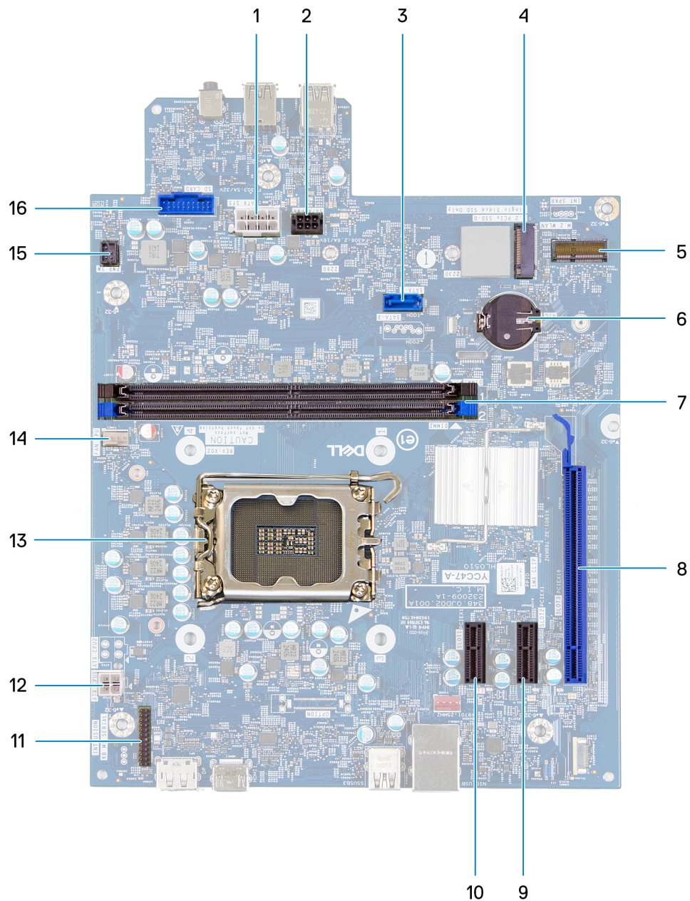
Figure 48. Présentation de la carte système
