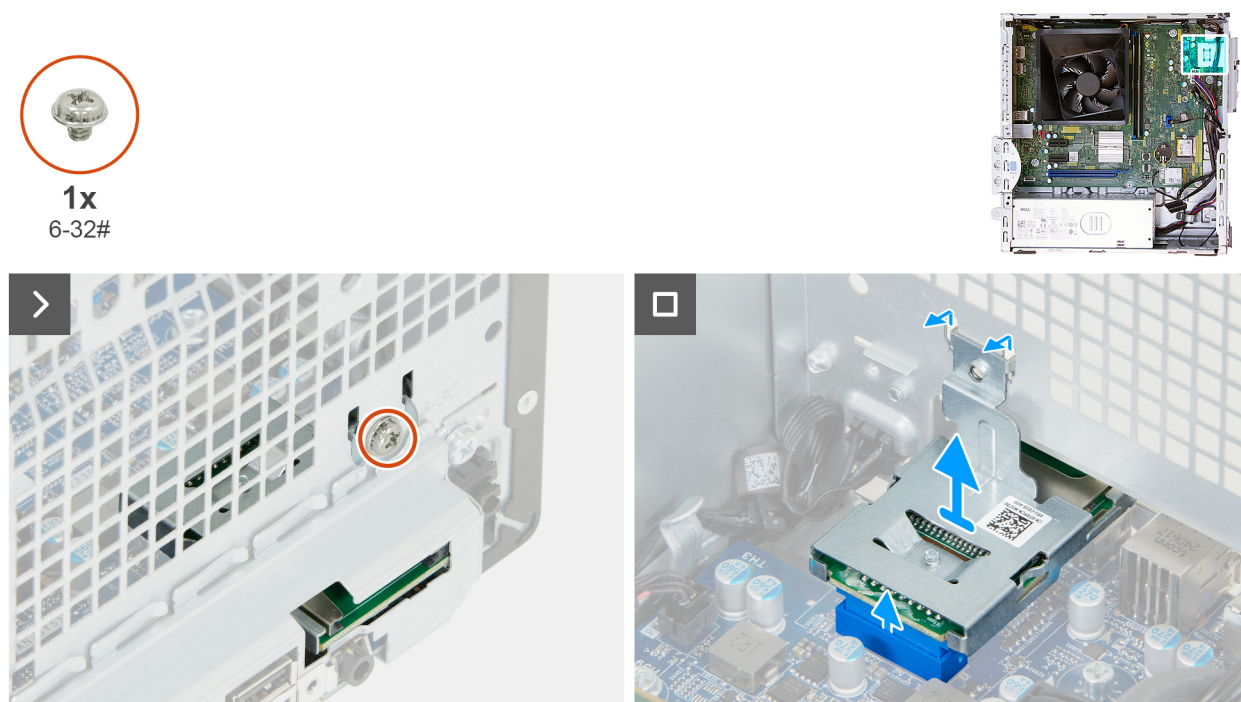
Figure 29. Retrait du lecteur de carte mémoire
