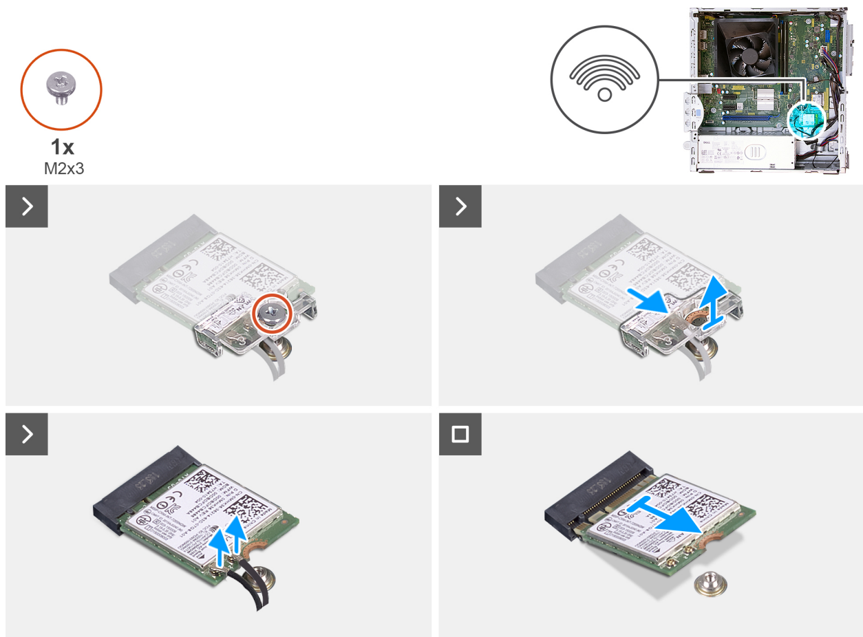
Figure 27. Retrait de la carte sans fil
