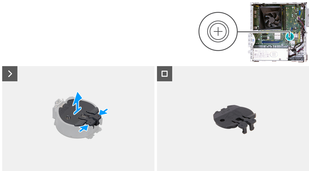
Figure 12. Retrait du capot de la pile bouton
