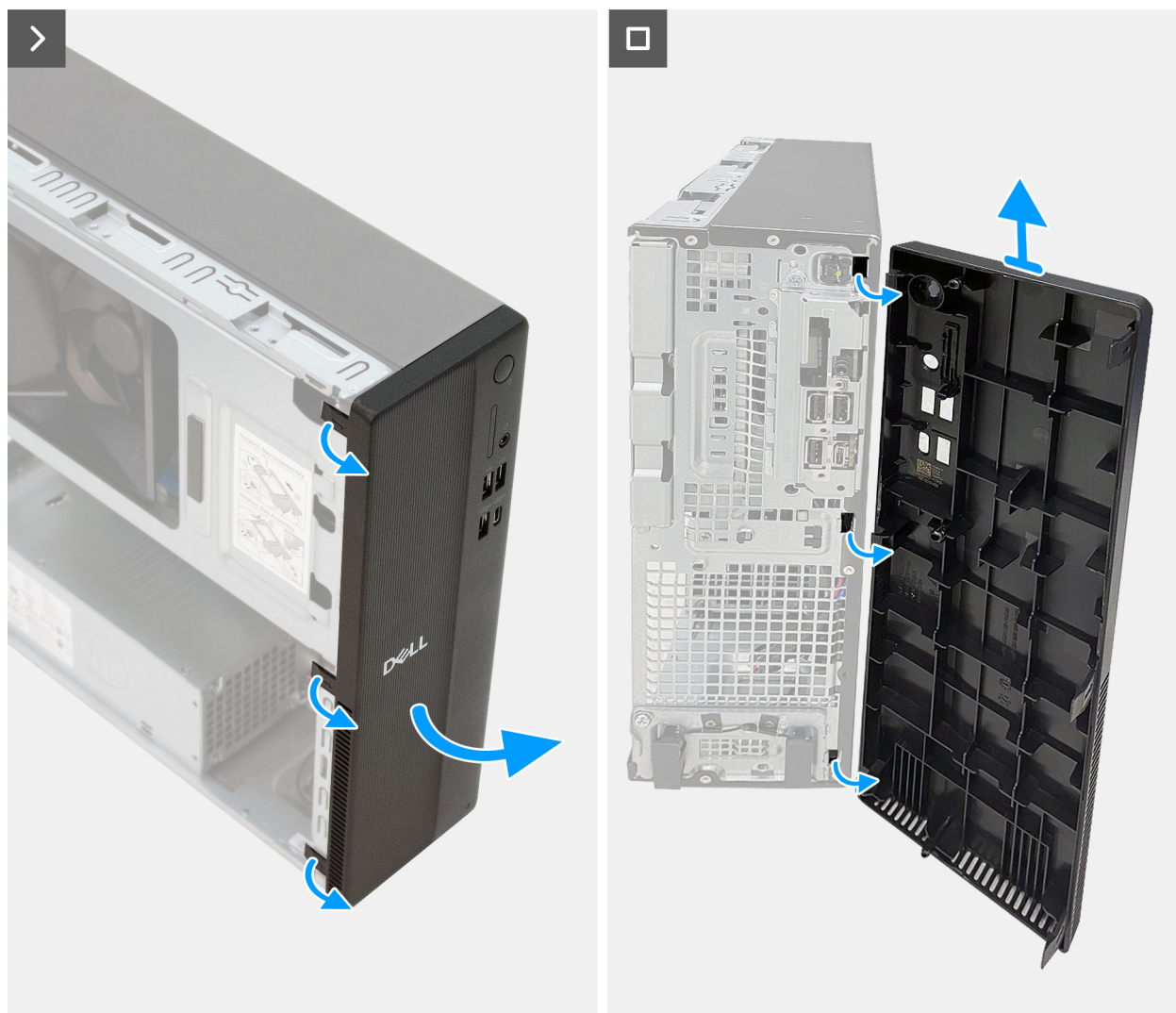
Figure 16. Retrait du capot avant
