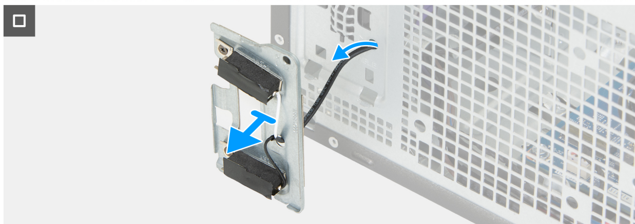
Figure 31. Retrait du module d'antenne
