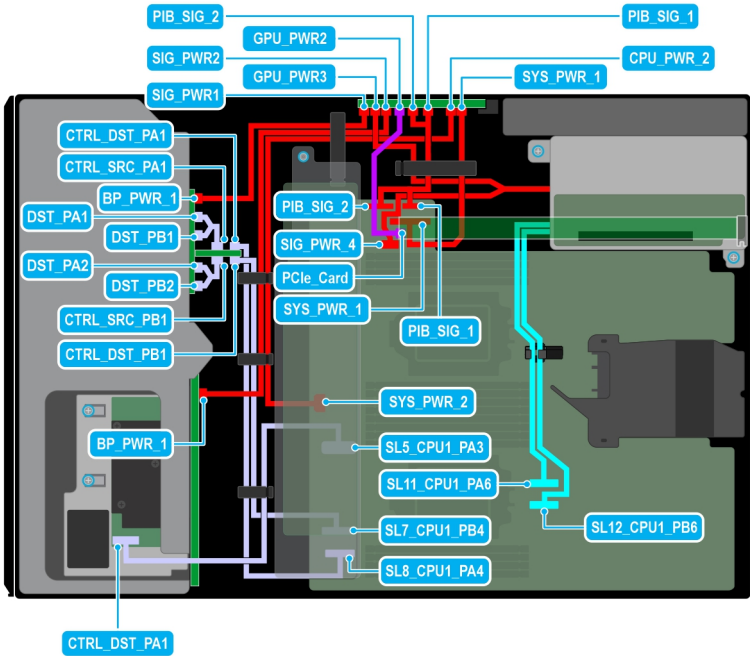
Ilustración 58. Configuración 20: 8 unidades de 3,5 pulgadas (SAS/SATA) + 8 unidades de 2,5 pulgadas (fPERC12 RAID NVMe) + GPUx1 en la CPU 2
