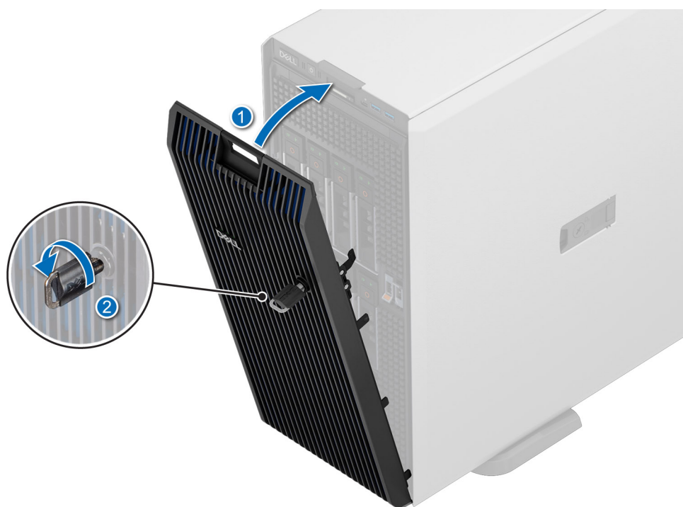
Ilustración 23. Instalación del bisel frontal
