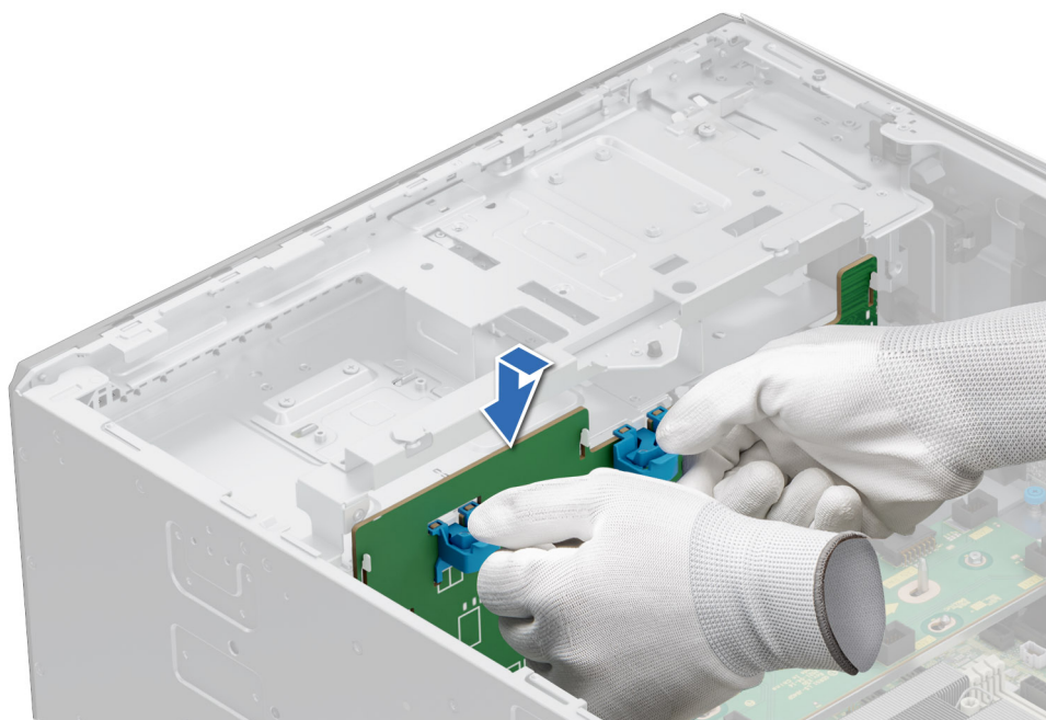
Ilustración 110. Instalación del backplane para unidades de 3,5 pulgadas
