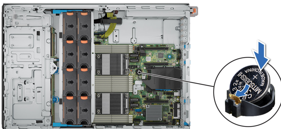
Ilustración 181. Instalación de la batería del sistema
