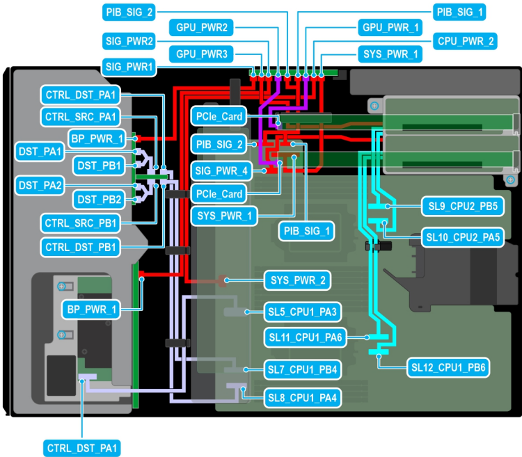
Ilustración 52. Configuración 14: 8 unidades de 3,5 pulgadas (SAS/SATA) + 8 unidades de 2,5 pulgadas (fPERC12 RAID NVMe) + GPUx2 en la CPU 2
