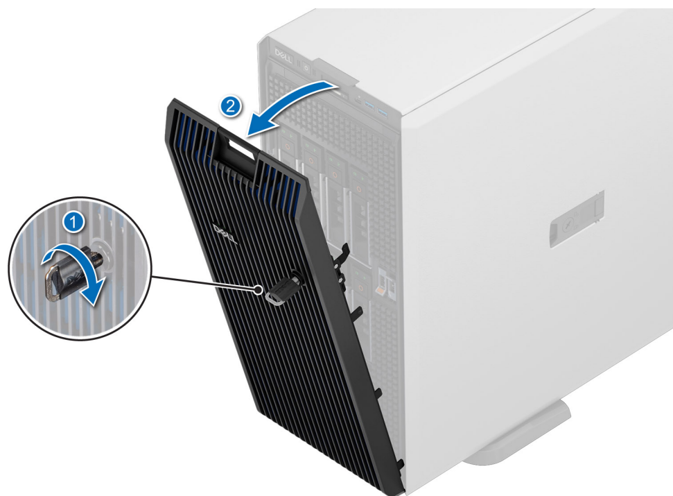
Ilustración 22. Extracción del bisel frontal
