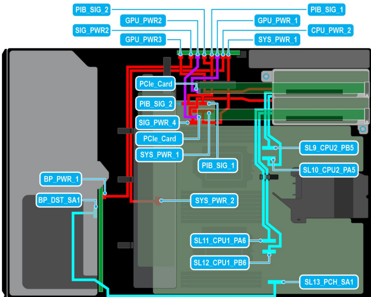
Ilustración 40. Configuración 2: 8 unidades de 3,5 pulgadas (chipset SATA) + GPUx2 en la CPU 2
