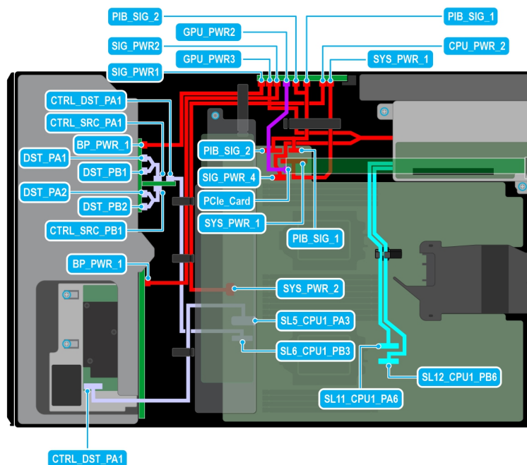
Figure 57. Configuration 19 : 8 disques de 3,5 pouces (SAS/SATA) + 8 disques de 2,5 pouces (NVMe RAID fPERC11) + 1 processeur graphique sur le processeur 2
