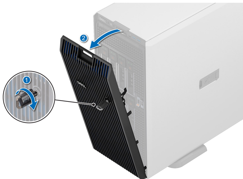
Figure 22. Retrait du panneau avant
