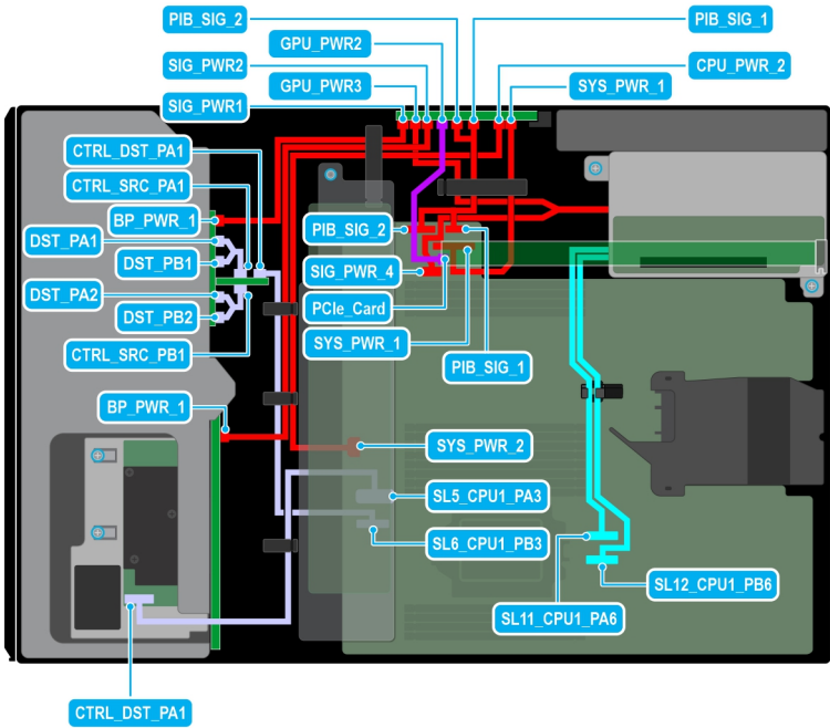
Figure 54. Configuration 16 : 8 disques de 3,5 pouces (SAS/SATA) + 8 disques de 2,5 pouces (NVMe RAID fPERC11) + 1 processeur graphique sur le processeur 1
