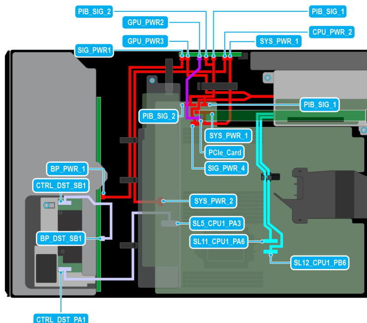
Figure 65. Configuration 27 : 12 disques de 3,5 pouces (SAS/SATA) + 1 processeur graphique sur le processeur 1
