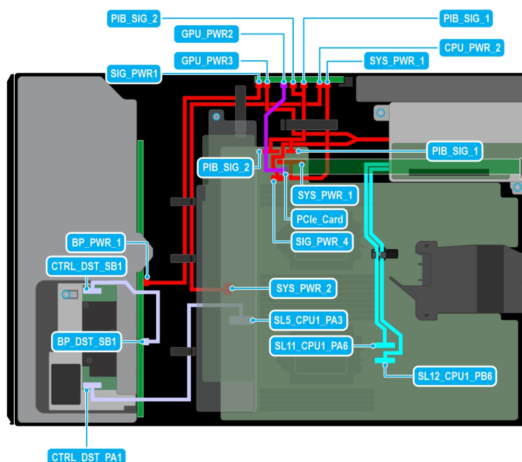
Figure 66. Configuration 28 : 12 disques de 3,5 pouces (SAS/SATA) + 1 processeur graphique sur le processeur 2
