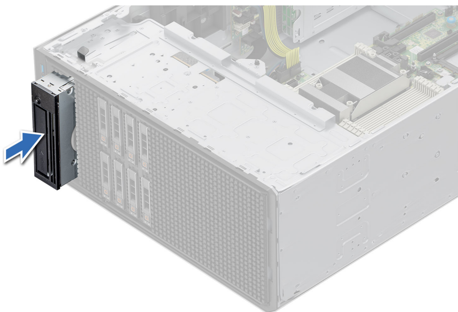
Figure 132. Installation de l'unité de sauvegarde sur bande
