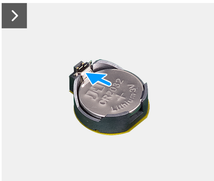
Ilustración 40. Extracción de la batería de tipo botón
