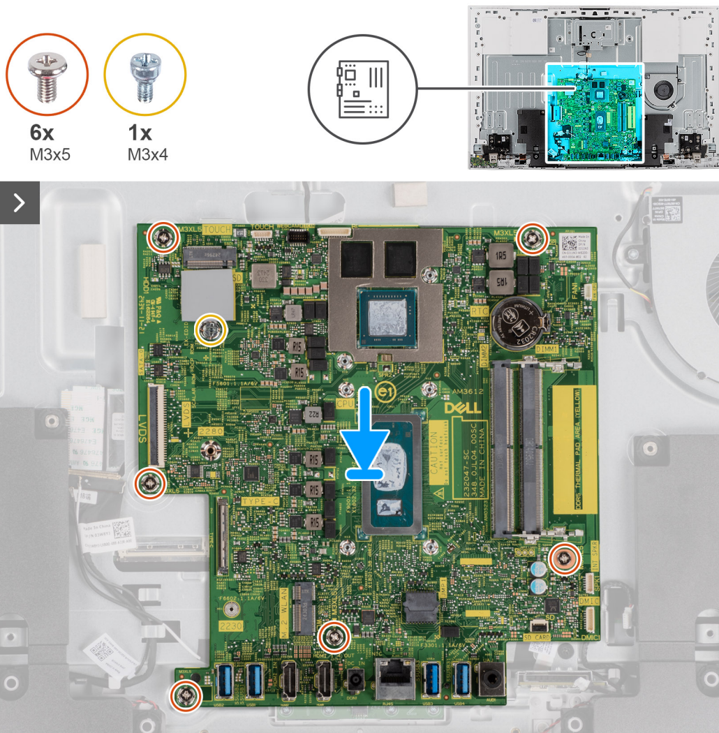
Ilustración 54. Coloque la tarjeta madre en el chasis
