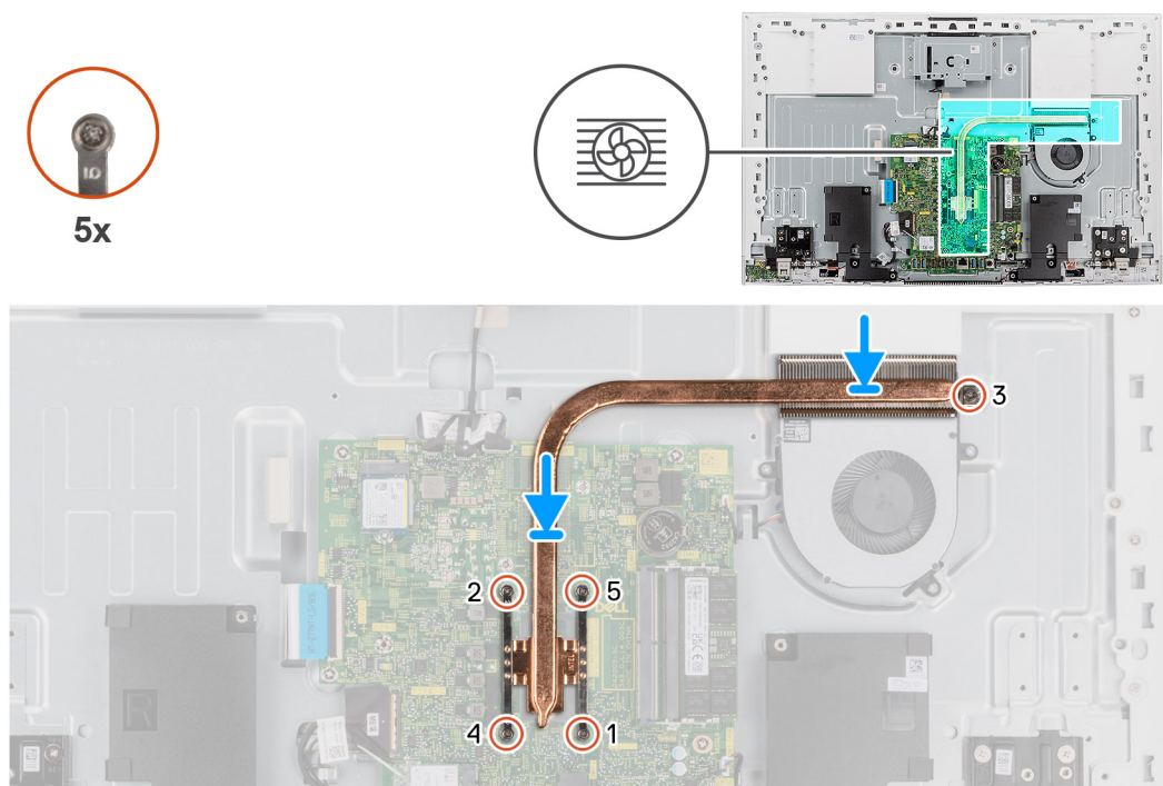
Ilustración 43. Instalación del disipador de calor: UMA
