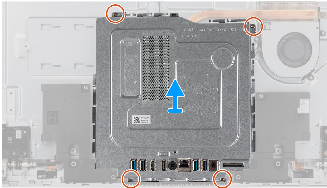
Ilustración 26. Extracción del protector de la tarjeta madre
