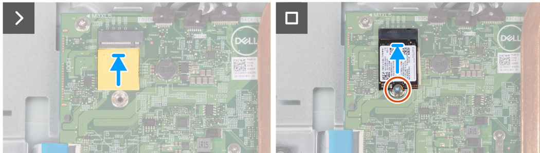
Ilustración 29. Instalación de la unidad de estado sólido M.2 2230
