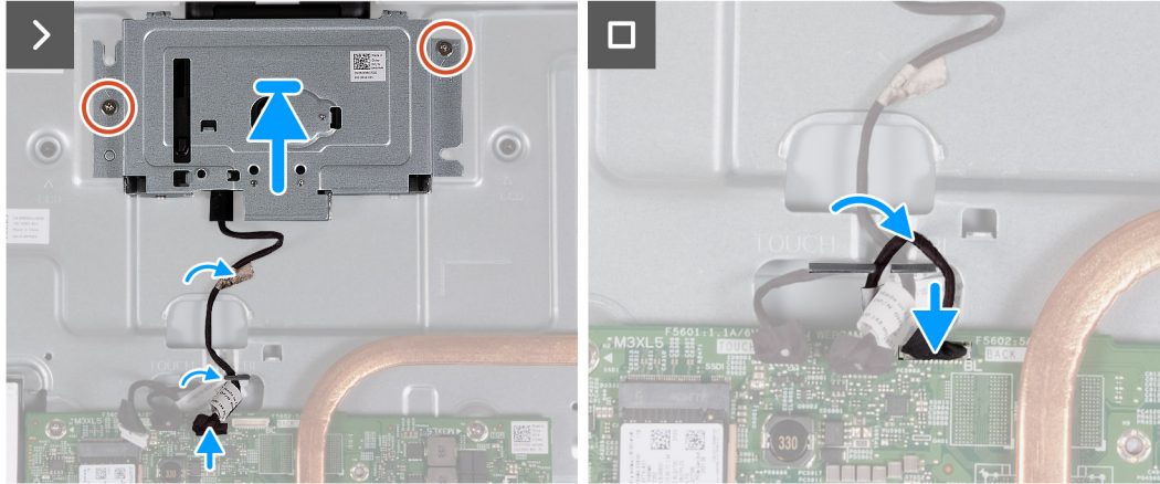
Ilustración 35. Instalación de la cámara
