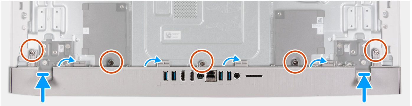
Ilustración 23. Instalación de la cubierta inferior
