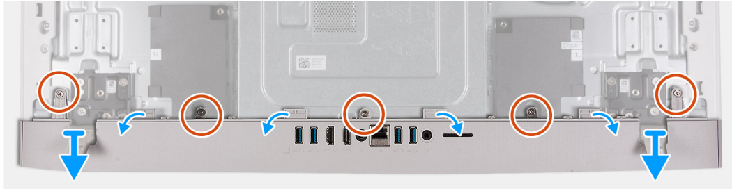
Ilustración 22. Extracción de la cubierta de I/O
