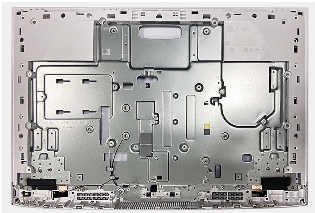
Ilustración 64. Extracción del ensamblaje de la trama intermedia
