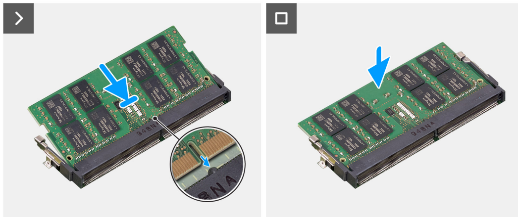
Ilustración 31. Instalación del módulo de memoria
