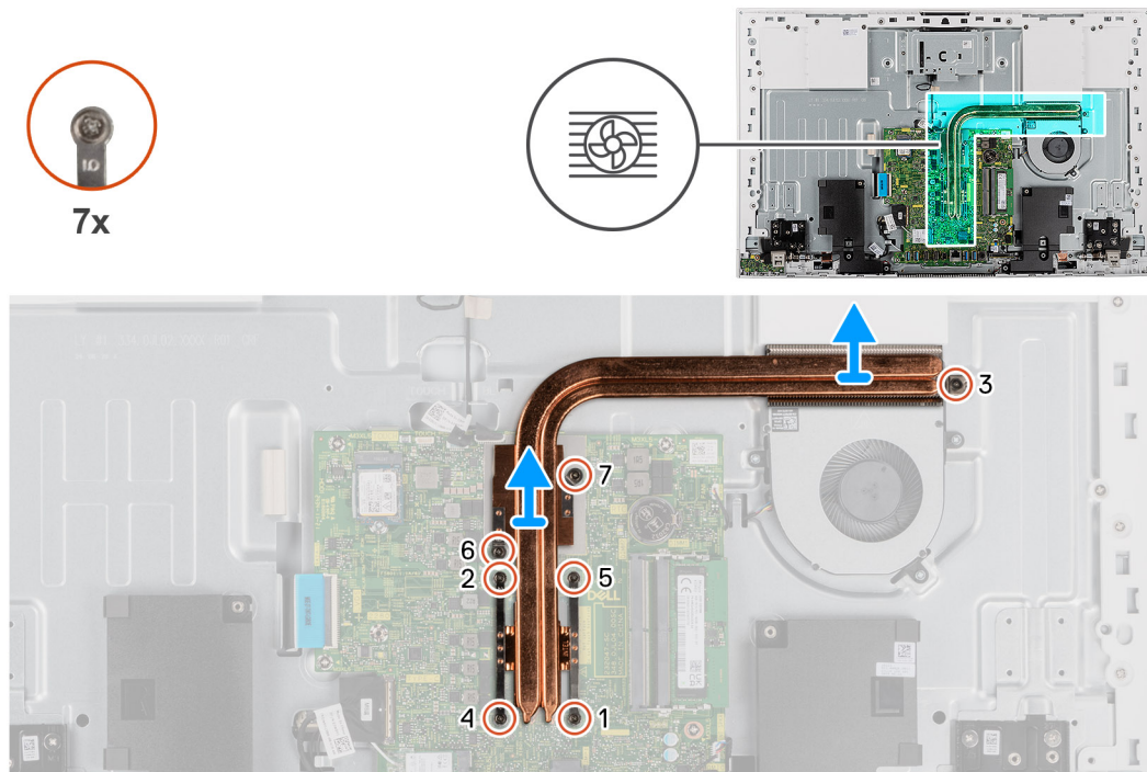
Ilustración 44. Extracción del disipador de calor: discreto
