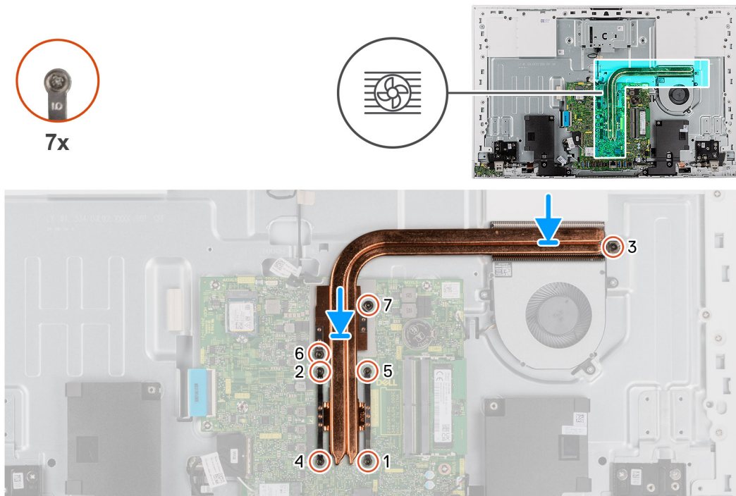
Ilustración 45. Instalación del disipador de calor: discreto
