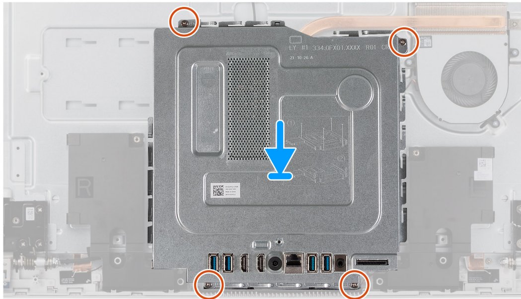
Ilustración 27. Instalación del protector de la tarjeta madre
