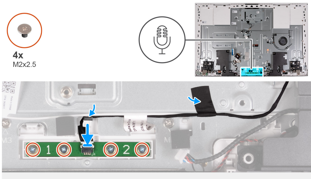
Ilustración 57. Instalación del módulo del micrófono
