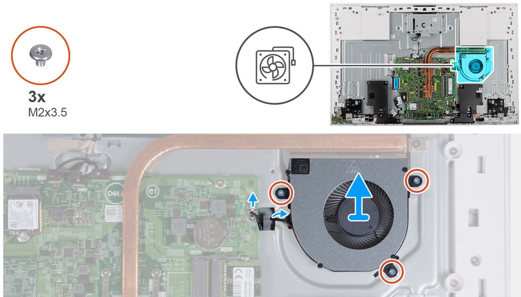
Ilustración 36. Extracción del ventilador
