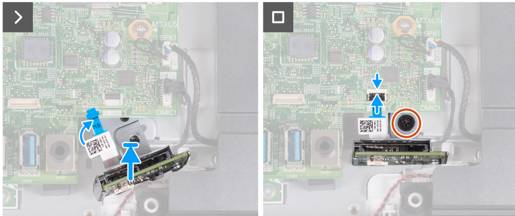
Ilustración 47. Instalación del lector de tarjetas de medios
