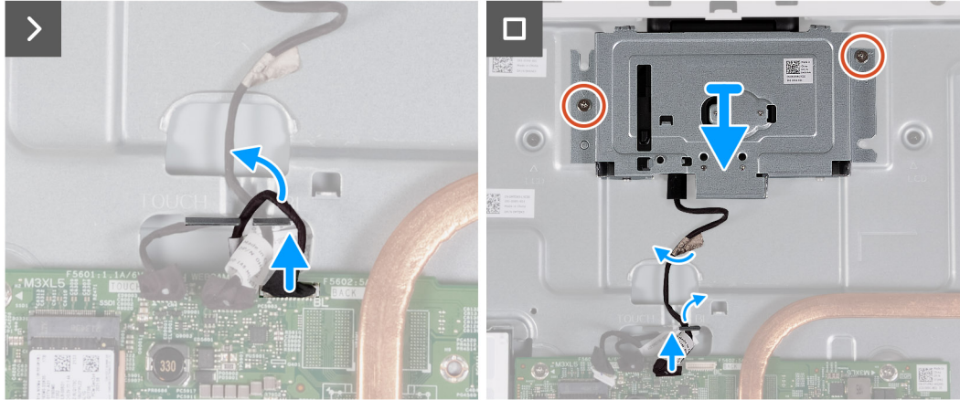
Ilustración 34. Extracción de la cámara
