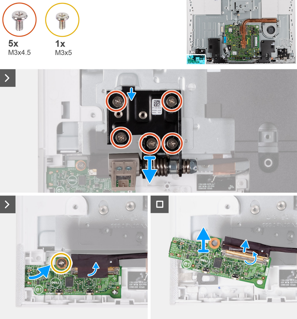
Ilustración 48. Extracción de la placa del botón de encendido con USB
