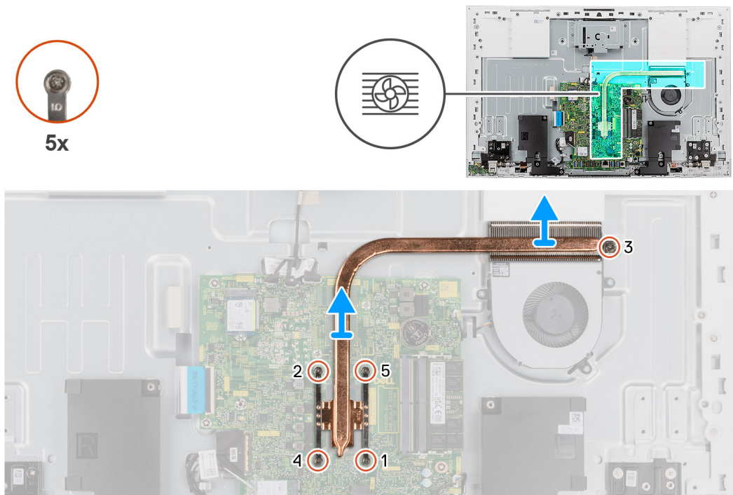
Ilustración 42. Extracción del disipador de calor: UMA
