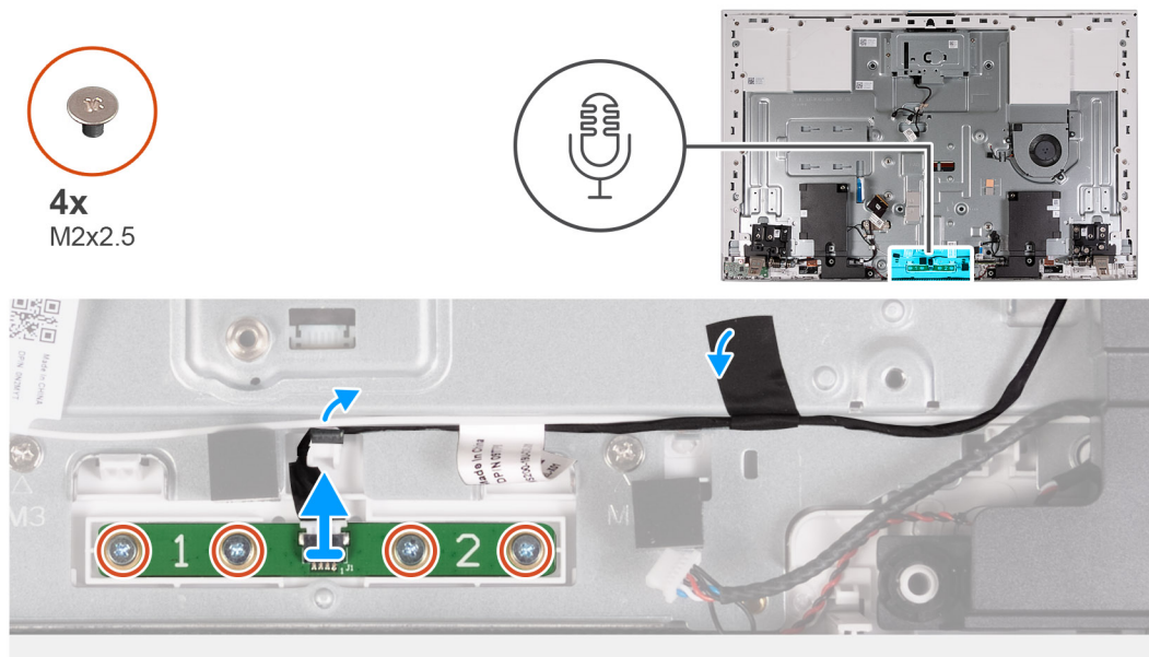
Ilustración 56. Extracción del módulo del micrófono
