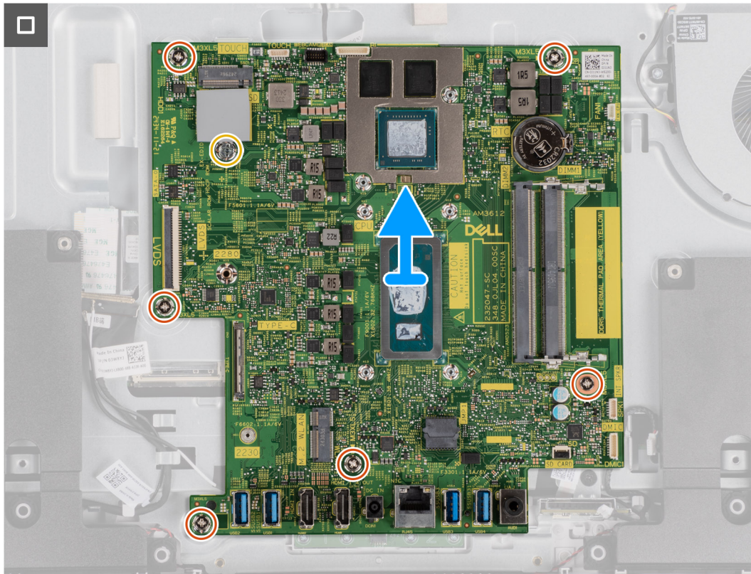
Ilustración 52. Levante la tarjeta madre del sistema para quitarla del chasis.
