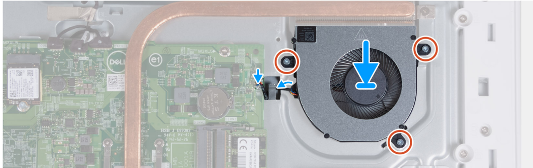
Ilustración 37. Instalación del ventilador
