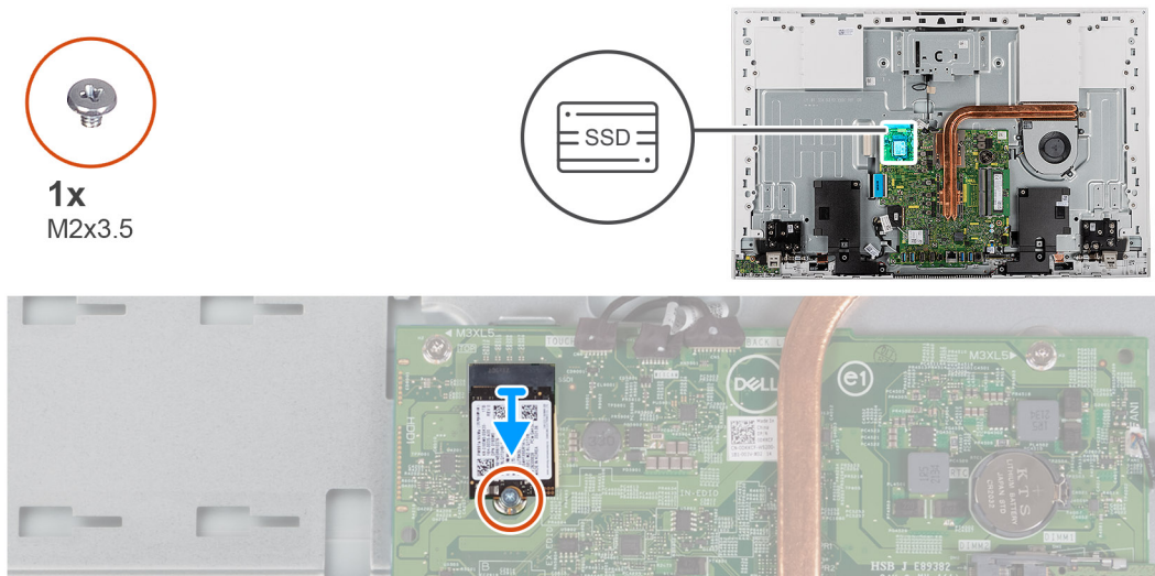
Ilustración 28. Extracción de la unidad de estado sólido M.2 2230
