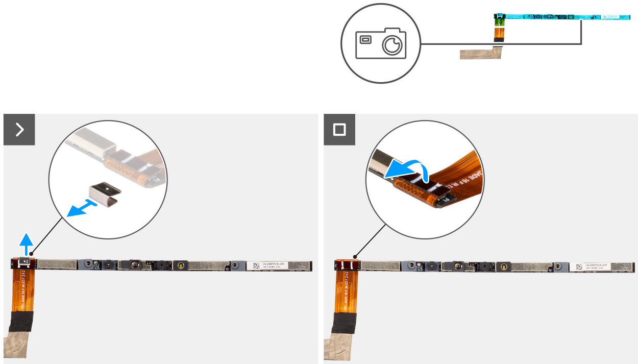
Ilustración 82. Extracción de la cámara
