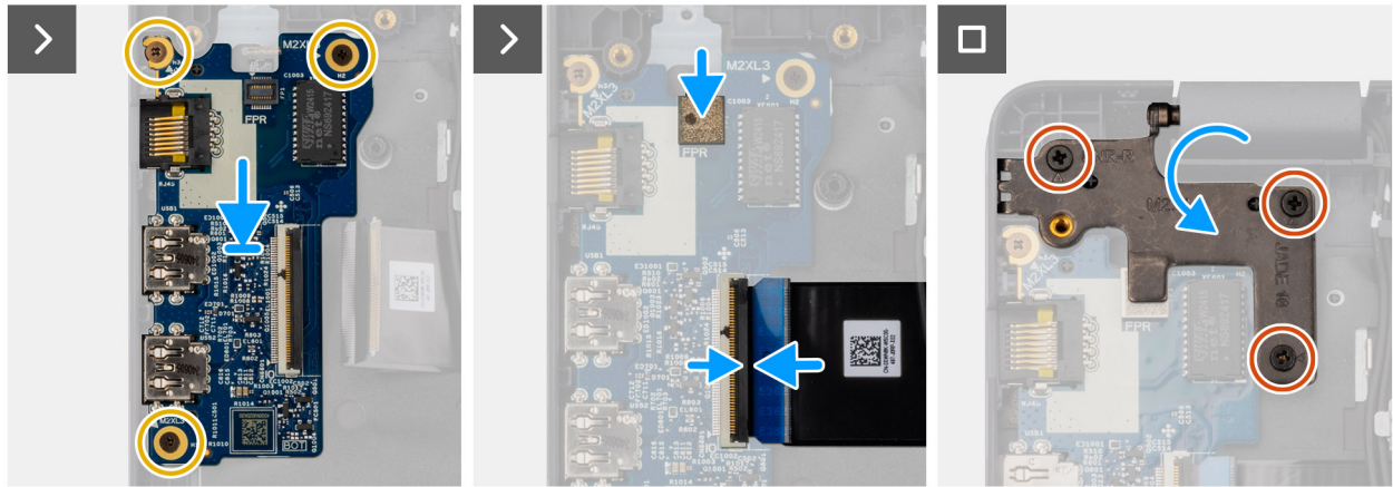
Ilustración 37. Instalación de la placa de I/O
