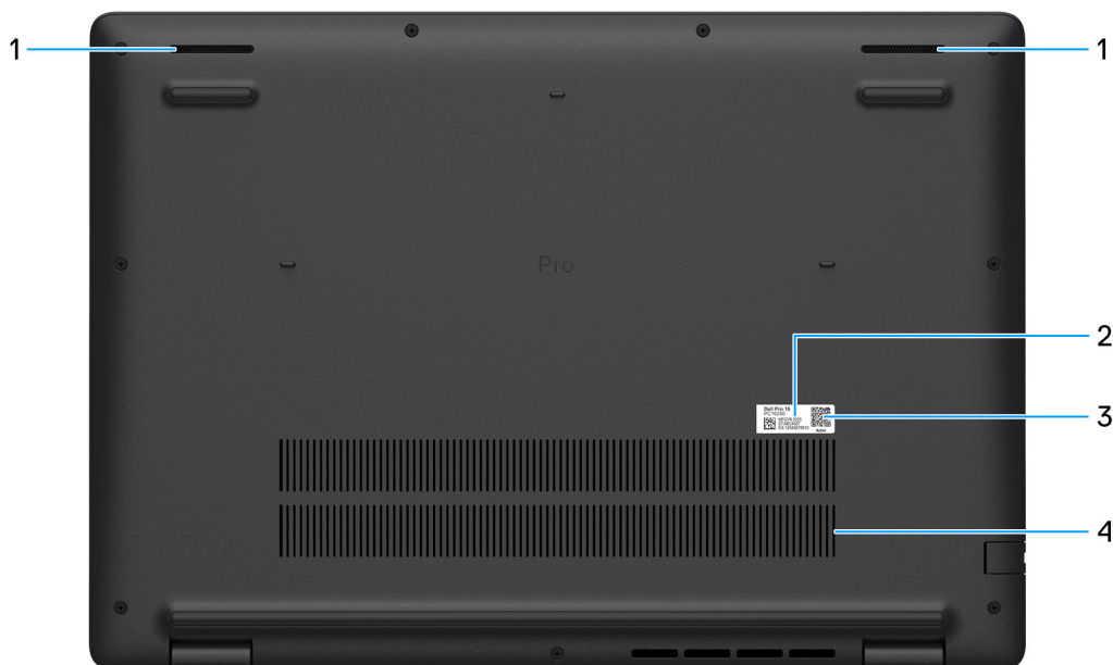
Ilustración 5. Vista inferior
