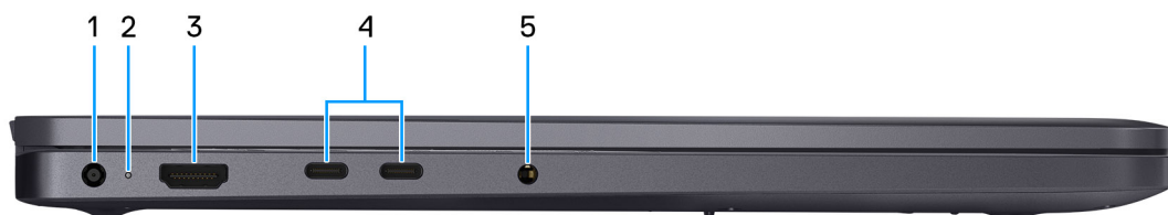
Ilustración 2. Vista izquierda
