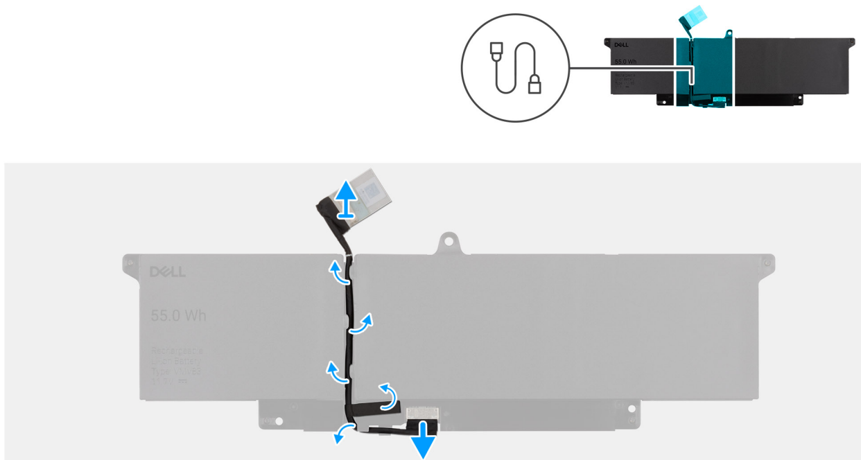
Ilustración 19. Extracción del cable de la batería
