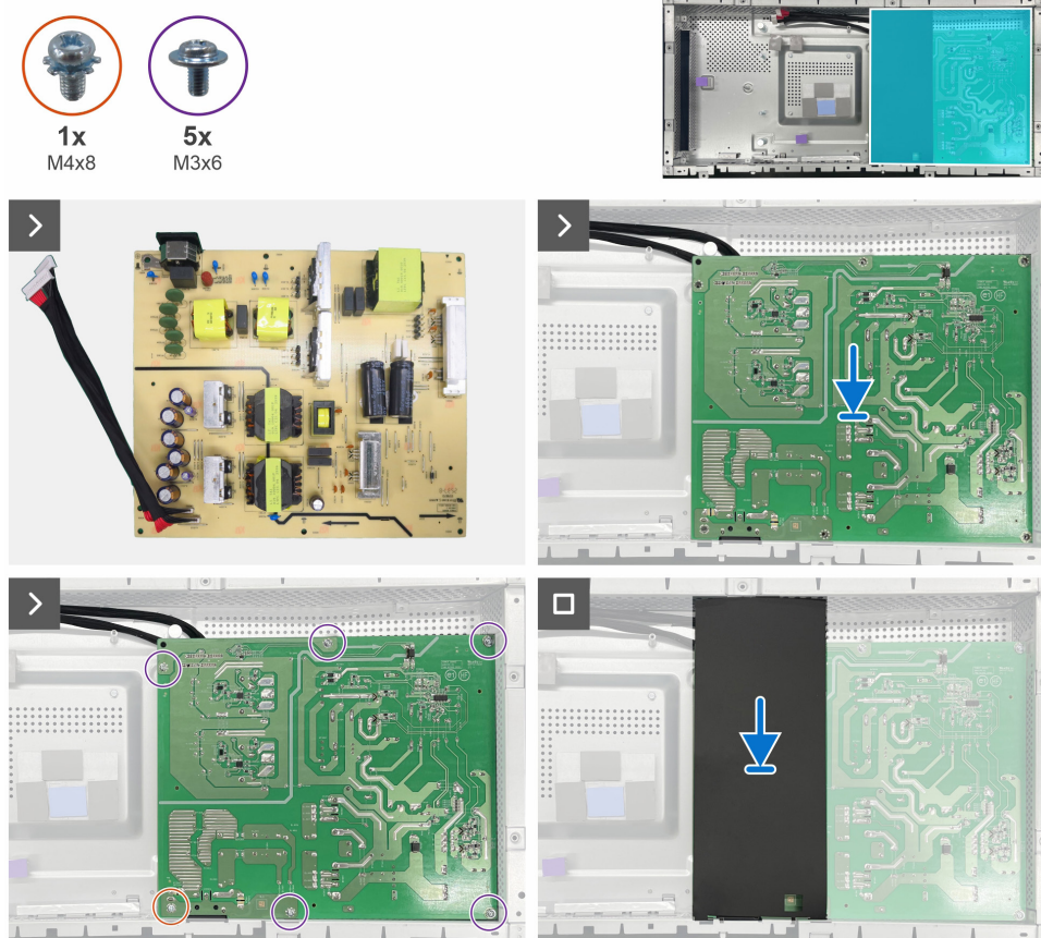
Figure 26. Installation de la carte d'alimentation
