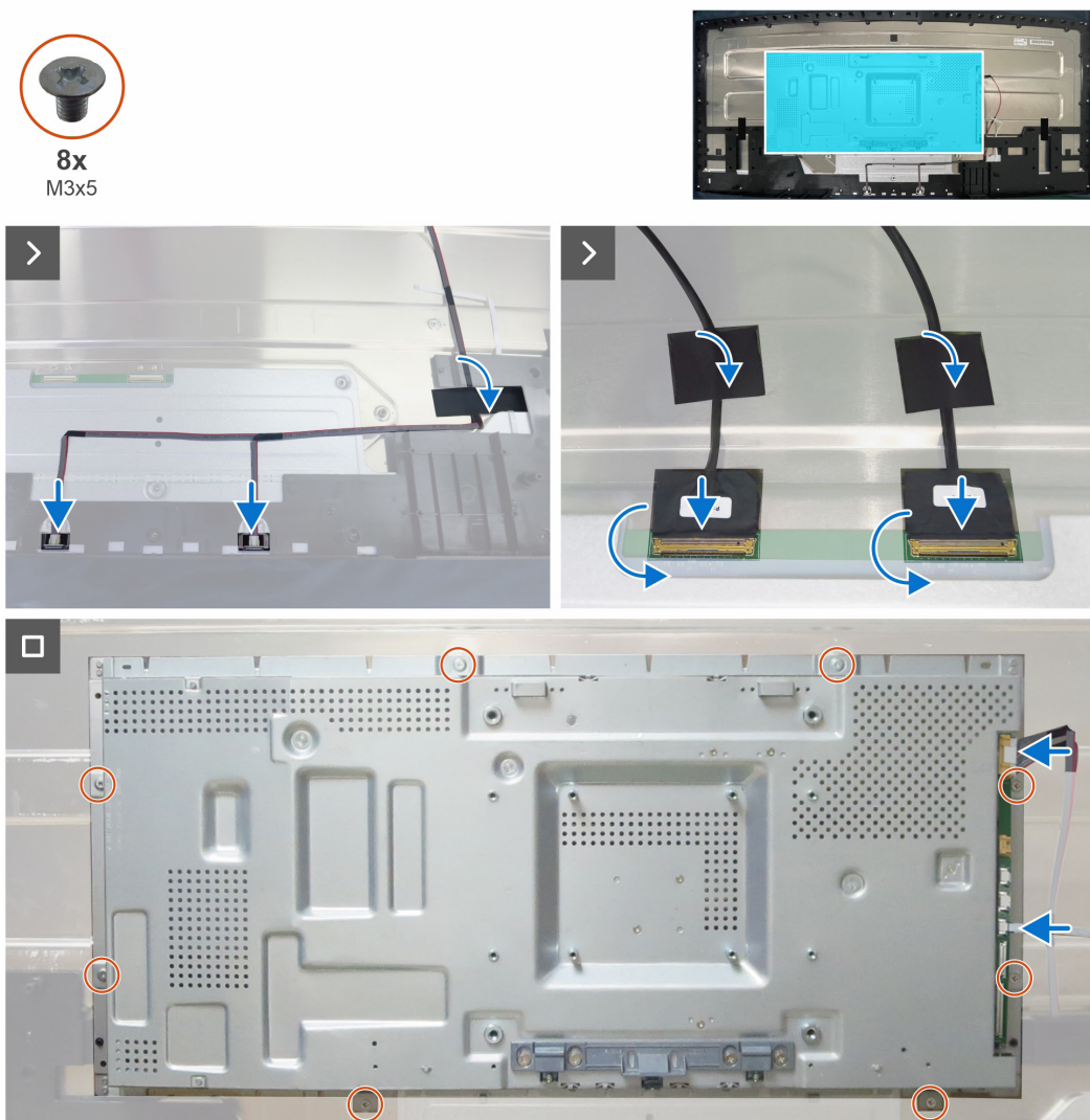
Figure 18. Installation du châssis principal
