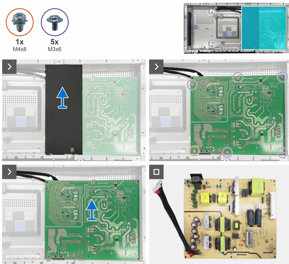
Figure 25. Retrait de la carte d'alimentation
