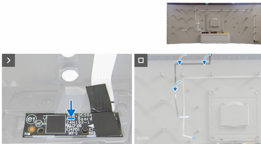
Figure 8. Installation de la carte ALS
