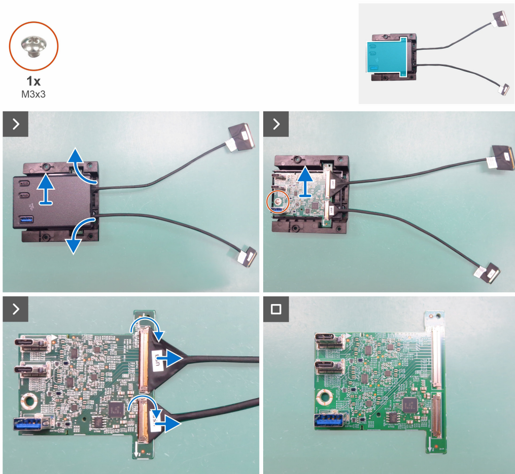
Figure 11. Retrait de la carte USB
