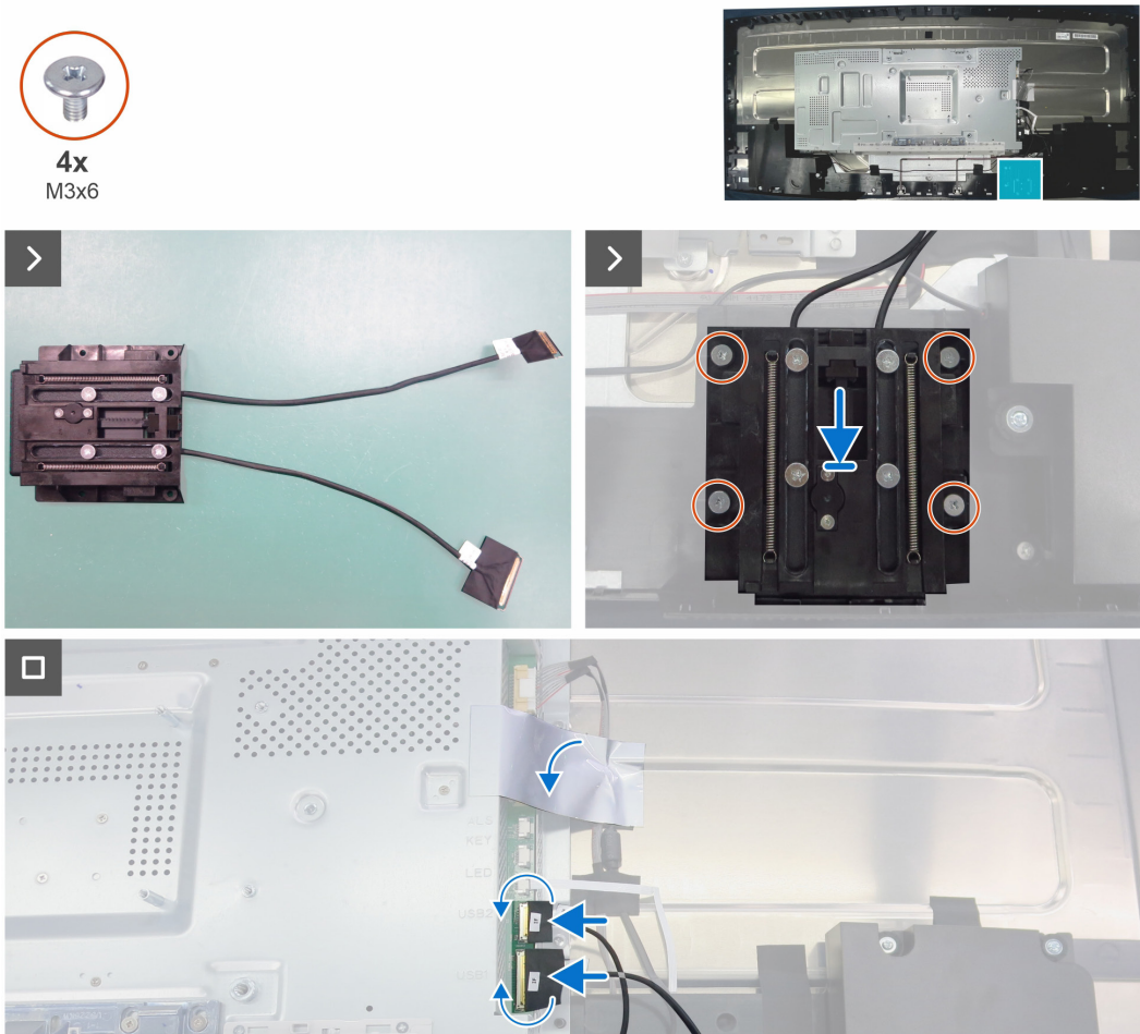
Figure 10. Installation du module QAP
