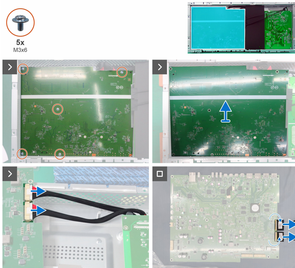
Figure 23. Retrait de la carte principale
