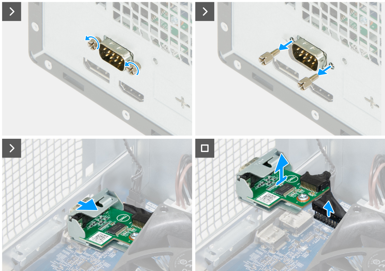
Abbildung 45. Entfernen des seriellen Anschlussmoduls
