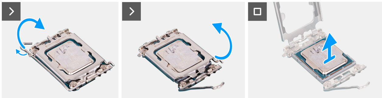
Abbildung 41. Entfernen des Prozessors
