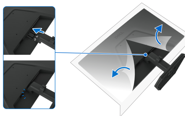
Figura 11. Fije el soporte
