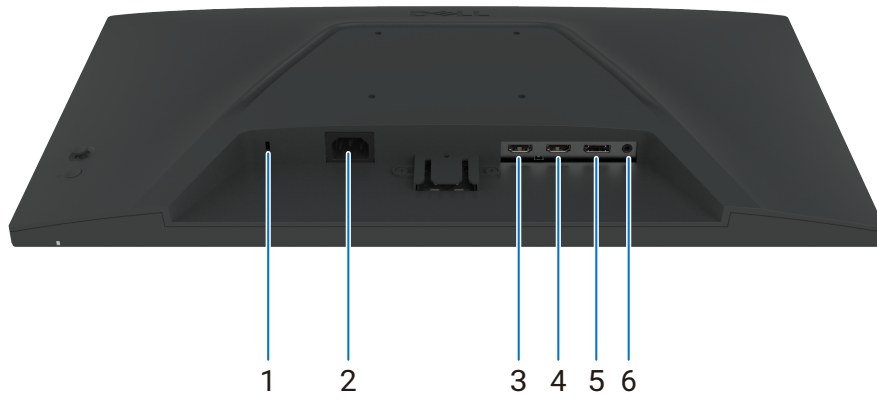
Figura 3. Vista inferior
