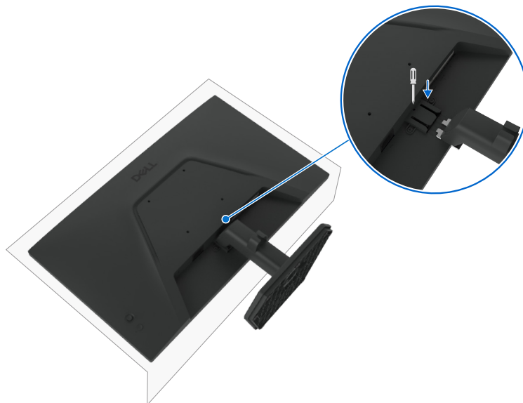
Figura 19. Desmontaje del soporte del monitor
