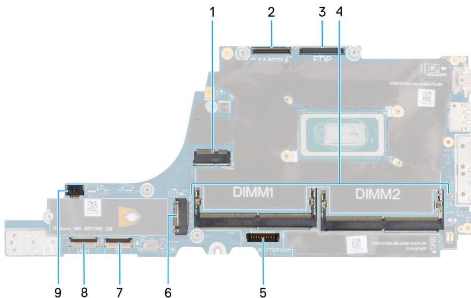
Abbildung 52. Anschlüsse auf der Hauptplatine
