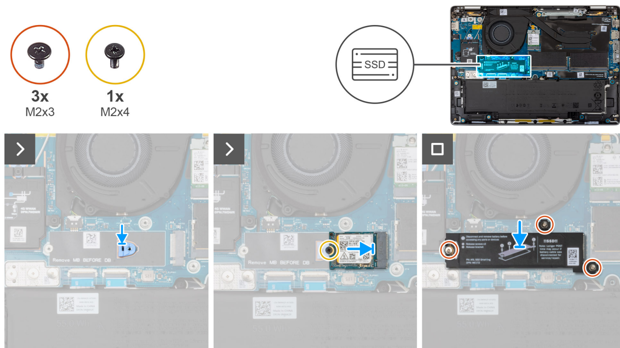
Abbildung 37. Einbauen des M.2-2280-SSD
