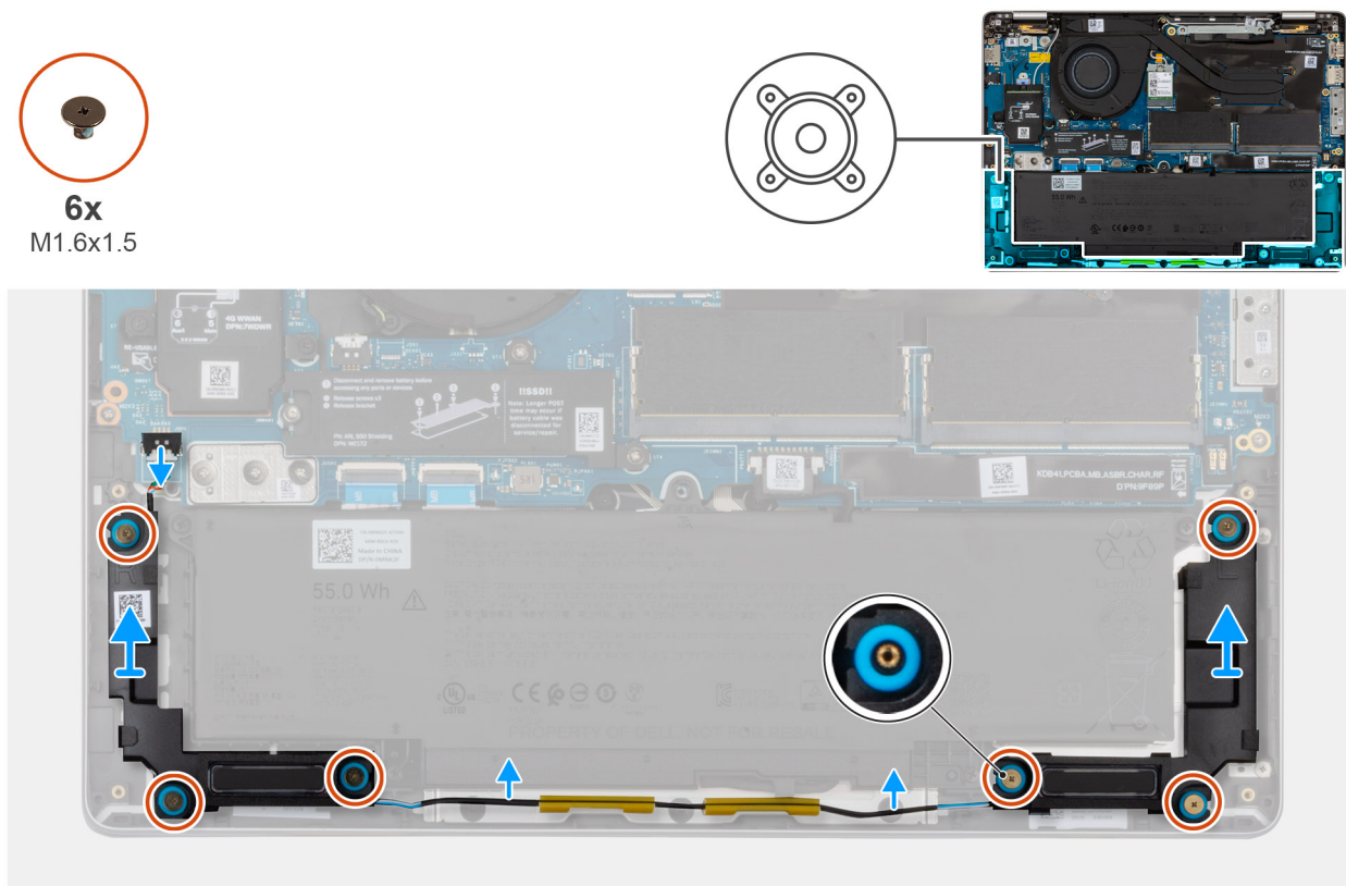
Abbildung 42. Entfernen der Lautsprecher
