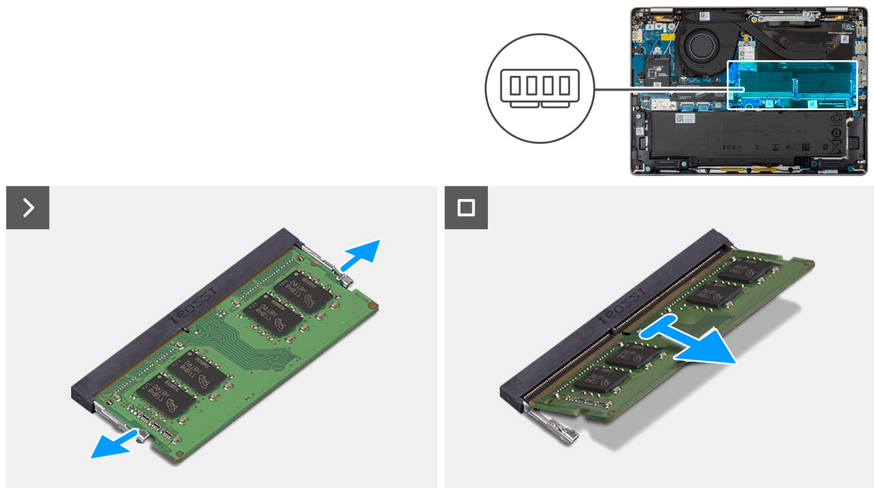
Abbildung 32. Entfernen des Arbeitsspeichersmoduls
