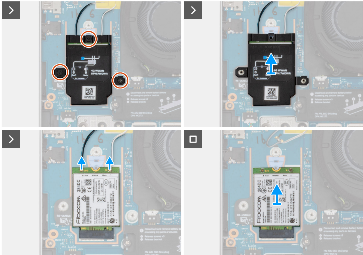
Abbildung 34. Entfernen der WWAN-Karte
