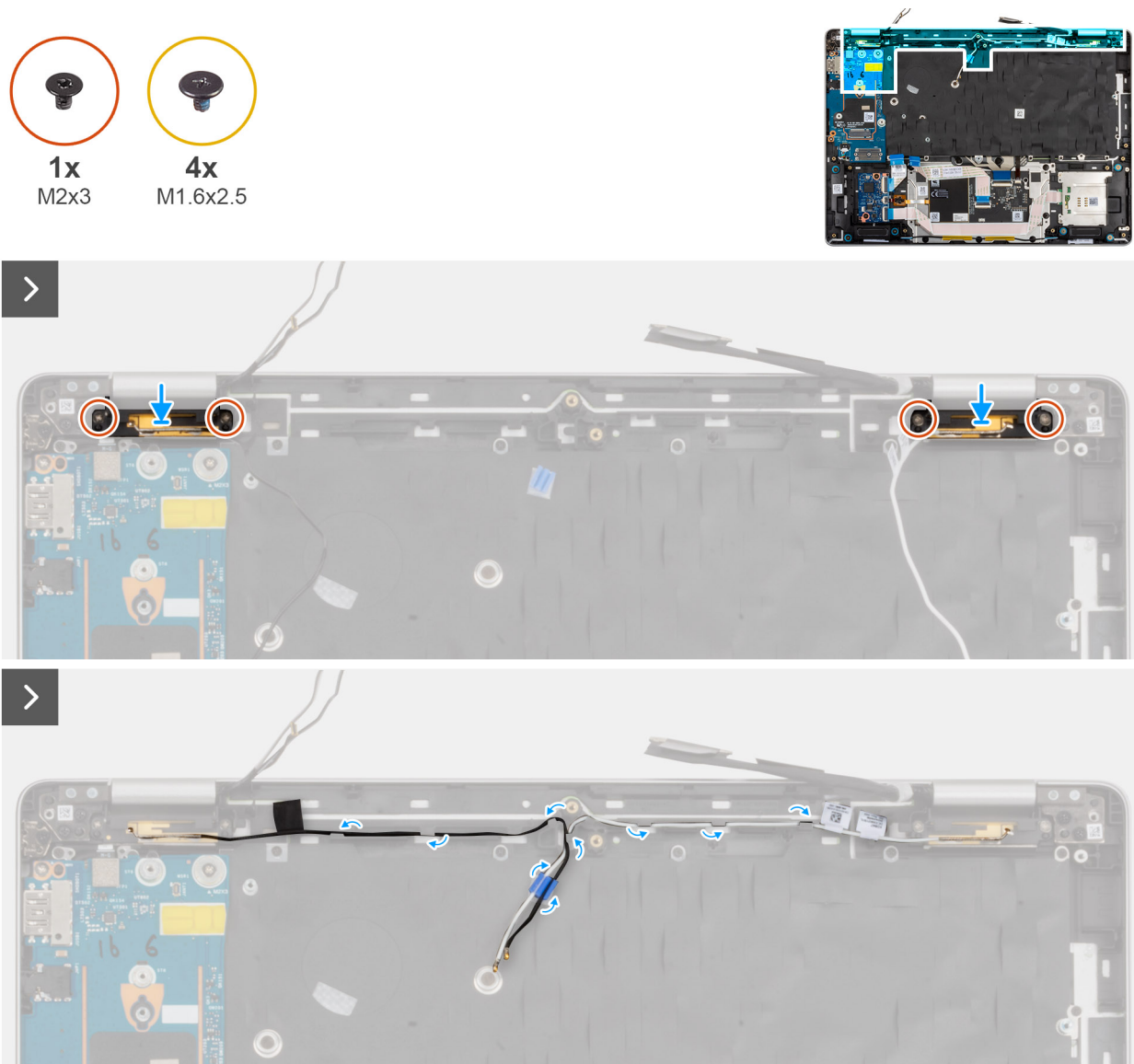
Abbildung 56. Einbauen des WLAN-Antennenmoduls
