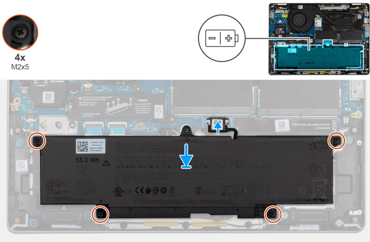
Abbildung 29. Einsetzen des Akkus
