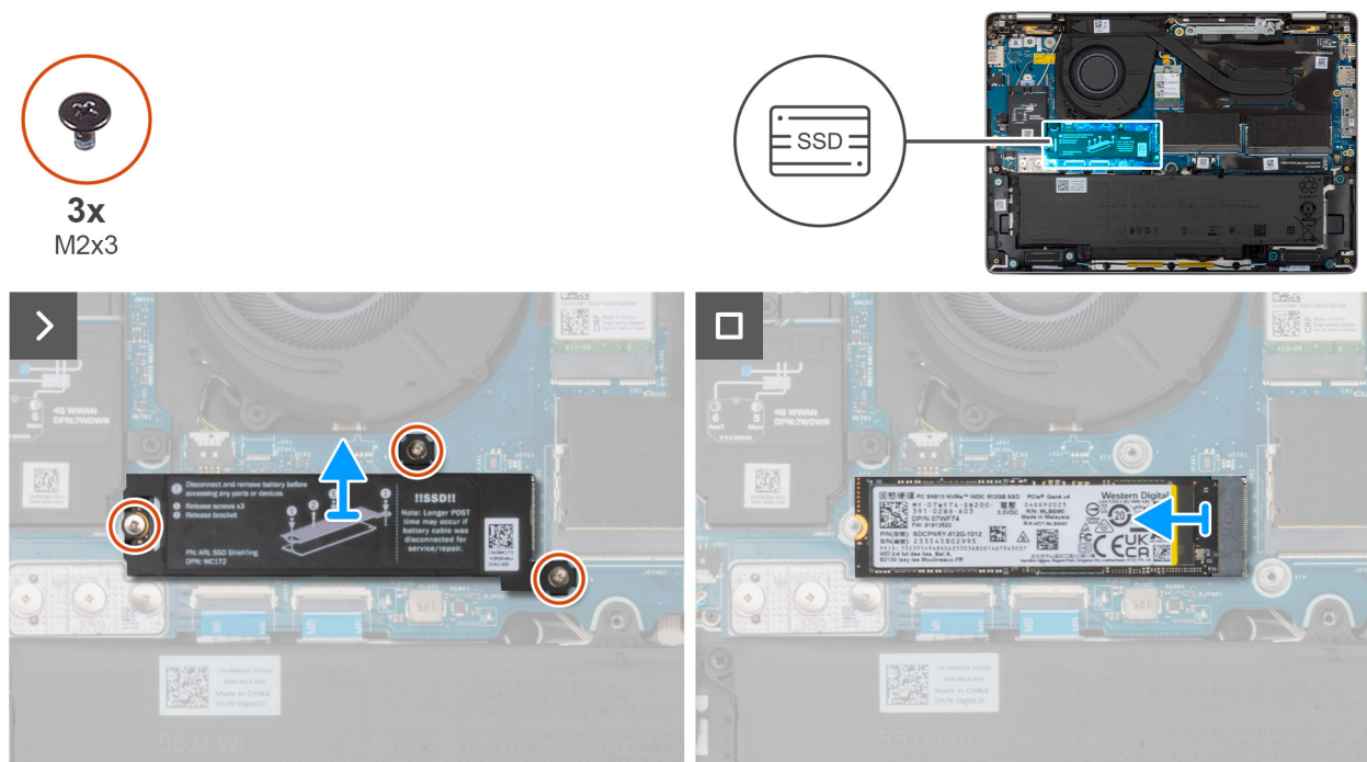
Abbildung 38. Entfernen der M.2-2280-SSD
