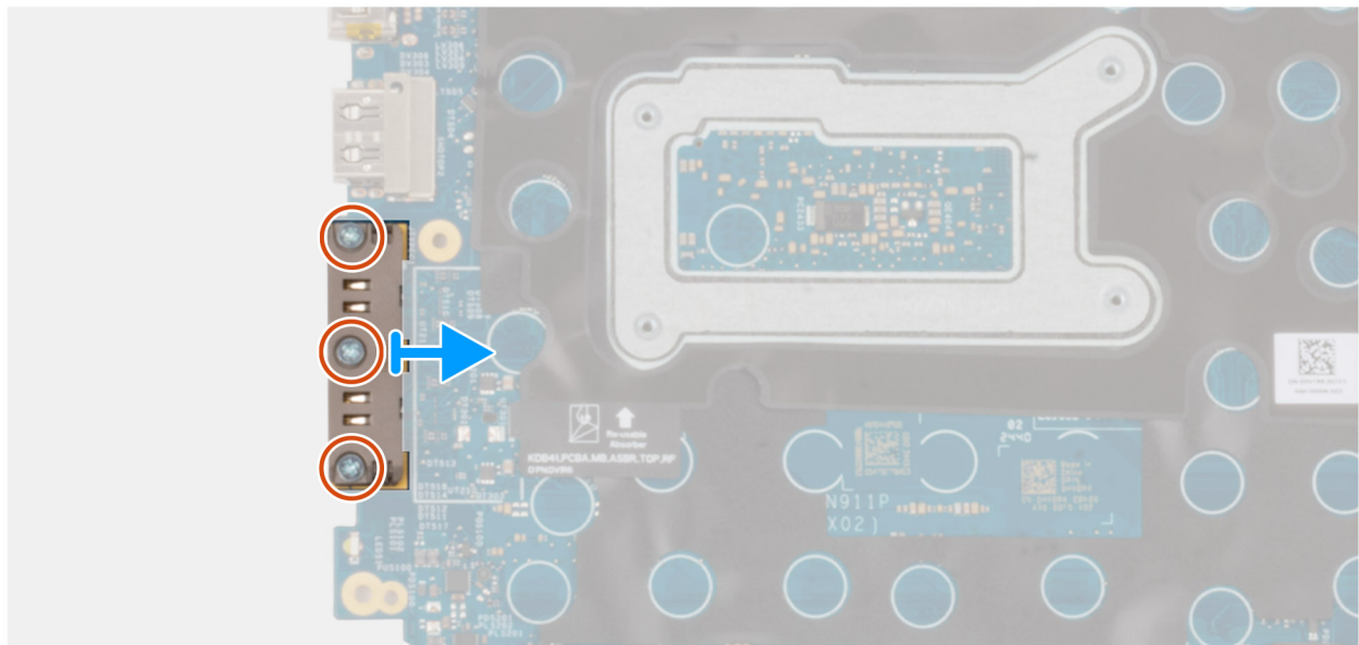
Abbildung 58. Entfernen des USB-Typ-C-Anschlussmoduls
