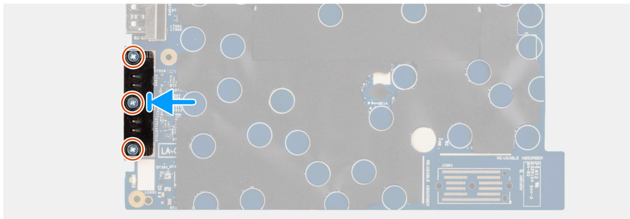
Abbildung 52. Installieren des USB-Typ-C-Anschlussmoduls
