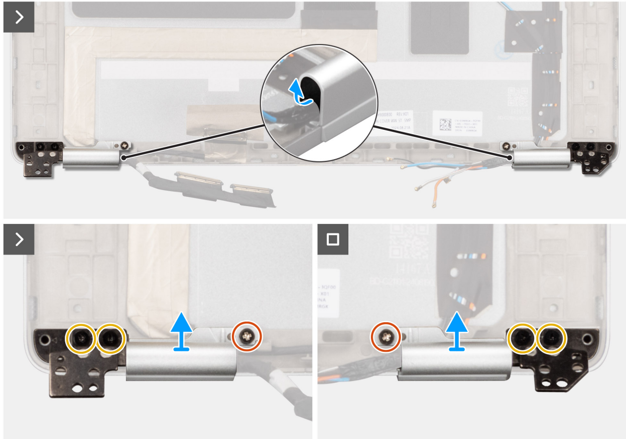
Abbildung 73. Entfernen der Bildschirmscharnierabdeckungen
