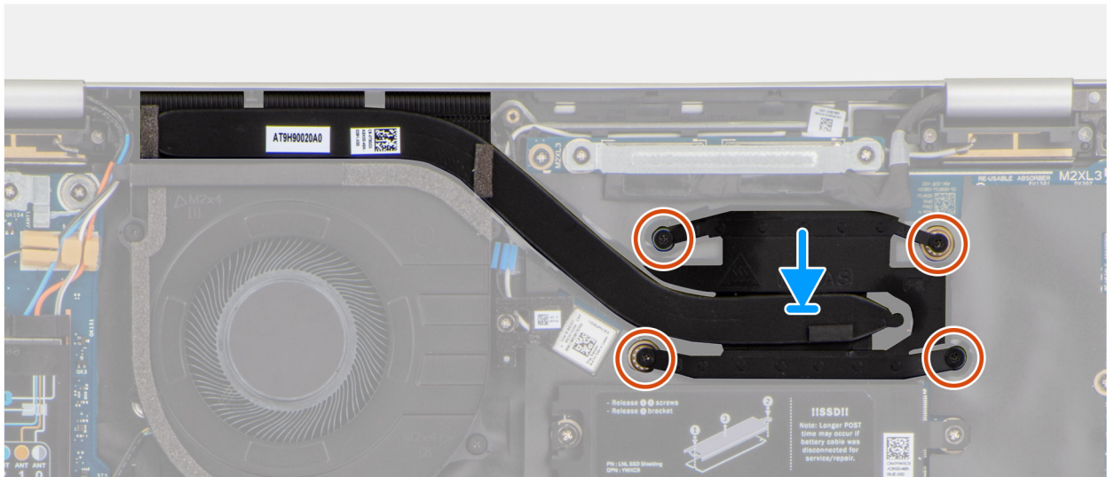
Abbildung 42. Installieren des Kühlkörpers
