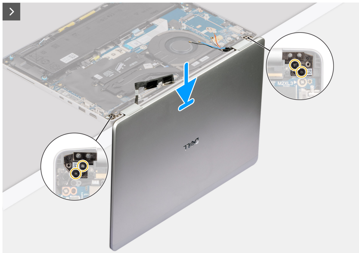
Abbildung 59. Einbauen der Displaybaugruppe
