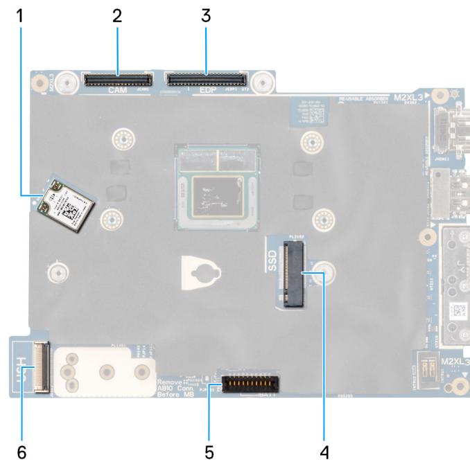
Abbildung 49. Anschlüsse auf der Hauptplatine
