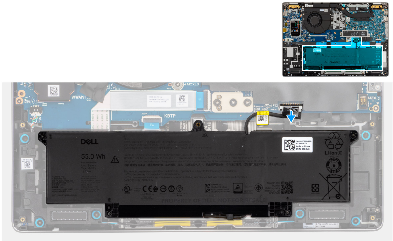
Abbildung 24. Trennen des Akkukabels
