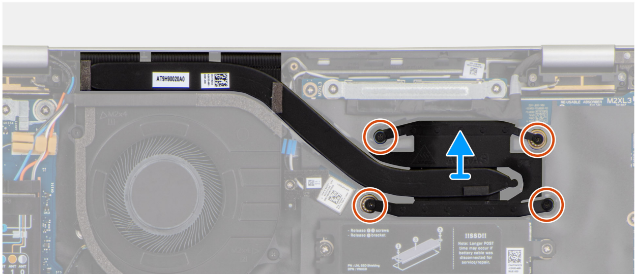
Abbildung 41. Entfernen des Kühlkörpers
