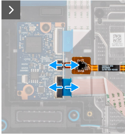
Abbildung 43. Entfernen der USH-Platine
