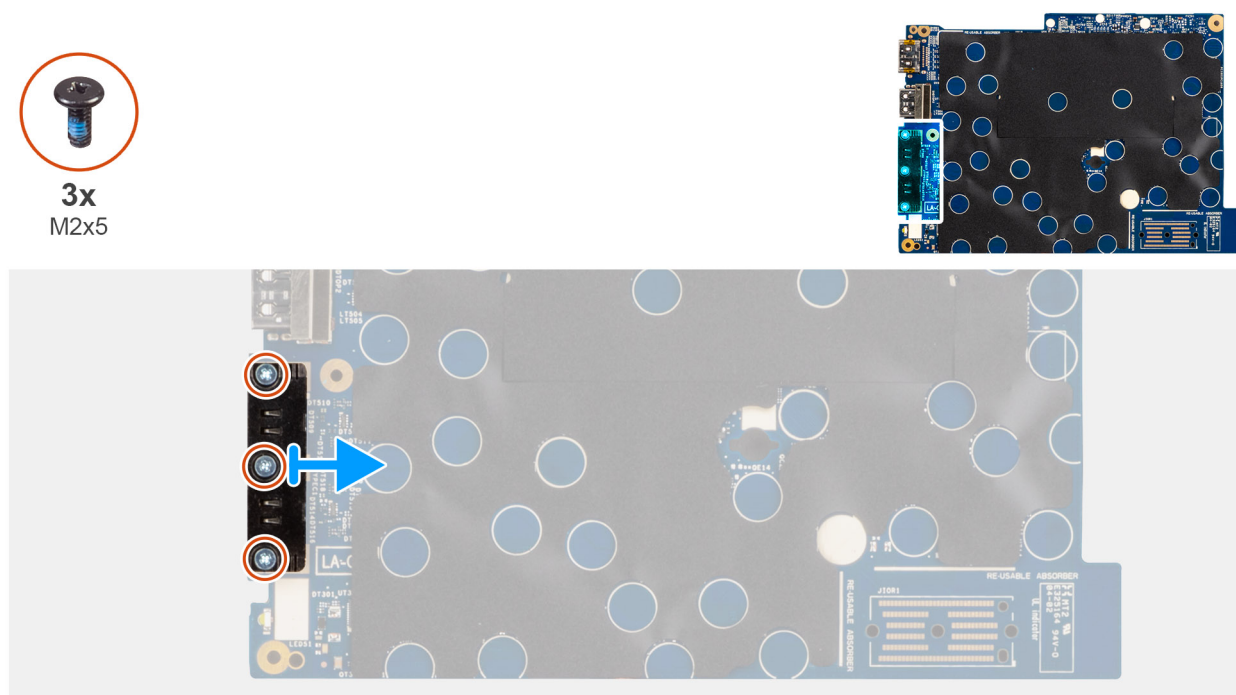
Abbildung 51. Entfernen des USB-Typ-C-Anschlussmoduls
