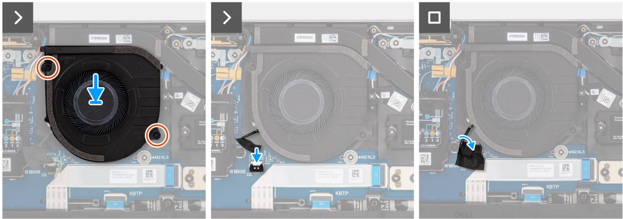
Abbildung 40. Installieren des Lüfters
