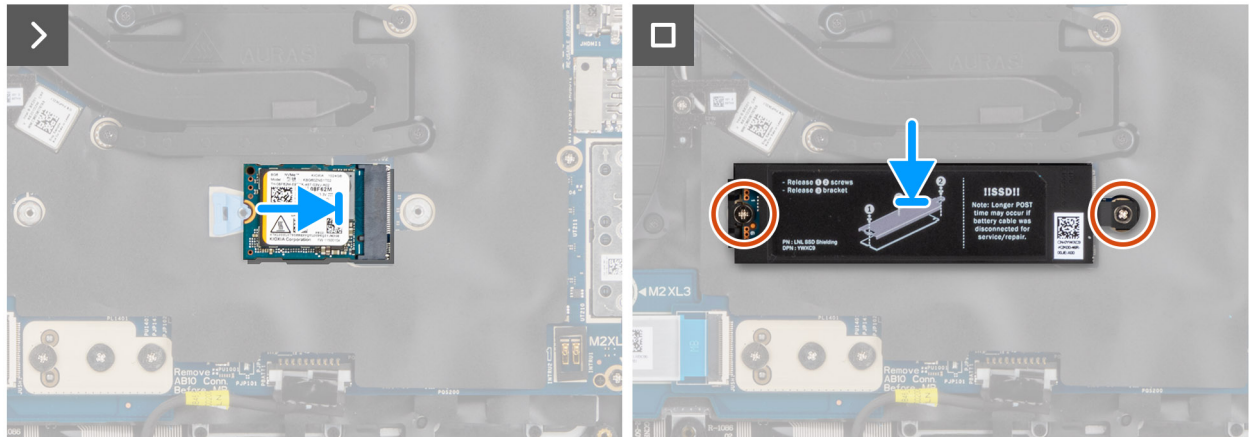
Abbildung 34. Einbauen des M.2-2280-SSD
