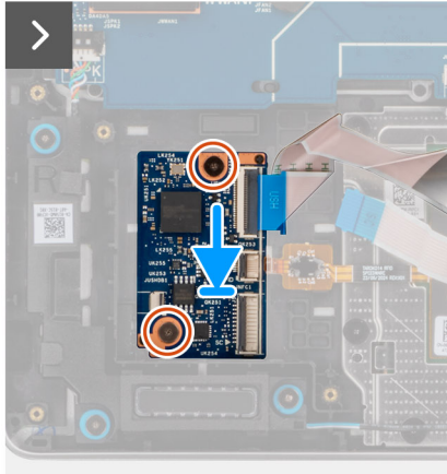
Abbildung 44. Einbauen der USH-Platine
