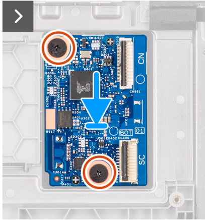
Abbildung 38. Einsetzen der USH-Platine
