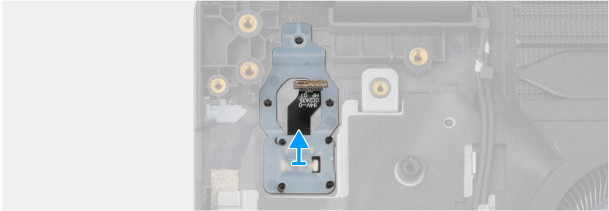
Abbildung 55. Entfernen des Netzschalters mit Fingerabdruck-Lesegerät
