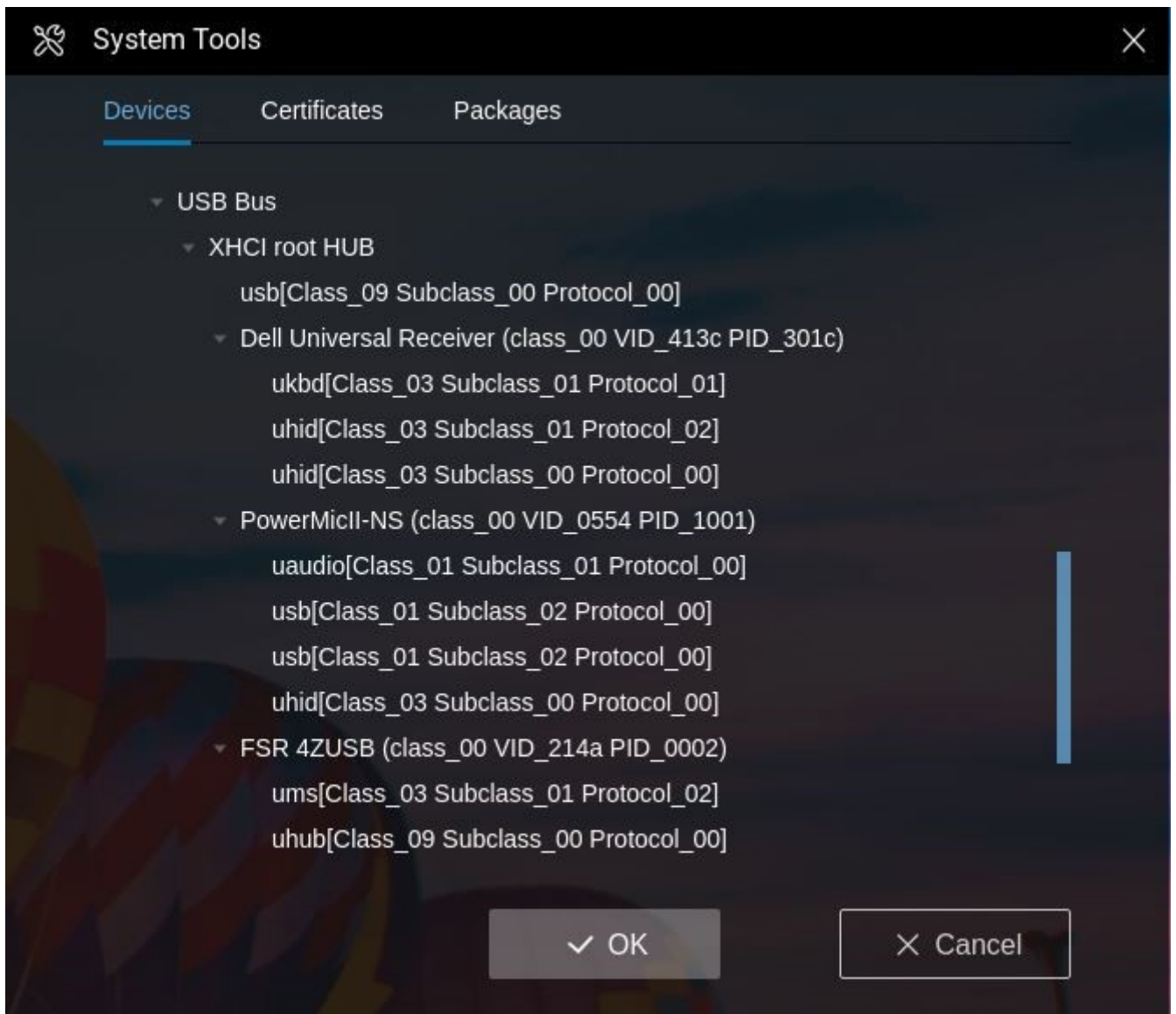
Figure 29. VID and PID
