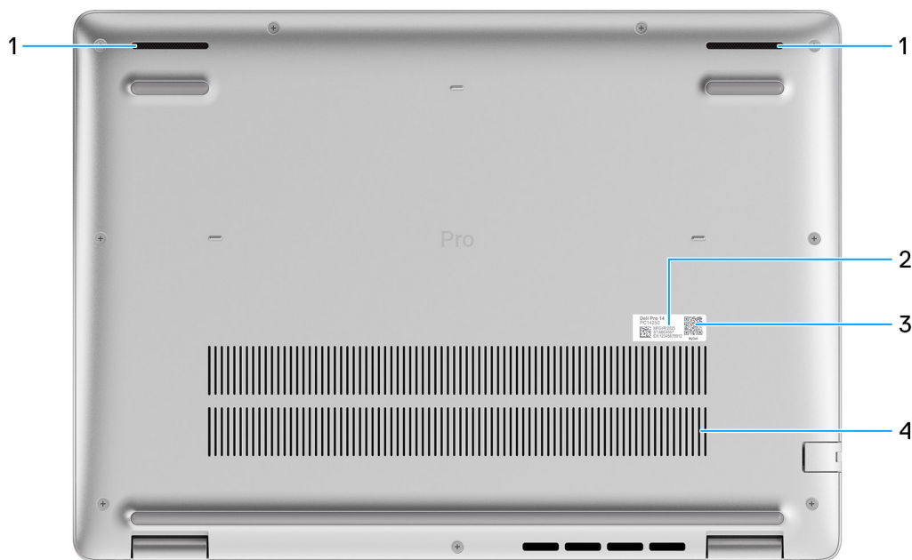
Figure 5. Vue du dessous
