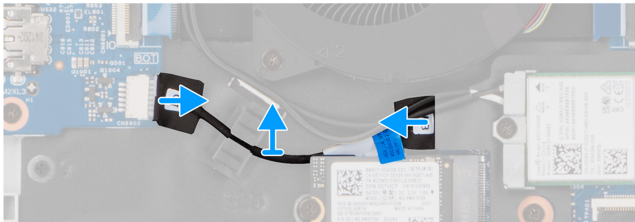
Figure 45. Retrait du câble vPro
