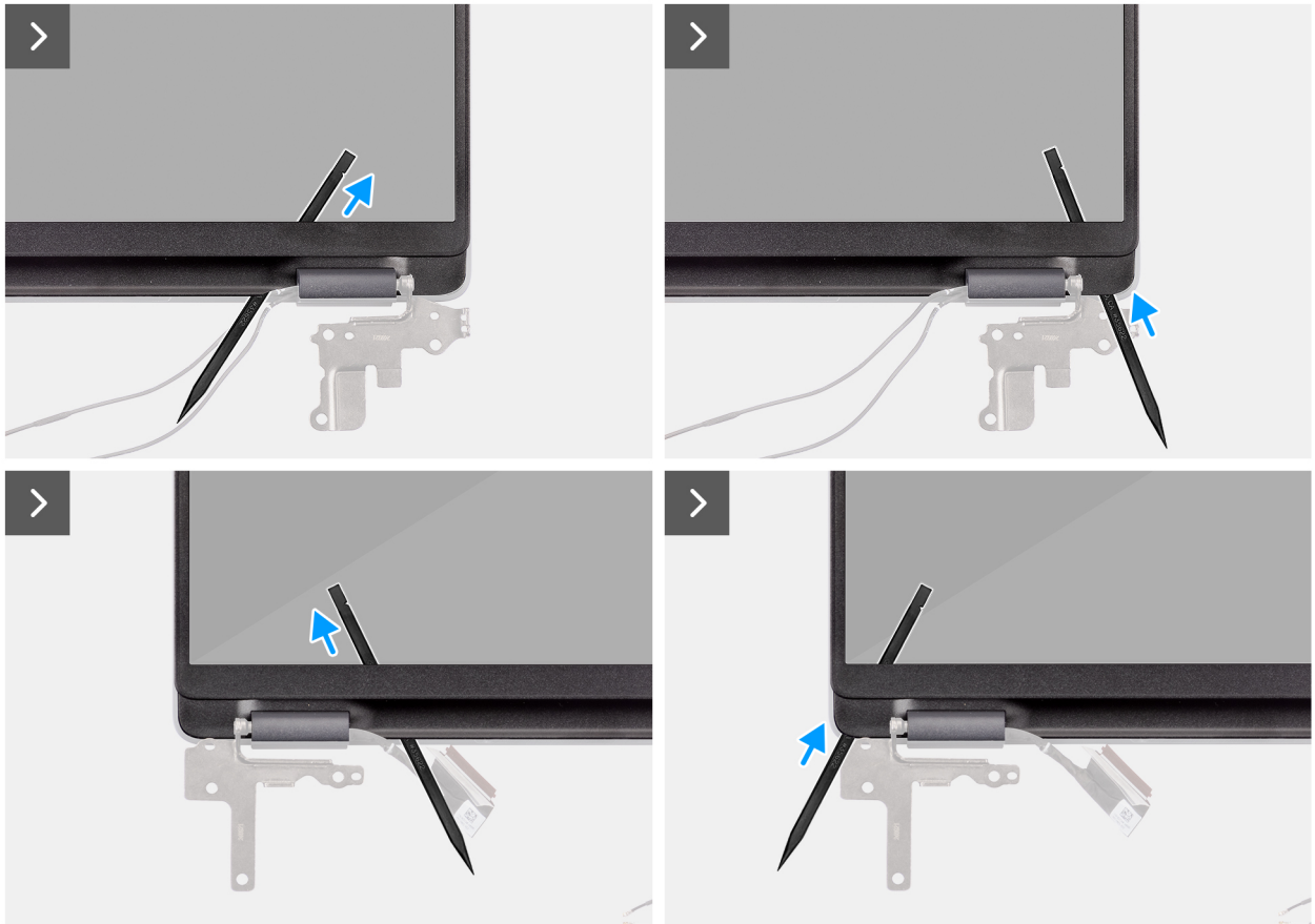
Figure 106. Retrait de la bordure d'écran
