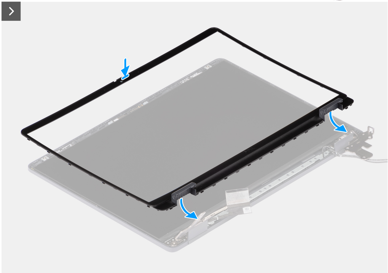
Figure 109. Installation de la bordure d'écran
