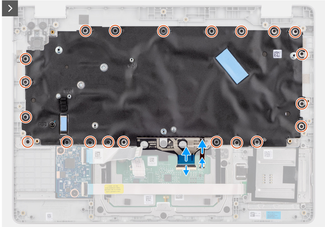
Figure 85. Retrait du clavier
