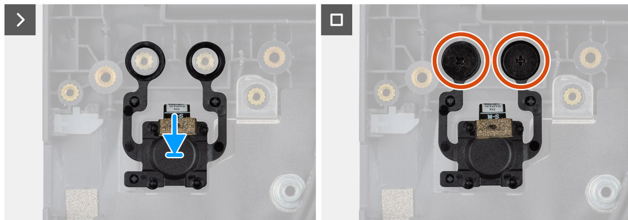
Figure 56. Installation du bouton d'alimentation avec lecteur d'empreintes digitales
