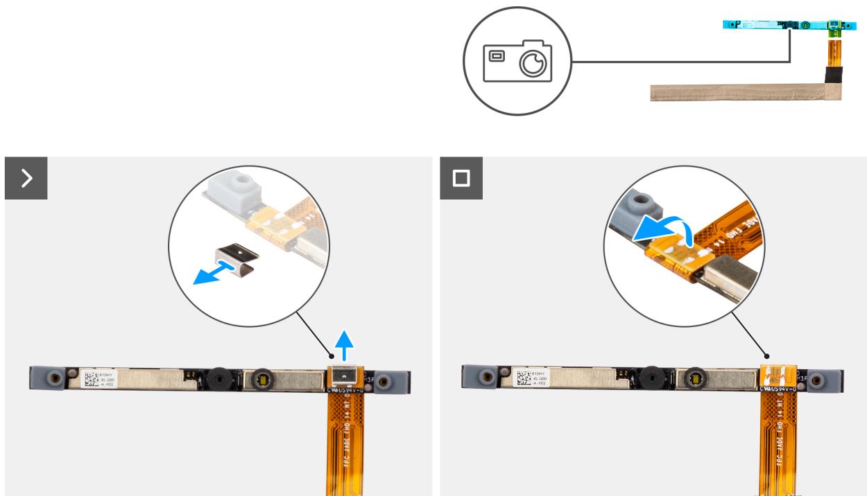
Figure 119. Retrait de la caméra
