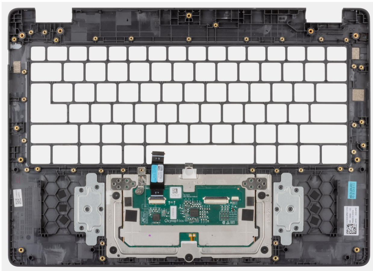
Figure 95. Retrait du repose-poignets et de l'assemblage
