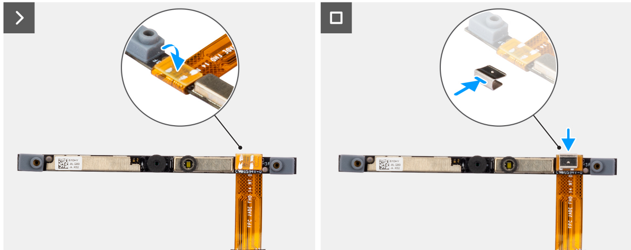
Figure 120. Installation de la caméra
