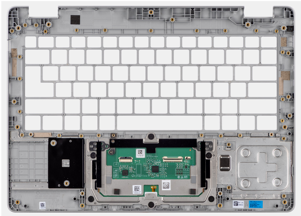
Figure 97. Retrait du repose-poignets et de l'assemblage
