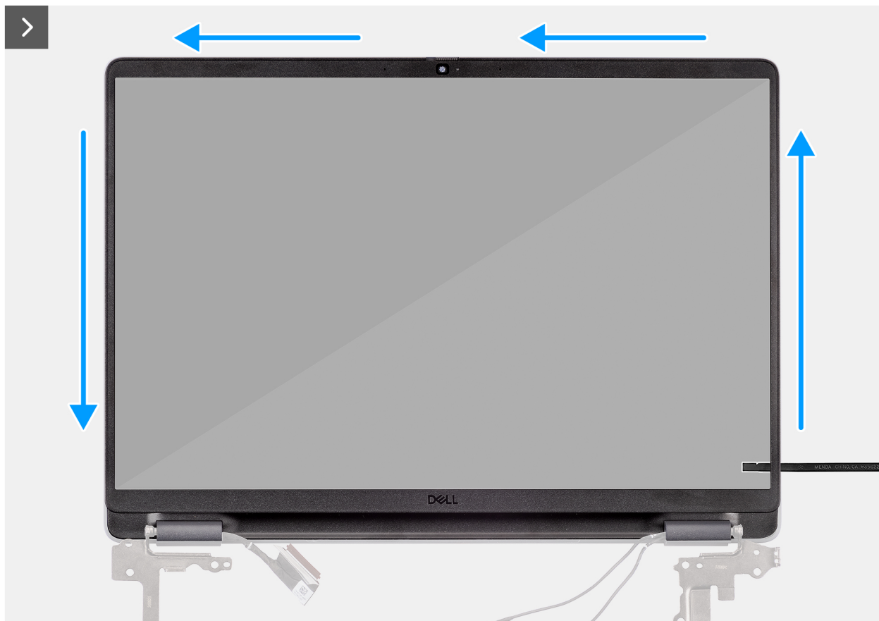
Figure 107. Retrait de la bordure d'écran
