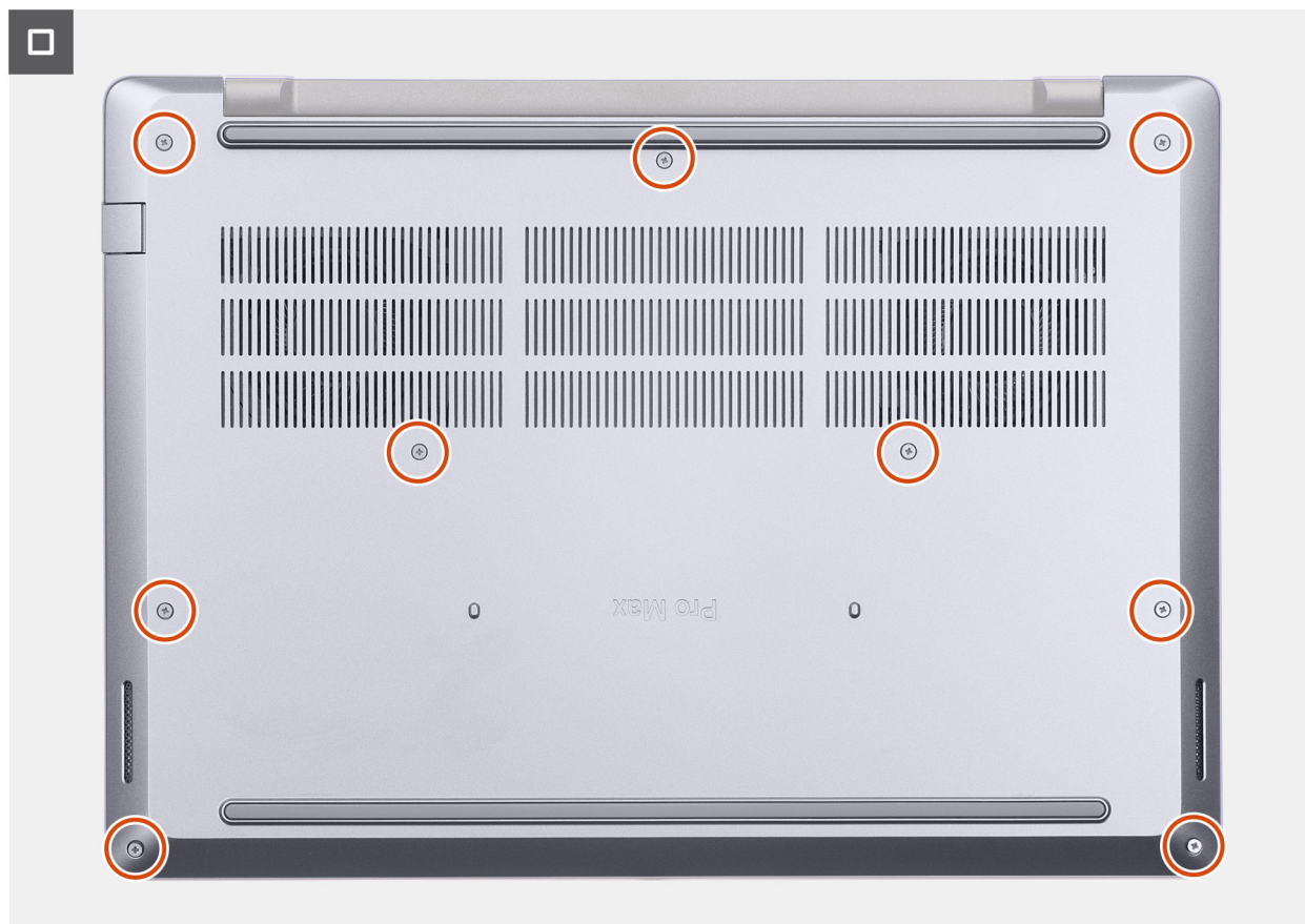
Figur 16. Installera kåpan
