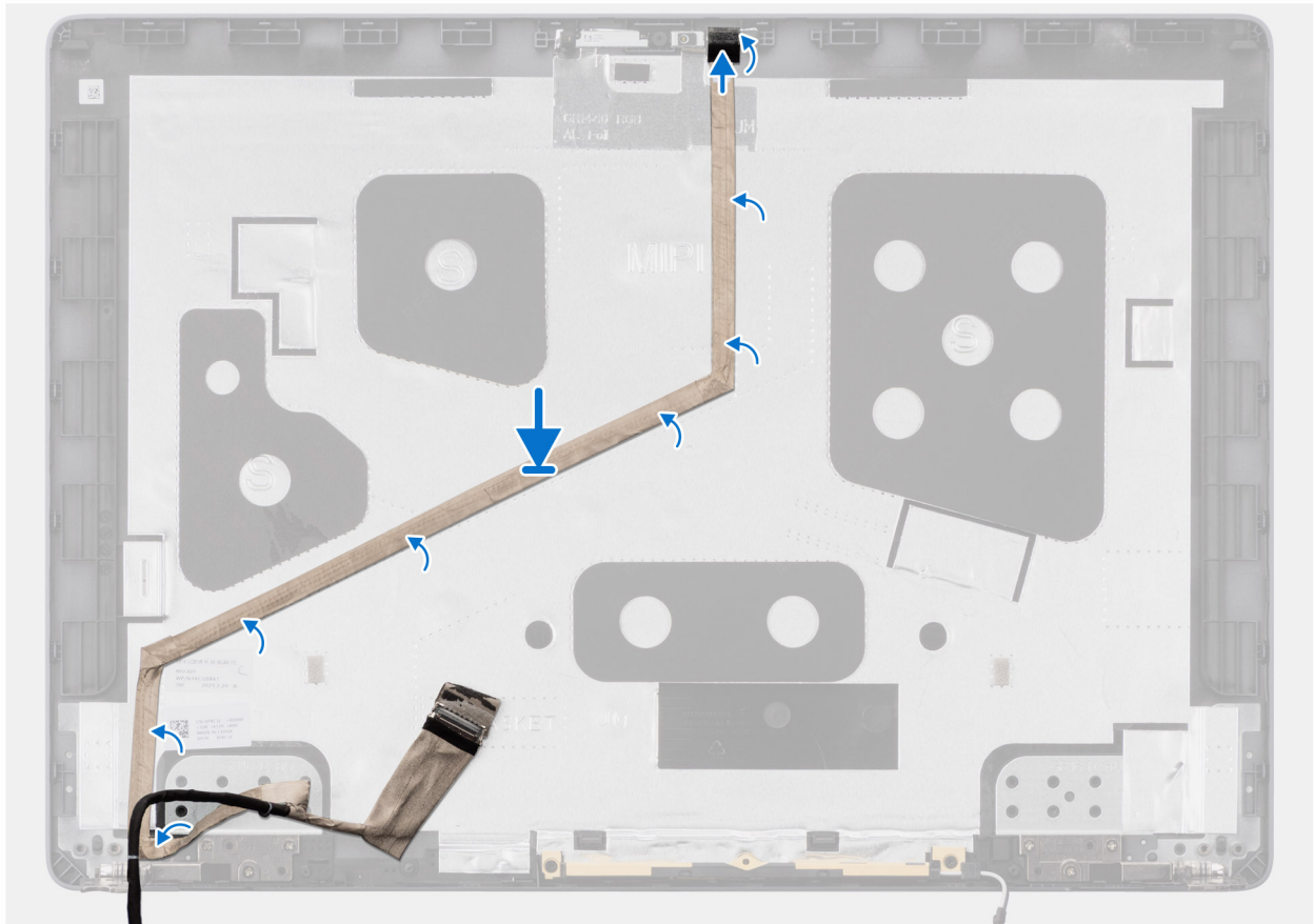
Figur 68. Installera bildskärmskabeln
