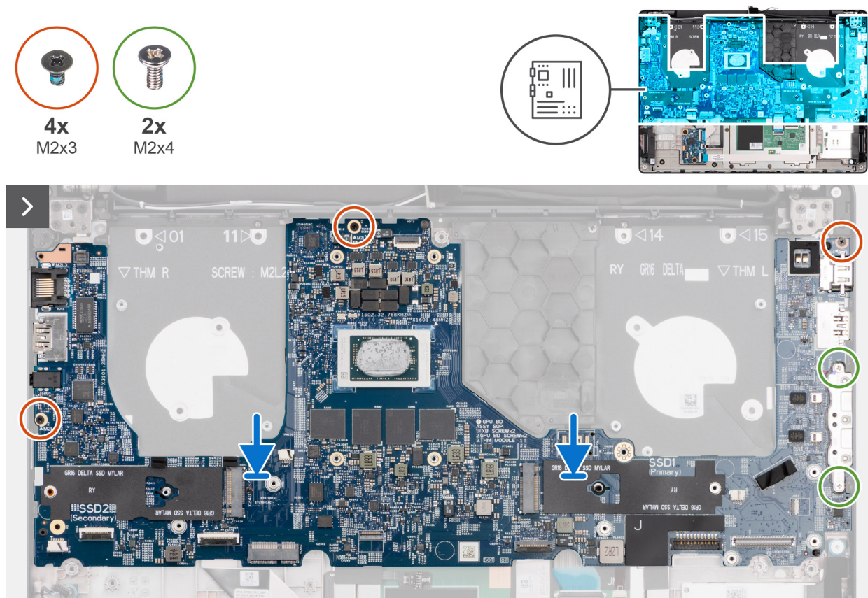
Figur 77. Installera moderkortet
