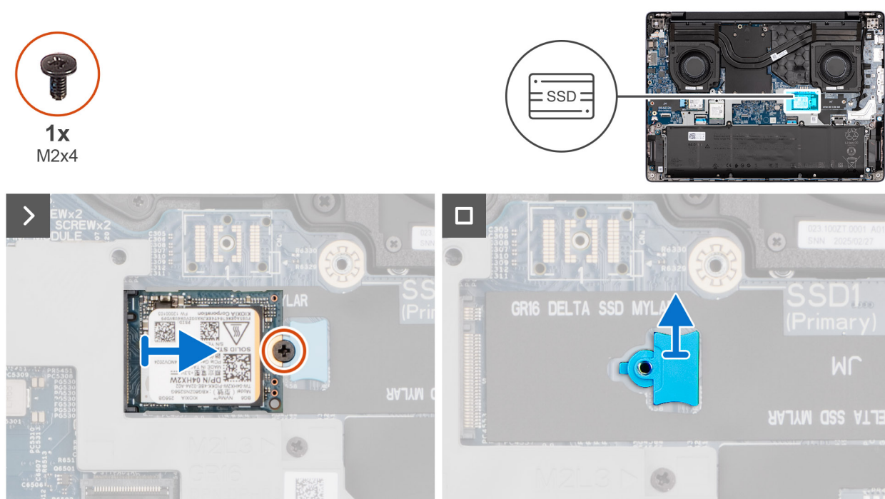
Figur 21. Ta bort M.2 2230 SSD-disken
