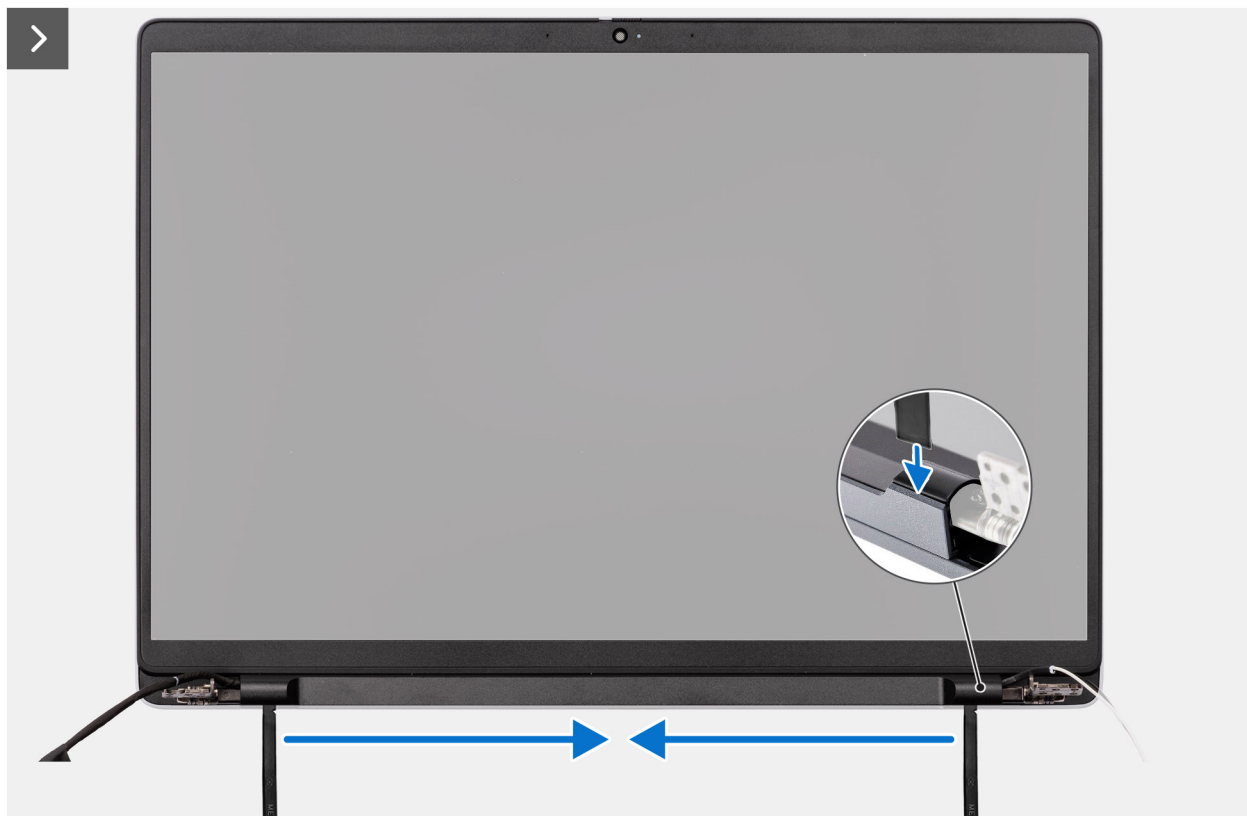
Figur 53. Ta bort bildskärmsramen
