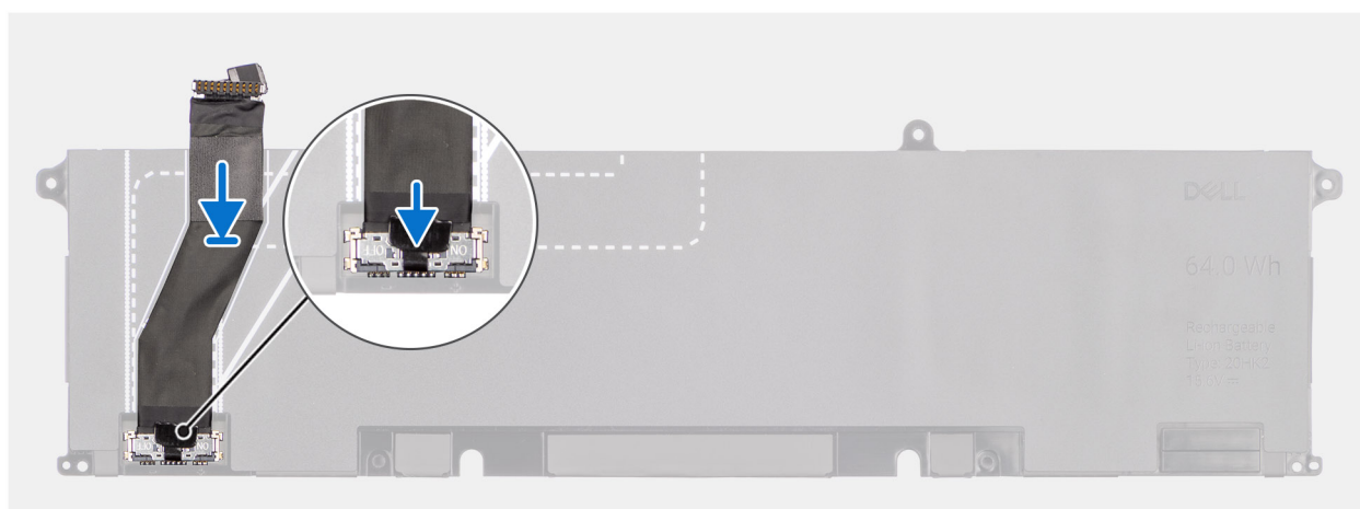
Figur 20. Ansluta batterikabeln
