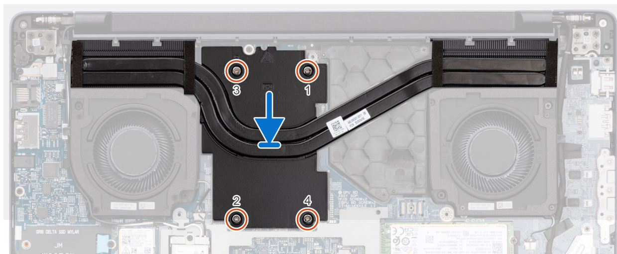
Figur 35. Installera kylflänsen
