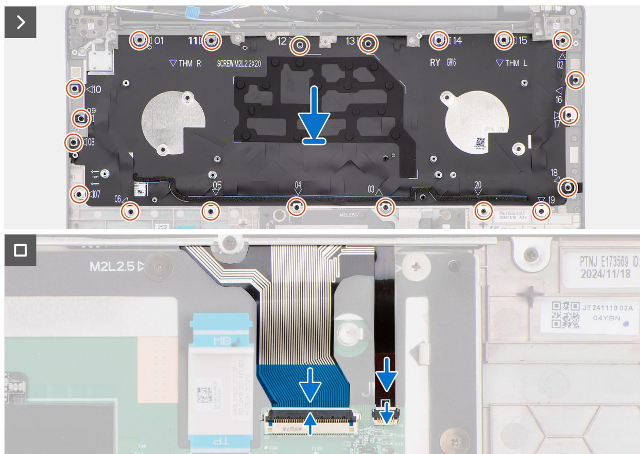
Figur 86. Installera tangentbordet
