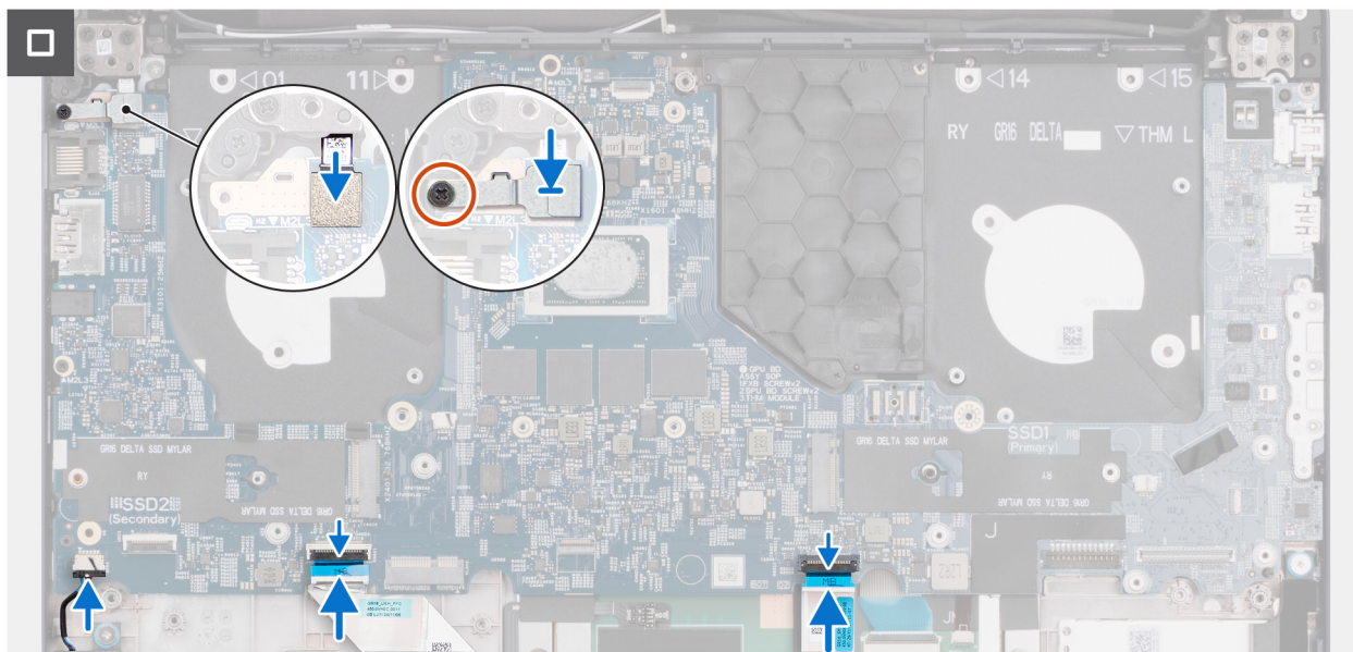
Figur 78. Installera moderkortet
