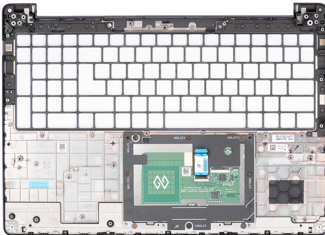
Figur 87. Handledsstöd
