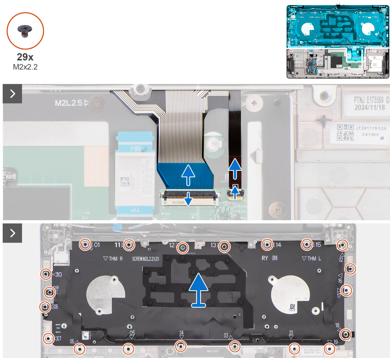
Figur 83. Ta bort tangentbordet
