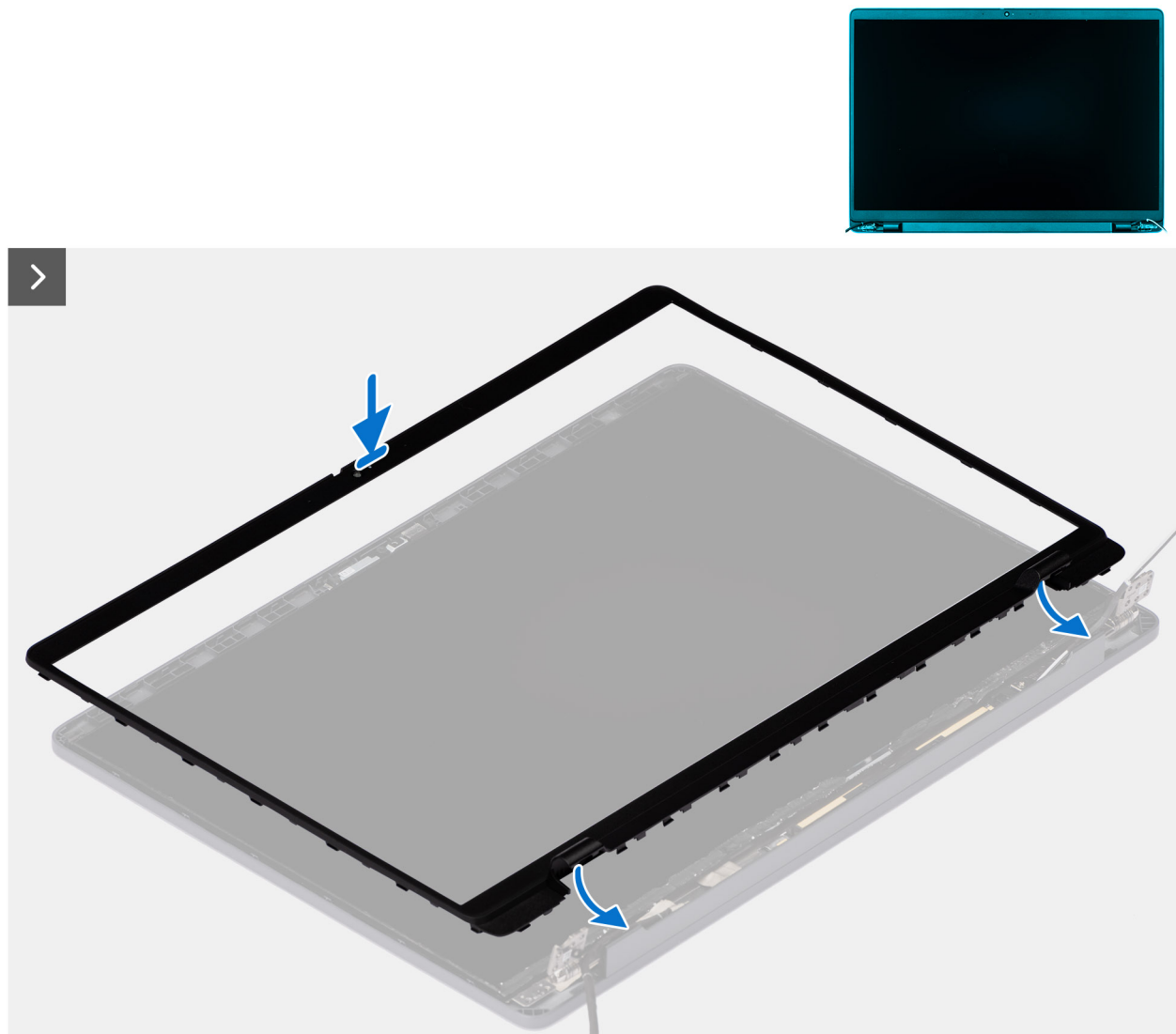
Figur 56. Installera bildskärmsramen
