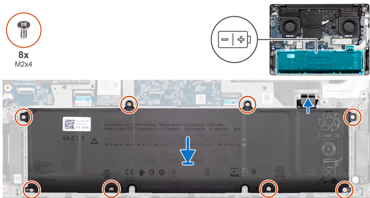
Figur 18. Installera batteriet
