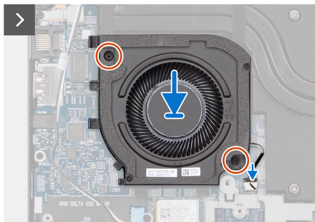
Figur 31. Installera den högra processorfläkten/processorfläkten
