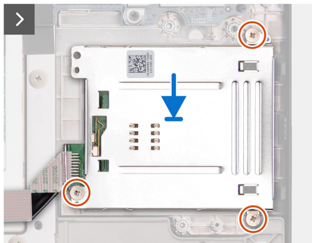
Figur 43. Installera smartkortläsaren
