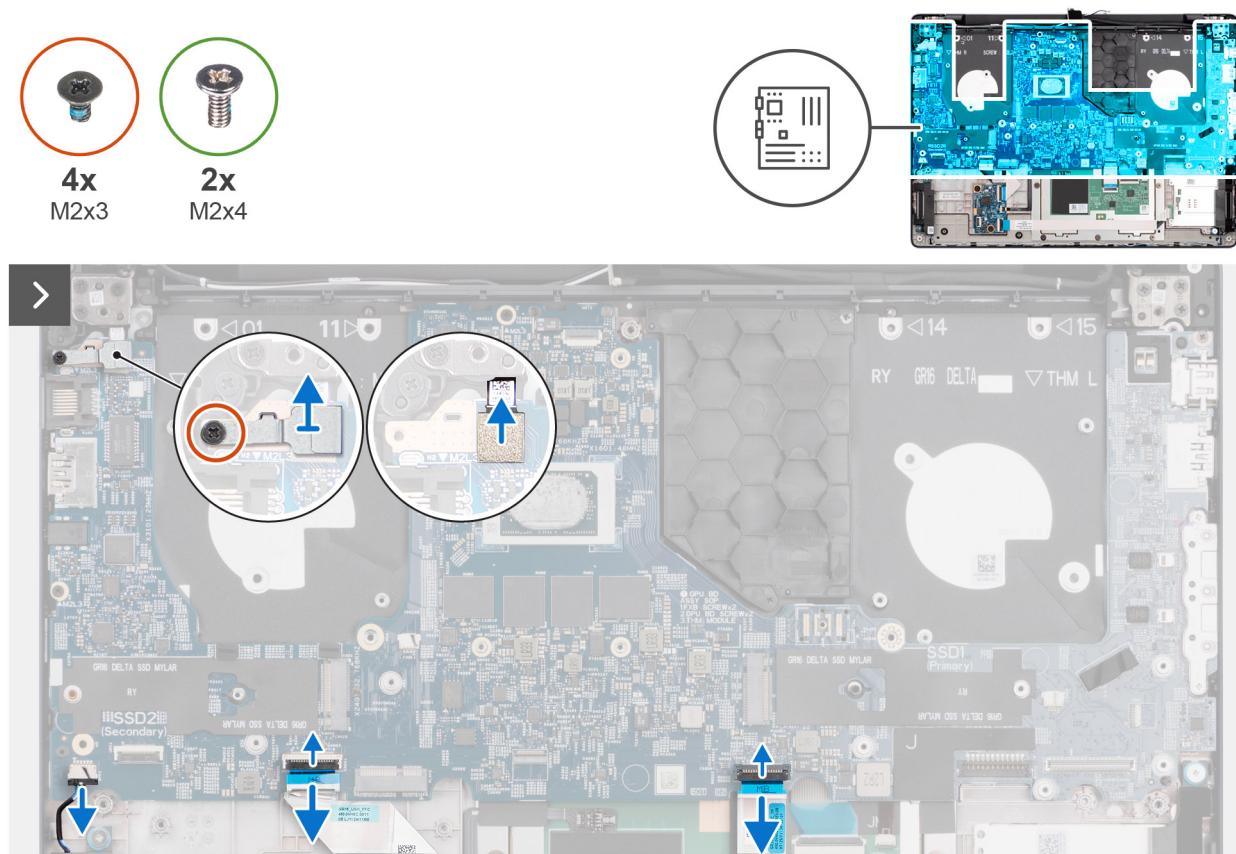
Figur 74. Ta bort systemkort
