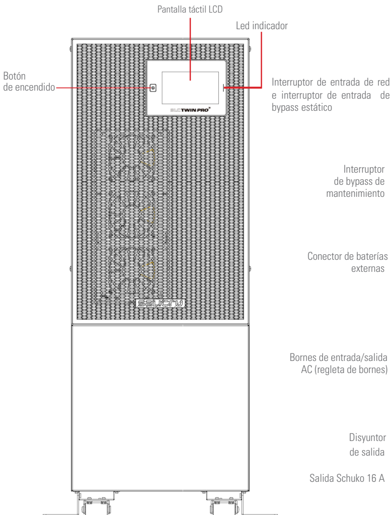
Fig. 1. Vista frontal de la serie SLC TWIN PRO3 10, 15 y 20 kVA.
