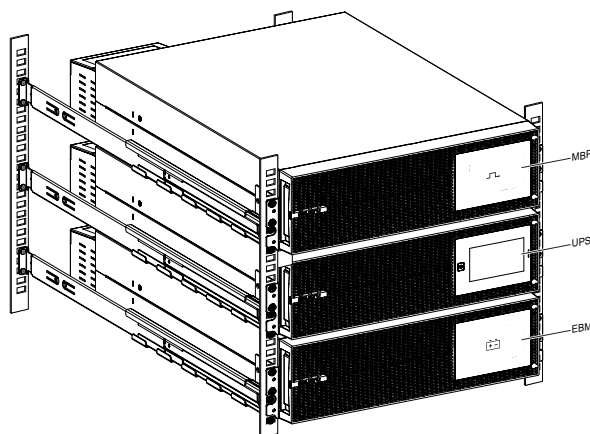
Fig. 21. Instalación del SAI y del módulo de baterías en el armario rack.
