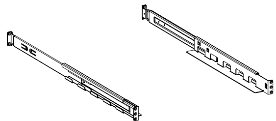
Fig. 18. Installation des supports sur le module onduleur.
