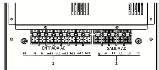
Fig. 26. Terminales de entrada/salida del SLC TWIN PRO3.
