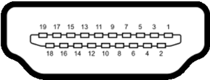
Afbeelding 8. HDMI-poort
