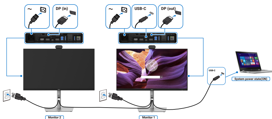
Rysunek 51. Podłączanie monitora w konfiguracji USB-C MST (Multi-Stream Transport) – włączanie
