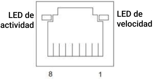
Figura 13. Puerto RJ45 (lado del conector)
